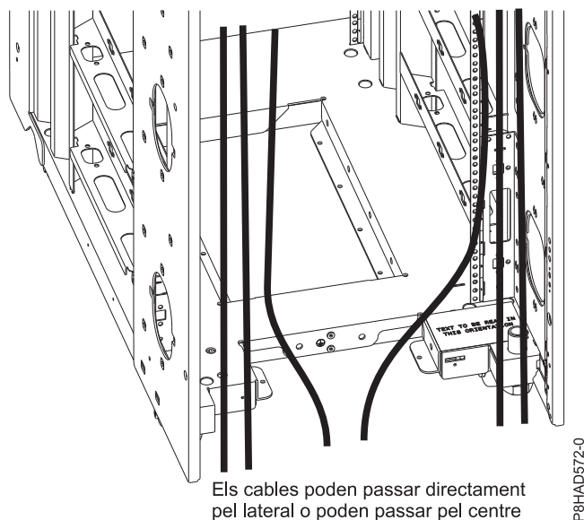
Figura 37. Cablatge per sota del terra
