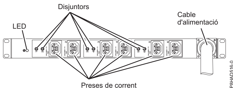
Figura 49. PDU HVDC
