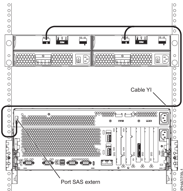
Figura 62. Un port d'adaptador SAS extern del sistema a un calaix d'expansió de discos
