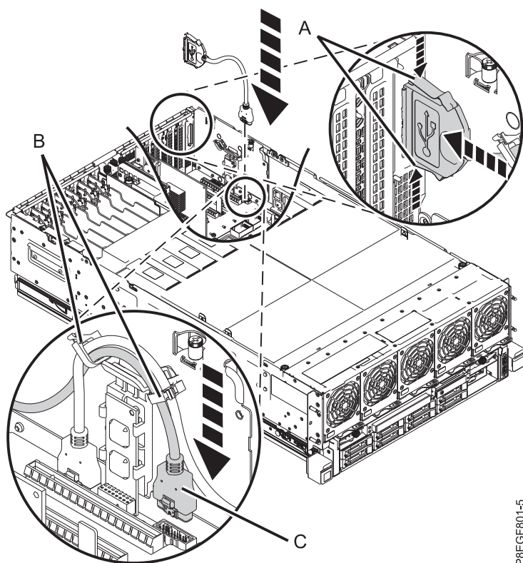
Figura 3. Substitució del cable posterior USB
