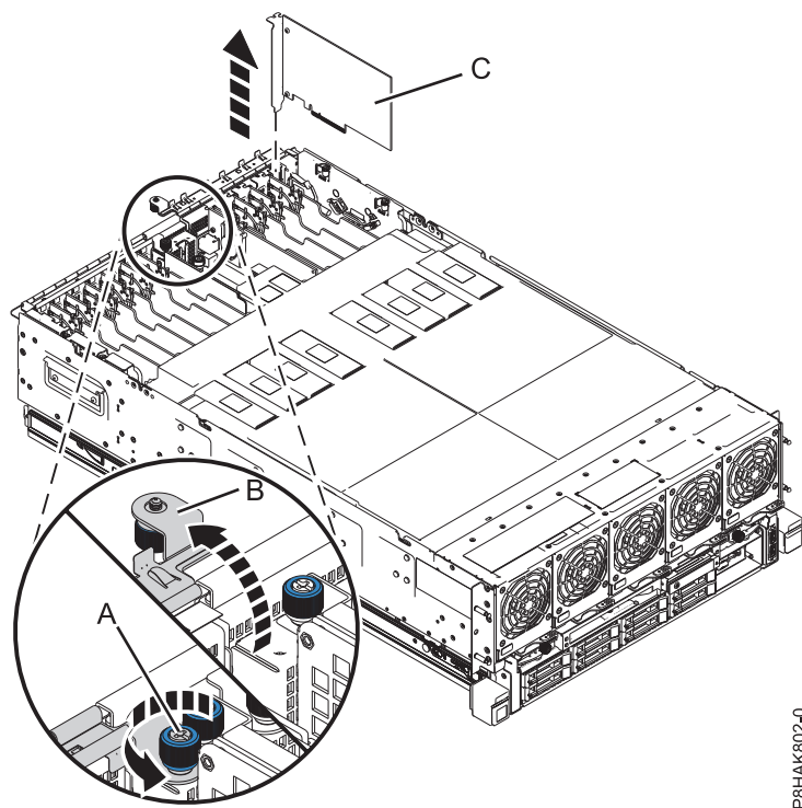
Figura 1. Extracció d'un adaptador PCIe
