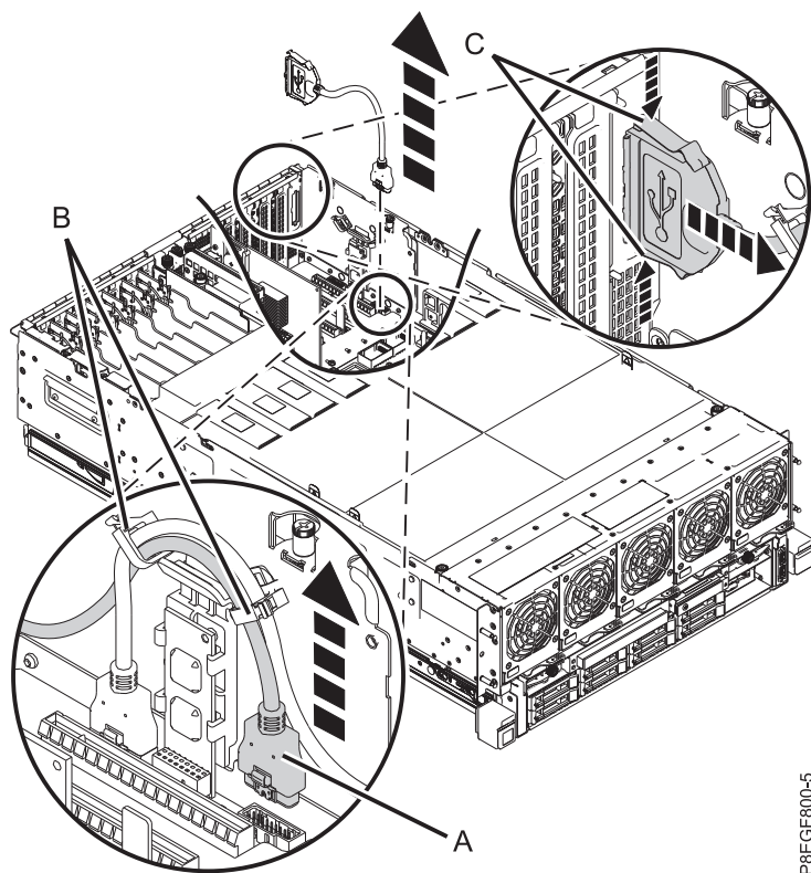
Figura 2. Extracció del cable posterior USB
