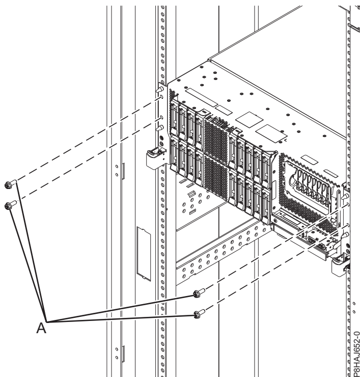
Figura 28. Extracció dels cargols frontals
