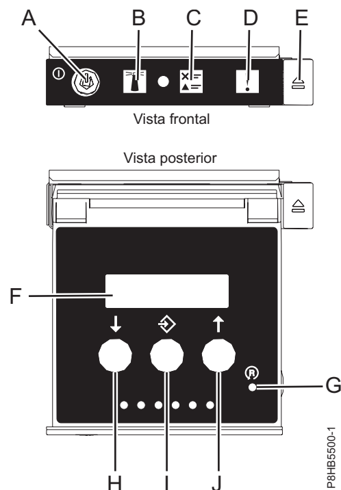
Figura 4. Tauler de control
