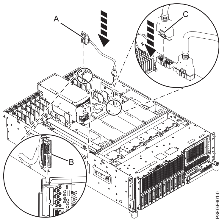
Figura 3. Substitució del cable posterior USB
