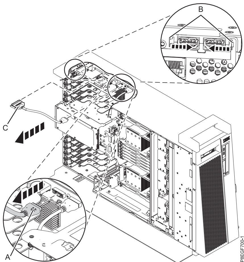
Figura 2. Extracció del cable posterior USB de la versió autònoma del model 8286-41A
