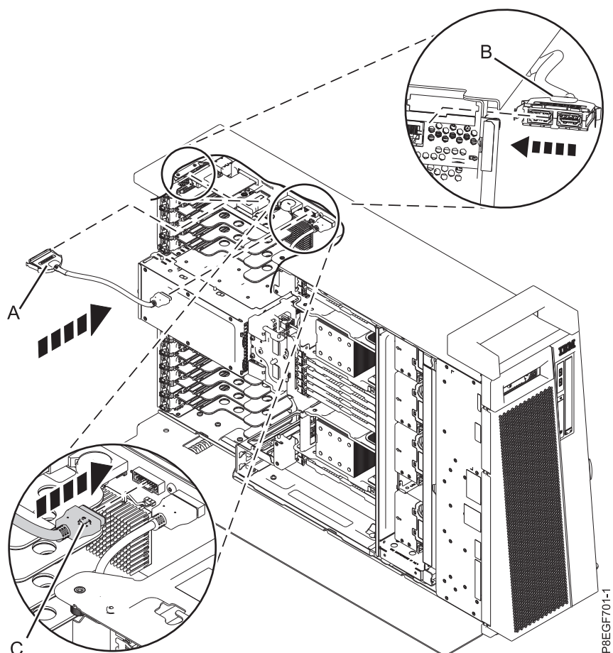
Figura 4. Substitució del cable posterior USB a la versió autònoma del model 8286-41A
