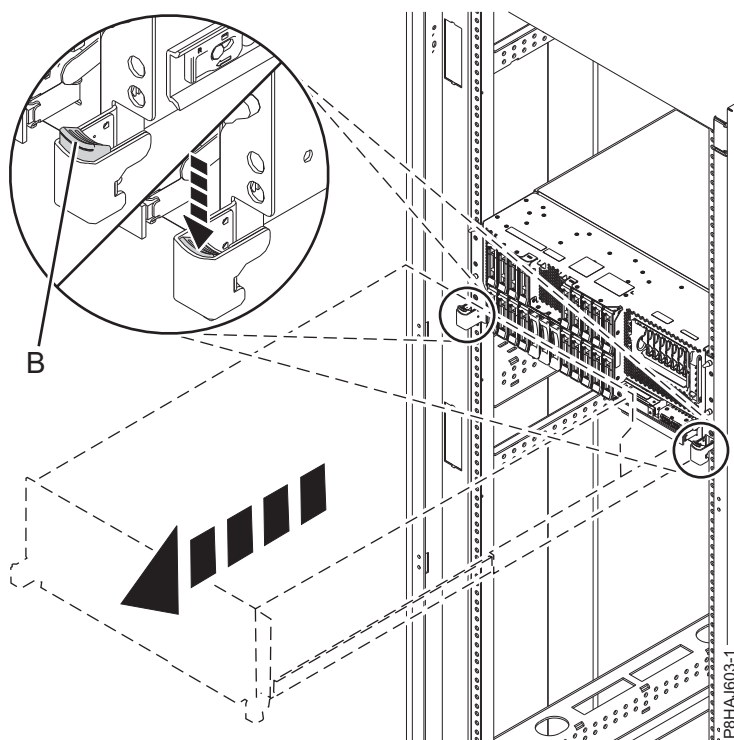
Figura 33. Alliberament dels pestells laterals
