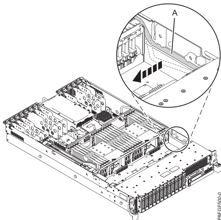
Figura 2. Com treure el cable USB del canal de cables
