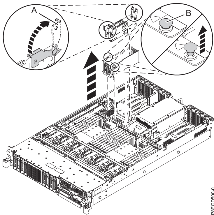
Figura 1. Extracció del receptacle i de les targetes del mòdul d'alimentació de reserva
