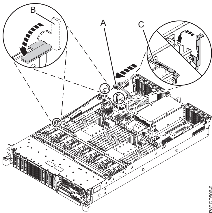
Figura 6. Substitució del cable posterior SAS de la part inferior a la ranura P1-C14
