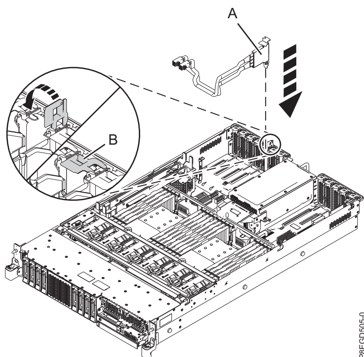
Figura 5. Col·locació del cable posterior SAS
