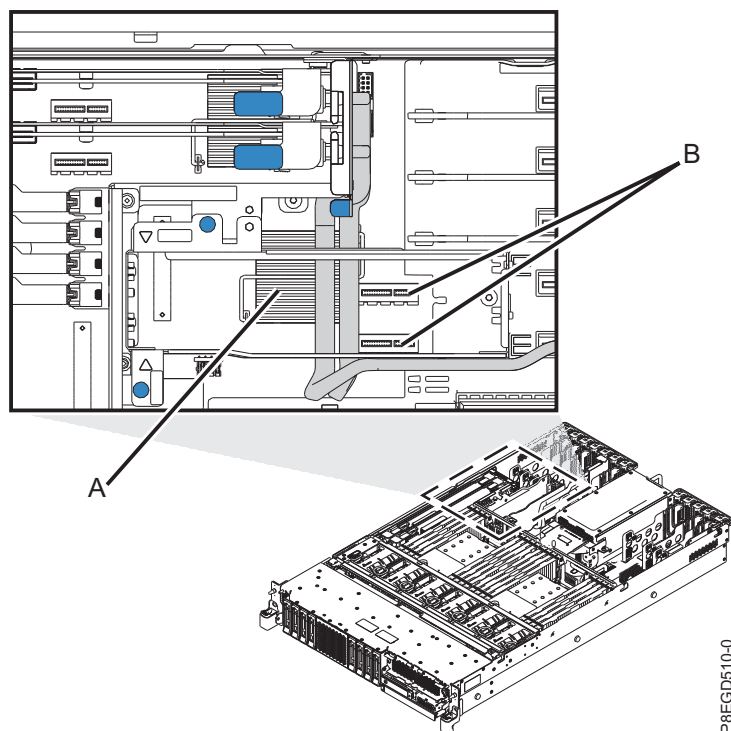
Figura 8. Com fer passar els cables posteriors SAS
