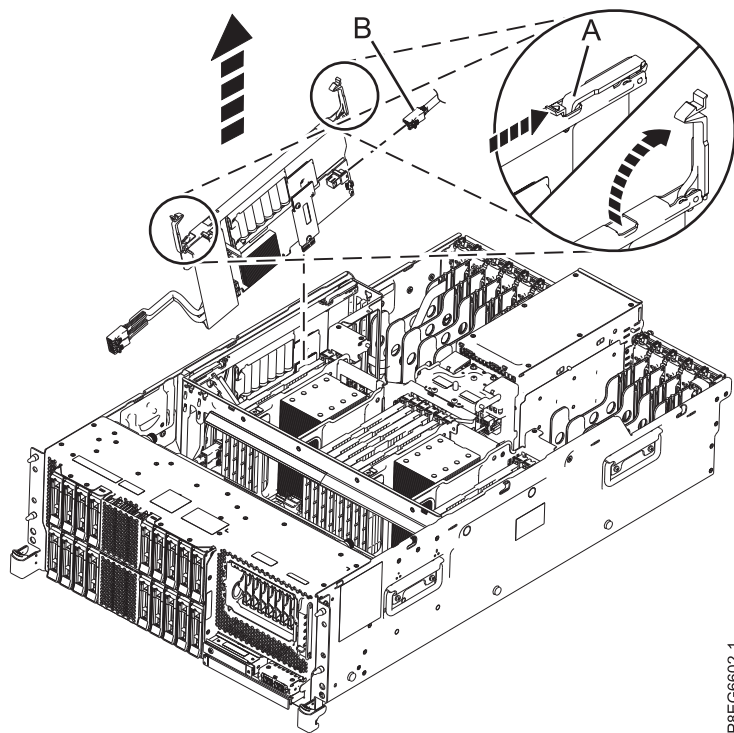
Figura 3. Extracció de l'adaptador intern SAS RAID de la ranura P1-C15
