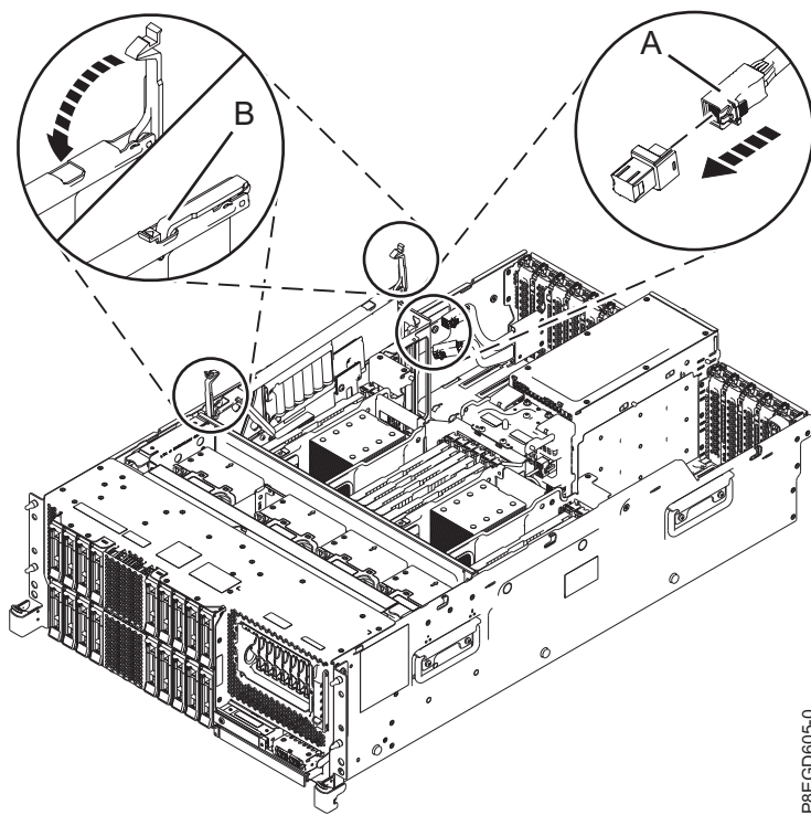
Figura 7. Substitució del cable posterior SAS a la ranura P1-C14
