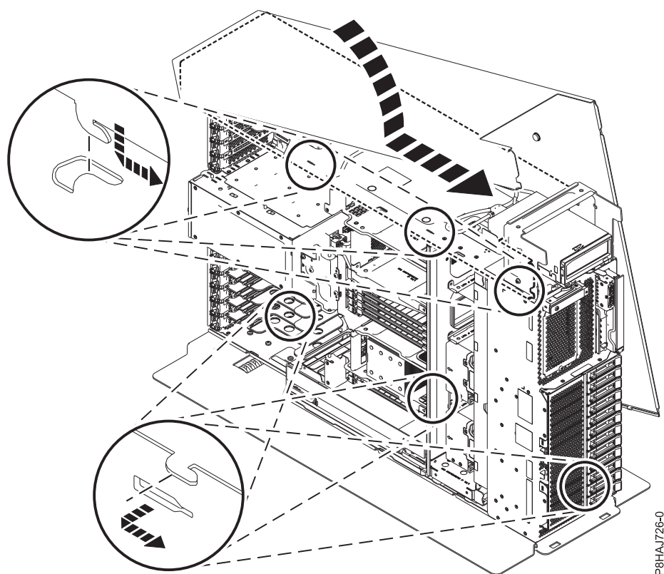
Figura 27. Instal·lació de la coberta lateral del model 8286-41A
