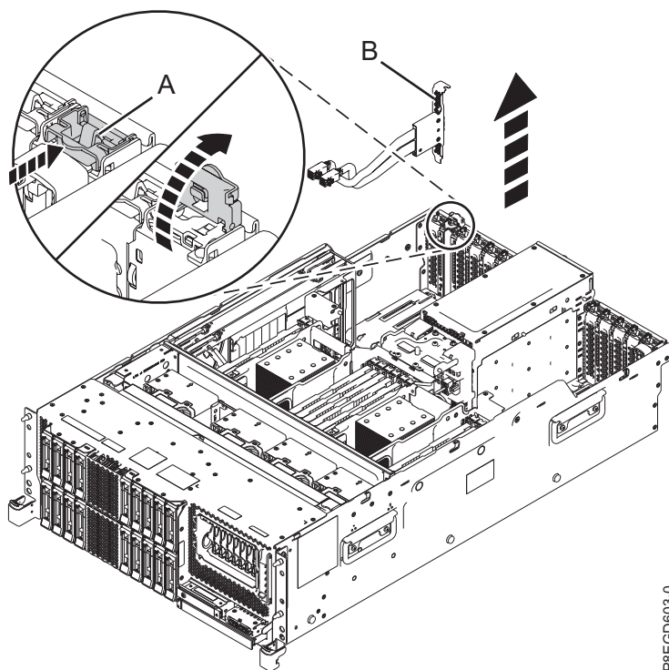
Figura 5. Extracció del cable posterior SAS
