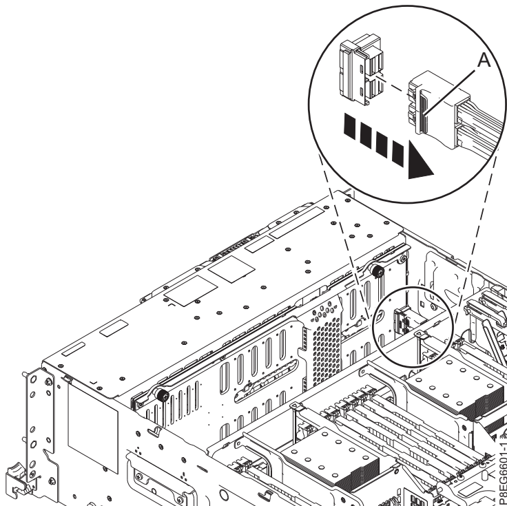
Figura 2. Com desendollar el cable SAS de la placa posterior de la unitat de disc
