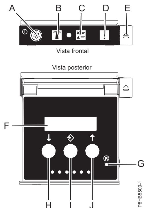
Figura 13. Tauler de control
