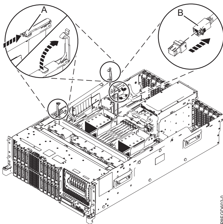
Figura 4. Extracció del cable posterior SAS de la ranura P1-C14
