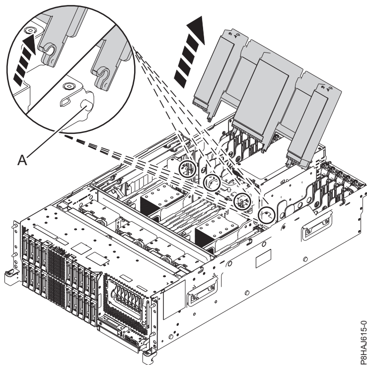
Figura 35. Extracció del deflector d'aire
