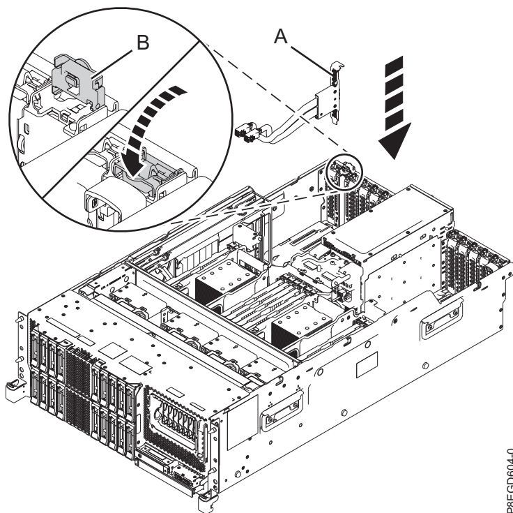
Figura 6. Col·locació del cable posterior SAS
