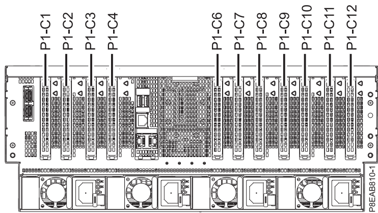
Figura 1. Vista posterior d'un sistema 8408-44E o 8408-E8E amb els codis d'ubicació de ranures de l'adaptador PCIe
