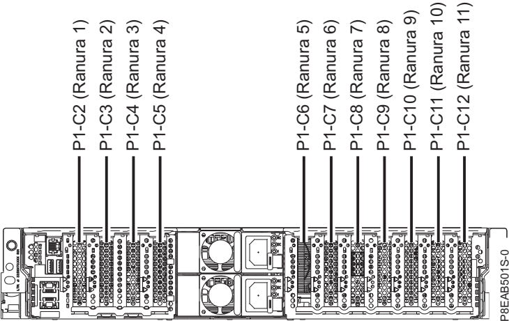
Figura 1. Vista posterior d'un sistema 5148-21L, 5148-22L, 8247-21L, 8247-22L, 8284-21A, o 8284-22A amb els codis d'ubicació de les ranures PCIe
