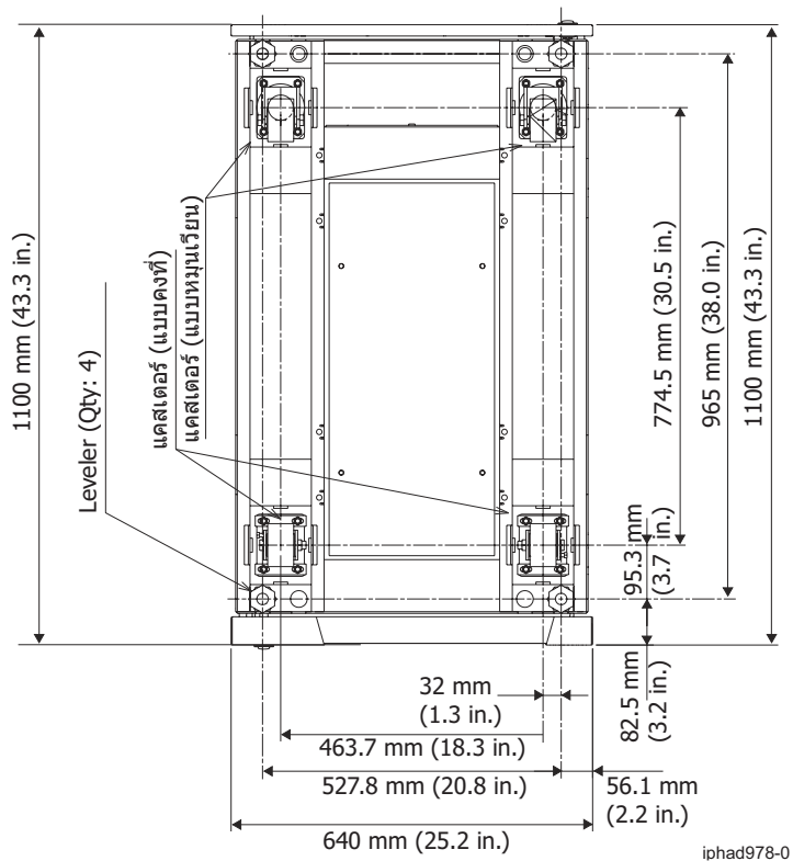
รูปที่ 4. ตำแหน่งลูกล้อและตัวปรับระดับ
