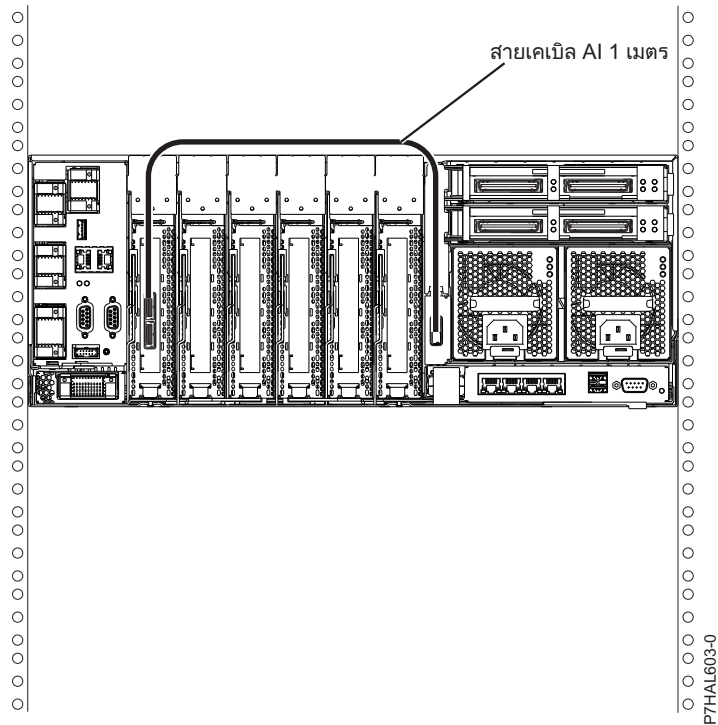
รูปที่ 147. จากอะแดปเตอร์ SAS ไปยังดิสก์สล็อต SAS ภายในผ่านทางพอร์ต SAS ภายนอกของระบบ
