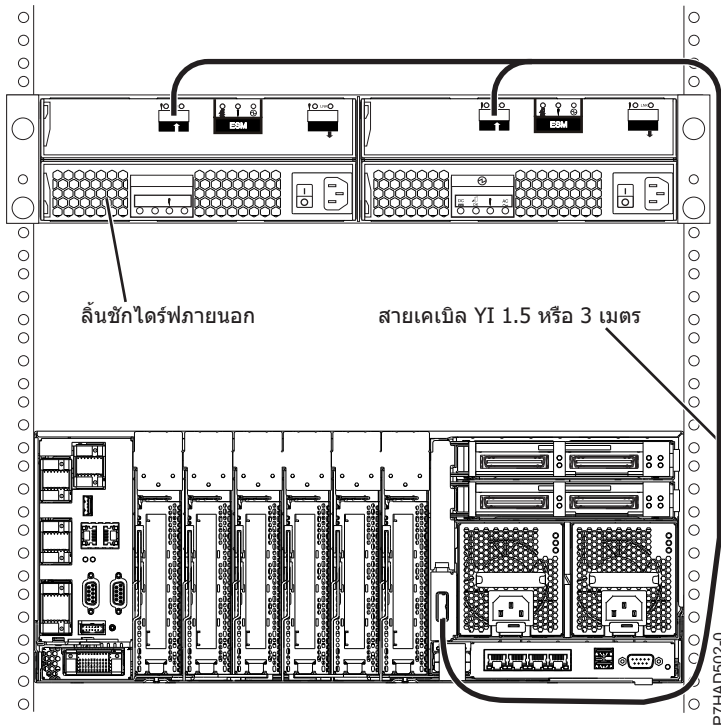
รูปที่ 146. พอร์ตอะแดปเตอร์ SAS ภายนอกของระบบกับลิ้นชักส่วนขยายดิสก์ (รุ่น 9117-MMB และ 9179-MHB)
