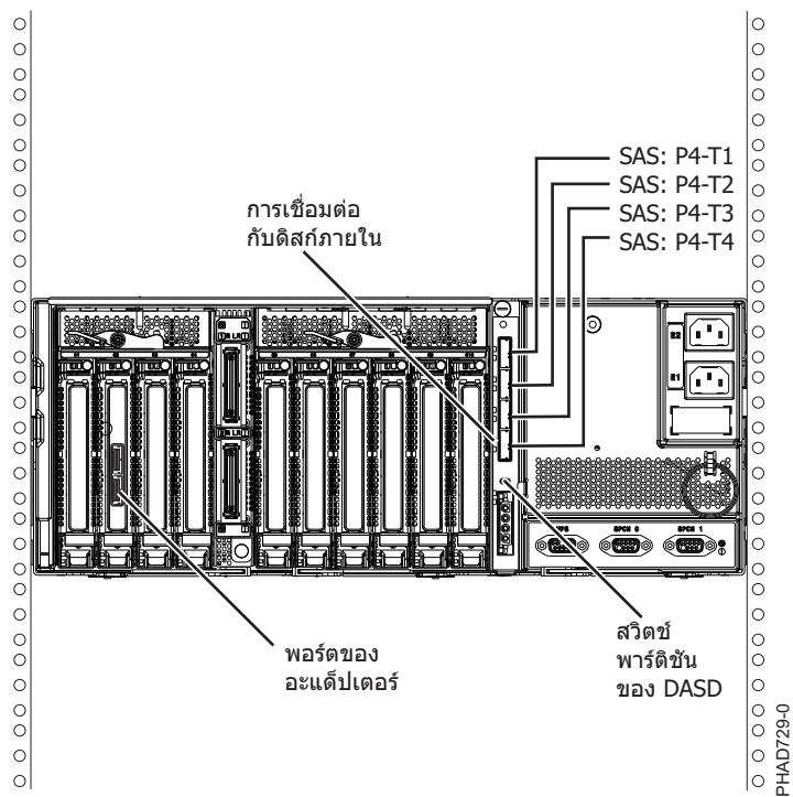
รูปที่ 163. จากอะแดปเตอร์ RAID SAS สองตัวไปยังลินซึกส่วนขยายดิสก์ในคอนฟิกูเรชันแบบ multi-initiator HA JBOD
