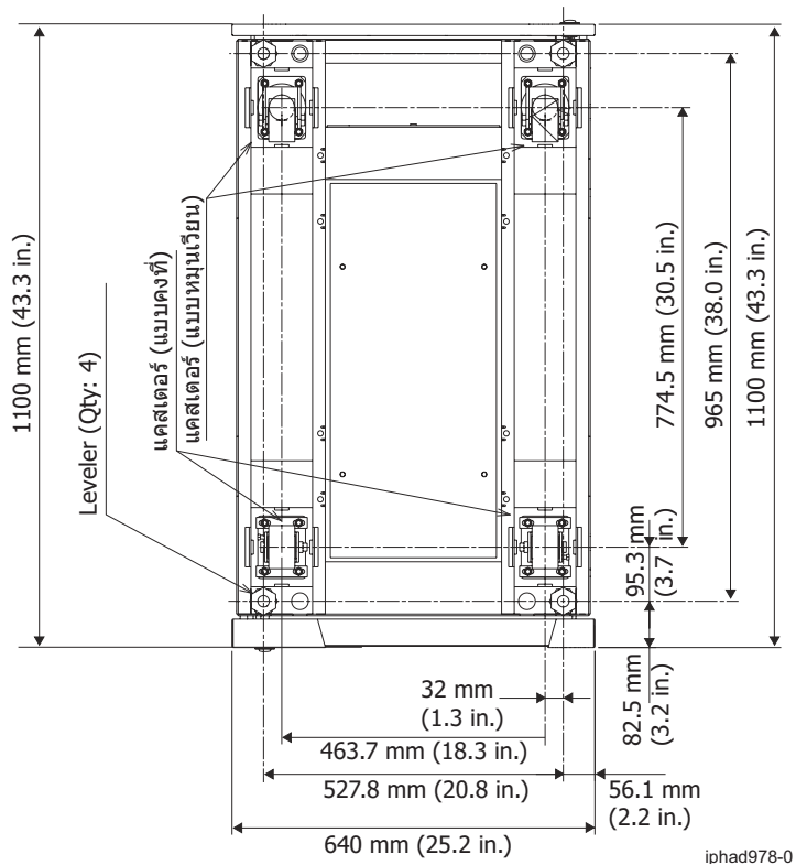
รูปที่ 26. ตำแหน่งลูกล้อและตัวปรับระดับ
