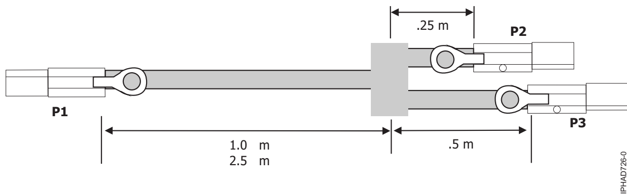
รูปที่ 144. ความยาวชุดสายเคเบิล SAS YI ภายนอก
