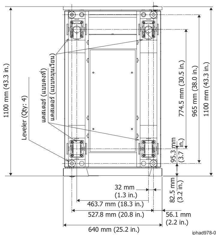
รูปที่ 9. ตำแหน่งลูกล้อและตัวปรับระดับ
