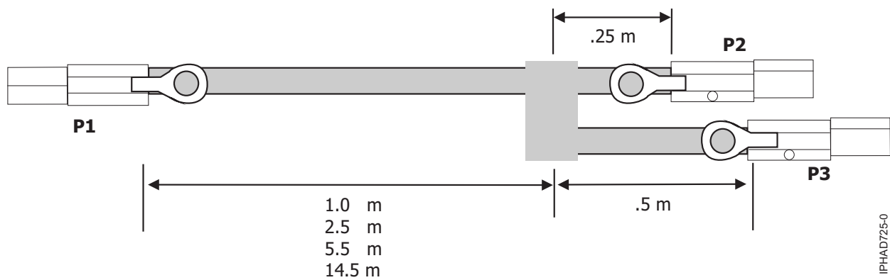
รูปที่ 143. ความยาวชุดสายเคเบิล SAS YO ภายนอก
