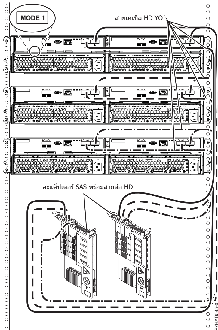
รูปที่ 175. การเชื่อมต่อโหมด 1 ของสามลิ้นชัก 5887 เข้ากับ สองอะแดปเตอร์ SAS ด้วยตัวเชื่อมต่อ HD
