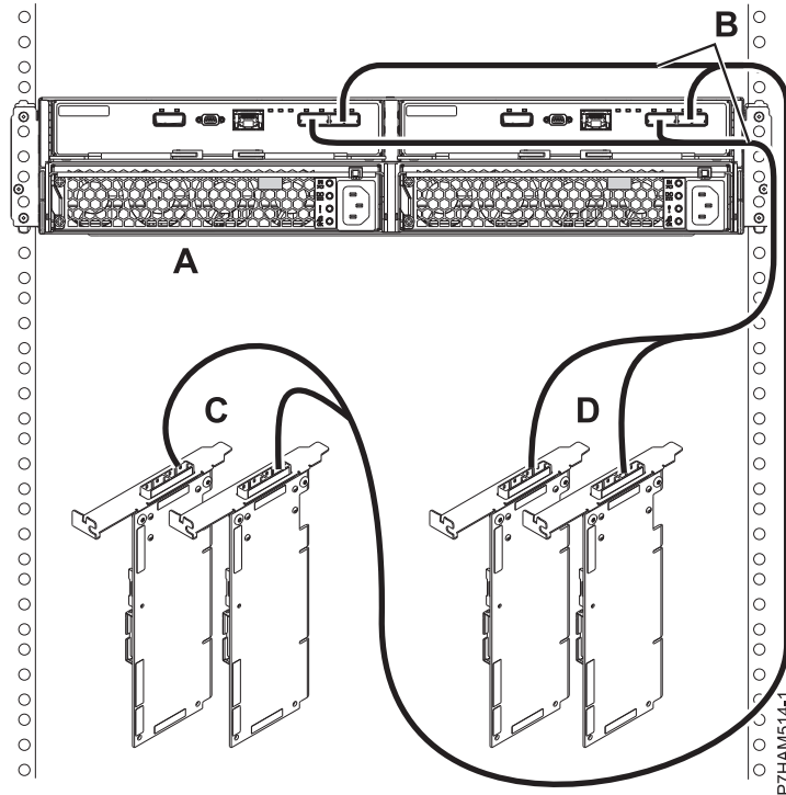
รูปที่ 167. การเชื่อมต่อโหมด 2 ของลิ้นชัก 5887 โดยใช้สายเคเบิล X กับสองคู่ของอะแดปเตอร์ SAS
