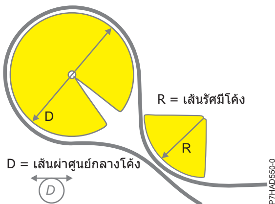
รูปที่ 140. รัศมีการดัดงอสาย
