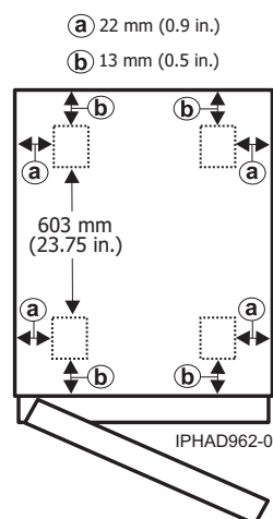
รูปที่ 22. ตำแหน่งลูกถ้วยของโมเดล 0554 และ 7014-S11
