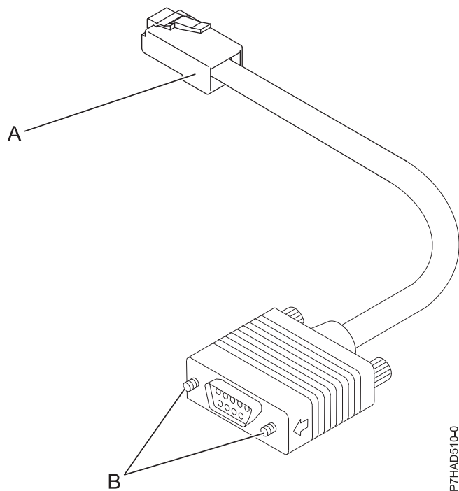
รูปที่ 133. โค้ดคุณลักษณะ 3930
