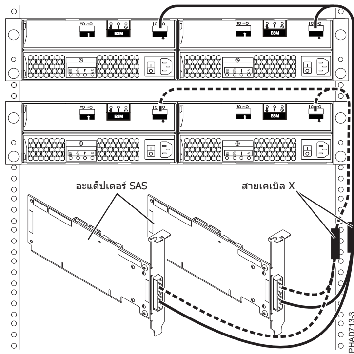
รูปที่ 155. จากอะแดปเตอร์ SAS RAID สองตัวไปยังลิ้นชัก ส่วนขยายดิสก์สองลิ้นชักในคอนฟิกรูเรชันแบบ multi-initiator HA RAID
