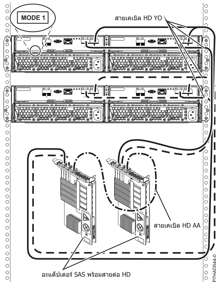
รูปที่ 174. การเชื่อมต่อโหมด 1 ของสองลิ้นชัก 5887 โดยใช้ตัวเชื่อมต่อ HD กับสองอะแดปเตอร์ SAS
