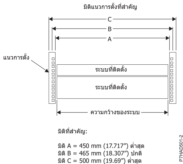
รูปที่ 34. มิติของ ขอบยึดที่สำคัญ
