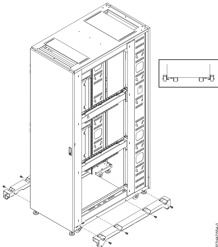
รูปที่ 32. ตำแหน่งของ Outtrigger
