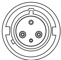
รูปที่ 38. เต้ารับชนิด IEC 60309 P+N+E
