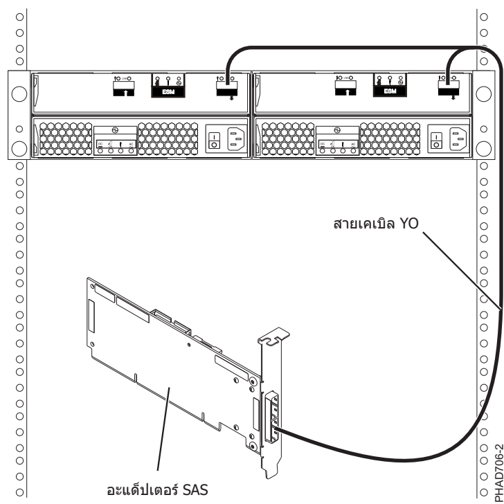
รูปที่ 145. จากอะแดปเตอร์ SAS ไปยังลิ้นชักส่วนขยายดิสก์หนึ่งลิ้นชัก
