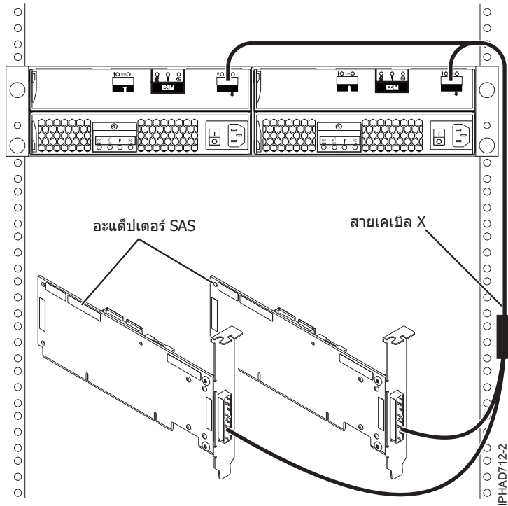
รูปที่ 154. จากอะแดปเตอร์ SAS RAID สองตัวไปยังลิ้นชักส่วนขยายดิสก์ในคอนฟิกรูเรชันแบบ multi-initiator HA RAID
