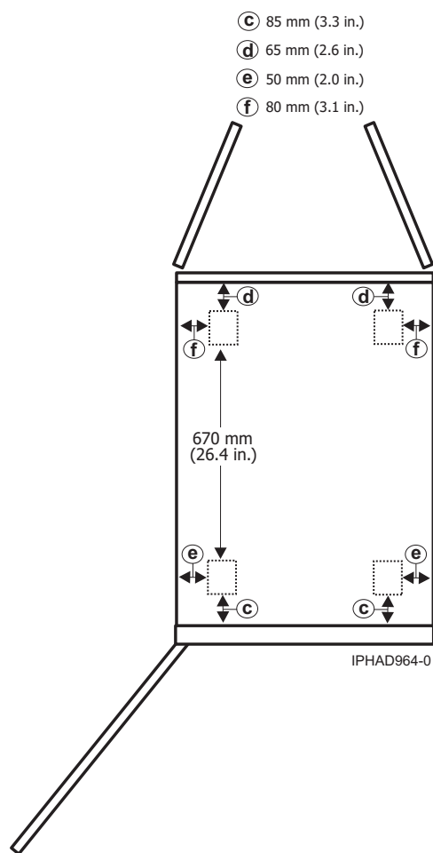
รูปที่ 25. ตำแหน่งลูกถ้วยของโมเดล 0555 และ 7014-S25
