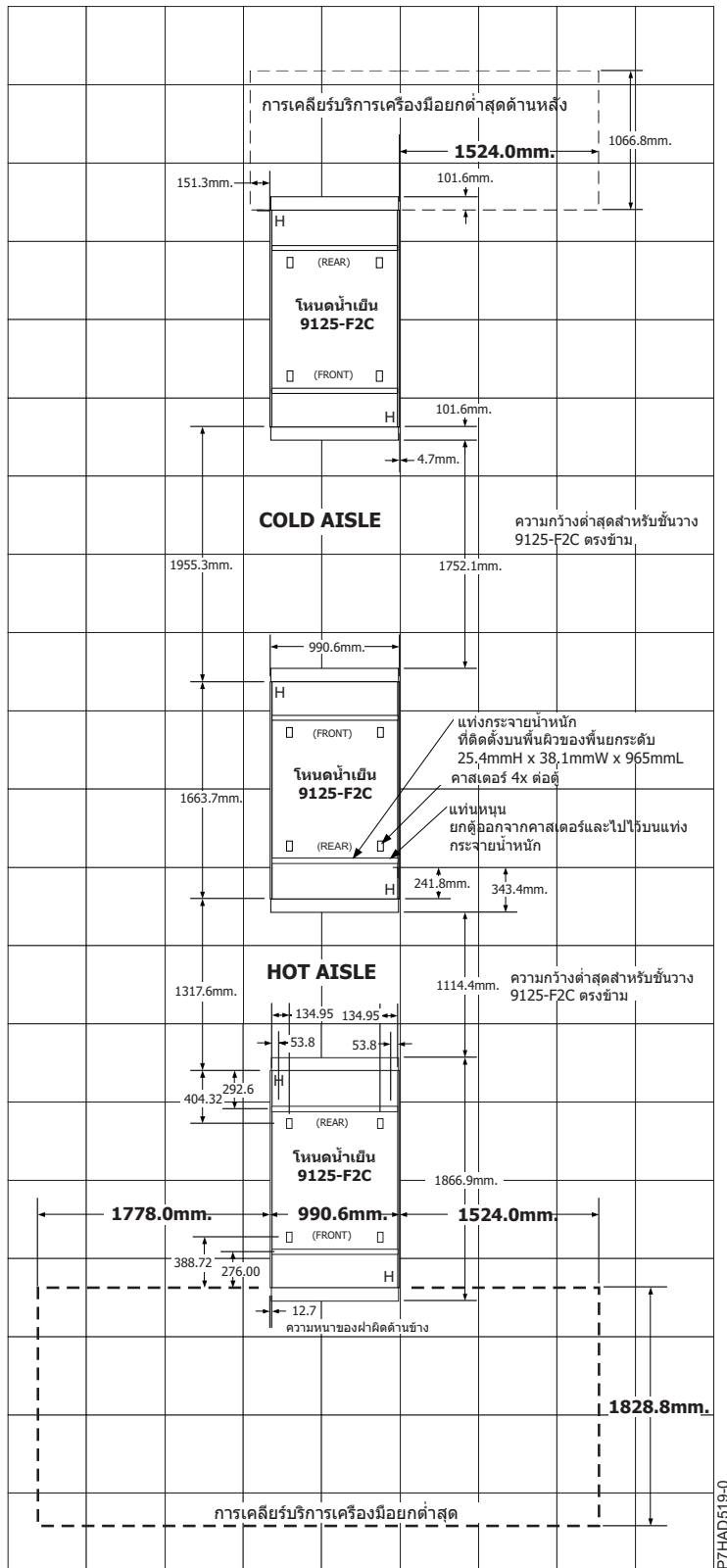
รูปที่ 1. ระยะห่างสำหรับเซอร์วิสสำหรับชั้นวางเดียว - ทางเดินร้อนและทางเดินเย็น
