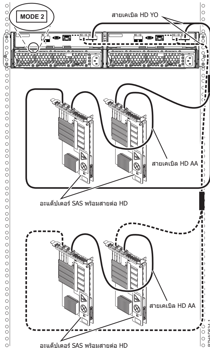
รูปที่ 176. การเชื่อมต่อโหมด 2 ของลิ้นชัก 5887 โดยใช้ตัวเชื่อมต่อ HD เข้ากับสองคู่ของอะแดปเตอร์ SAS
