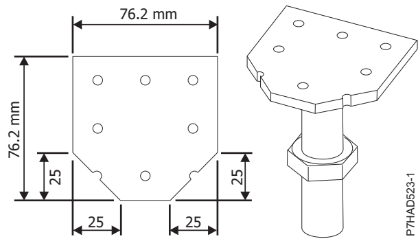
รูปที่ 4. มิติของแท่นตัด
