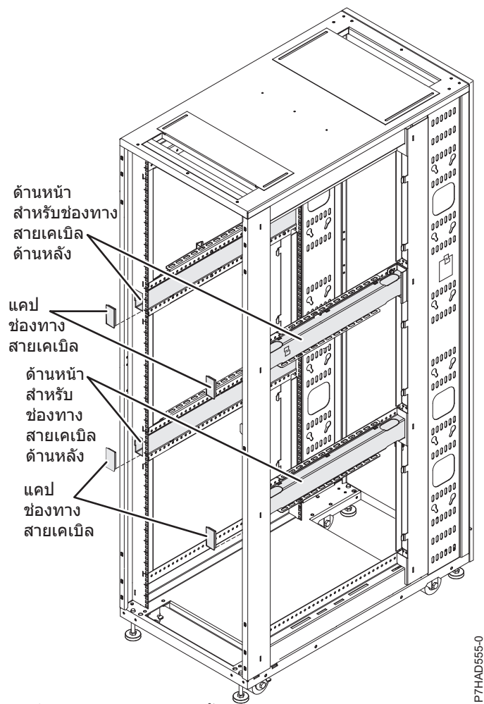
รูปที่ 29. การเดินสายภายในชั้นวาง
