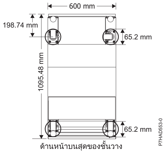
รูปที่ 28. ตำแหน่งลูกล้อ
