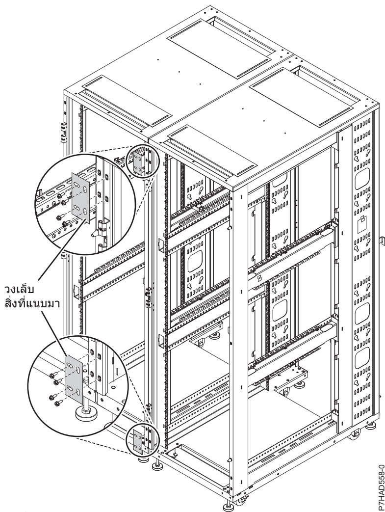
รูปที่ 33. กรอบยึด
