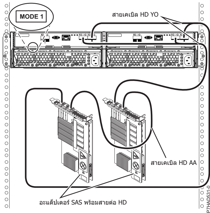
รูปที่ 173. การเชื่อมต่อ โหมด 1 ของลิ้นชัก 5887 เข้ากับสองอะแดปเตอร์ SAS ด้วยตัวเชื่อมต่อ HD
