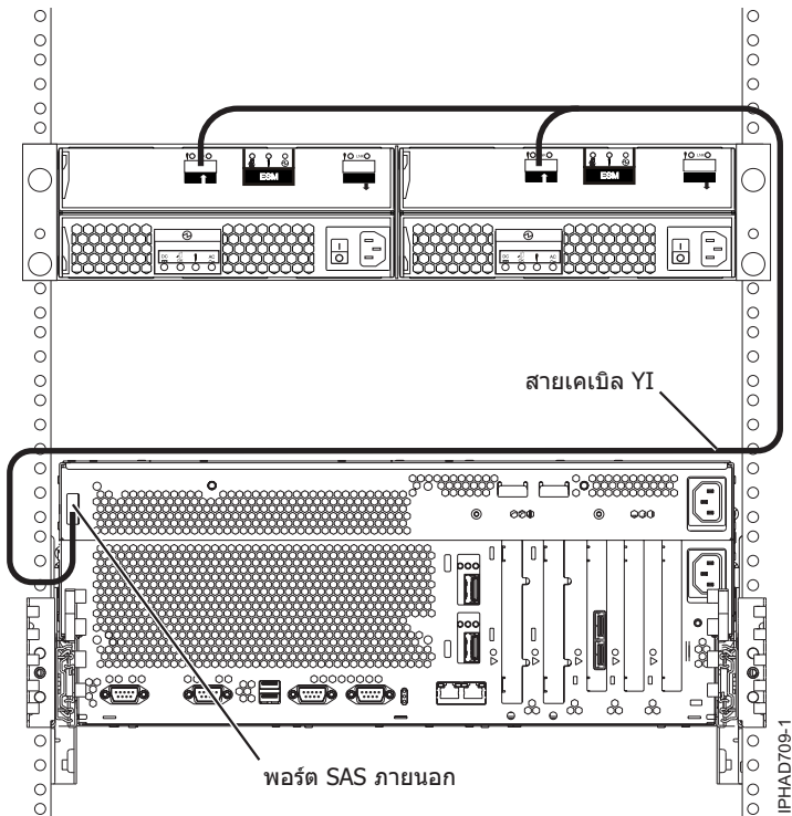
รูปที่ 151. จากพอร์ตของอะแดปเตอร์ SAS ภายนอกของระบบไปยังลิ้นชักส่วนขยายดิสก์
