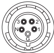
รูปที่ 36. ปลั๊กแบบ Pin Out
