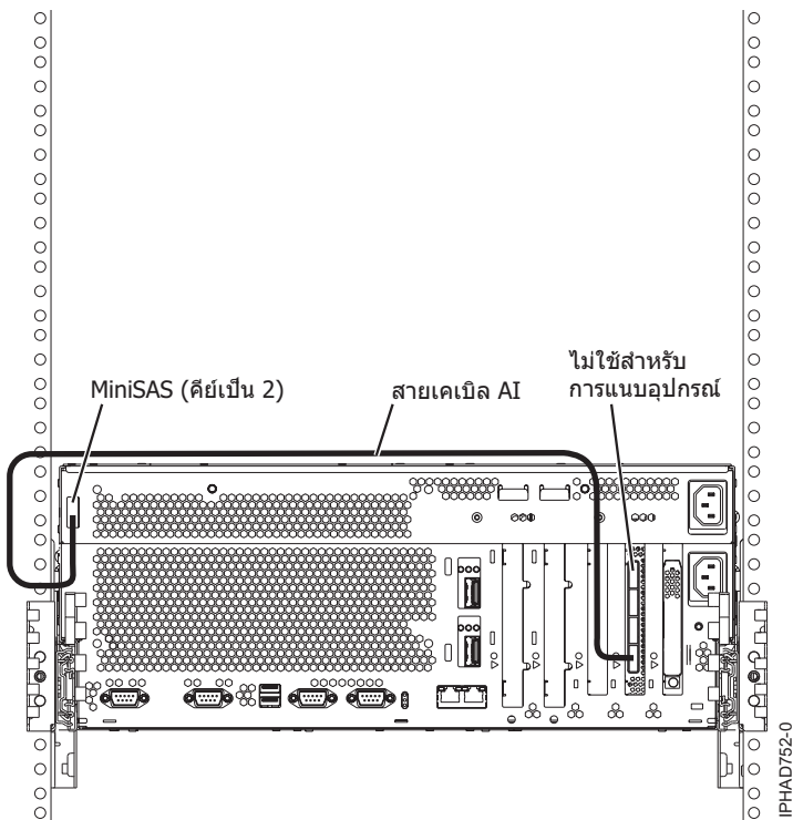
รูปที่ 153. อะแดปเตอร์ FC5904 หรือ FC5908 ที่เชื่อมต่อกับ ลินซ์ส่วนขยายดิสก์
