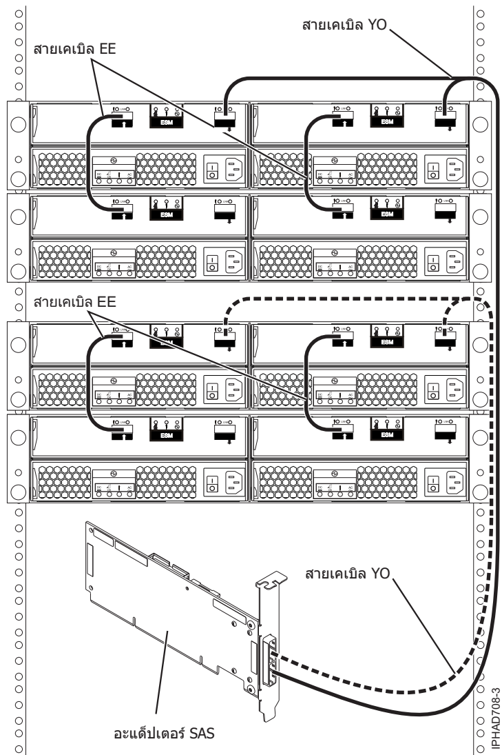
รูปที่ 147. จากอะแดปเตอร์ SAS ไปยังลิ้นชักส่วนขยายดิสก์ 4 ลิ้นชัก
