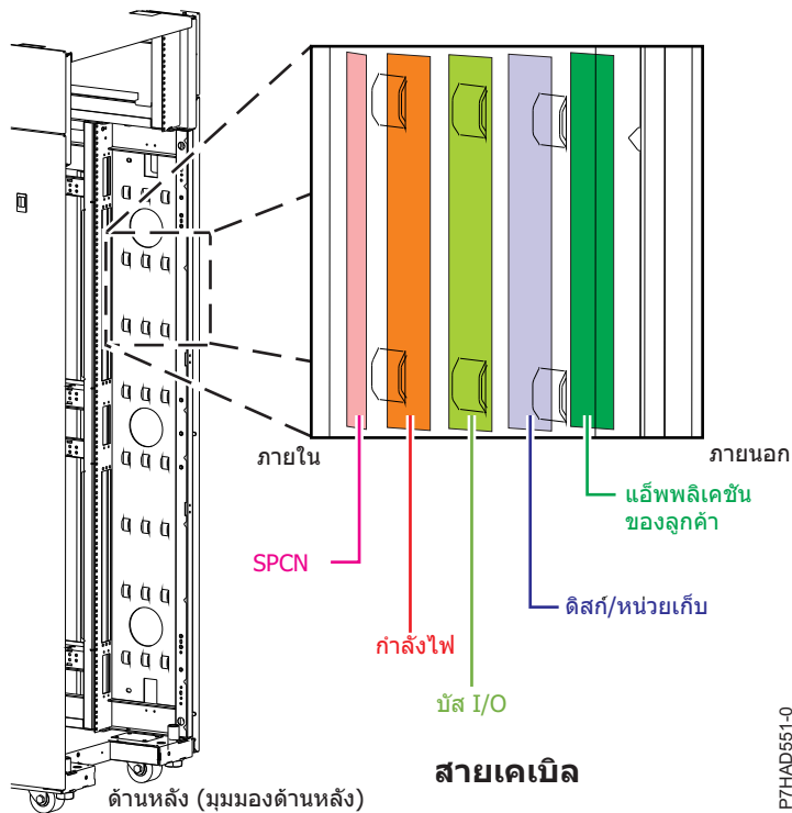
รูปที่ 139. แลนช์บริดจ์การจัดการสาย
