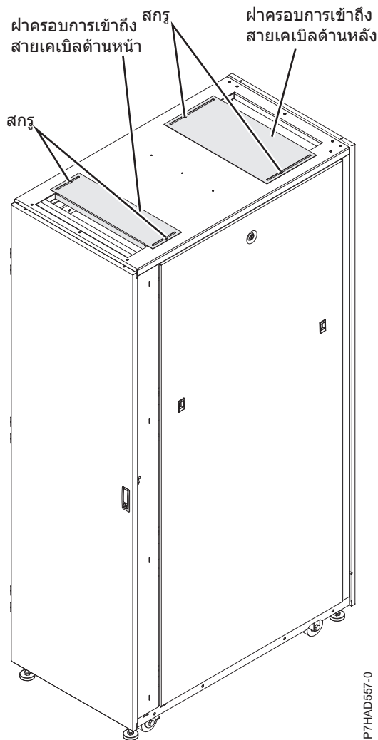
รูปที่ 31. ฝาครอบ การเข้าถึงสายเคเบิล
