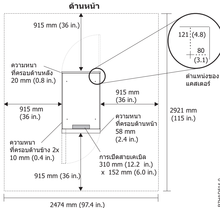
รูปที่ 27. พื้นที่ว่างใช้งานและตำแหน่งลูกกลิ้งสำหรับชั้นวาง 7014-T00, 7014-T42 และ 0553
