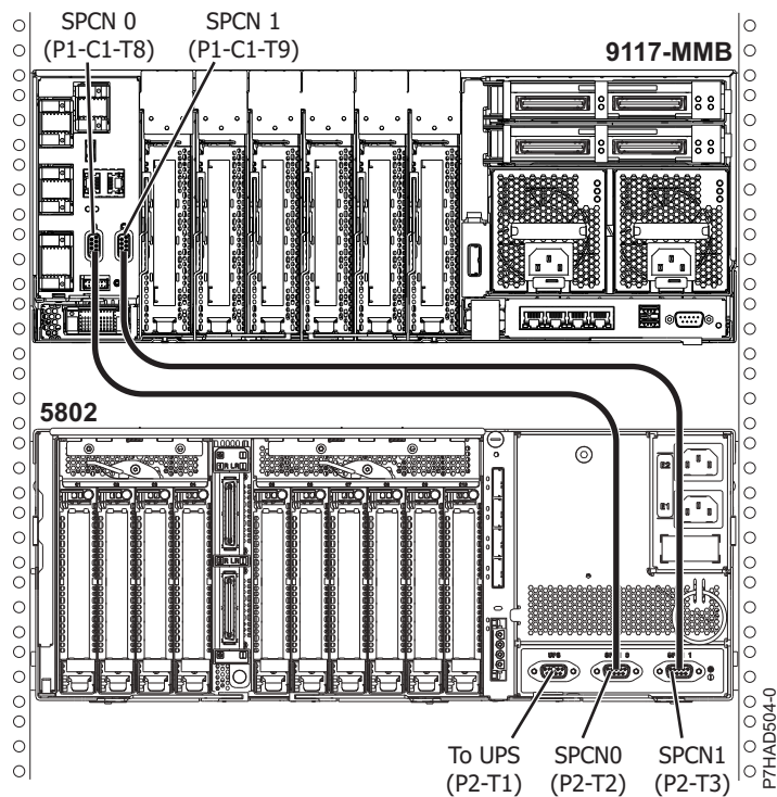
รูปที่ 135. ตำแหน่งการติดตั้งสายเคเบิลจากมุมมองด้านหลังของ 8412-EAD, 9117-MMB, 9117-MMC, 9117-MMD, 9179-MHB, 9179-MHC, 9179-MHD และ 5208 หรือ 5877
