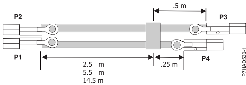
รูปที่ 142. ความยาวชุดสายเคเบิล SAS X ภายนอก
