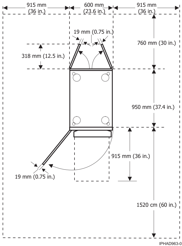
รูปที่ 24. รูปแผนผังโมเดล 0555 และ 7014-S25
