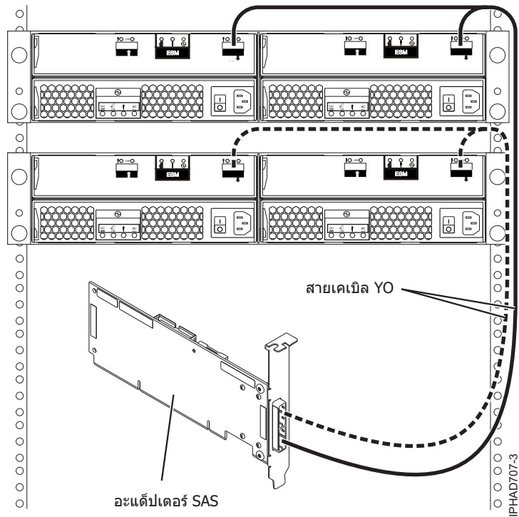
รูปที่ 146. จากอะแดปเตอร์ SAS ไปยังลิ้นชักส่วนขยายดิสก์ 2 ลิ้นชัก
