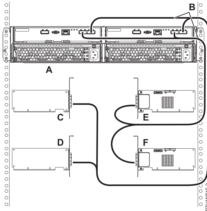
รูปที่ 168. การเชื่อมต่อโหมด 4 ของลิ้นชัก 5887 โดยใช้สายเคเบิล X กับสวิตช์อะแดปเตอร์ SAS เดียว
