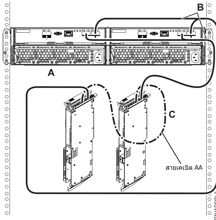
รูปที่ 172. การเชื่อมต่อโหมด 1 ของล้นชัก 5887 โดยการใช้สายเคเบิล YO กับอะแดปเตอร์ SAS คู่
