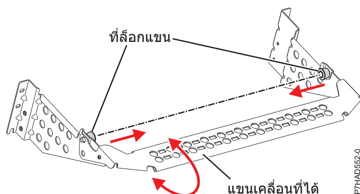
รูปที่ 141. ที่ค้ำในการจัดการสายเคเบิล
