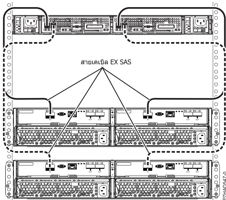
รูปที่ 178. การเชื่อมต่อลินซ์ 5887 สองลินซ์โดยใช้สายเคเบิล HDEX กับ EDR1 เดียว
