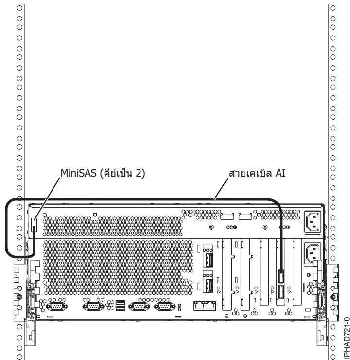
รูปที่ 152. จากอะแดปเตอร์ SAS ไปยังดิสก์สล็อต SAS ภายในผ่านทางพอร์ต SAS ภายนอกของระบบ
