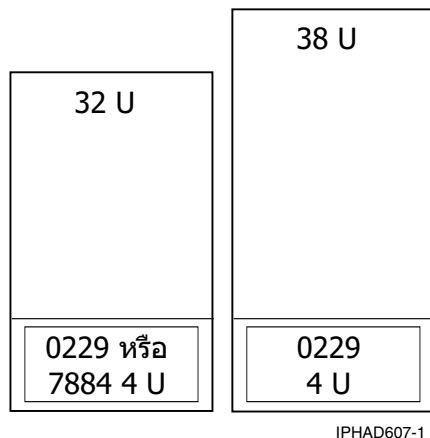
รูปที่ 10. โค้ดคุณลักษณะ 7884: 9406-520 และ 9111-520 ในชั้นวาง
