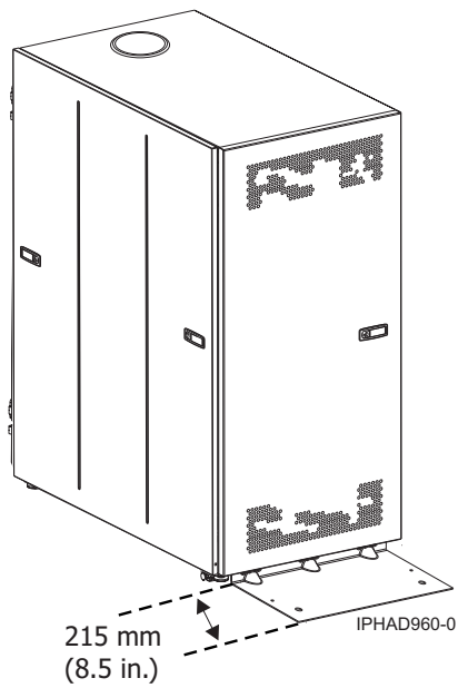
รูปที่ 23. โมเดล 0555 และ 7014-S25 ที่มีฐานกันสั่น
