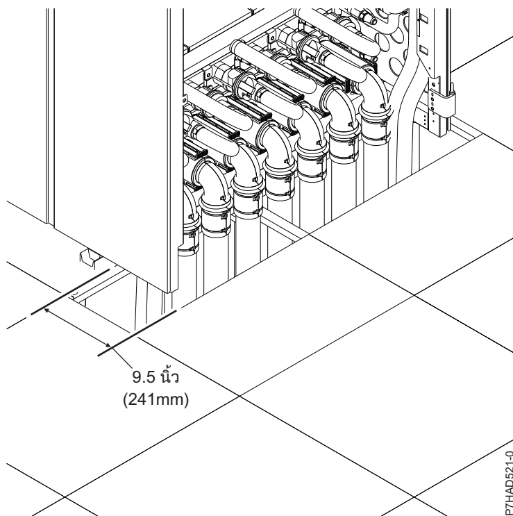
รูปที่ 3. ช่องเจาะที่พื้น
