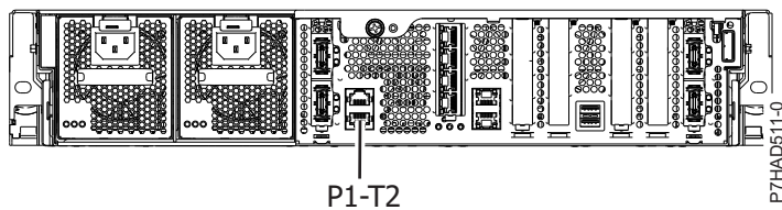
รูปที่ 136. มุมมองด้านหลังที่มีตำแหน่งการติดตั้งสายเคเบิลของ 8231-E2B, 8231-E1C, 8231-E1D, 8231-E2C, 8231-E2D และ 8268-E1D
