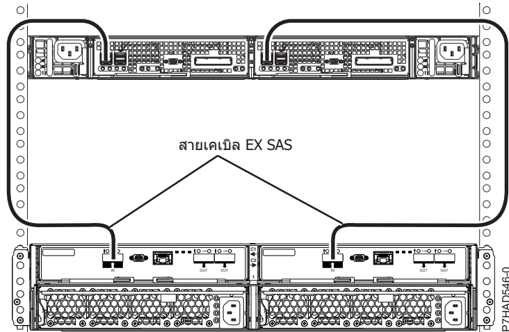
รูปที่ 177. การเชื่อมต่อลินซ์ 5887 เดียวโดยใช้สายเคเบิล HDEX กับ EDR1 เดียว
