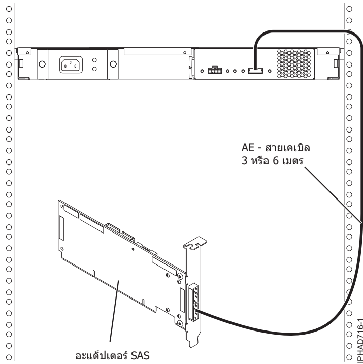
รูปที่ 149. จากอะแดปเตอร์ SAS ไปยังลิ้นชักส่วนขยายสื่อบันทึก
