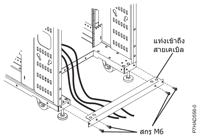
รูปที่ 30. แถบสำหรับเข้าถึงสายเคเบิล
