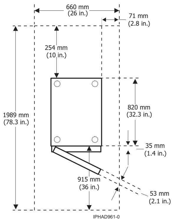
รูปที่ 21. รูปแผนผังโมเดล 0554 และ 7014-S11
