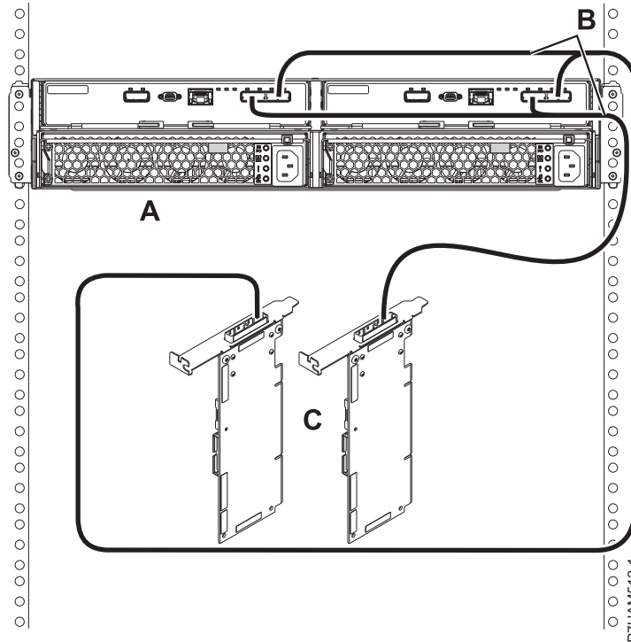
รูปที่ 169. การเชื่อมต่อโหมด 1 ของลินซึก 5887 โดยการใช้สายเคเบิล YO กับอะแดปเตอร์ SAS คู่
