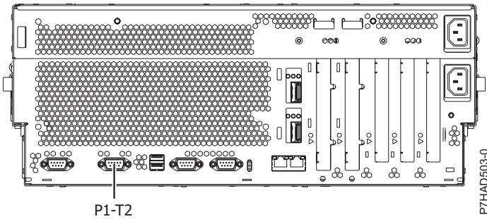
รูปที่ 134. 8233-E8B และ 8236-E8C มุมมอง ด้านหลังที่มีตำแหน่งติดตั้งสายเคเบิล
