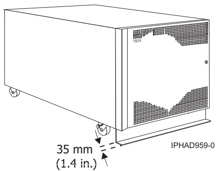
รูปที่ 20. โมเดล 0554 และ 7014-S11 ที่มี คานกันสั่น
