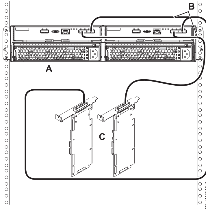
รูปที่ 164. การเชื่อมต่อโหมด 1 ของลินซึก 5887 โดยการใช้สายเคเบิล YO กับอะแดปเตอร์ SAS คู่
