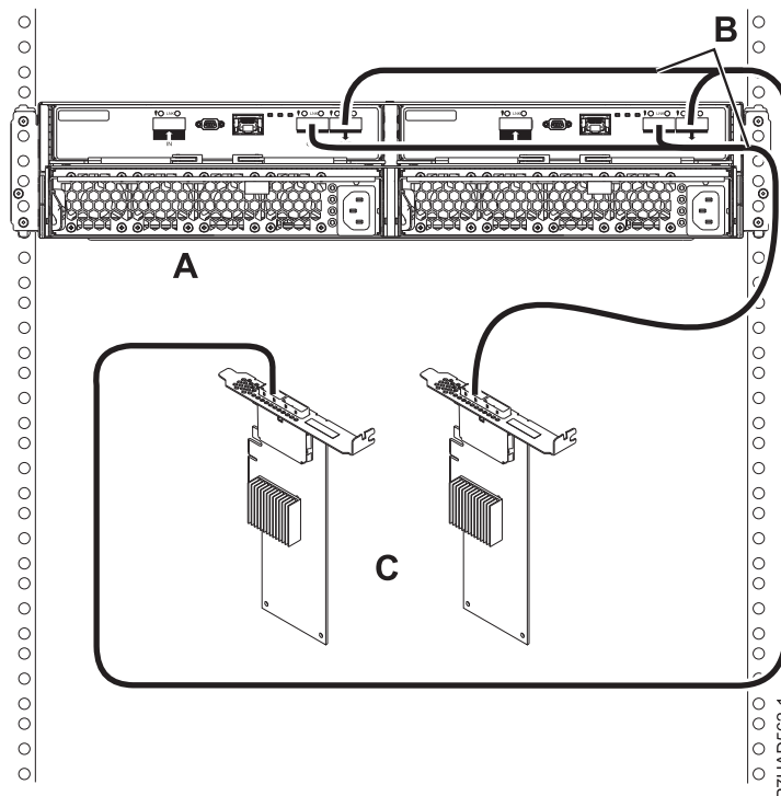
รูปที่ 160. การเชื่อมต่อโหมด 1 ของลิ้นชัก 5887 โดยการใช้สายเคเบิล YO กับอะแดปเตอร์ SAS คู่
