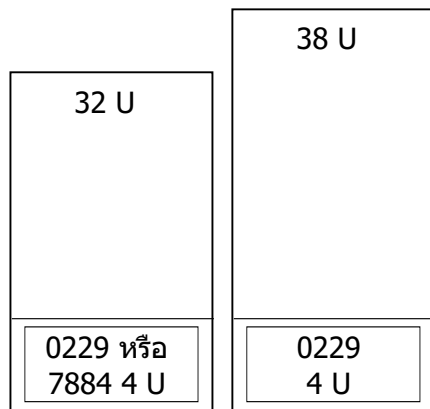
รูปที่ 5. โค้ดคุณลักษณะ 7884: 9406-520 และ 9111-520 ในชั้นวาง
