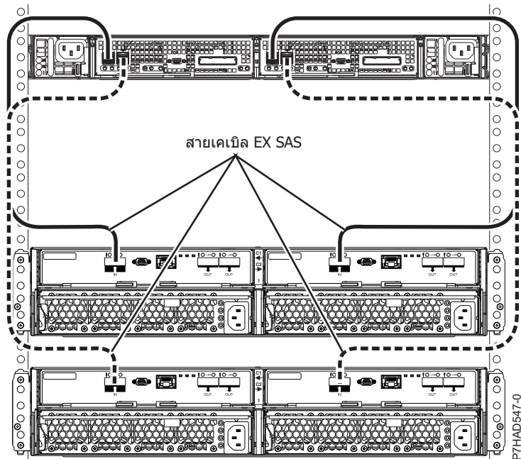
รูปที่ 173. การเชื่อมต่อลิ้นชัก 5887 สองลิ้นชักโดยใช้สายเคเบิล HDEX กับ EDR1 เดียว
