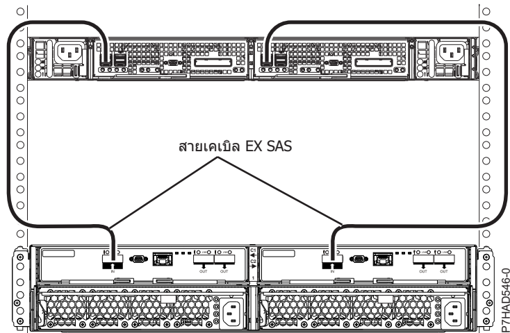
รูปที่ 172. การเชื่อมต่อลิ้นชัก 5887 เดียวโดยใช้สายเคเบิล HDEX กับ EDR1 เดียว
