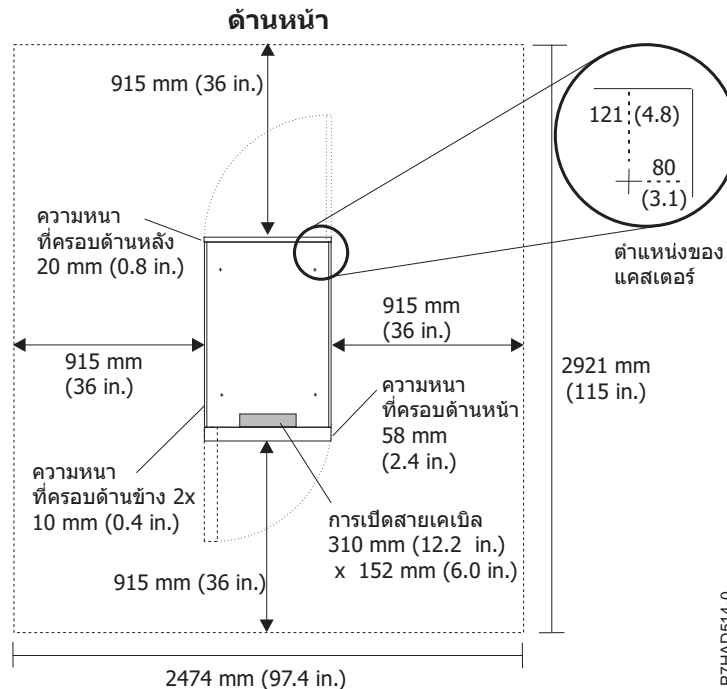
รูปที่ 22. พื้นที่ว่างใช้งานและตำแหน่งลูกกลิ้งสำหรับชั้นวาง 7014-T00, 7014-T42 และ 0553
