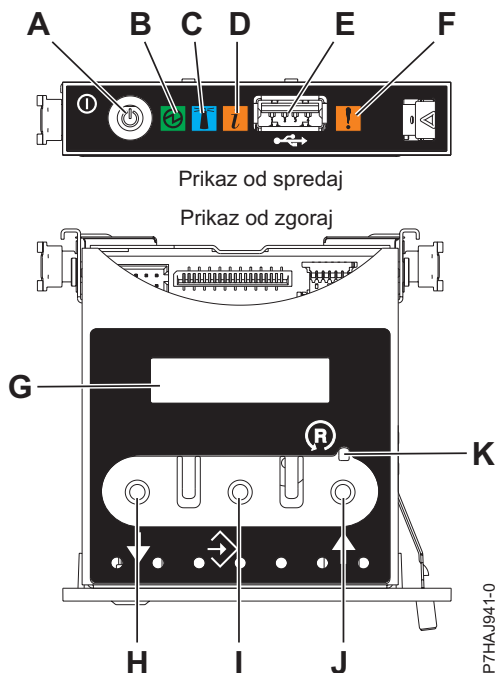
Slika 4. Nadzorna plošča
