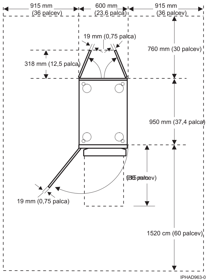
Slika 19. Prikaz načrta modelov 0555 in 7014-S25
