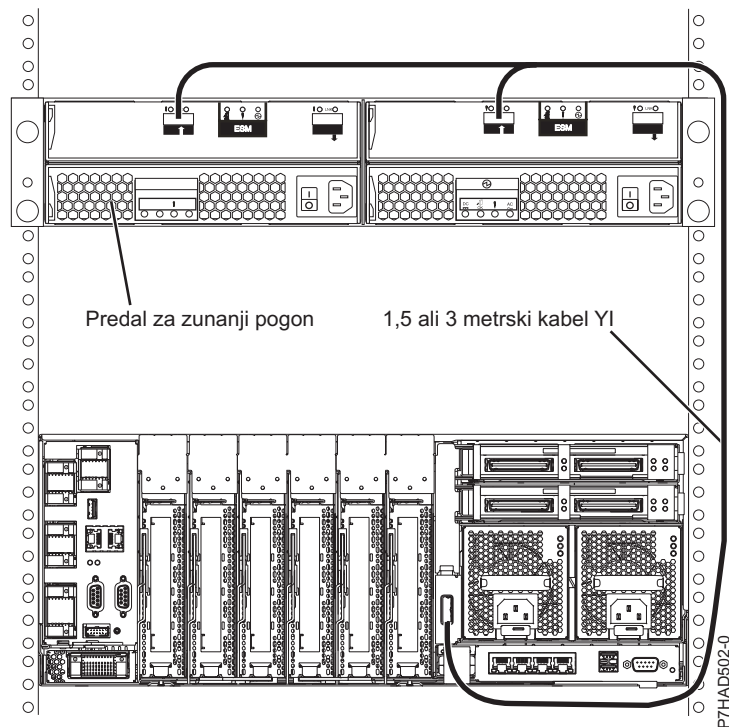
Slika 146. Sistemska zunanja vrata vmesnika SAS s predalom za razširitev diskov (modela 9117-MMB in 9179-MHB)
