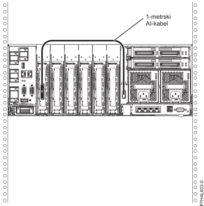
Slika 147. Vmesnik SAS z notranjimi diskovnimi režami SAS prek sistemskih zunanjih vrat SAS
