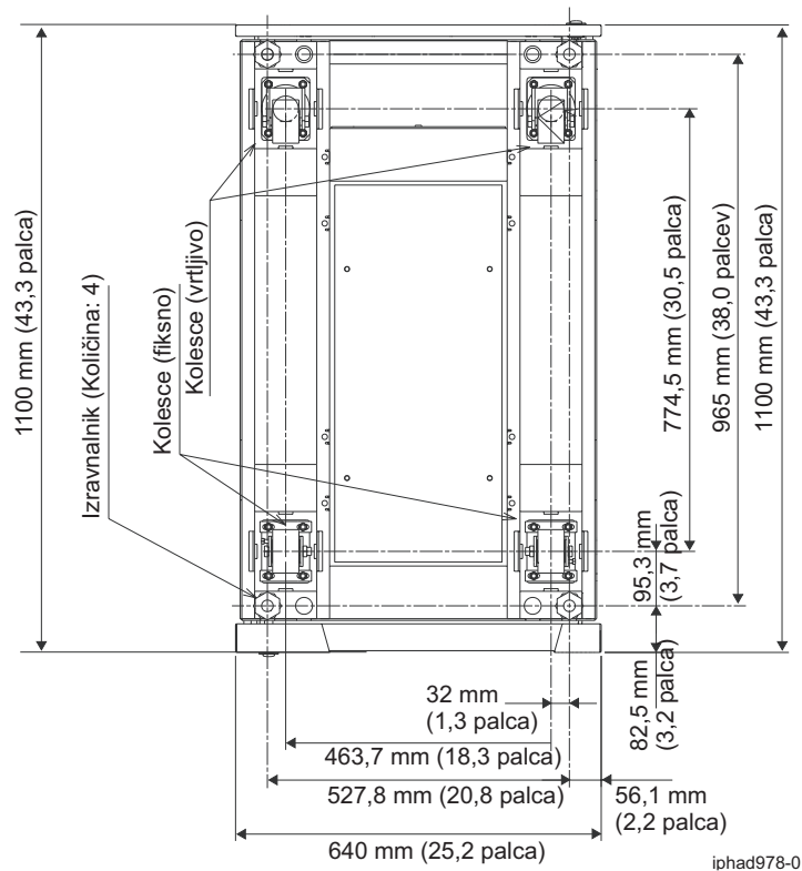
Slika 26. Lokacije kolesc in izravnalnikov
