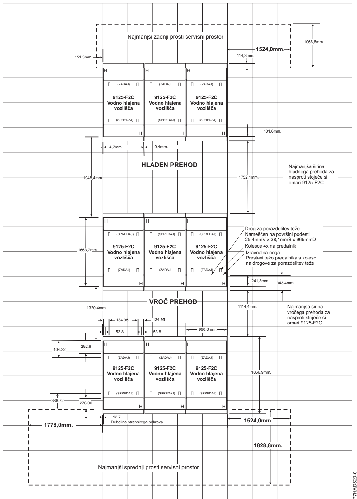
Slika 2. Prosti servisni prostor za več omar - Vroč in hladen prehod
