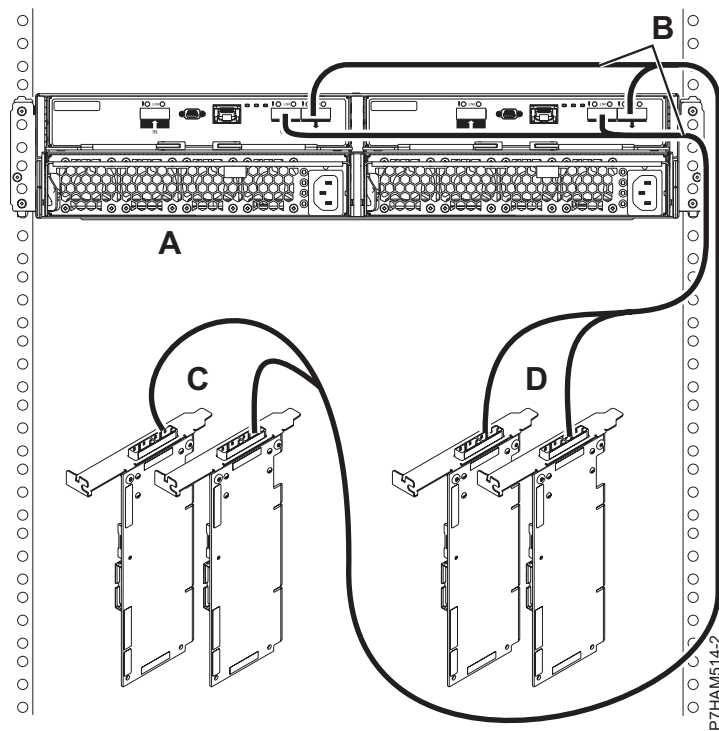
Slika 167. Povezava predala 5887 v načinu 2 s kabli X z dvema paroma vmesnikov SAS
