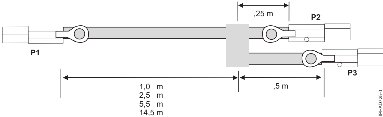
Slika 143. Dolžine kablov v zunanjem SAS YO-kabelskem kompletu
