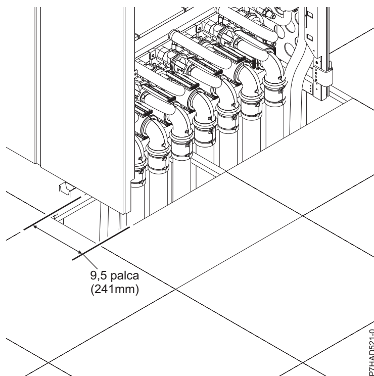
Slika 3. Izrez tal
