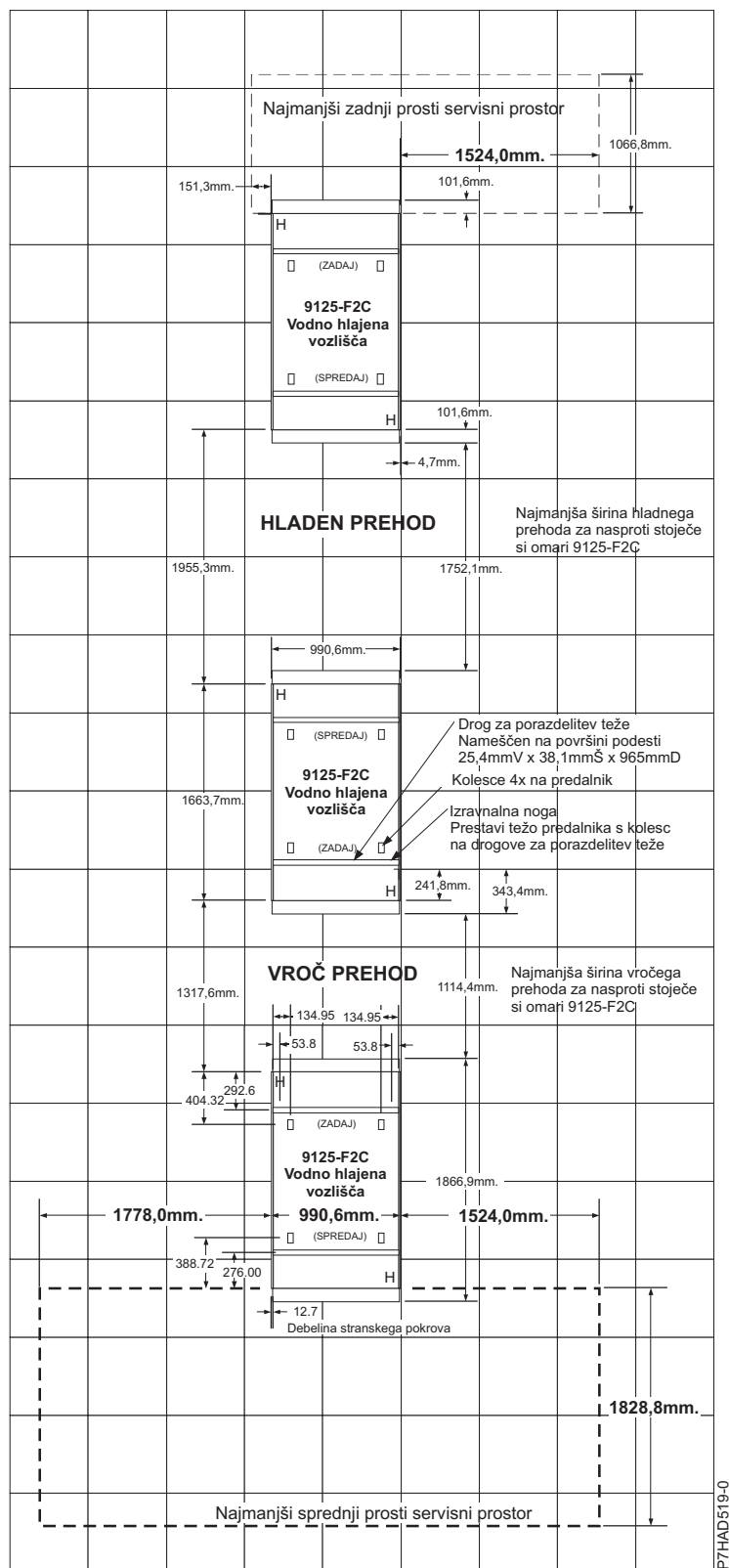
Slika 1. Prosti servisni prostor za eno omaro - Vroč in hladni prehod
