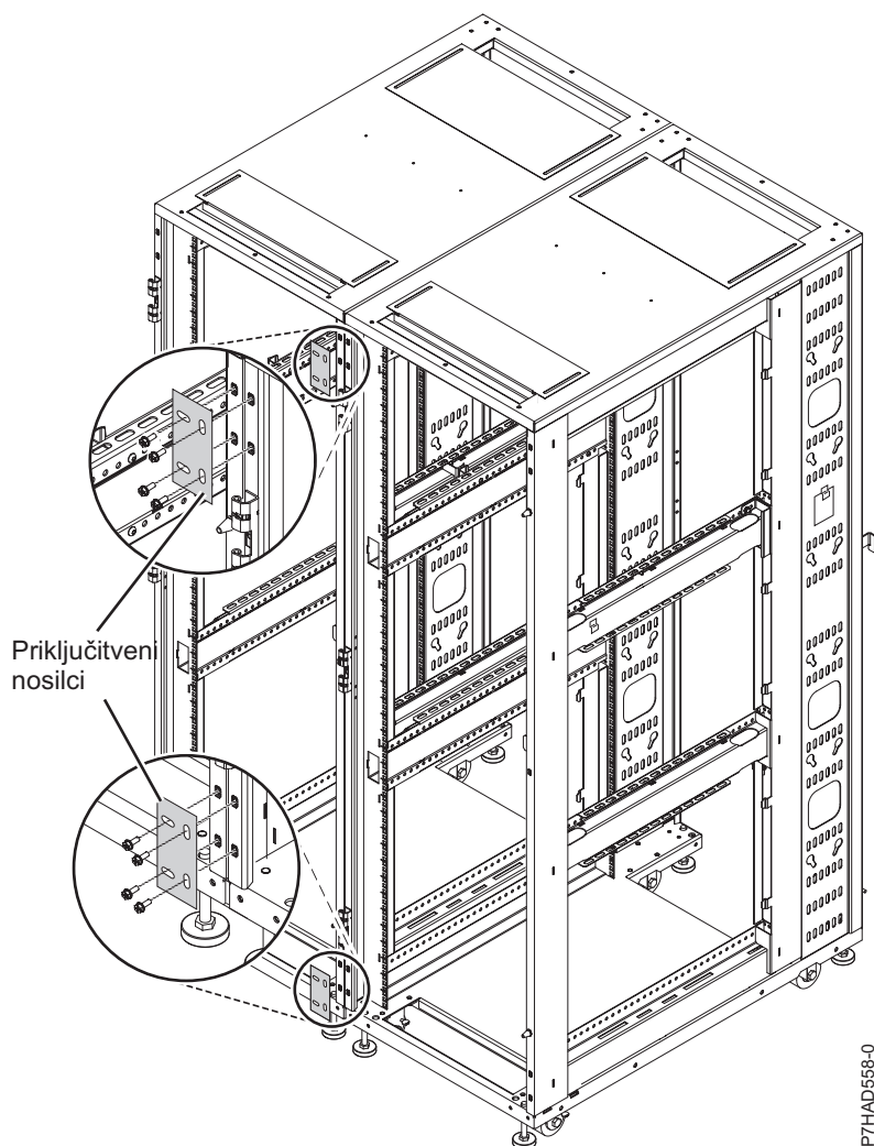
Slika 33. Spojke
