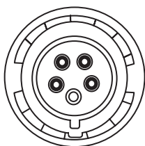
Slika 36. Opis nožic vtiča
