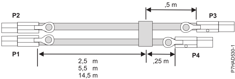
Slika 142. Dolžine kablov v zunanjem SAS X-kabelskem kompletu
