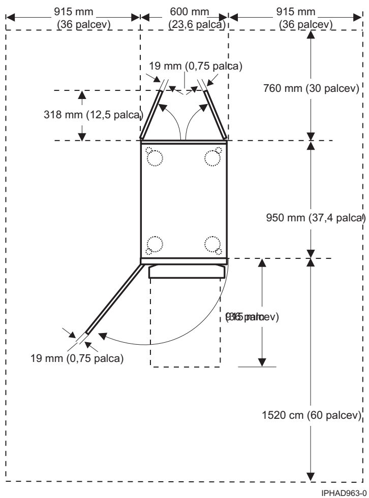
Slika 24. Prikaz načrta modelov 0555 in 7014-S25
