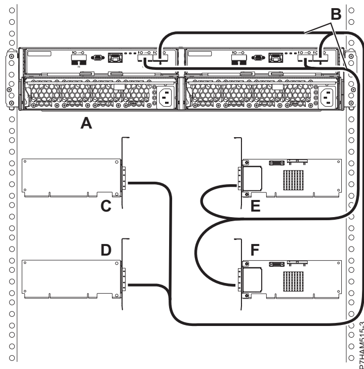
Slika 168. Povezava predala 5887 v načinu 4 s kabli X s štirimi posameznimi vmesniki SAS
