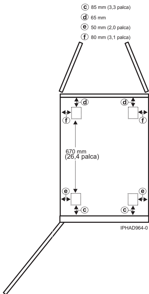
Slika 25. Lokacije kolesc za modela 0555 in 7014-S25
