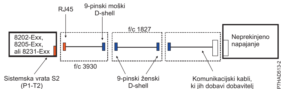
Slika 138. Ožičenje neprekinjenega napajanja za 8202-E4B, 8202-E4C, 8205-E6B, 8205-E6C, 8231-E2B, 8231-E1C, 8231-E1D, 8231-E2C, 8231-E2D in 8268-E1D
