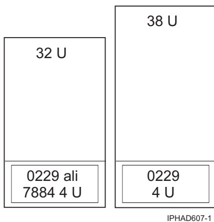
Slika 10. Koda možnosti 7884: 9406-520 in 9111-520 v omari
