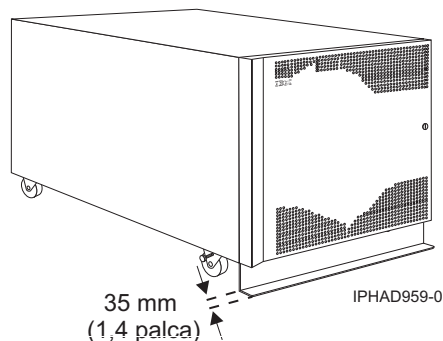
Slika 15. Modela 0554 in 7014-S11 s stabilizatorjem
