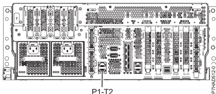
Slika 132. Pogled od zadaj za 8202-E4B, 8202-E4C, 8202-E4D, 8205-E6B, 8205-E6C in 8205-E6D z mesti za namestitev kablov
