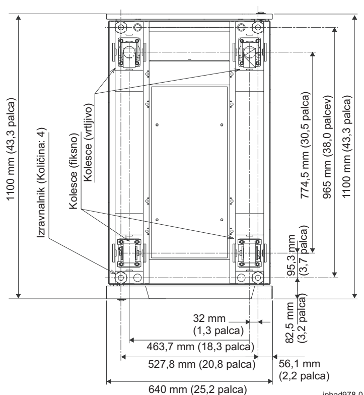
Slika 5. Lokacije kolesc in izravnalnikov
