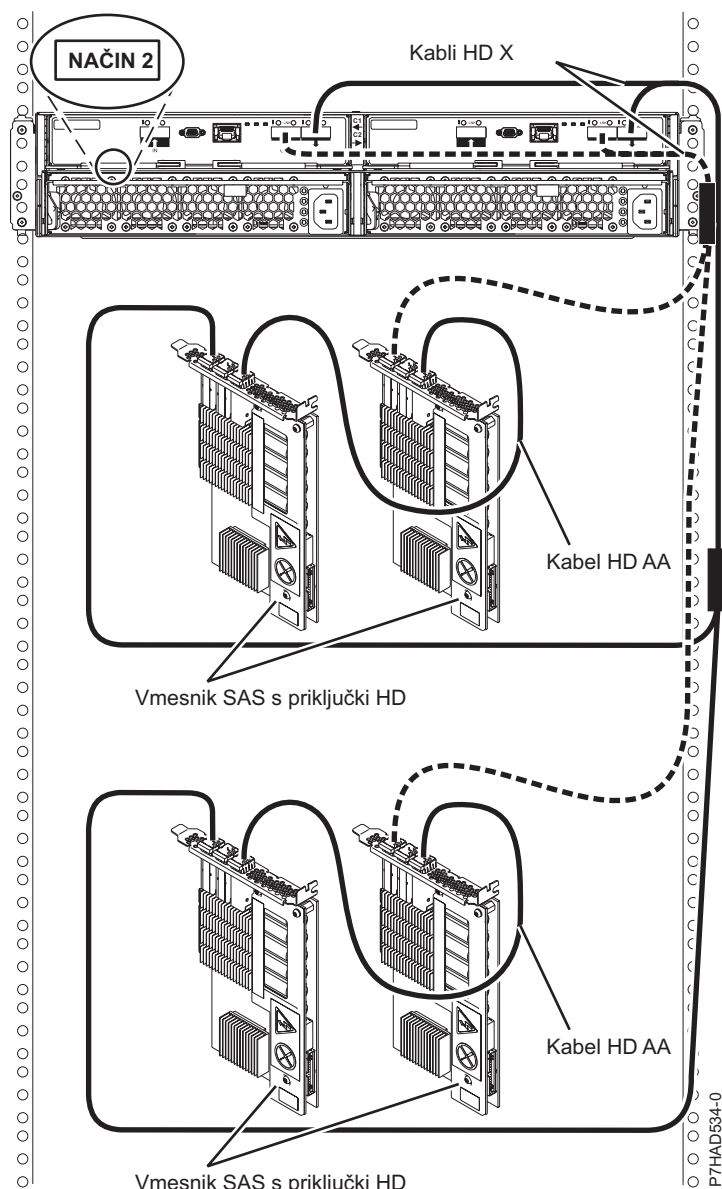
Slika 172. Povezava predala 5887 v načinu 2 s spojniki HD z dvema paroma vmesnikov SAS
