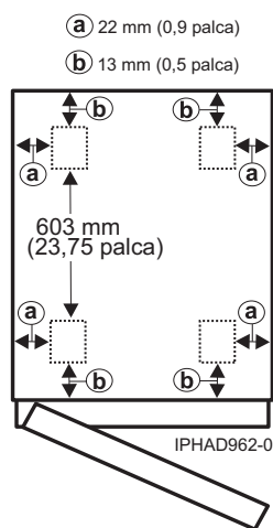
Slika 18. Lokacije kolesc za modela 0554 in 7014-S11
