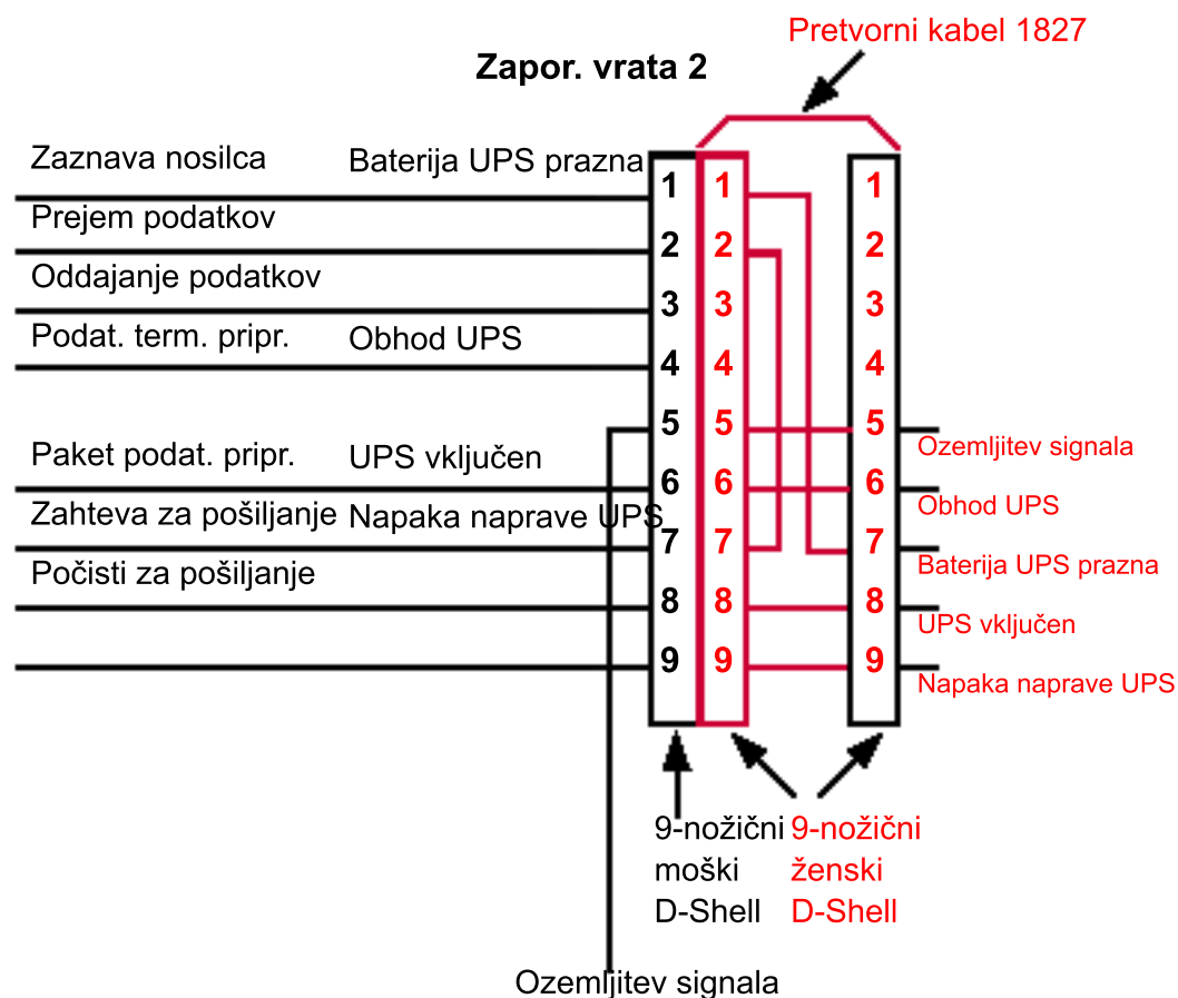
Slika 128. Ožičenje kabla 1827
