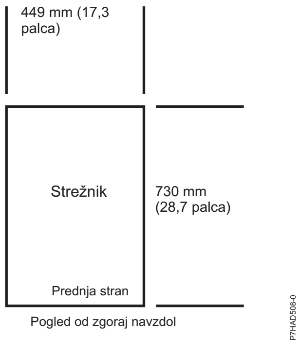
Slika 1. Prikazi načrtov za modele 8202-E4B, 8202-E4C, 8202-E4D, 8205-E6B, 8205-E6C in 8205-E6D (vgradni strežniki)
