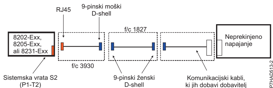
Slika 134. Ožičenje neprekinjenega napajanja za 8202-E4B, 8202-E4C, 8205-E6B, 8205-E6C, 8231-E2B, 8231-E1C, 8231-E1D, 8231-E2C, 8231-E2D in 8268-E1D
