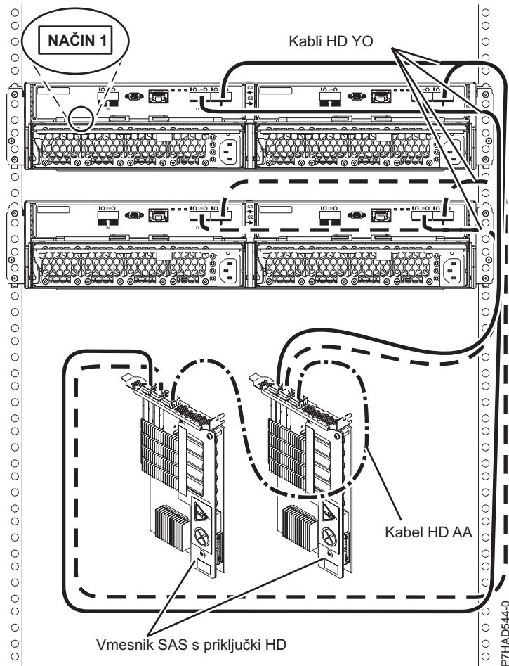
Slika 170. Povezava predalov 5887 v načinu 1 s spojniki HD z dvema vmesnikoma SAS
