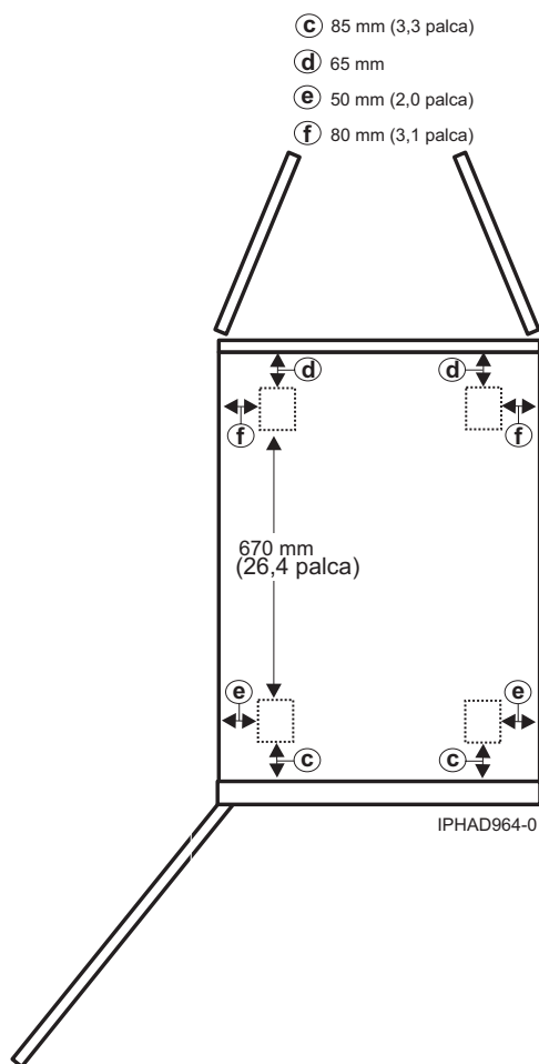
Slika 21. Lokacije kolesc za modela 0555 in 7014-S25
