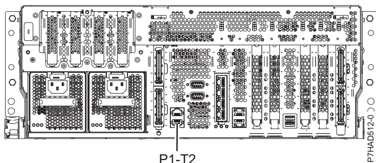
Slika 133. Pogled od zadaj za 8202-E4B, 8202-E4C, 8202-E4D, 8205-E6B, 8205-E6C in 8205-E6D z mesti za namestitve kablov
