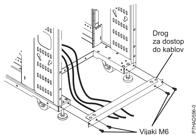
Slika 26. Drog za dostop do kablov
