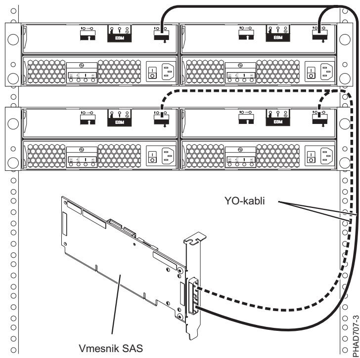
Slika 142. Vmesnik SAS z dvema predaloma za razširitev diskov
