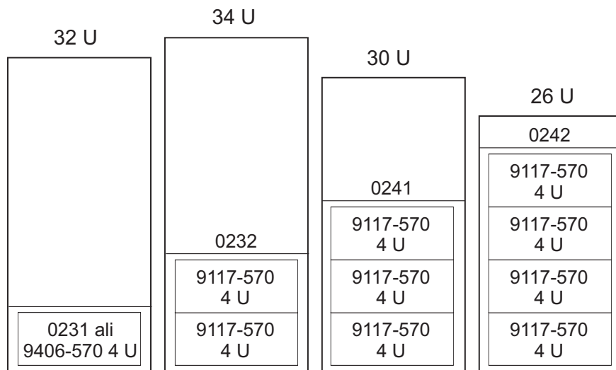
Slika 8. 570 v omari
