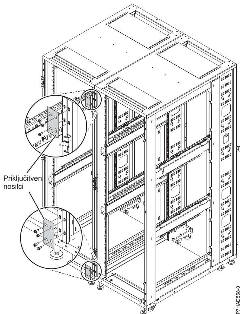
Slika 29. Spojke
