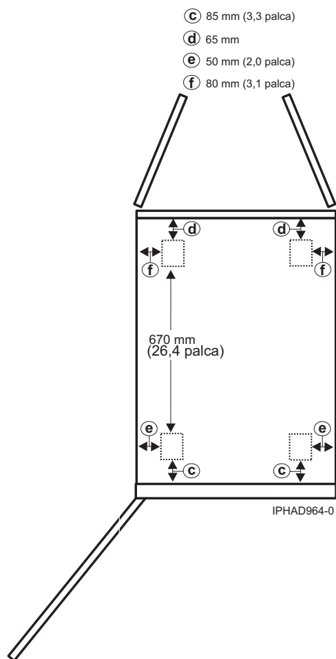
Slika 21. Lokacije koles za modela 0555 in 7014-S25
