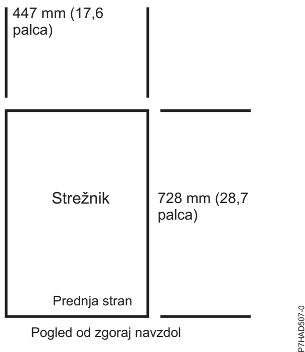
Slika 1. Pogled načrta za model 8231-E2B, 8231-E1C, 8231-E1D, 8231-E2C, 8231-E2D in 8268-E1D (vgradni strežnik)
