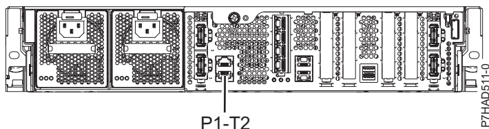
Slika 132. Pogled od zadaj za lokacijo namestitve kablov za 8231-E2B, 8231-E1C, 8231-E1D, 8231-E2C, 8231-E2D in 8268-E1D
