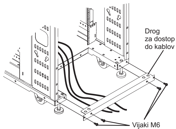
Slika 26. Drog za dostop do kablov
