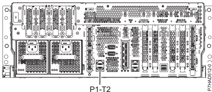
Slika 133. Pogled od zadaj za 8202-E4B, 8202-E4C, 8202-E4D, 8205-E6B, 8205-E6C in 8205-E6D z mesti za namestitev kablov
