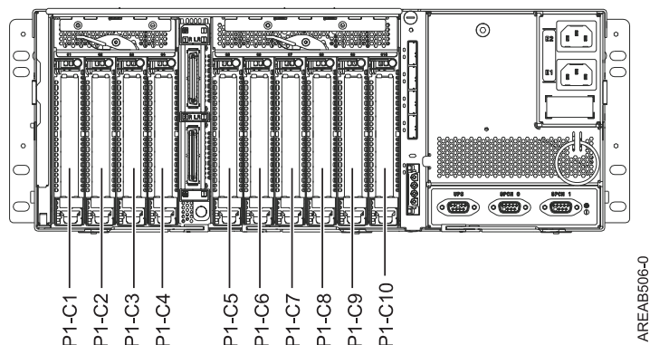
Slika 2. Prikaz od zadaj. Ta slika kaže prikaz razširitvene enote od zadaj.
