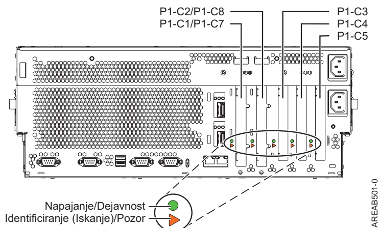
Slika 2. Prikaz ohišja od zadaj z lokacijskimi kodami. Tabela 11 prikazuje pogled sistemske enote od zadaj z lokacijskimi kodami za reže PCI in GX+.
