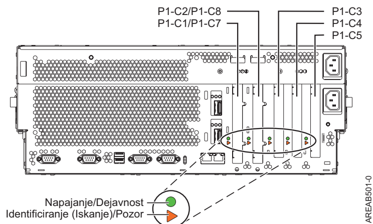
Slika 1. Prikaz sistema od zadaj z lokacijskimi kodami. Tabela 4 prikazuje pogled sistema od zadaj z lokacijskimi kodami za reže PCI in GX.
