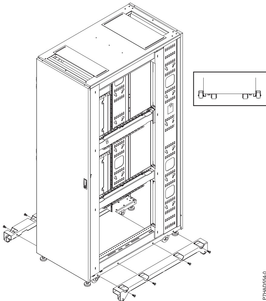
Obrázok 27. Umiestnenie podpier
