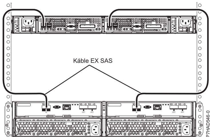
Obrázok 172. Pripojenie jednej zásuvky 5887 pomocou káblov HD EX k jednému EDR1
