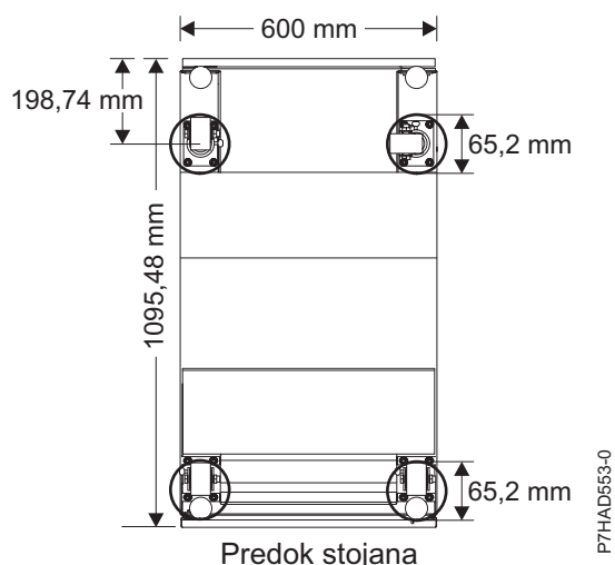
Obrázok 23. Umiestnenie koliesok
