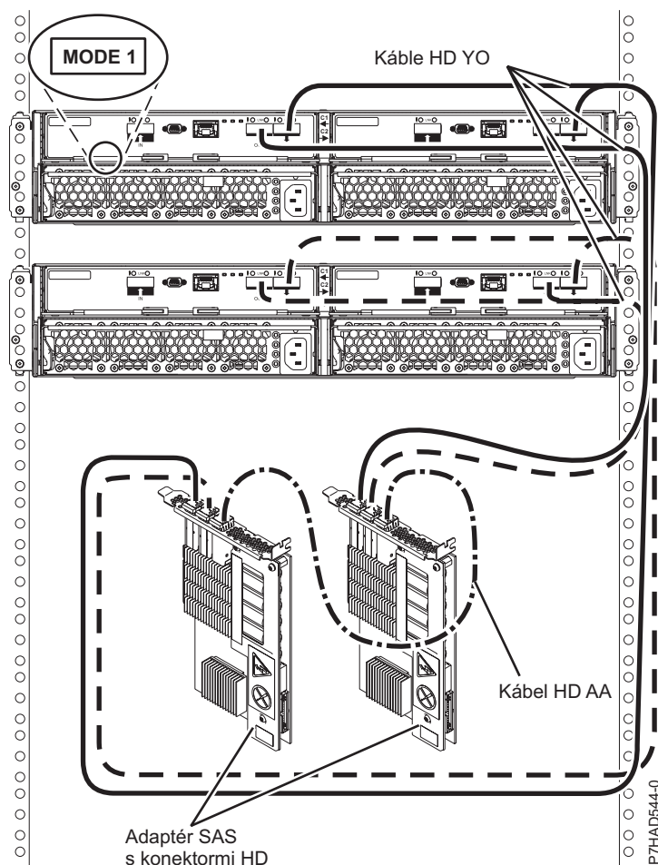
Obrázok 169. Pripojenie v režime 1 dvoch zásuviek 5887 pomocou konektorov HD k dvom adaptérom SAS
