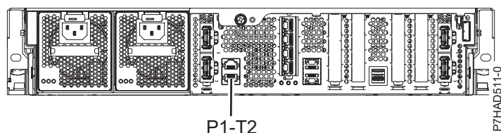
Obrázok 131. Pohľad zozadu na 8231-E2B, 8231-E1C, 8231-E1D, 8231-E2C, 8231-E2D a 8268-E1D s miestom inštalácie kábla
