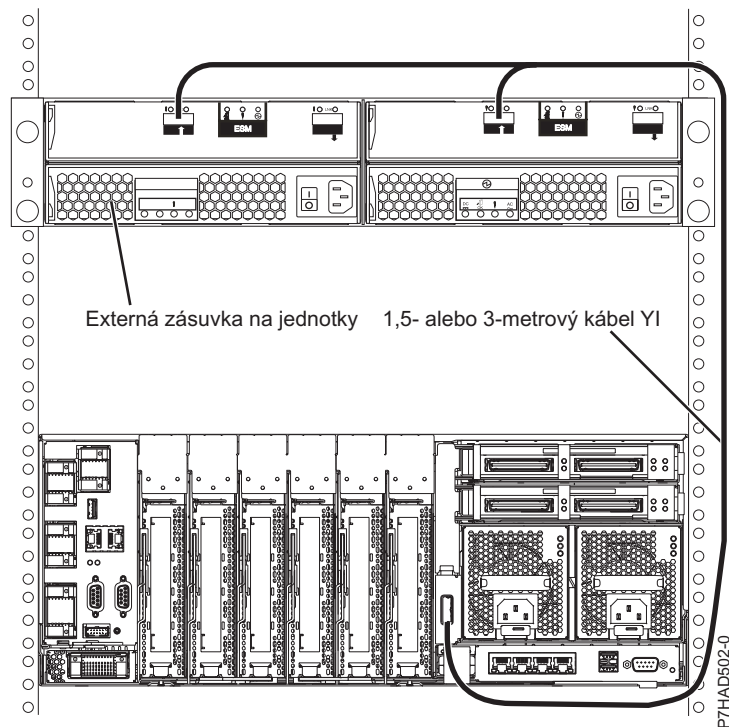
Obrázok 146. Systémový externý port adaptéra SAS k rozširujúcej zásuvke disku (modely 9117-MMB a 9179-MHB).
