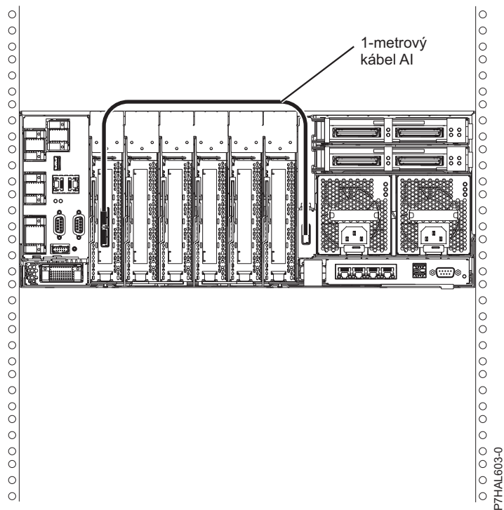
Obrázok 147. Adaptér SAS k interným slotom diskov SAS cez systémový externý port SAS
