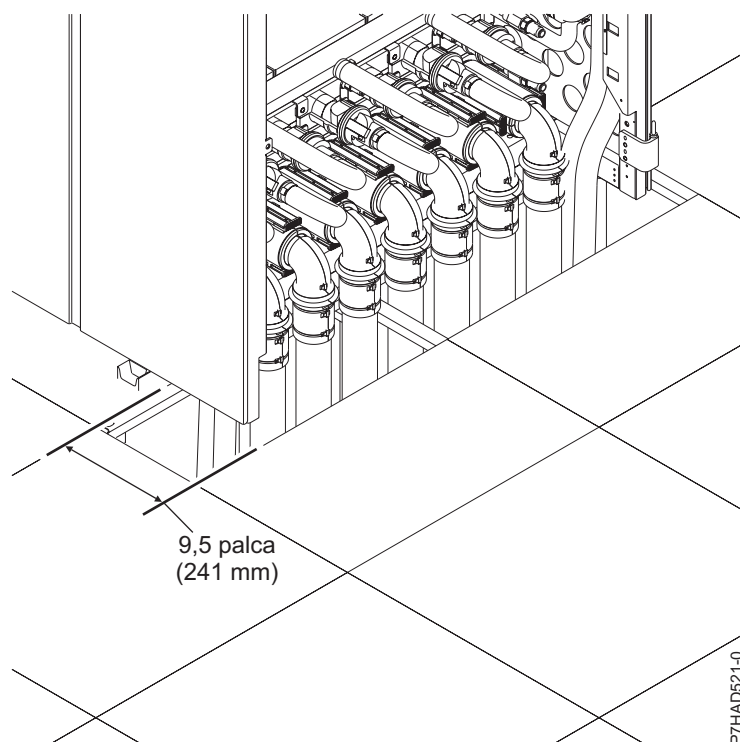
Obrázok 3. Otvor v podlahe
