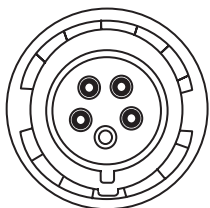
Obrázok 36. Zapojenie zástrčky
