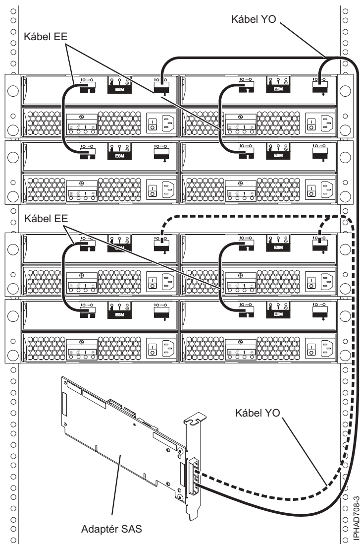
Obrázok 147. Adaptér SAS k štyrom rozširujúcim zásuvkám disku
