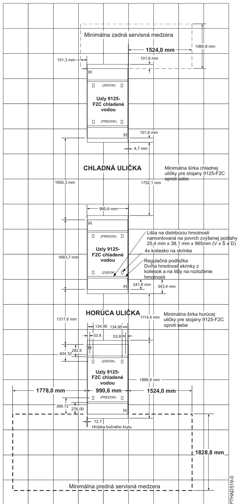
Obrázok 1. Servisné medzery pre jeden stojan - horúca a chladná ulička
