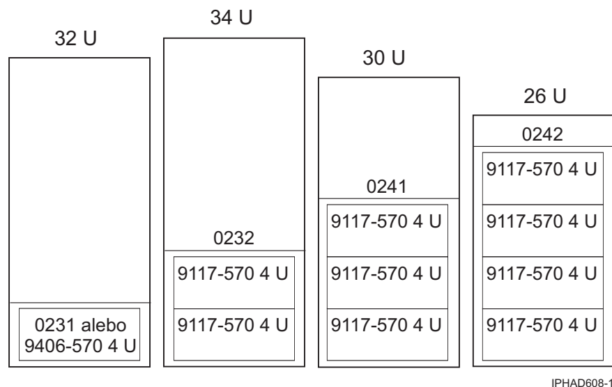
Obrázok 12. 570 v stojane
