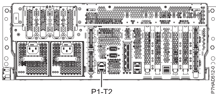
Obrázok 137. Pohľad zozadu na 8202-E4B, 8202-E4C, 8202-E4D, 8205-E6B, 8205-E6C a 8205-E6D s miestom inštalácie kábla
