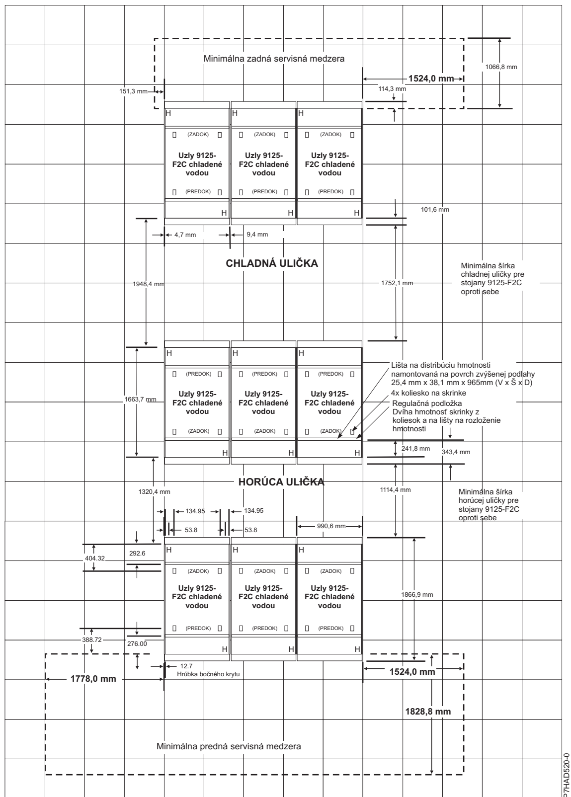
Obrázok 2. Servisné medzery pre viacero stojanov - horúca a chladná ulička
