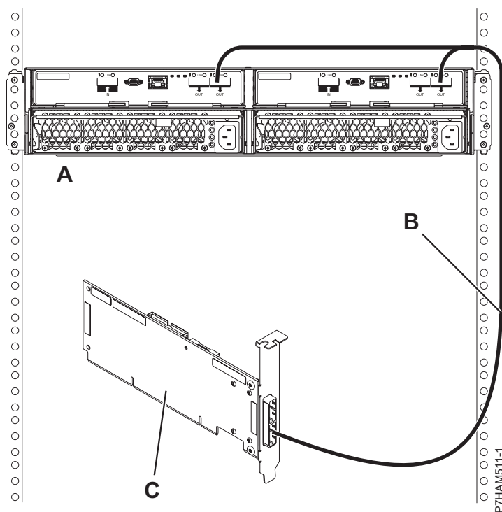
Obrázok 164. Pripojenie v režime 1 zásuvky 5887 pomocou kábla YO k jednému adaptéru SAS
