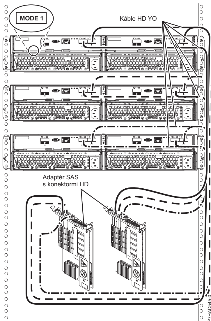
Obrázok 175. Pripojenie v režime 1 troch zásuviek 5887 k dvom adaptérom SAS s konektormi HD
