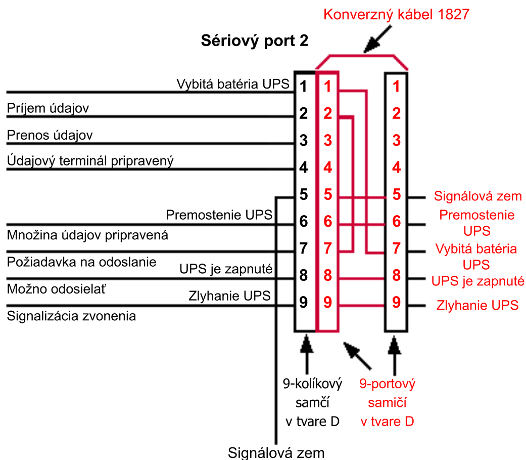
Obrázok 132. Zapojenie kábla 1827
