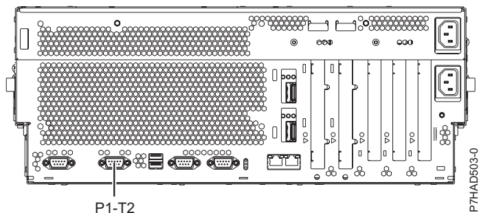
Obrázok 134. Pohľad zozadu na 8233-E8B a 8236-E8C s miestom inštalácie kábla
