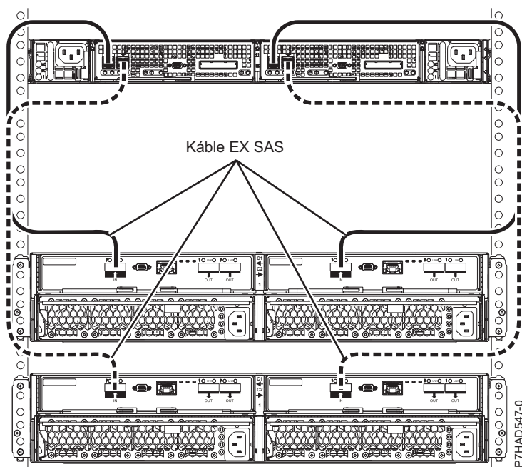
Obrázok 178. Pripojenie dvoch zásuviek 5887 pomocou káblov HD EX k jednému EDR1
