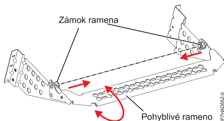
Obrázok 141. Konzola na organizáciu káblov
