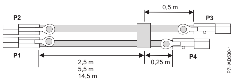
Obrázok 142. Dĺžky káblov zostavy externých káblov X SAS
