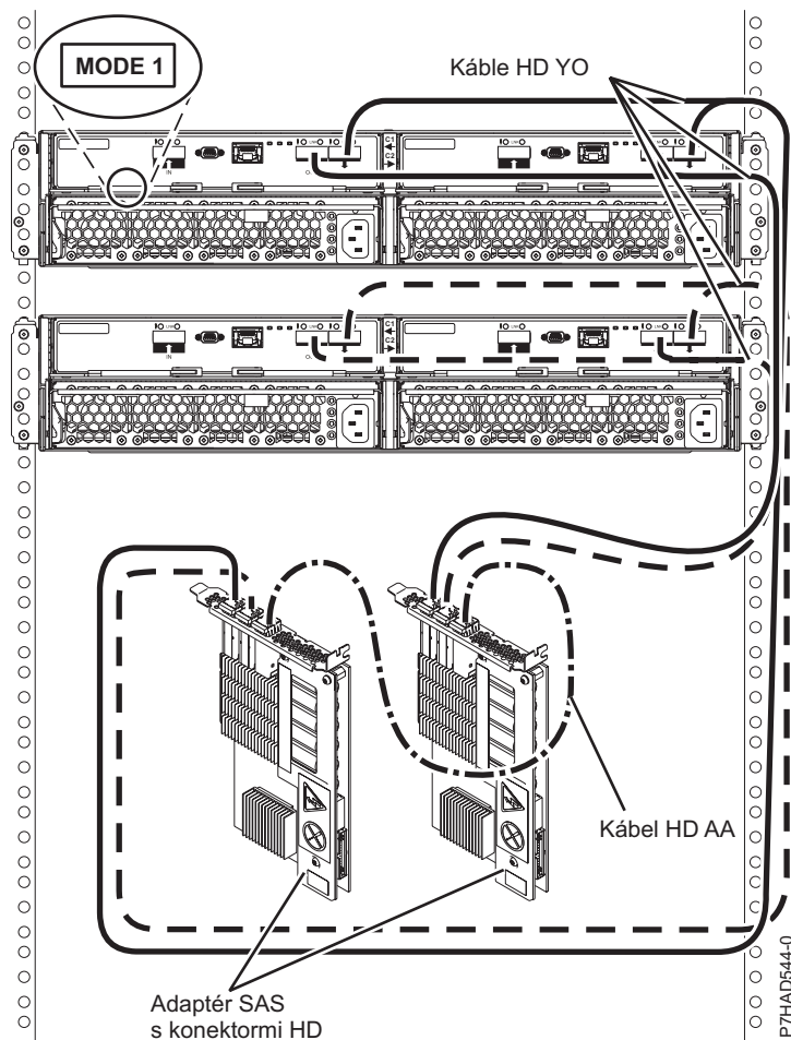
Obrázok 174. Pripojenie v režime 1 dvoch zásuviek 5887 pomocou konektorov HD k dvom adaptérom SAS
