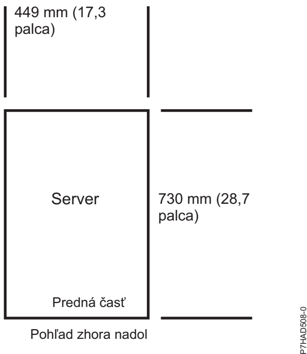
Obrázok 1. Pôdorys modelu 8202-E4B, 8202-E4C, 8202-E4D, 8205-E6B, 8205-E6C a 8205-E6D (servery namontované v stojane)
