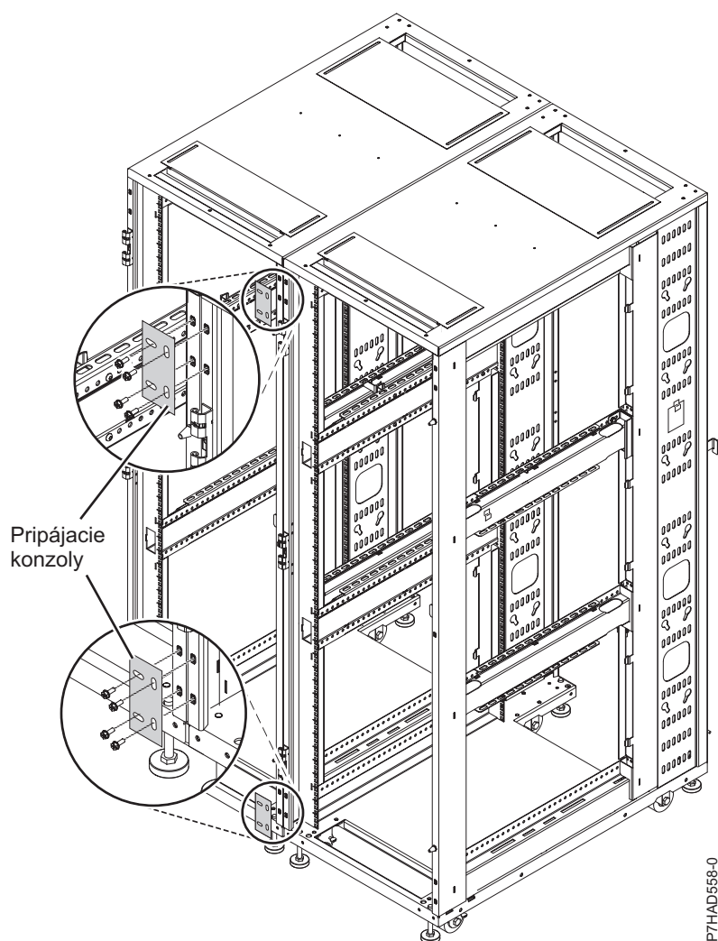
Obrázok 29. Pripájacie konzoly
