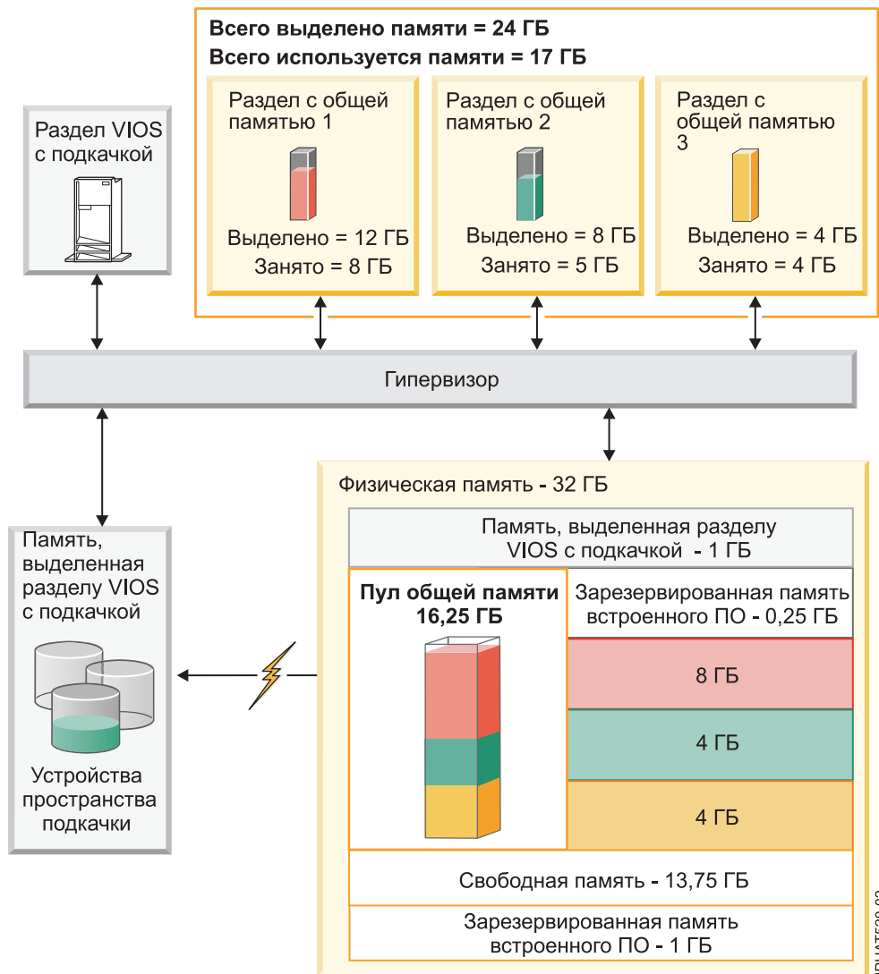
Рисунок 2. Сервер с физически невозполнимой конфигурацией общей памяти
