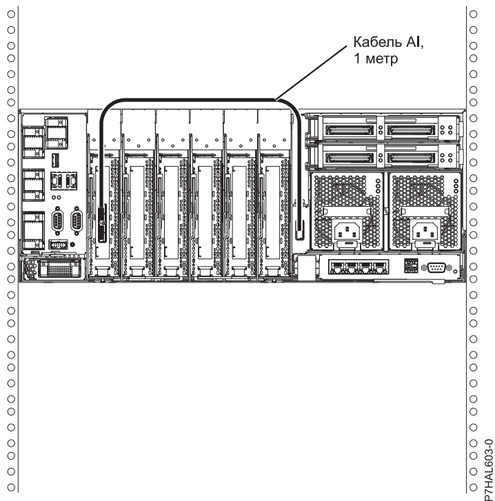
Рисунок 147. Подключение адаптера SAS к внутренним разъемам дисков SAS через внешний порт SAS системы
