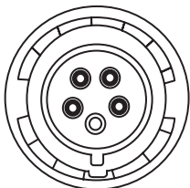
Рисунок 31. Распайка вилки
