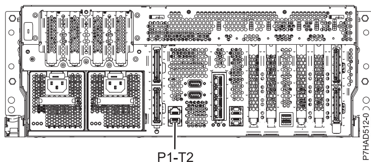
Рисунок 132. 8202-E4B, 8202-E4C, 8202-E4D, 8205-E6B, 8205-E6C и 8205-E6D с разъемом для подключения кабеля (вид сзади)
