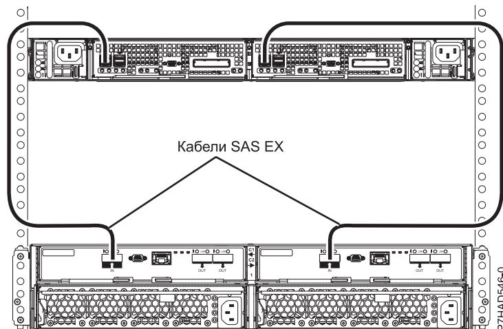
Рисунок 172. Подключение одного блока 5887 с помощью кабелей HD EX к одному EDR1
