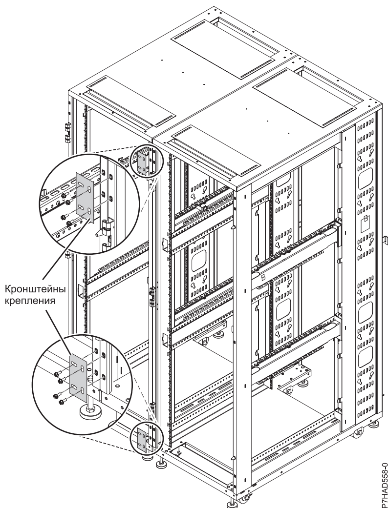
Рисунок 28. Кронштейны крепления
