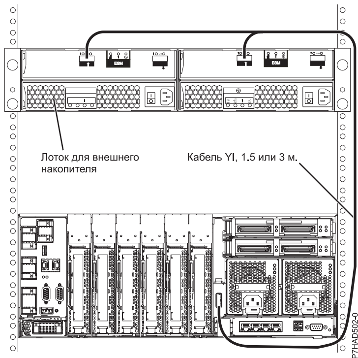
Рисунок 146. Подключение внешнего порта адаптера SAS системы к блоку расширения для дисков (модели 9117-MMB и 9179-MHB).
