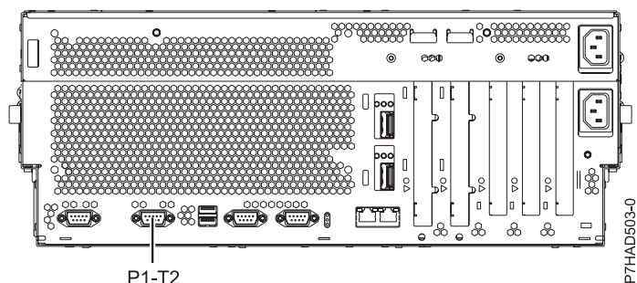
Рисунок 129. 8233-E8B и 8236-E8C, вид сзади с разъемом для подключения кабеля
