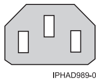
Рисунок 119. Розетка, тип 15
