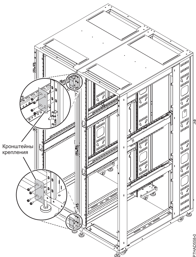
Рисунок 28. Кронштейны крепления
