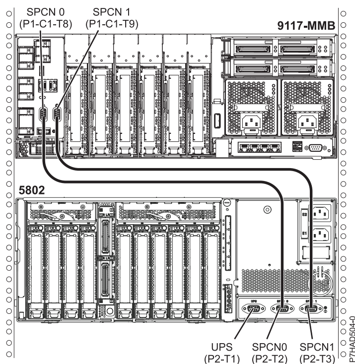
Рисунок 130. Расположение установки кабелей 8412-EAD, 9117-MMB, 9117-MMC, 9117-MMD, 9179-MHB, 9179-MHC, 9179-MHD и 5208 или 5877, вид сзади
