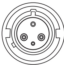
Рисунок 35. Розетка, тип IEC 60309 3P+N+E
