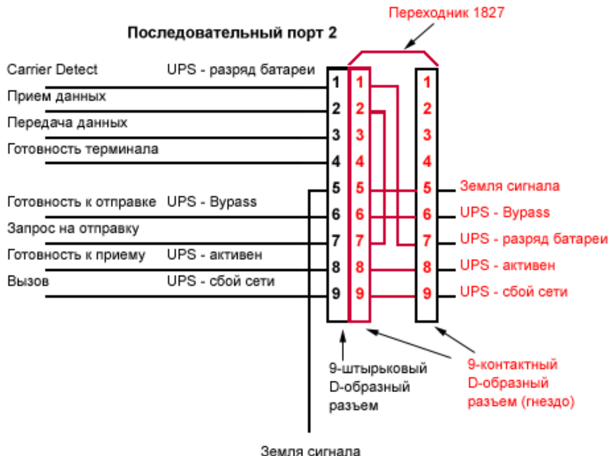
Рисунок 128. Подключение кабеля 1827
