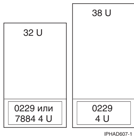
Рисунок 6. Код компонента 7884: 9406-520 и 9111-520 в стойке
