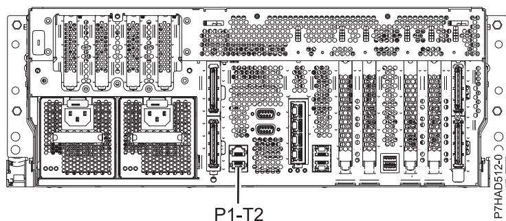
Рисунок 133. 8202-E4B, 8202-E4C, 8202-E4D, 8205-E6B, 8205-E6C и 8205-E6D с разъемом для подключения кабеля (вид сзади)
