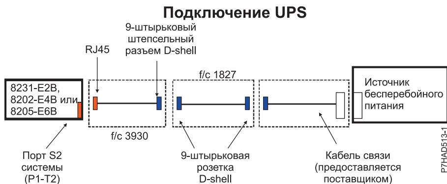
Рисунок 134. Подключение источника бесперебойного питания для 8202-E4B, 8202-E4C, 8205-E6B, 8205-E6C, 8231-E2B, 8231-E1C, 8231-E1D, 8231-E2C, 8231-E2D и 8268-E1D
