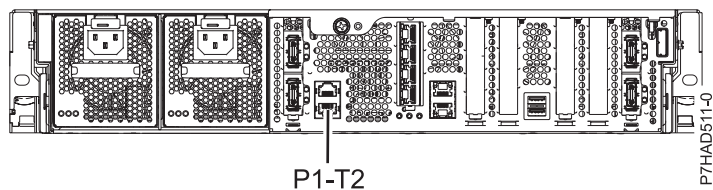
Рисунок 132. 8231-E2B, 8231-E1C, 8231-E1D, 8231-E2C, 8231-E2D и 8268-E1D, вид сзади с разъемом для подключения кабеля
