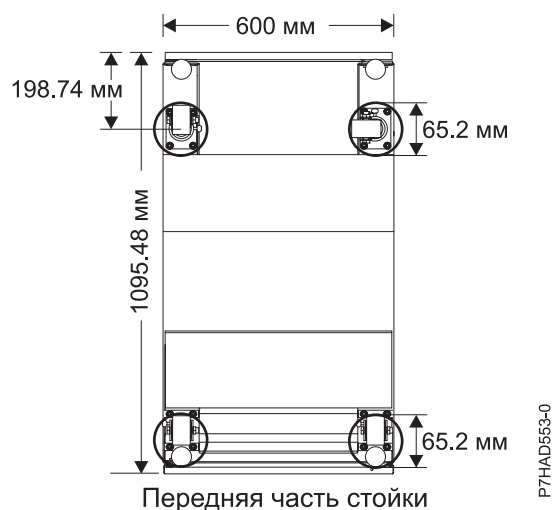
Рисунок 24. Расположения роликов
