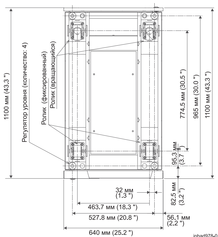
Рисунок 5. Расположения роликов и регуляторов уровня
