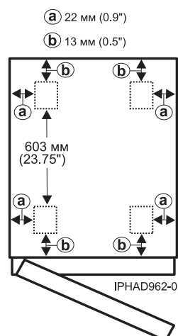
Рисунок 18. Расположения роликов для моделей 0554 и 7014-S11
