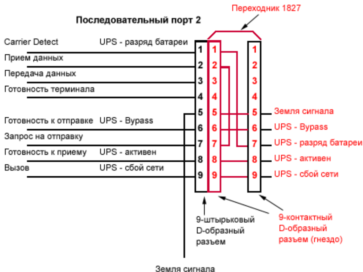
Рисунок 128. Подключение кабеля 1827
