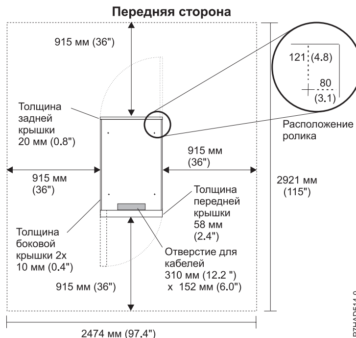
Рисунок 23. Зона обслуживания и ролики для стоек 7014-T00, 7014-T42 и 0553.
