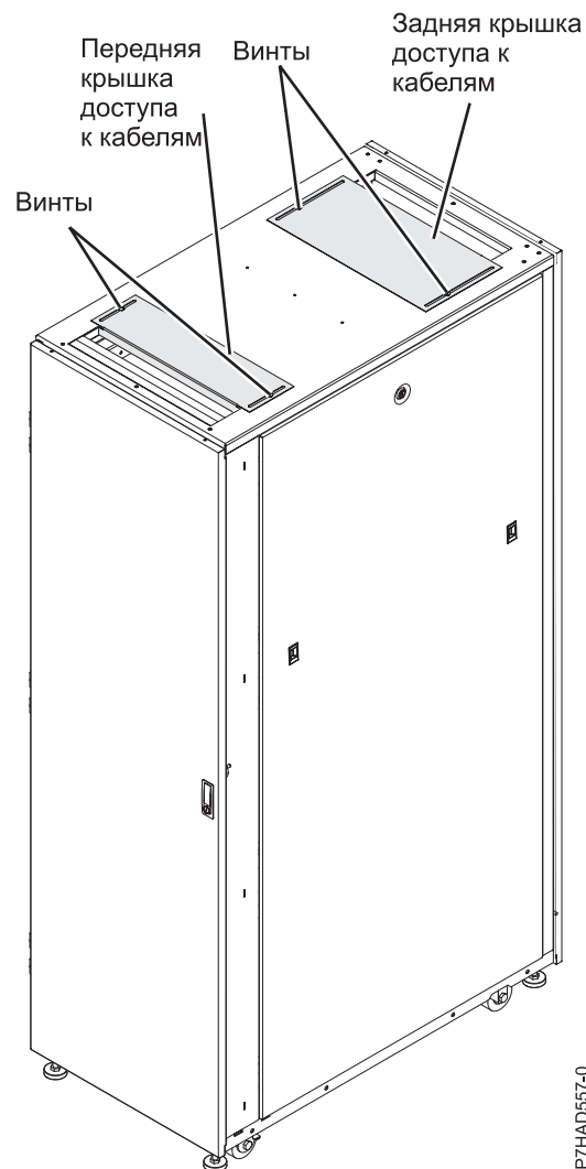
Рисунок 27. Крышки доступа к кабелям
