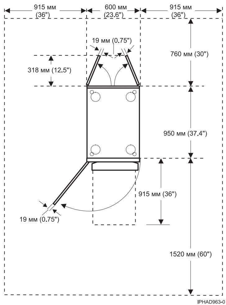
Рисунок 20. Схема расположения модели 0555 и 7014-S25
