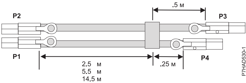
Рисунок 138. Длины внешних кабелей X SAS с разъемами
