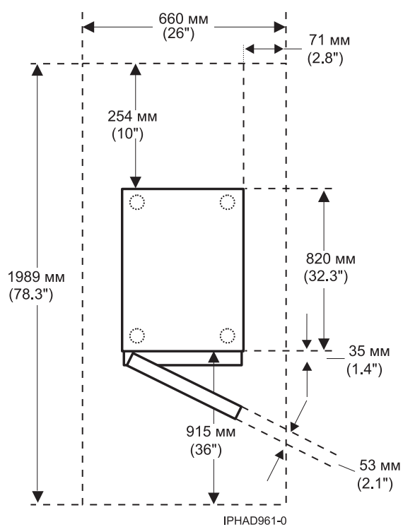
Рисунок 17. Схема расположения модели 0554 и 7014-S11
