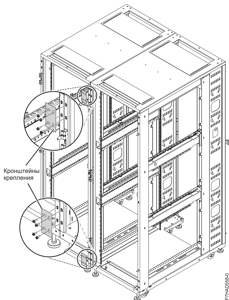
Рисунок 29. Кронштейны крепления
