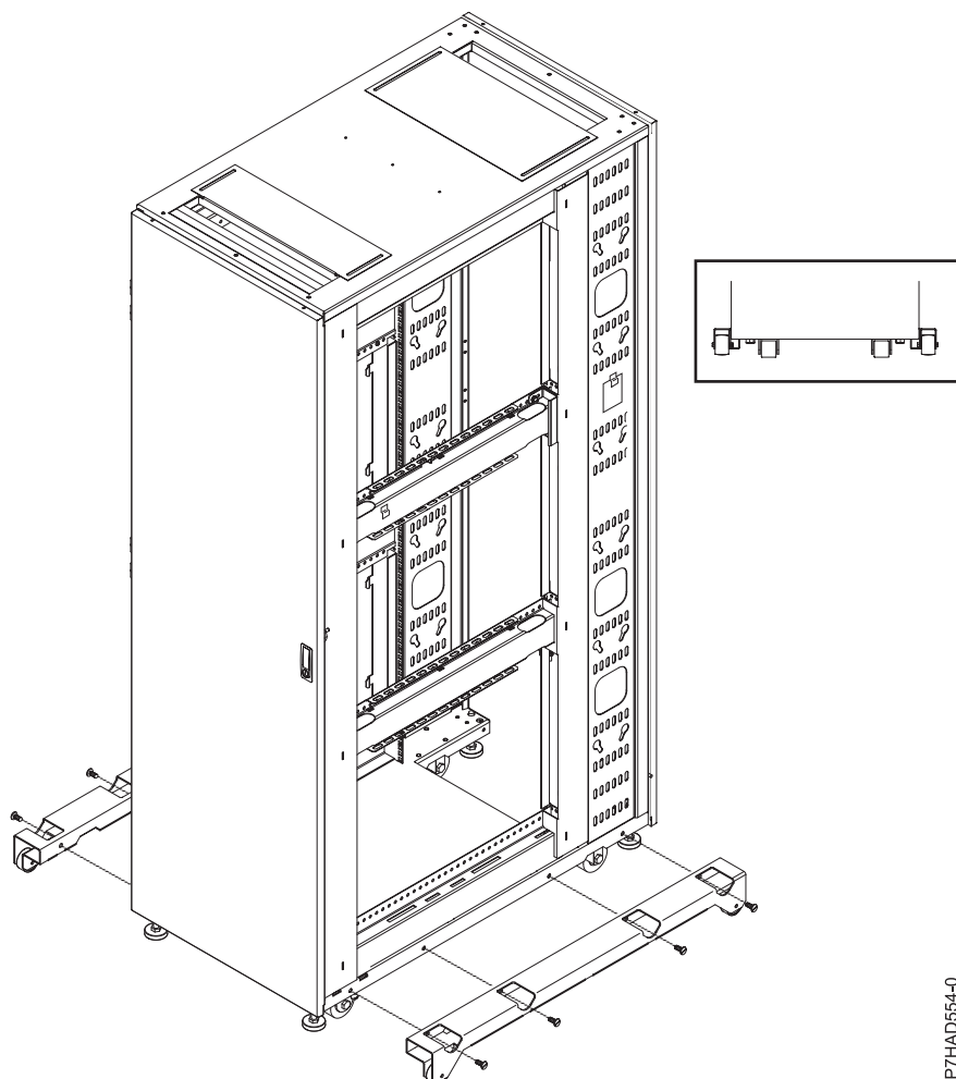
Рисунок 28. Расположения боковых опор
