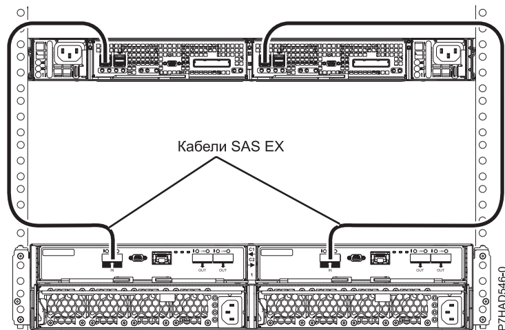
Рисунок 173. Подключение одного блока 5887 с помощью кабелей HD EX к одному EDR1
