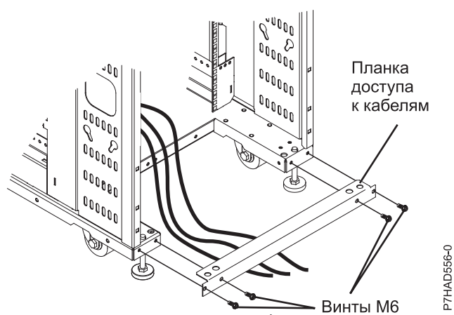
Рисунок 26. Планка доступа к кабелям
