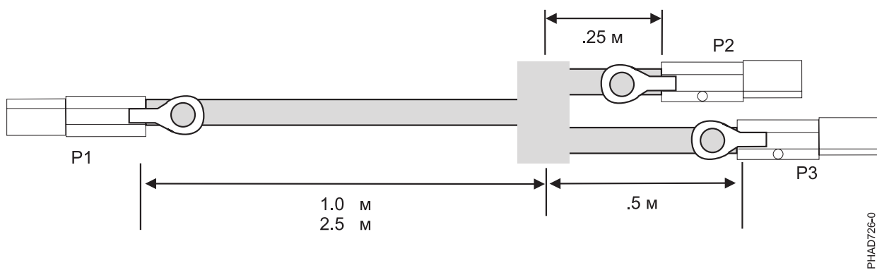
Рисунок 140. Длины внешних кабелей YI SAS
