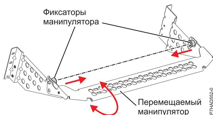
Рисунок 137. Кронштейн управления кабелями
