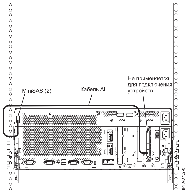
Рисунок 149. Адаптер FC5904 или FC5908, подключенный к блокам расширения диска
