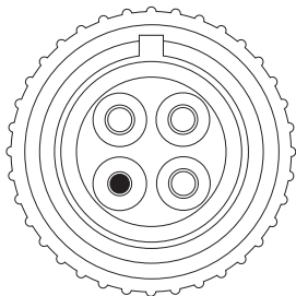
Рисунок 114. Вилка, тип RS 7328DP
