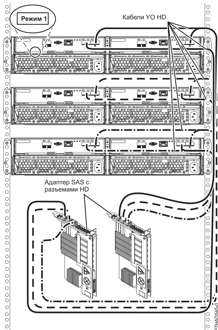
Рисунок 171. Подключение трех блоков 5887 к двум адаптерам SAS с помощью разъемов HD, режим 1
