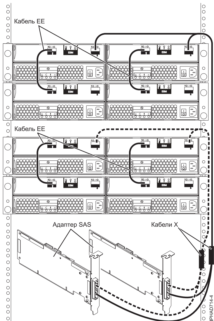
Рисунок 152. Подключение четырех адаптеров RAID SAS к двум блокам расширения дисковой памяти в конфигурации RAID мультиинициатора высокой готовности
