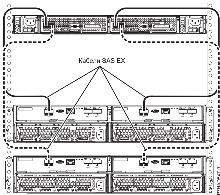
Рисунок 174. Подключение двух блоков 5887 с помощью кабелей HD EX к одному EDR1
