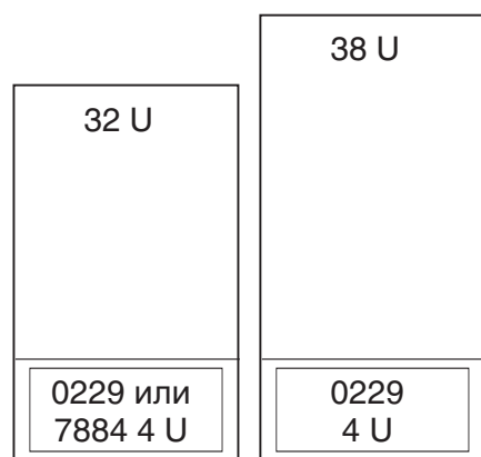
Рисунок 6. Код компонента 7884: 9406-520 и 9111-520 в стойке
