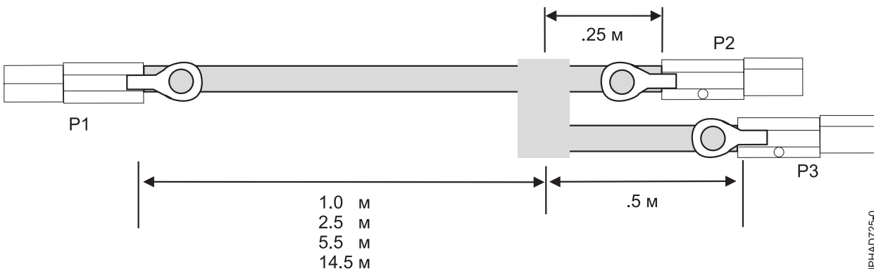
Рисунок 139. Длины внешних кабелей YO SAS
