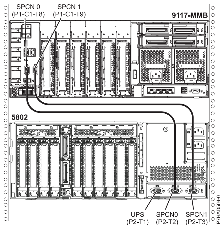
Рисунок 131. Расположение установки кабелей 8412-EAD, 9117-MMB, 9117-MMC, 9117-MMD, 9179-MHB, 9179-MHC, 9179-MHD и 5208 или 5877, вид сзади
