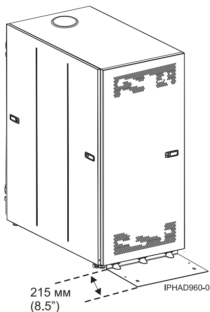
Рисунок 19. Модели 0555 и 7014-S25 с опорами стабилизации
