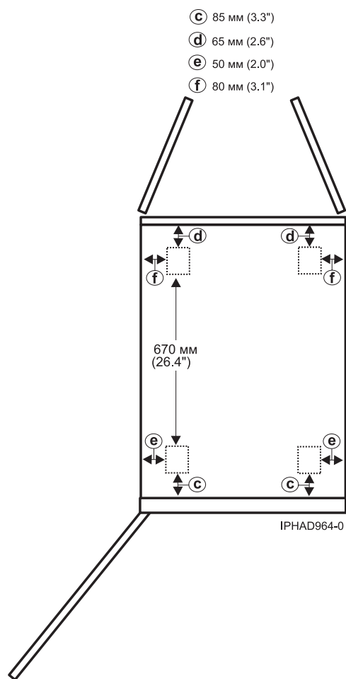
Рисунок 21. Расположения роликов для моделей 0555 и 7014-S25
