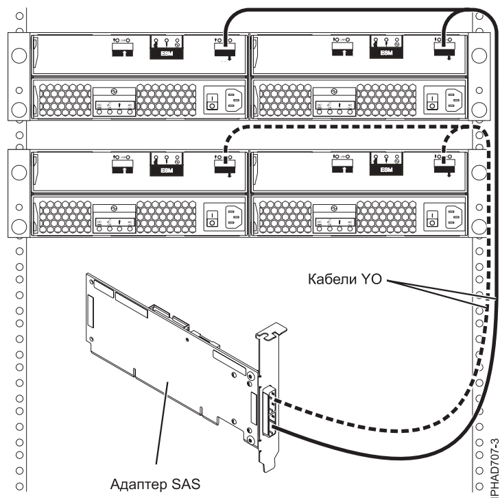
Рисунок 142. Подключение адаптера SAS к двум блокам расширения для дисков
