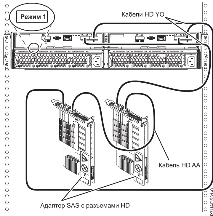
Рисунок 169. Подключение блока 5887 к двум адаптерам SAS с помощью разъемов HD, режим 1
