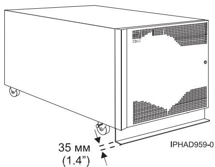
Рисунок 16. Модели 0554 и 7014-S11 с планками стабилизации
