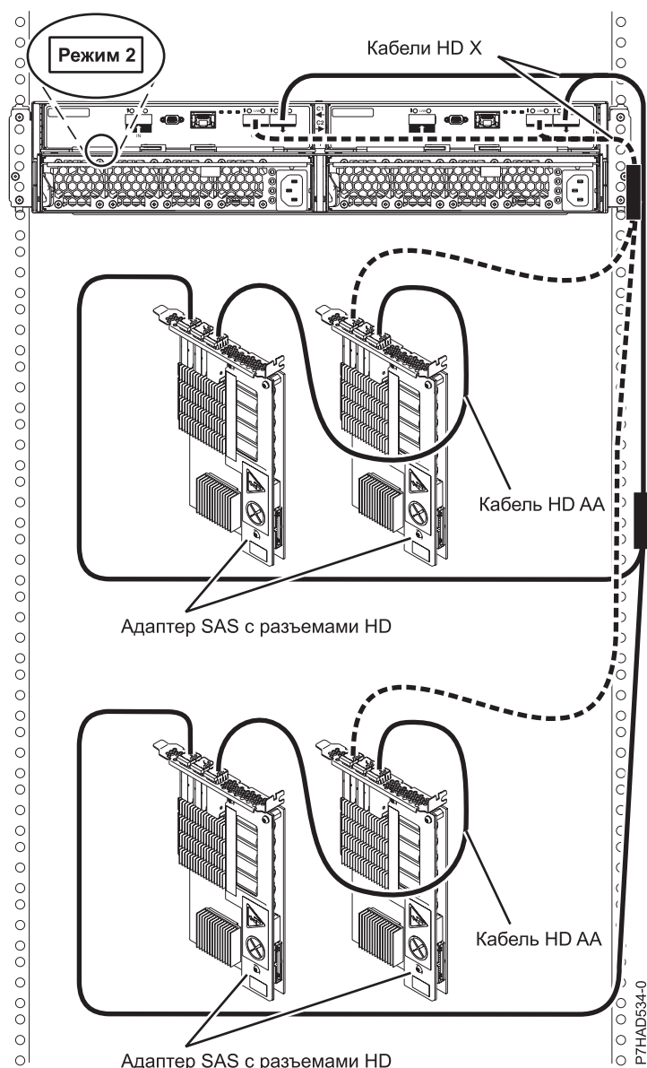
Рисунок 172. Подключение блока 5887 к двум парам адаптерам SAS с помощью разъемов HD, режим 2
