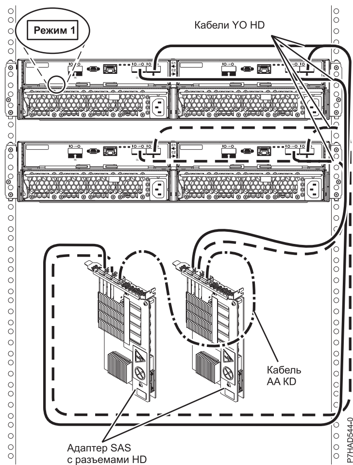
Рисунок 170. Подключение двух блоков 5887 к двум адаптерам SAS с помощью разъемов HD, режим 1
