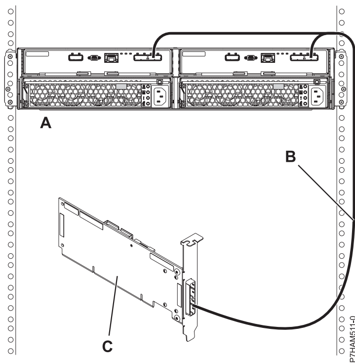
Рисунок 160. Подключение блока 5887 к одному адаптеру SAS с помощью кабеля YO, режим 1
