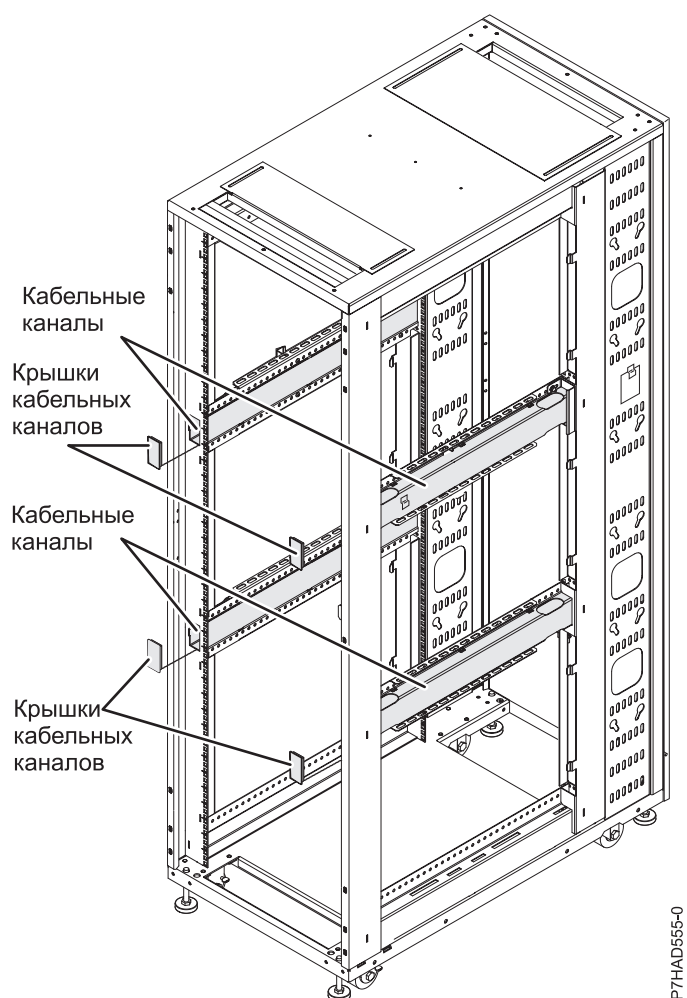
Рисунок 25. Прокладка кабелей внутри стойки
