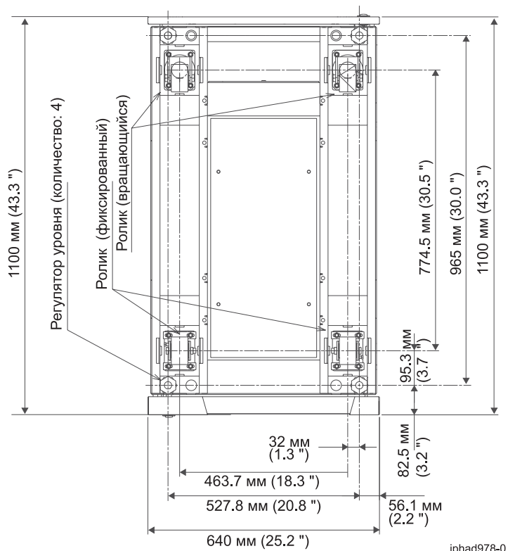
Рисунок 22. Расположения роликов и регуляторов уровня
