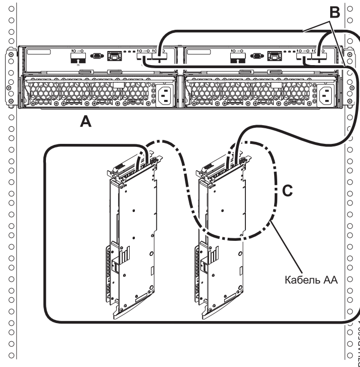
Рисунок 168. Подключение блока 5887 к двум адаптерам SAS с помощью кабелей YO, режим 1
