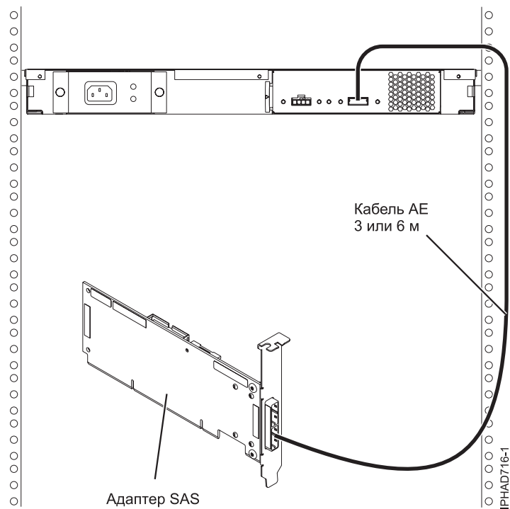
Рисунок 145. Подключение адаптера SAS к блоку расширения для внешних накопителей
