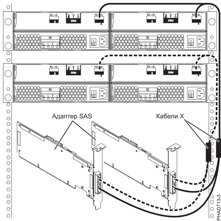
Рисунок 151. Подключение двух адаптеров RAID SAS к двум блокам расширения дисковой памяти в конфигурации RAID мультиинициатора высокой готовности
