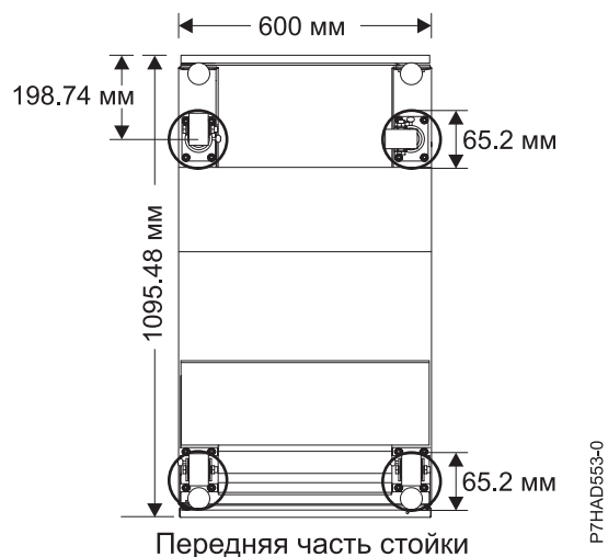
Рисунок 24. Расположения роликов
