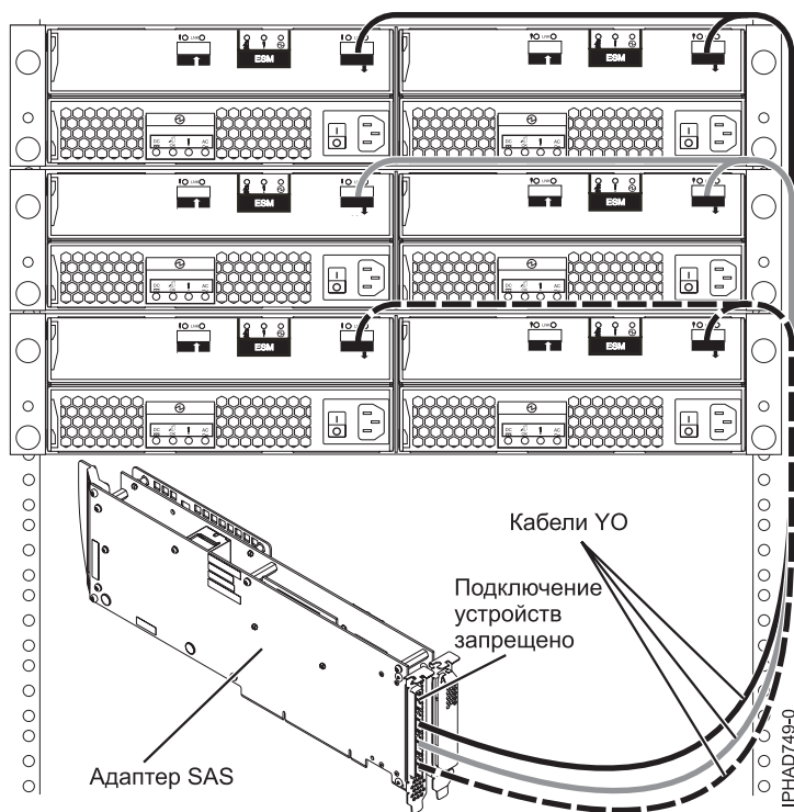
Рисунок 144. Подключение трехпортового адаптера SAS к блокам расширения для дисков
