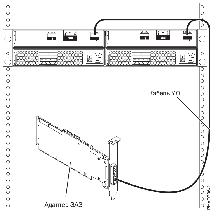
Рисунок 141. Подключение адаптера SAS к блоку расширения для дисков
