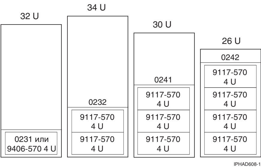
Рисунок 8. 570 в стойке
