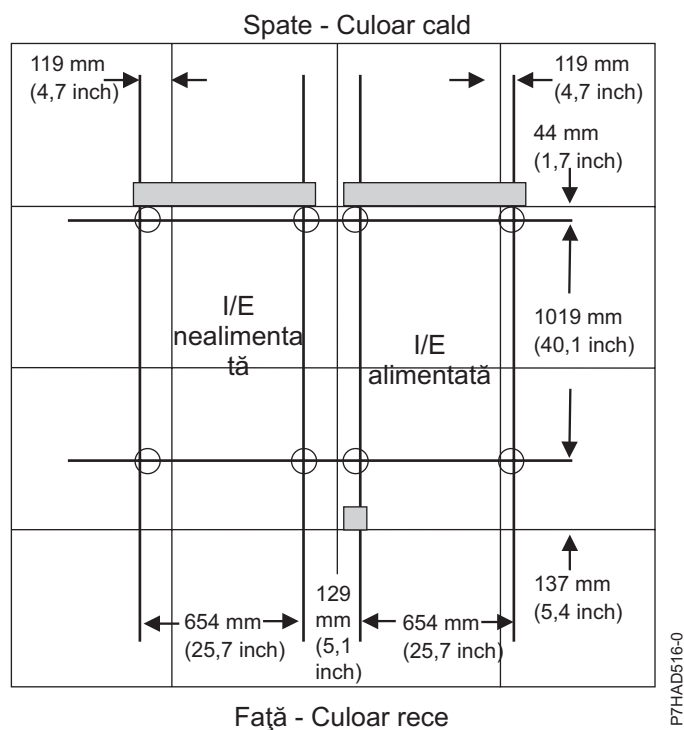
Figura 70. Amplasarea dulapului pentru plăci de 600 mm (23,6 inch)
