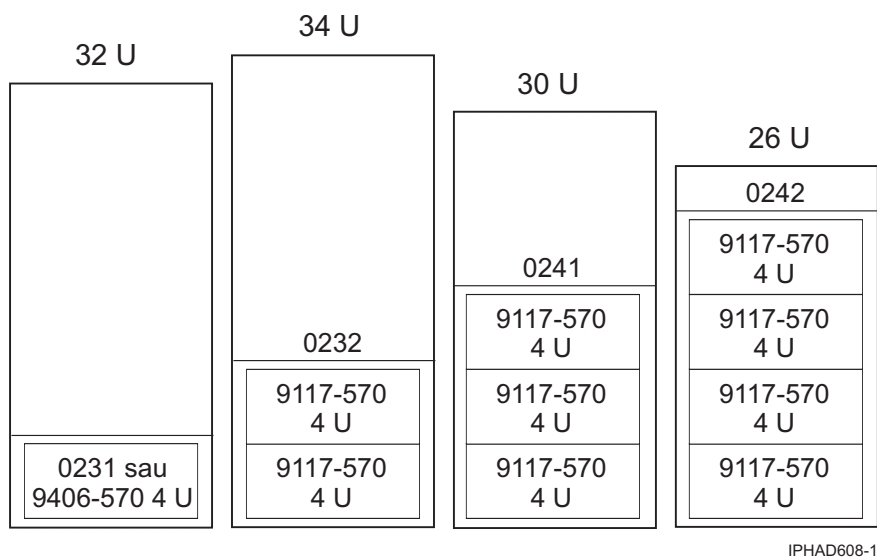
Figura 81. 570 în dulap
