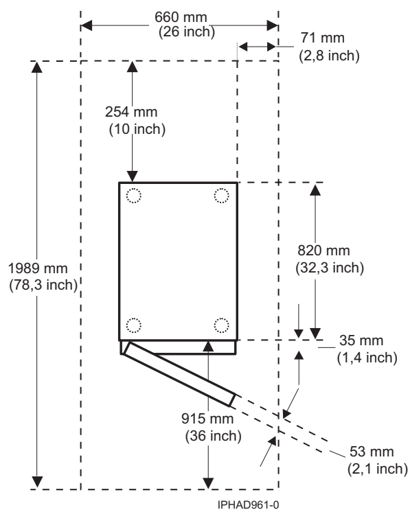
Figura 90. Vedere în plan pentru modelul 0554 și 7014-S11
