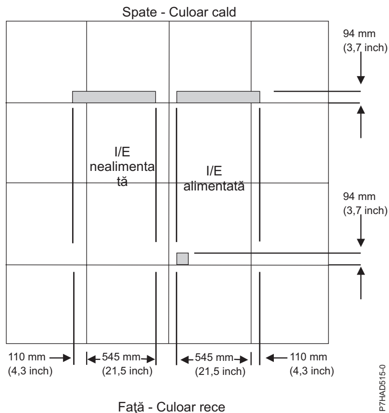
Figura 63. Amplasarea decupărilor pentru cabluri pentru două dulapuri la plăci de 610 mm (24 inch)
