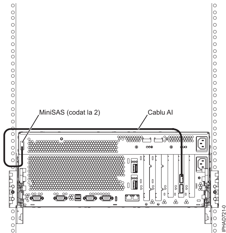
Figura 221. Adaptorul SAS la sloturi de disc SAS intern prin portul SAS extern al sistemului
