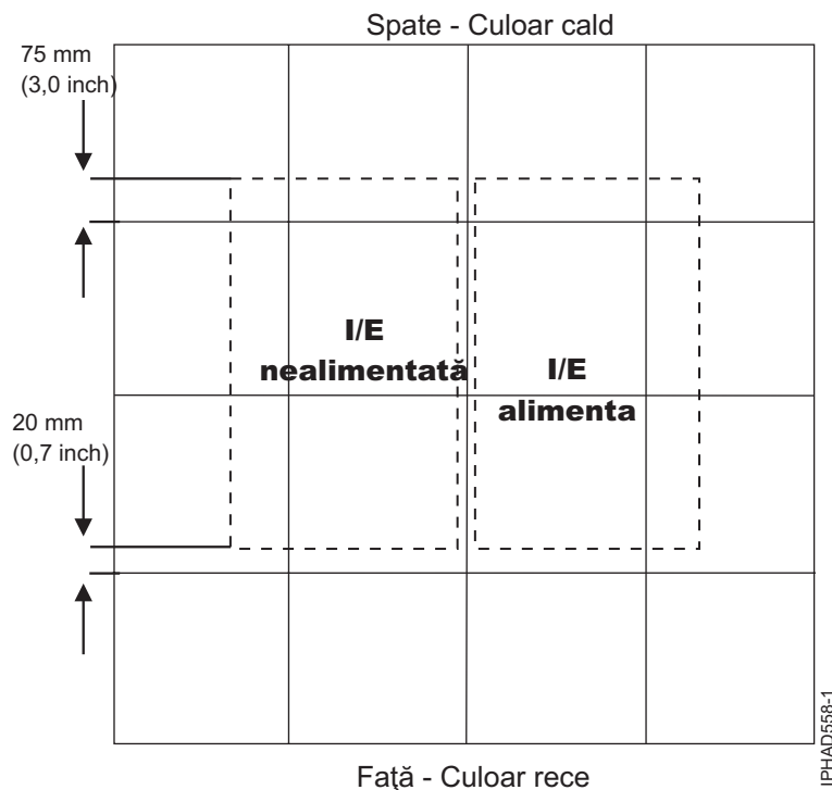
Figura 62. Amplasarea a două dulapuri pe plăci de 610 mm (24 inch)
