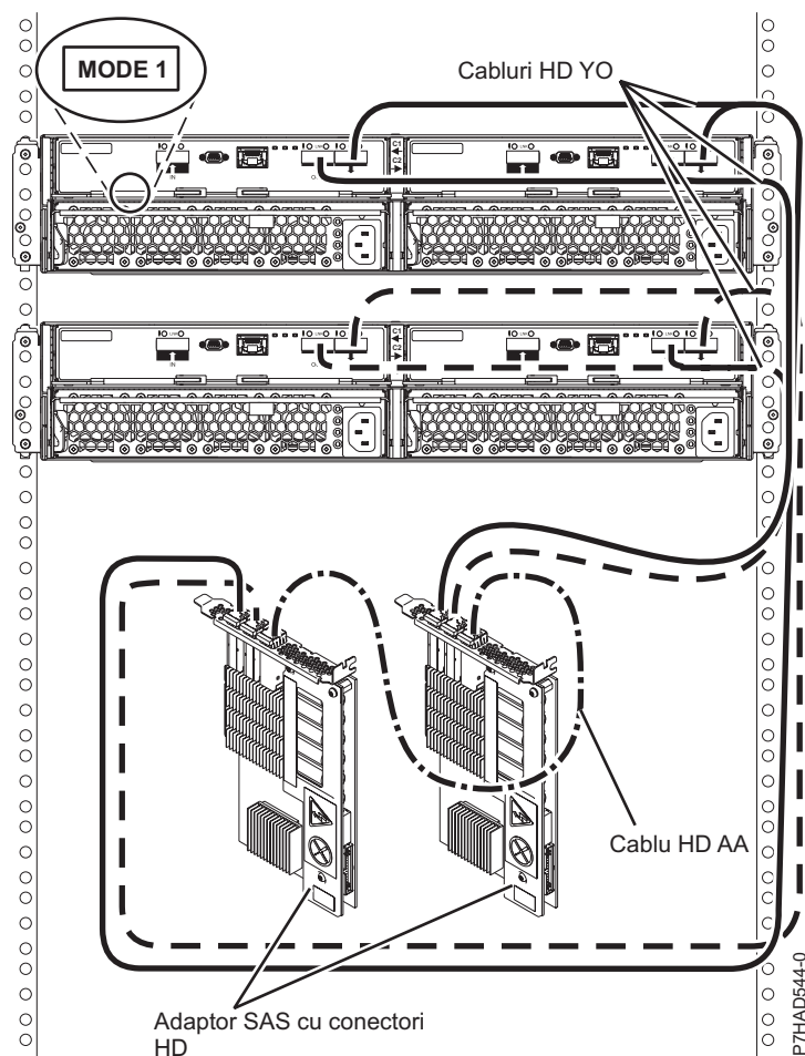
Figura 243. Conectarea de mod 1 a două sertare 5887 utilizând conectori HD la două adaptoare SAS
