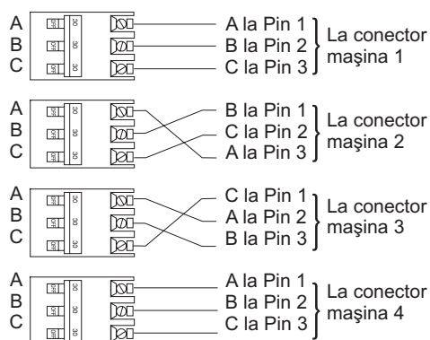
Figura 56. Echilibrarea sarcinii panoului de alimentare
