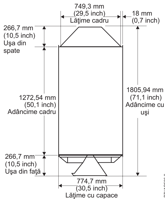
Figura 37. Vedere în plan pentru sisteme cu un cadru și uși acustice
