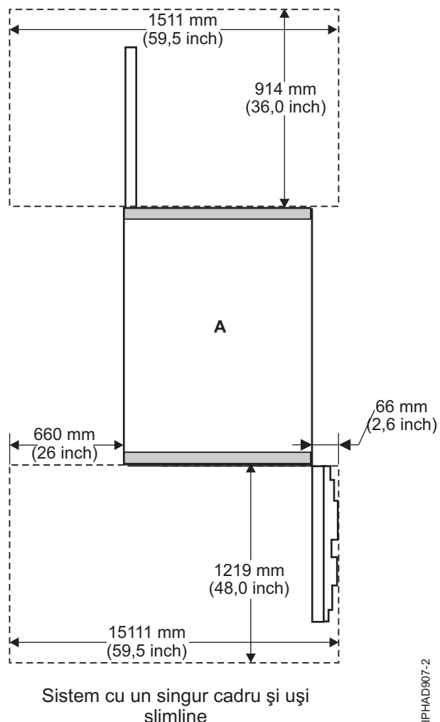
Figura 41. Spațiu de acces pentru service pentru un cadru de unitate de sistem sau un dulap I/E cu uși slimline
