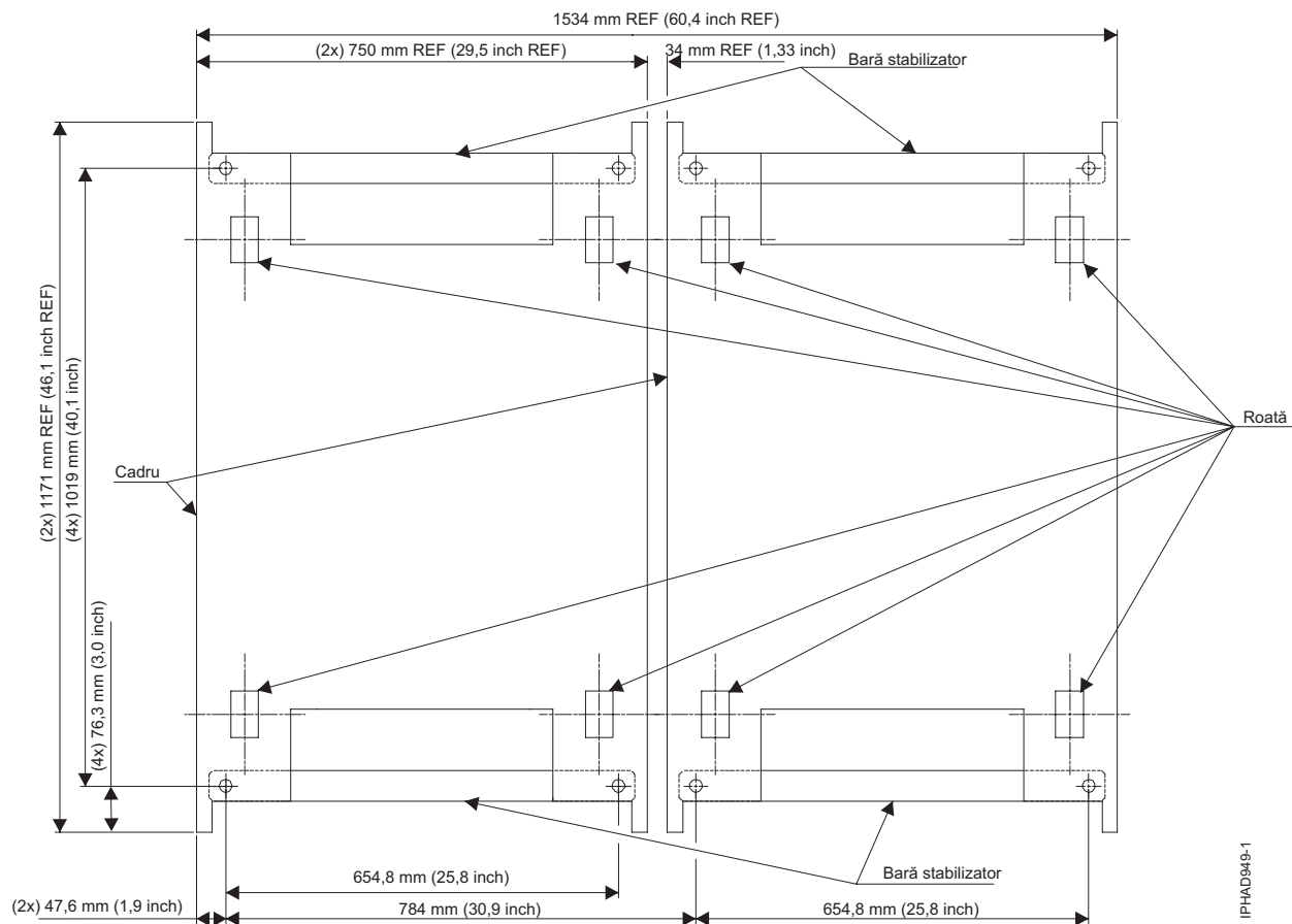
Figura 20. Dispunerea barei de stabilizare (vedere de sus)
