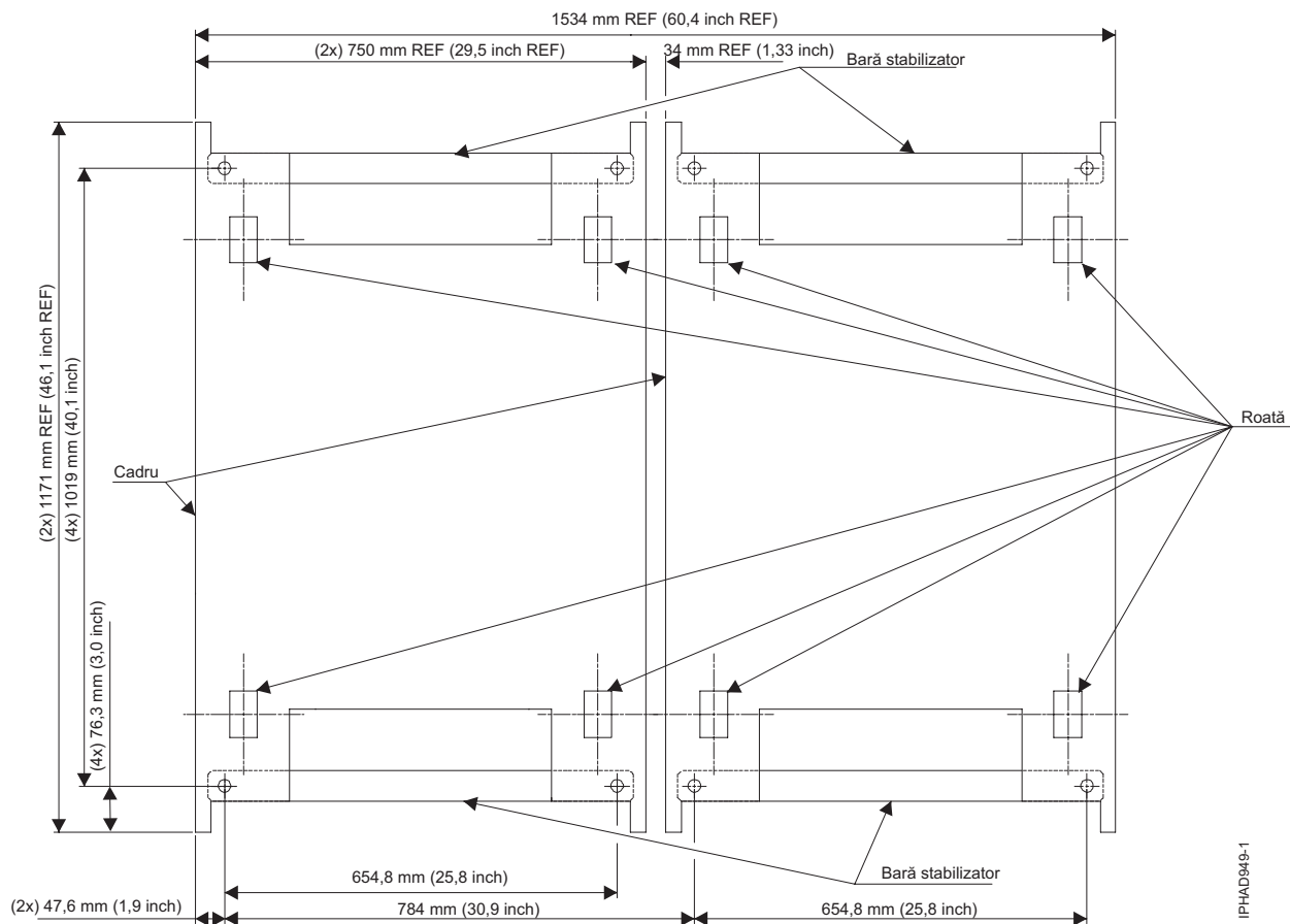
Figura 50. Dispunerea barei de stabilizare (vedere de sus)
