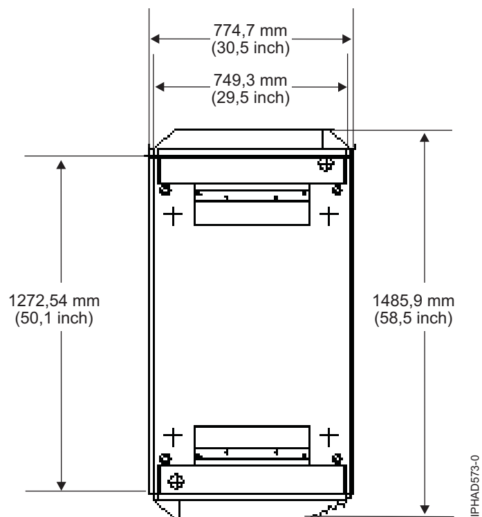
Figura 39. Vedere în plan pentru sisteme cu un cadru și uși slimline
