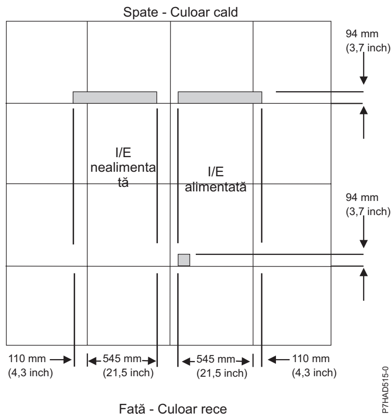
Figura 69. Amplasarea decupărilor pentru două cabluri la plăci de 600 mm (23,6 inch)
