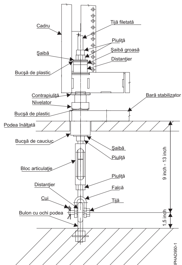
Figura 51. Accesorii de fixare a cadrului ansamblu întinzător cu filet pentru podea înălțată de 228,6 - 330,2 mm (9 - 13 inch) (număr parte componentă 44P2999)
