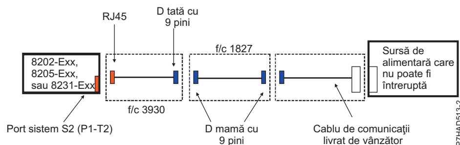
Figura 207. Cablarea sursei de alimentare neîntreruptibilă pentru 8202-E4B, 8202-E4C, 8205-E6B, 8205-E6C, 8231-E2B, 8231-E1C, 8231-E1D, 8231-E2C, 8231-E2D și 8268-E1D
