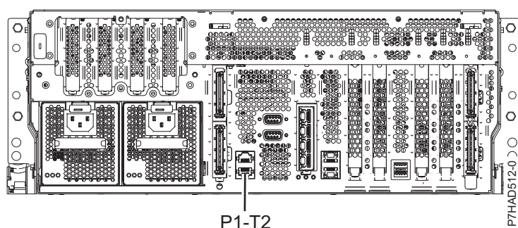
Figura 206. Vedere din spate cu locația instalării cablurilor pentru 8202-E4B, 8202-E4C, 8202-E4D, 8205-E6B, 8205-E6C și 8205-E6D
