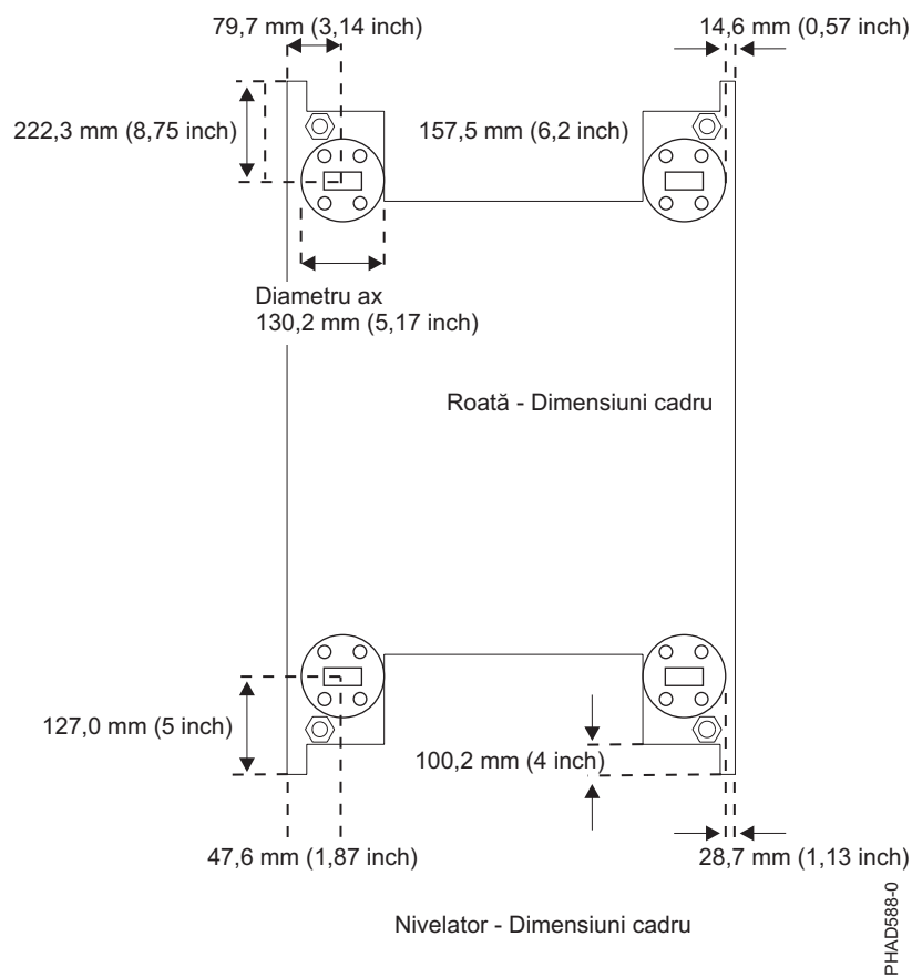
Figura 40. Suport de nivelare și dimensiunile cadrului
