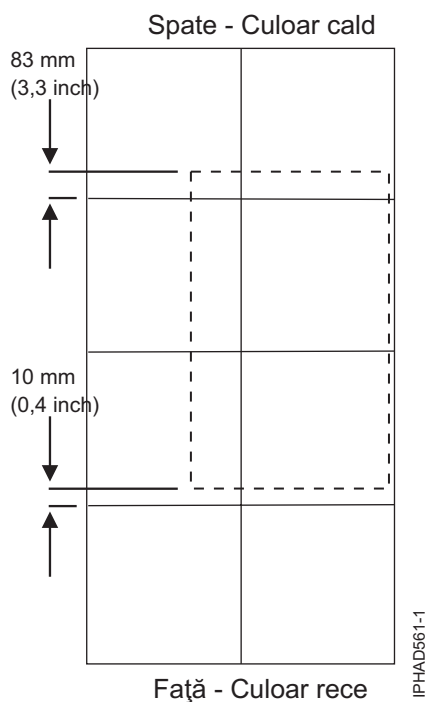
Figura 13. Amplasarea dulapului pentru plăci de 600 mm (23,6 inch)
