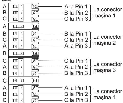
Figura 57. Echilibrarea sarcinii panoului de alimentare
