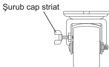
Figura 17. Șurubul roții
