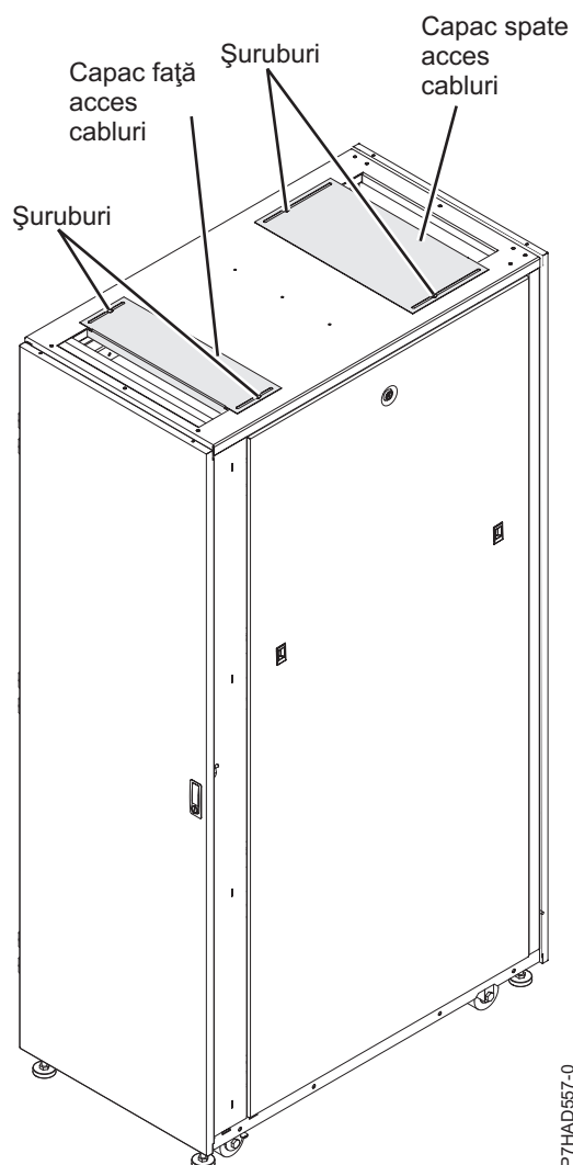
Figura 100. Capacele de acces la cabluri
