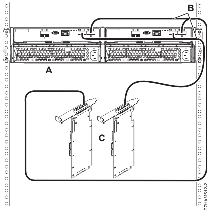
Figura 238. Conexiune mod 1 a unui sertar 5887 utilizând cabluri YO către adaptoare duble SAS
