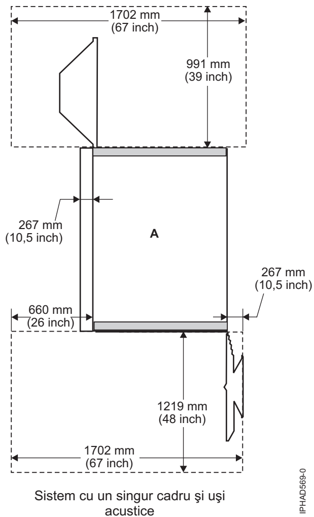
Figura 7. Spațiu de acces pentru service pentru un cadru de unitate de sistem sau un dulap I/E cu uși acustice
