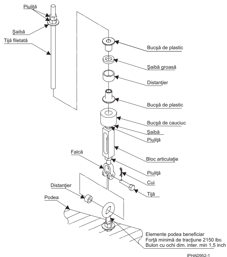
Figura 22. Accesorii de fixare a cadrului ansamblu întinzător cu filet pentru podea înălțată de 228,6 - 330,2 mm (9 - 13 inch) (număr parte componentă 44P2999)
