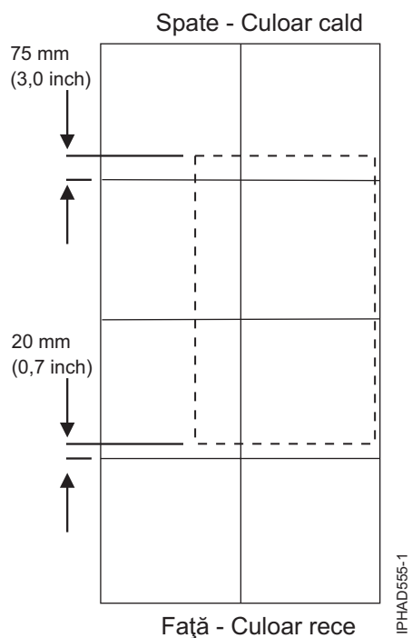
Figura 11. Amplasarea dulapului pentru plăci de 610 mm (24 inch)
