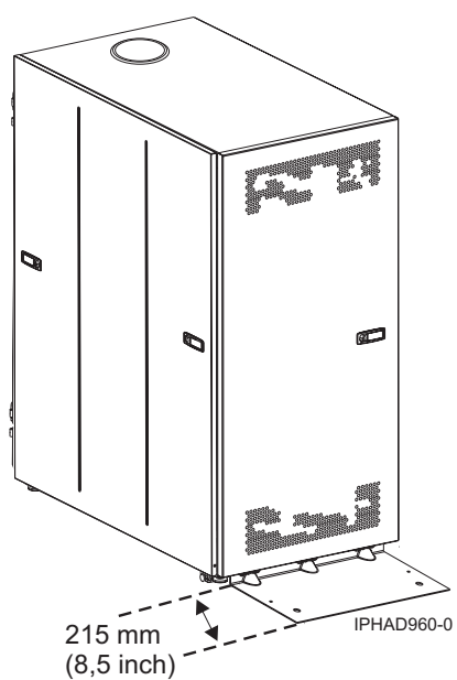
Figura 92. Model 0555 și 7014-S25 cu picior stabilizator
