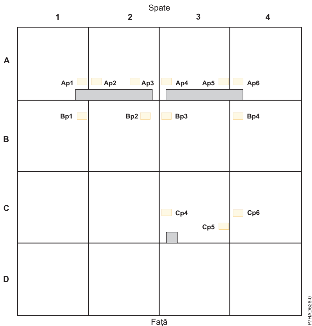
Figura 71. Amplasarea unui pedestal suplimentar
