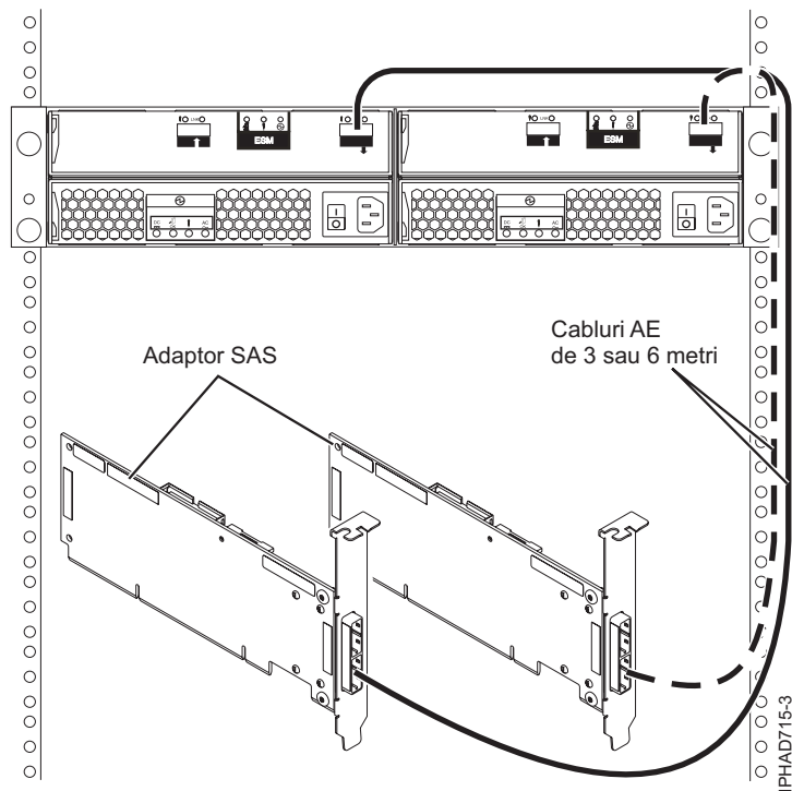
Figura 231. Două adaptoare SAS RAID la un sertar de expansiune pentru discuri într-o configurație JBOD HA inițializator multiplu
