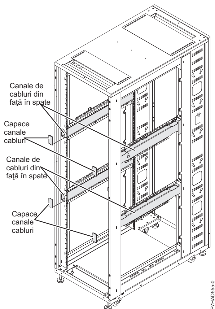
Figura 98. Cablarea în dulap
