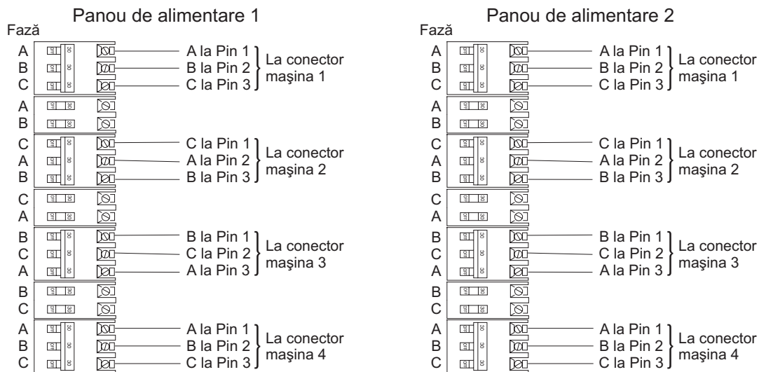
Figura 28. Echilibrarea sarcinii panoului de alimentare
