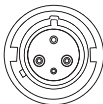
Figura 111. Tipul de priză 60309 P+N+E
