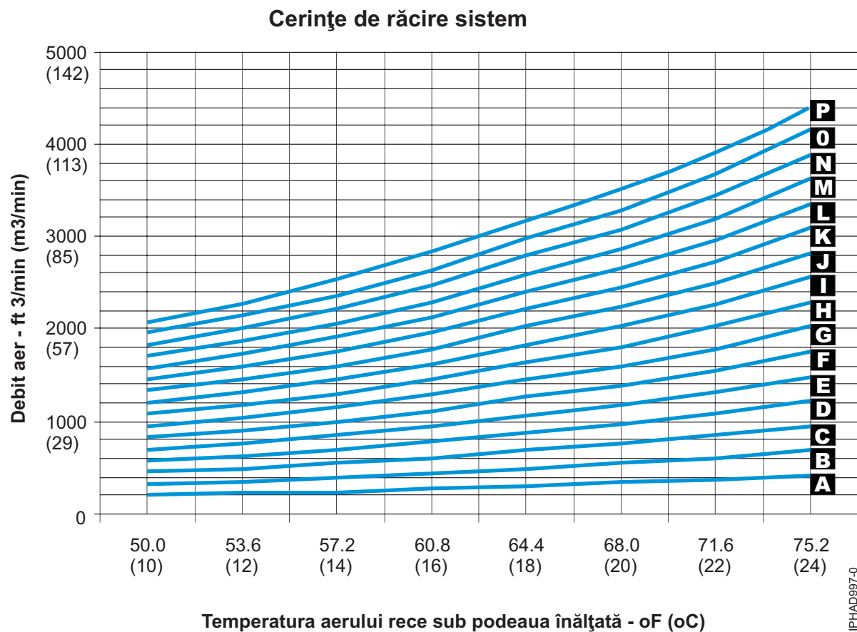
Figura 34. Cerințele de răcire
