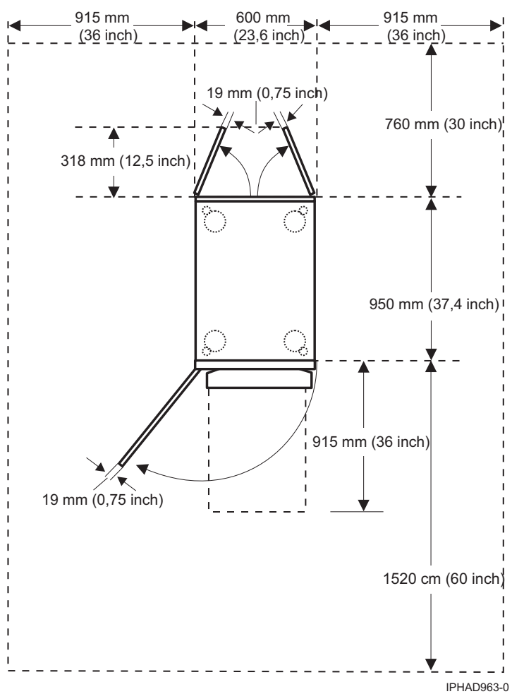
Figura 93. Vedere în plan pentru modelul 0555 și 7014-S25
