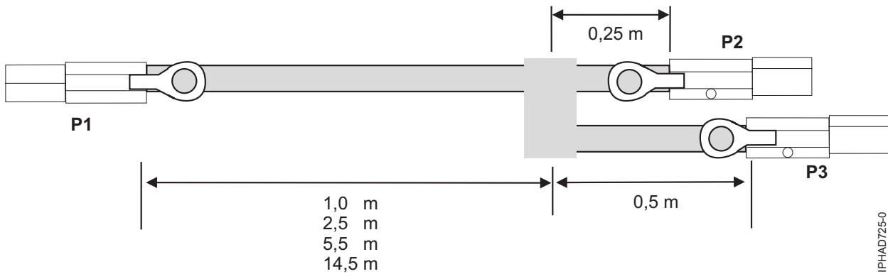
Figura 212. Lungimile de cablu pentru ansamblul cablu YO extern SAS
