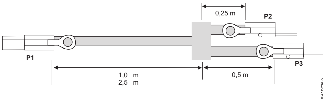
Figura 213. Lungimile de cablu pentru ansamblul cablu YI extern SAS
