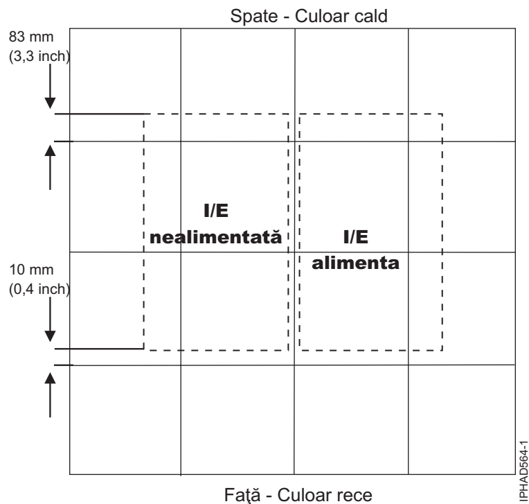
Figura 68. Amplasarea a două dulapuri pe plăci de 600 mm (23,6 inch)
