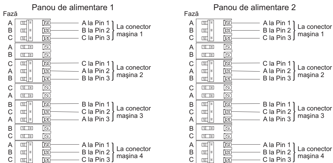
Figura 58. Echilibrarea sarcinii panoului de alimentare
