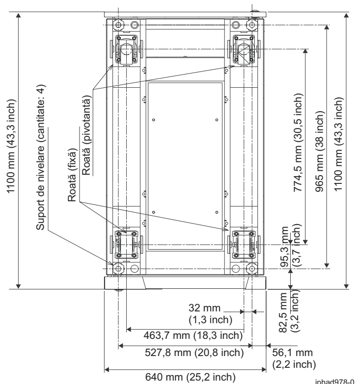
Figura 95. Locațiile roților și nivelatoarelor
