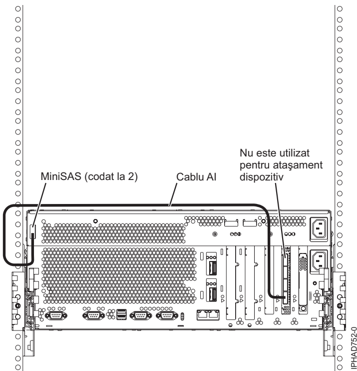
Figura 222. Adaptor FC5904 sau FC5908 atașat la sertare de expansiune pentru discuri
