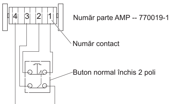
Schemă întrerupător UEPO cameră
