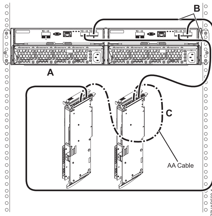
Figura 241. Conexiune mod 1 a unui sertar 5887 utilizând cabluri YO către adaptoare duble SAS
