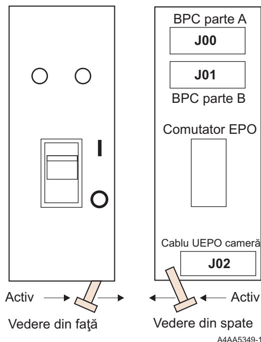
Figura 30. Oprerea de urgență a alimentării camerei calculatorului
