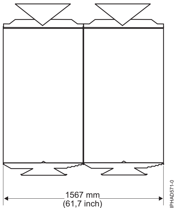
Figura 38. Vedere în plan pentru sisteme cu două cadre și uși acustice
