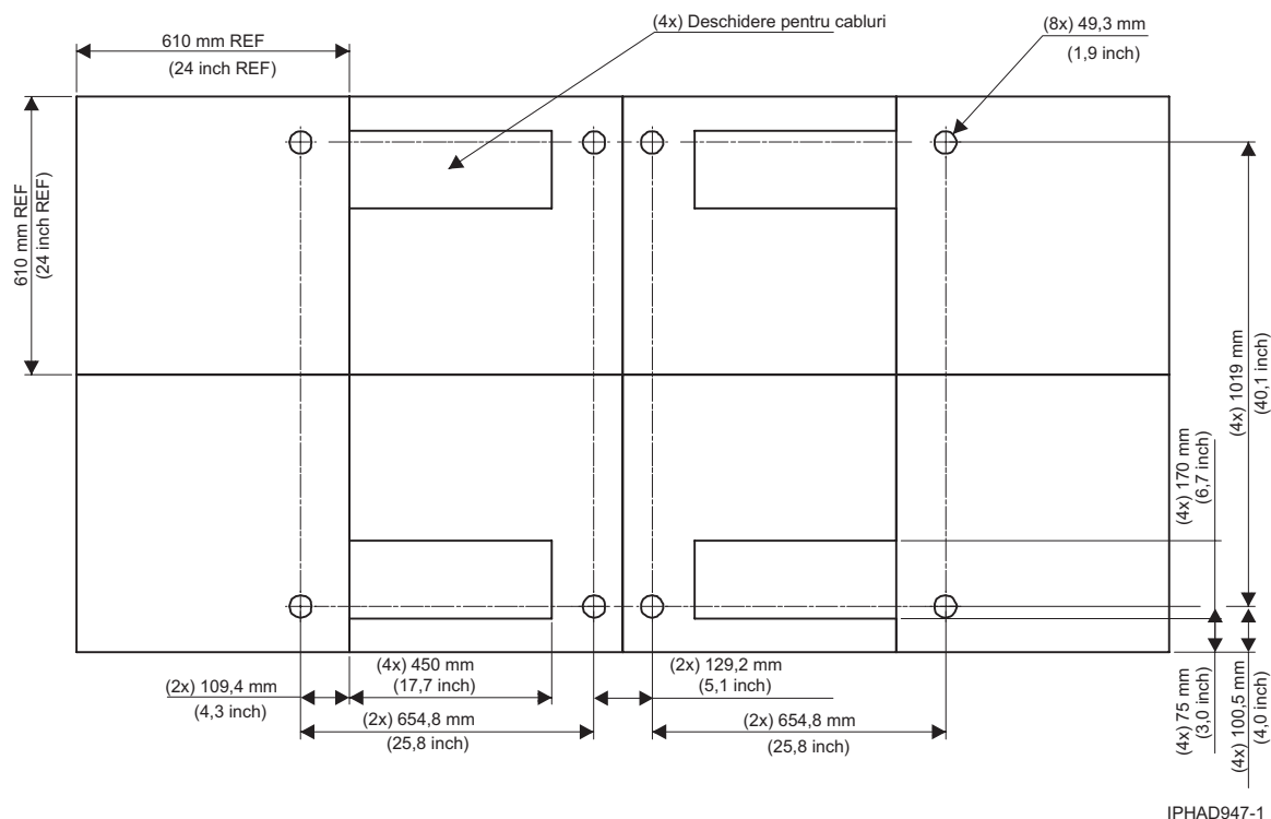
Figura 48. Poziționarea buloanelor cu ochi pentru podeaua cu plăci de 610 mm (24 inch)
