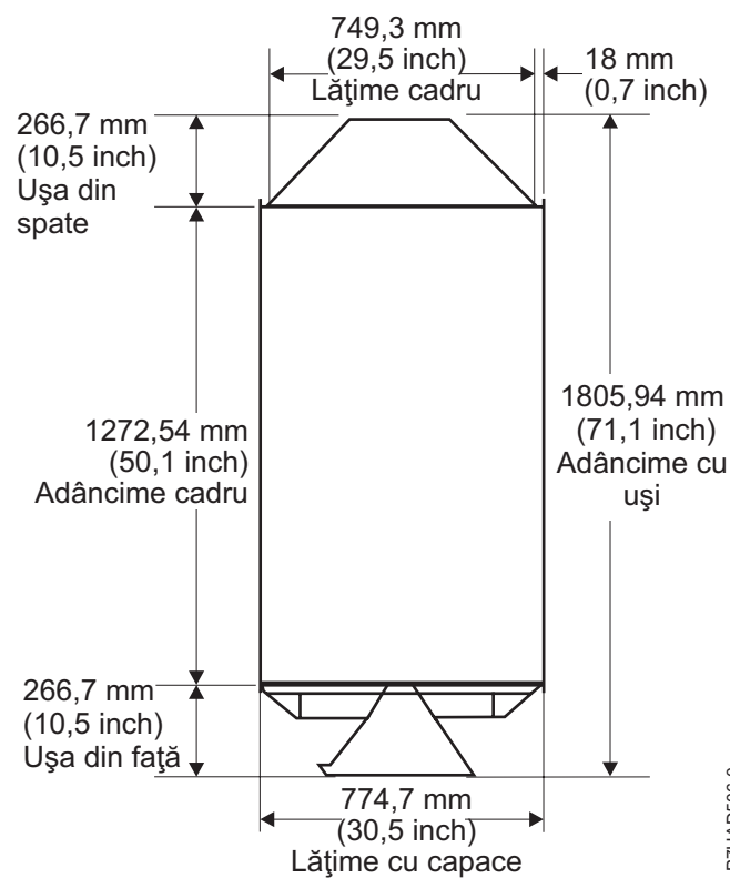
Figura 1. Vedere în plan pentru sisteme cu un cadru și uși acustice
