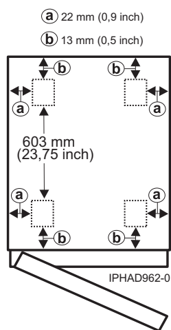
Figura 91. Locațiile roților pentru modelul 0554 și 7014-S11
