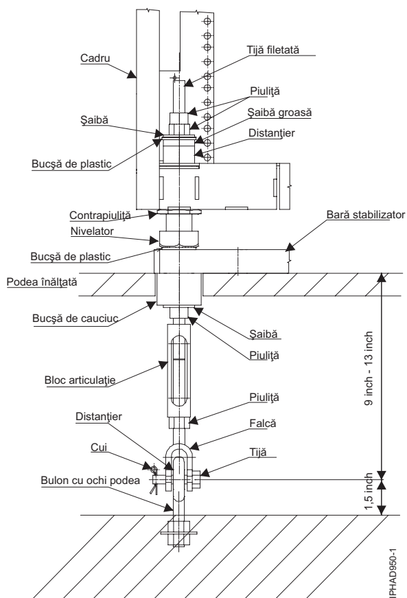
Figura 21. Accesorii de fixare a cadrului ansamblu întinzător cu filet pentru podea înălțată de 228,6 - 330,2 mm (9 - 13 inch) (număr parte componentă 44P2999)
