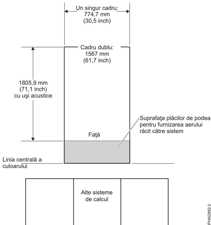
Figura 35. Cerințele zonei de circulație a aerului răcit
