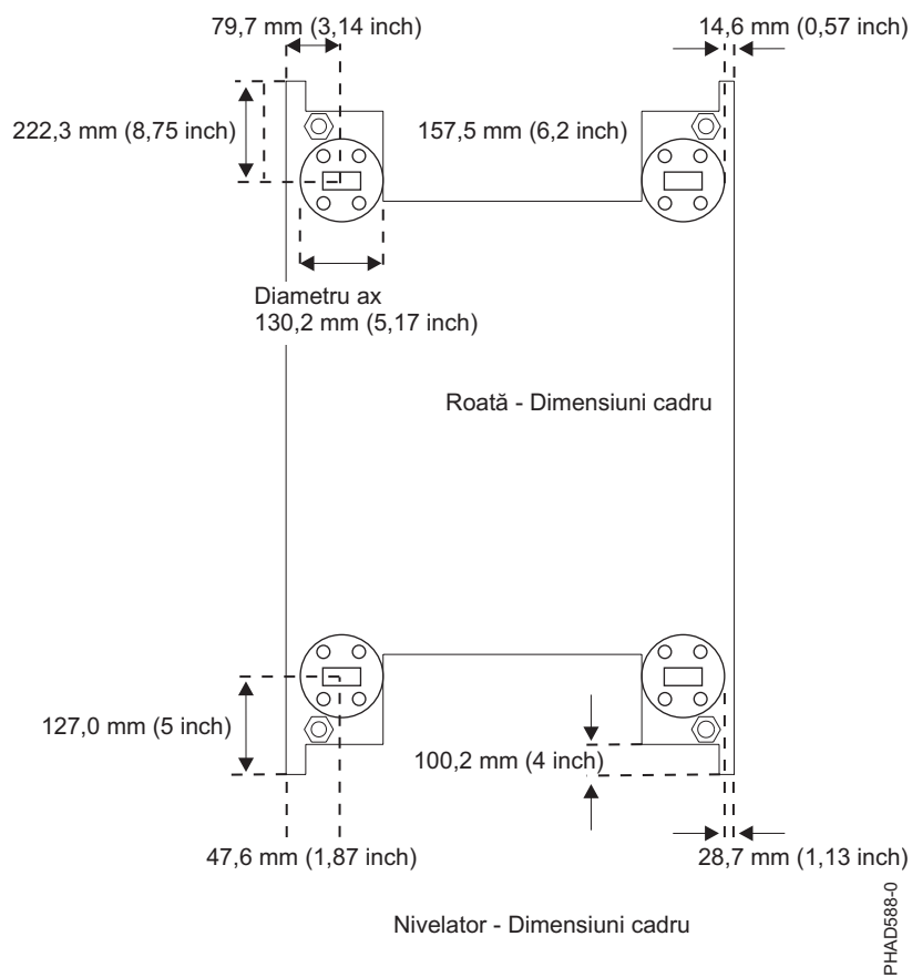
Figura 4. Suport de nivelare și dimensiunile cadrului
