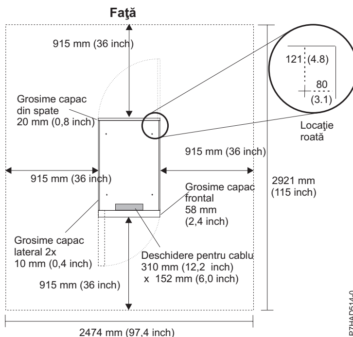
Figura 96. Spațiul de acces pentru service și locul roților pentru dulapurile 7014-T00, 7014-T42 și 0553
