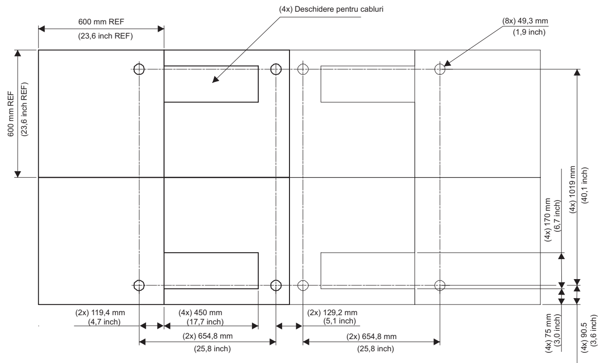
Figura 49. Poziționarea buloanelor cu ochi pentru podeaua cu plăci de 600 mm (23,6 inch)
