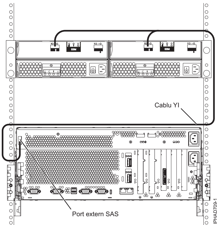
Figura 220. Port de adaptor SAS extern de sistem la un sertar de expansiune pentru discuri
