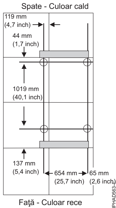
Figura 67. Modelul găurilor de fixare a dulapului
