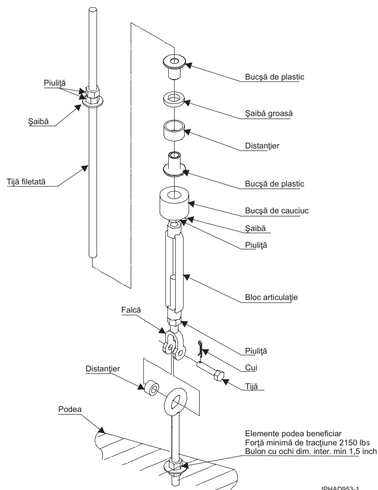
Figura 24. Accesorii de fixare a cadrului ansamblu întinzător cu filet pentru podea înălțată de 304,8 - 558,8 mm (12 - 22 inch) (număr parte componentă 44P3000)
