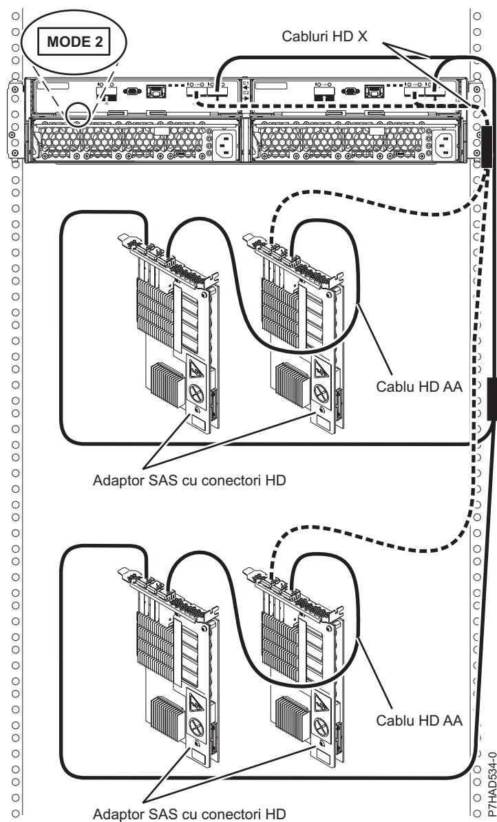
Figura 245. Conexiune de mod 2 a unui sertar 5887 utilizând conectori HD către două perechi de adaptoare SAS
