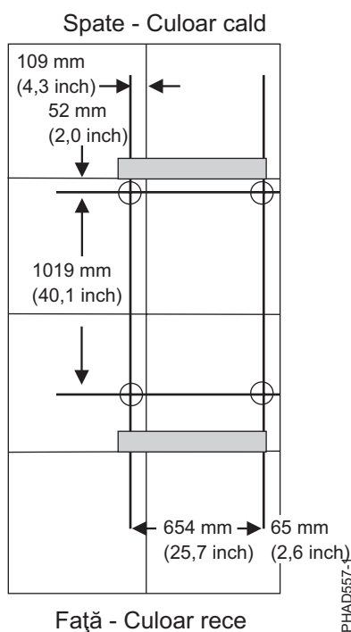
Figura 18. Model găuri de fixare pentru un singur dulap. Desen cu podeaua înălțată cu panouri de podea de 610 mm (24 inch)
