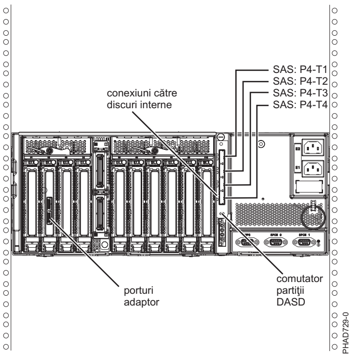
Figura 232. Două adaptoare SAS RAID la un sertar de expansiune pentru discuri într-o configurație JBOD HA inițializator multiplu
