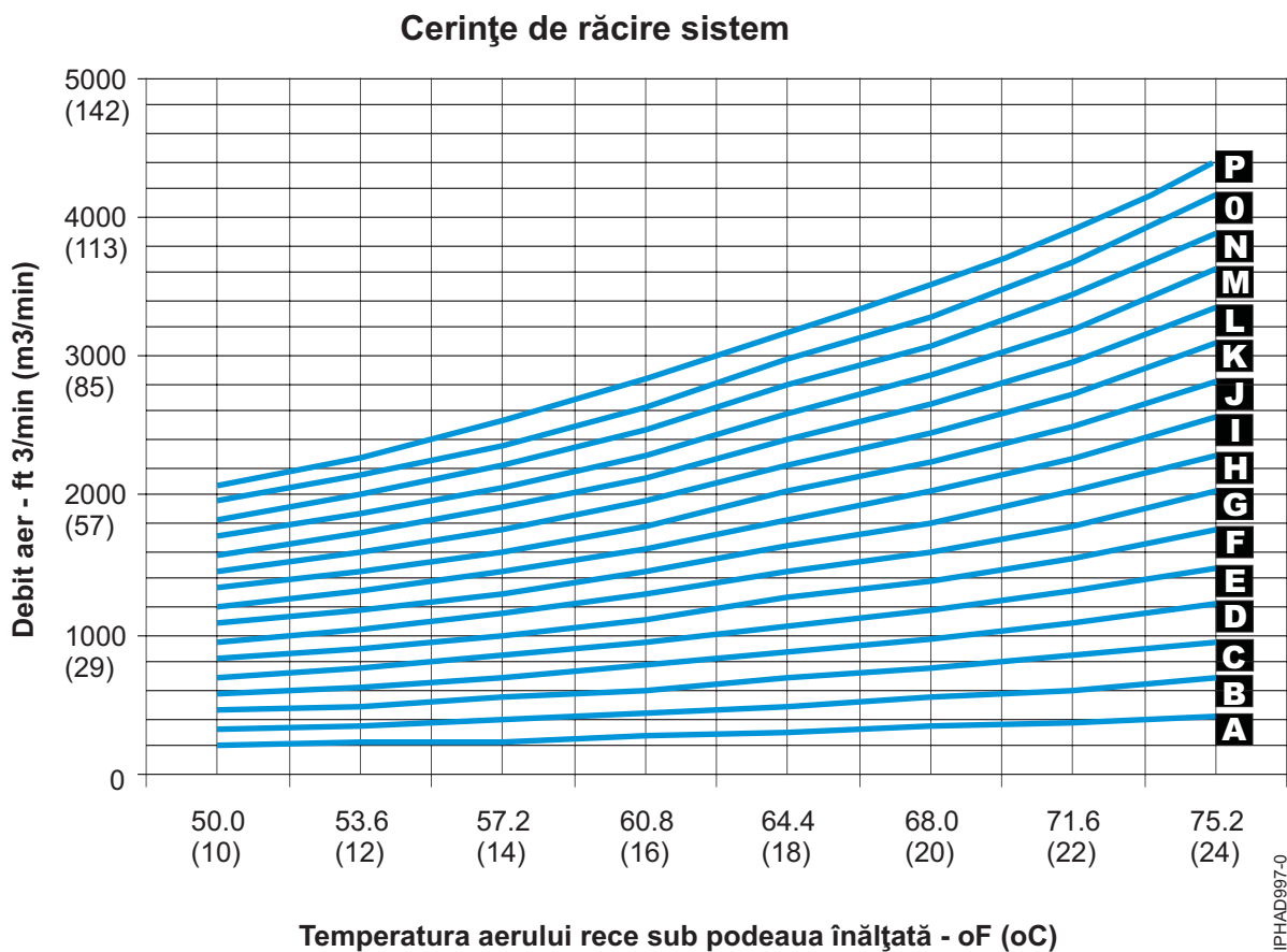
Figura 73. Cerințele de răcire
