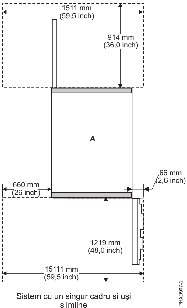
Figura 5. Spațiu de acces pentru service pentru un cadru de unitate de sistem sau un dulap I/E cu uși slimline
