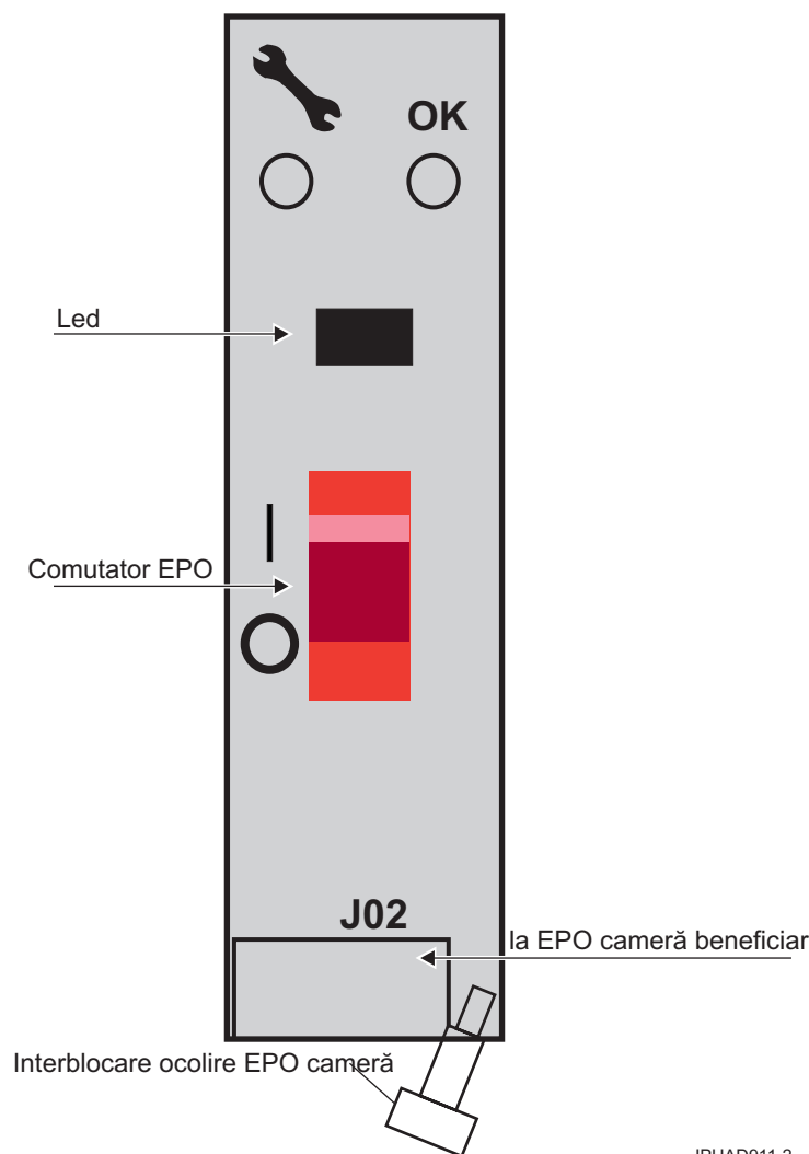
Figura 29. Oprirea de urgență a alimentării unității
