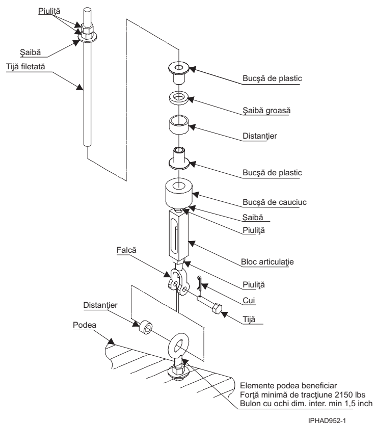
Figura 52. Accesorii de fixare a cadrului ansamblu întinzător cu filet pentru podea înălțată de 228,6 - 330,2 mm (9 - 13 inch) (număr parte componentă 44P2999)
