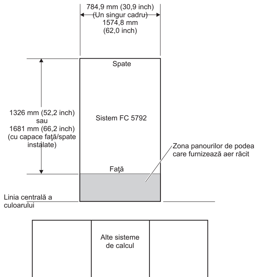
Figura 74. Zona fluxului de aer răcit
