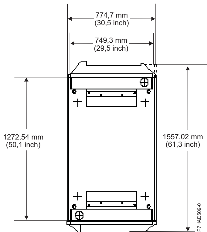
Figura 3. Vedere în plan pentru sisteme cu un cadru, uși slimline și schimbător de căldură pentru ușa din spate
