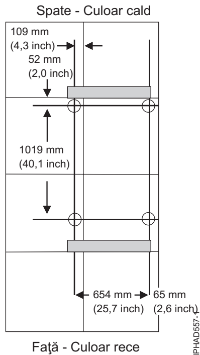
Figura 61. Modelul găurilor de fixare pentru un singur dulap
