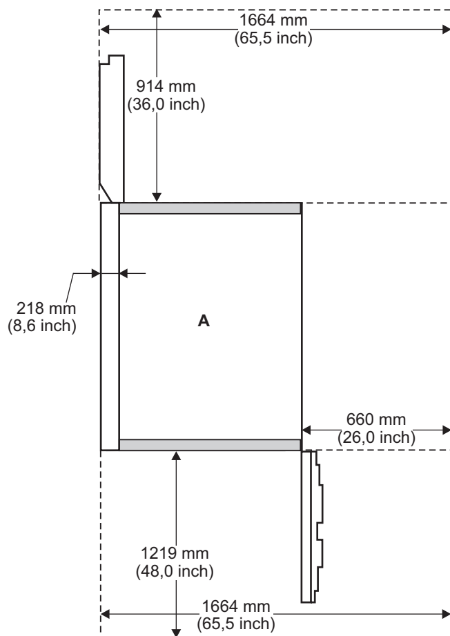
Sistem cu un singur cadru și uși acustice (cu spațiu alternativ de acces pentru service pe partea dreaptă)
