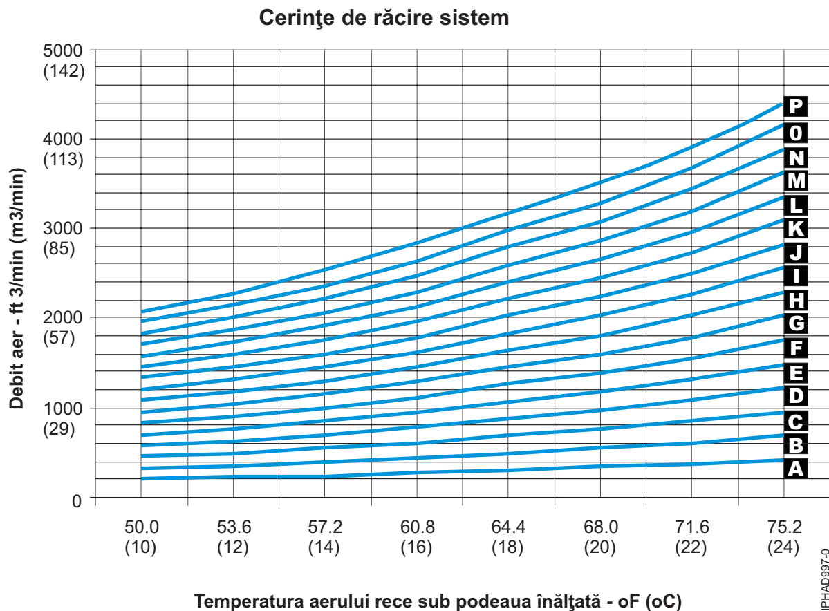
Figura 32. Cerințele de răcire
