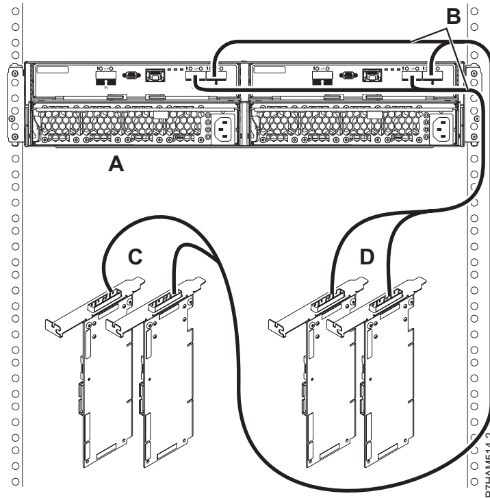
Figura 236. Conexiune mod 2 a unui sertar 5887 utilizând cabluri X către două perechi de adaptoare SAS
