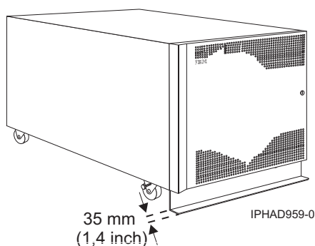
Figura 89. Model 0554 și 7014-S11 cu bară de stabilizator
