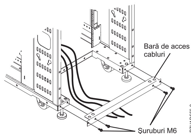
Figura 99. Bară de acces la cabluri
