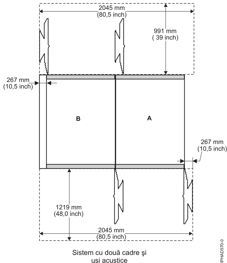
Figura 46. Spații de acces pentru sisteme cu cadru I/E dublu și uși acustice
