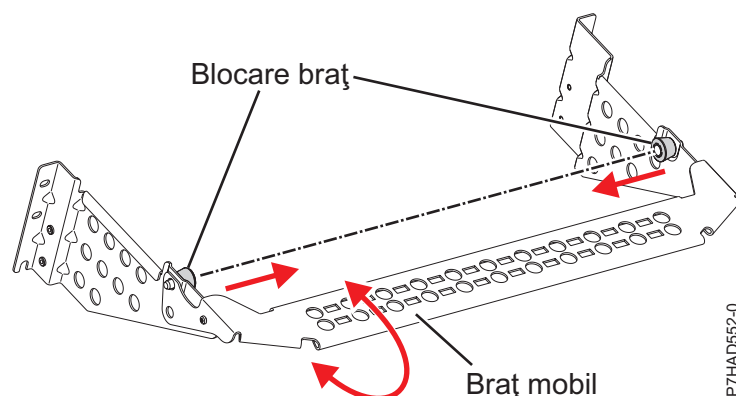
Figura 210. Colțar pentru pozarea cablurilor
