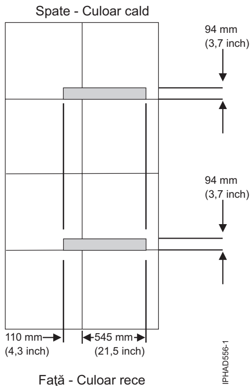
Figura 12. Amplasarea decupărilor pentru cabluri la plăci de 610 mm (24 inch)
