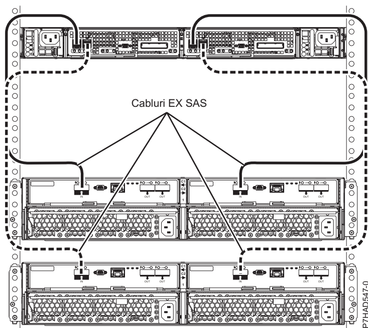
Figura 247. Conectarea a două sertare 5887 utilizând cabluri HD EX la un EDR1
