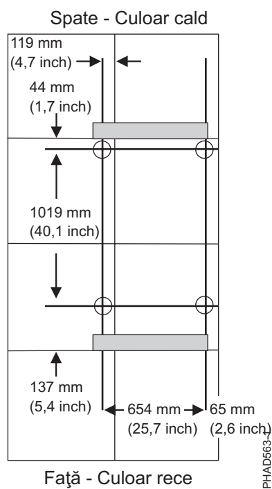
Figura 19. Modelul găurilor de fixare a dulapului. Podea înălțată cu plăci de 600 mm (23,6 inch)
