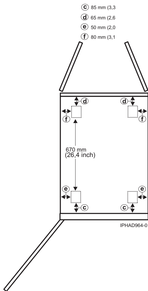
Figura 94. Locațiile roților pentru modelul 0555 și 7014-S25
