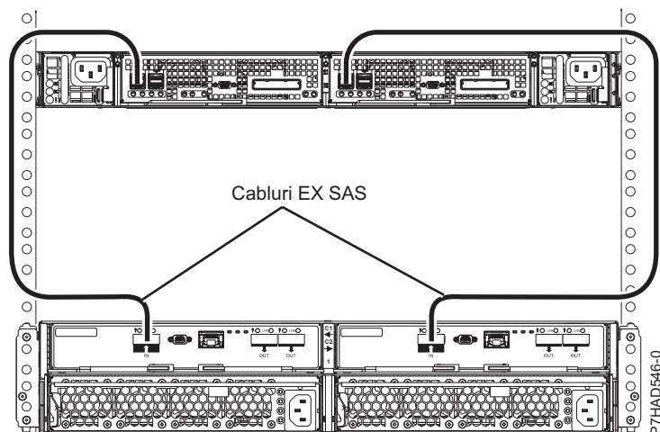
Figura 246. Conectarea unui sertar 5887 utilizând cabluri HD EX la un EDR1
