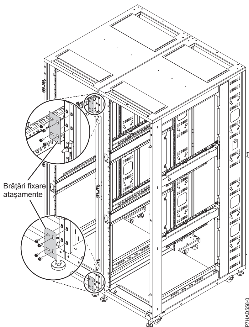
Figura 102. Colțare de atașare
