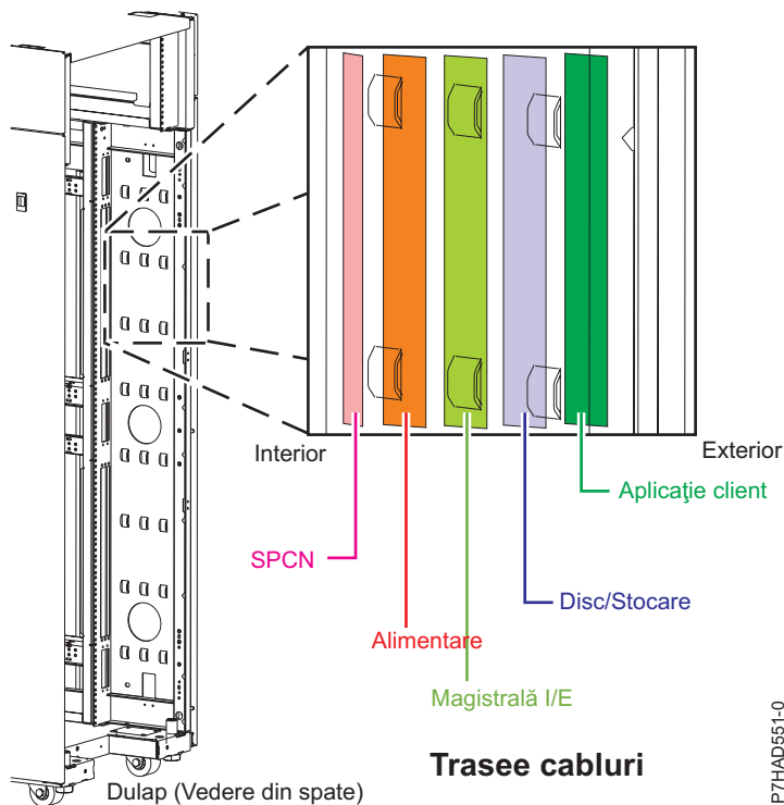
Figura 208. Clemele punții de pozare a cablurilor
