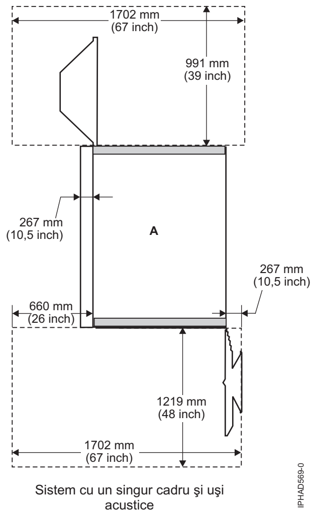
Figura 44. Spațiu de acces pentru service pentru un cadru de unitate de sistem sau un dulap I/E cu uși acustice
