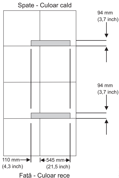
Figura 14. Amplasarea decupărilor pentru cabluri la plăci de 600 mm (23,6 inch)
