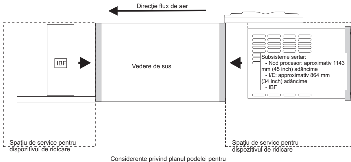
Figura 9. Considerente privind planul podelei pentru unitățile singulare
