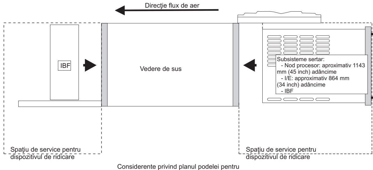
Figura 36. Considerente privind planul podelei pentru unitățile singulare
