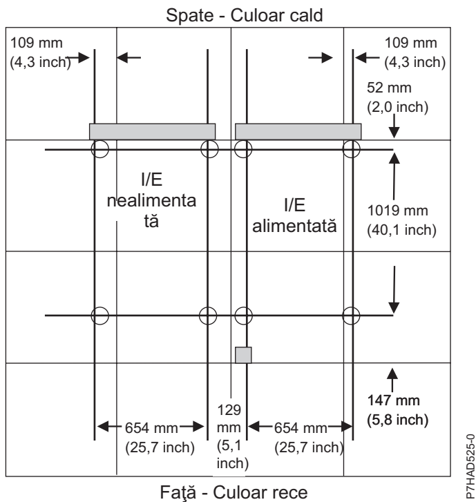
Figura 64. Amplasarea găurilor de fixare pentru două dulapuri
