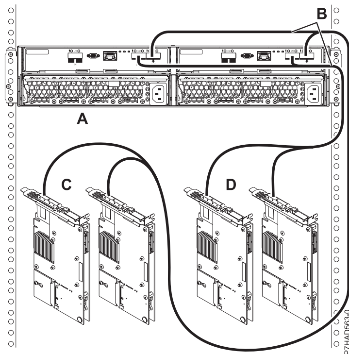
Figura 239. Două perechi de adaptoare FC 5805 sau FC 5903 la un sertar 5887 via o conexiune de mod 2.
