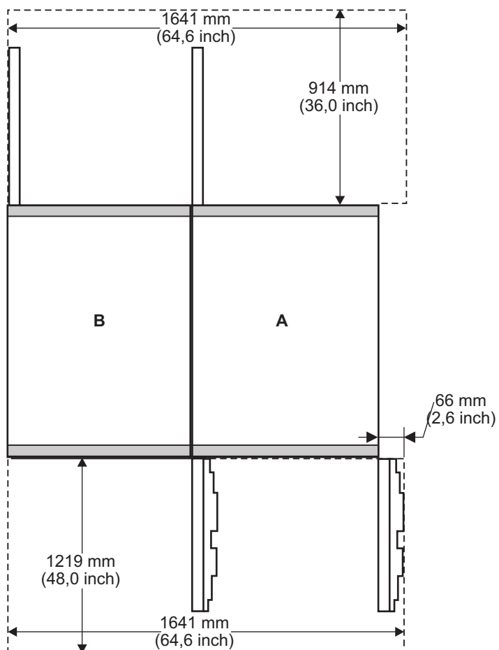
Sistem cu cadru dublu și uși slimline
