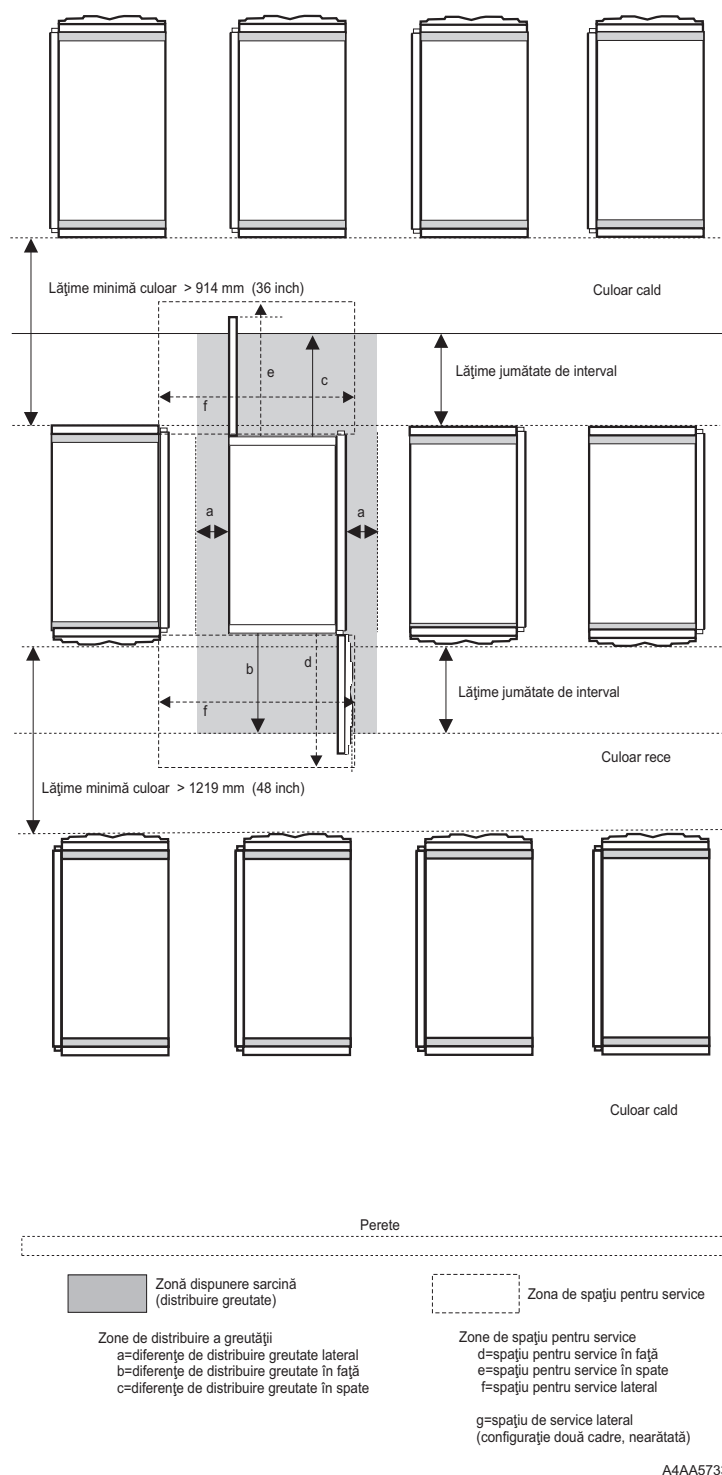
Figura 25. Dispunerea de podea recomandată pentru mai multe sisteme
