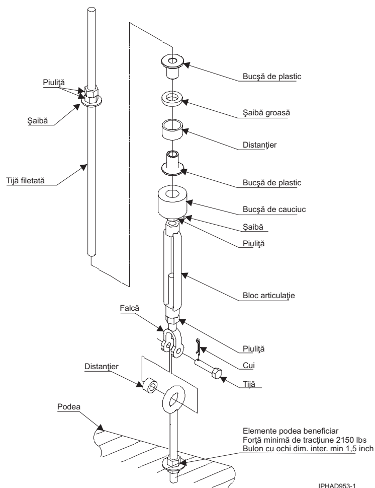
Figura 54. Accesorii de fixare a cadrului ansamblu întinzător cu filet pentru podea înălțată de 304,8 - 558,8 mm (12 - 22 inch) (număr parte componentă 44P3000)
