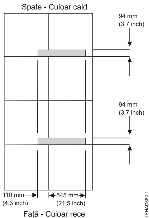
Figura 66. Amplasarea decupărilor pentru cabluri la plăci de 600 mm (23,6 inch)
