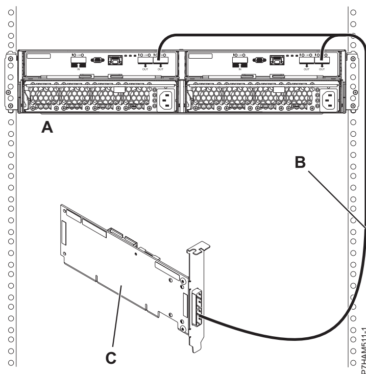
Figura 233. Conexiune mod 1 a sertarului 5887 utilizând un cablu YO către un adaptor singular SAS
