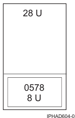
Figura 12. Cod caracteristică 0578 - unitate de expansiune PCI-X în dulap
