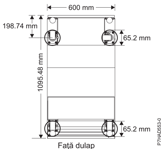
Figura 23. Locațiile roților
