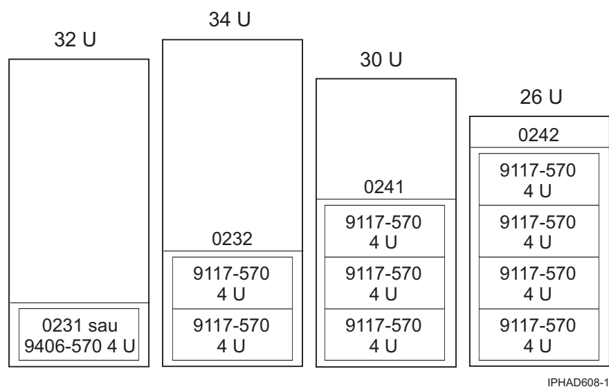
Figura 7. 570 în dulap
