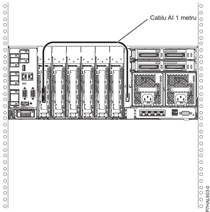
Figura 147. Adaptor SAS la sloturi de disc SAS intern prin portul SAS extern al sistemului
