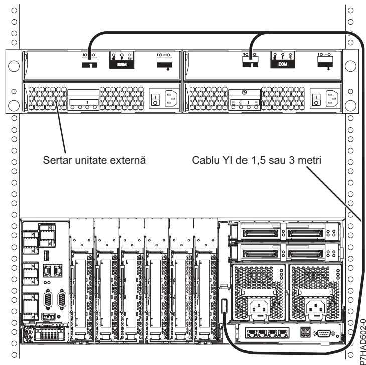
Figura 146. Port de adaptor SAS extern de sistem la un sertar de expansiune pentru discuri (modelele 9117-MMB și 9179-MHB)
