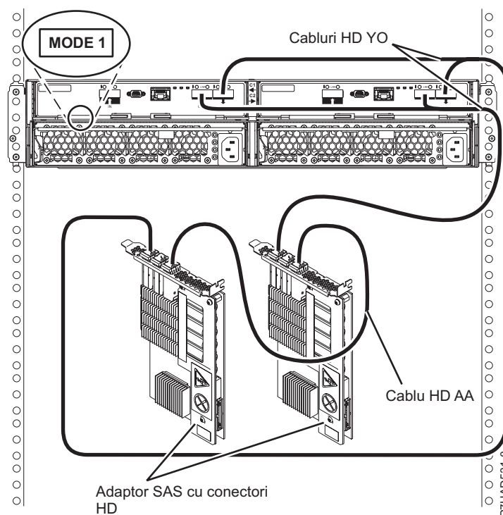
Figura 173. Conexiune de mod 1 a unui sertar 5887 la două adaptoare SAS cu conectori HD
