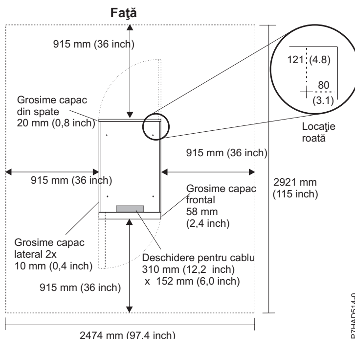
Figura 27. Spațiul de acces pentru service și locul roților pentru dulapurile 7014-T00, 7014-T42 și 0553
