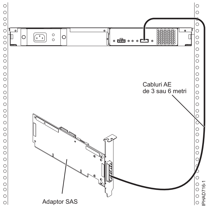
Figura 149. Adaptor SAS la un sertar de expansiune pentru medii
