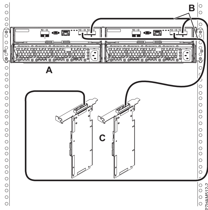
Figura 169. Conexiune mod 1 a unui sertar 5887 utilizând cabluri YO către adaptoare duble SAS
