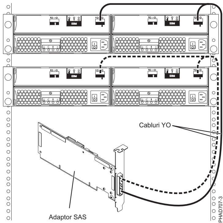
Figura 146. Adaptor SAS la două sertare de expansiune pentru discuri
