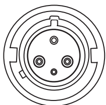
Figura 40. Tipul de priză IEC 60309 3P+N+E
