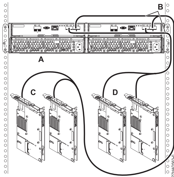
Figura 170. Două perechi de adaptoare FC 5805 sau FC 5903 la un sertar 5887 via o conexiune de mod 2.
