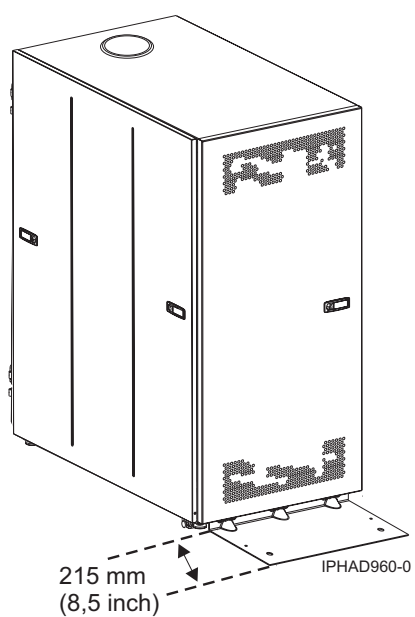
Figura 23. Model 0555 și 7014-S25 cu picior stabilizator
