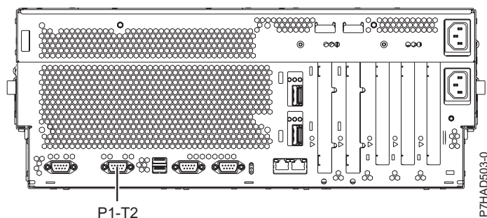
Figura 134. 8233-E8B și 8236-E8C - vedere din spate cu locația de instalare cabluri
