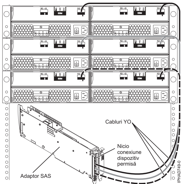
Figura 148. Adaptor SAS cu trei porturi la sertare de expansiune pentru discuri
