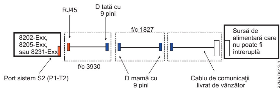
Figura 138. Cablarea sursei de alimentare neîntreruptibilă pentru 8202-E4B, 8202-E4C, 8205-E6B, 8205-E6C, 8231-E2B, 8231-E1C, 8231-E1D, 8231-E2C, 8231-E2D și 8268-E1D
