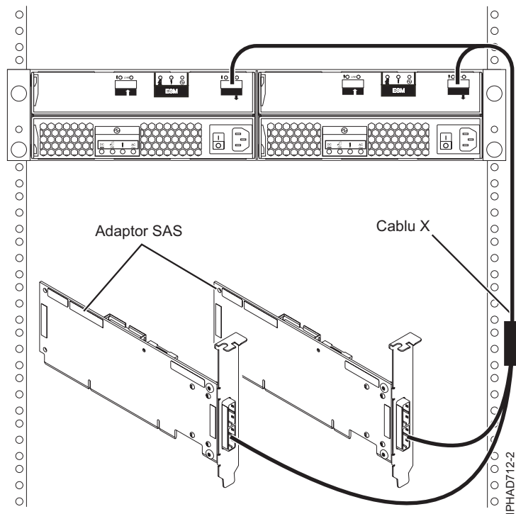
Figura 154. Două adaptoare RAID SAS la un sertar de expansiune pentru discuri într-o configurație RAID HA inițiator multiplu
