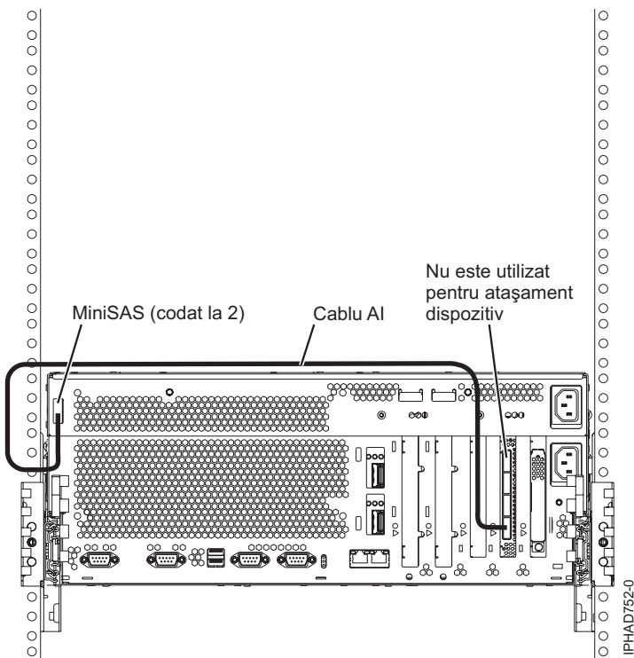
Figura 153. Adaptor FC5904 sau FC5908 atașat la sertare de expansiune pentru discuri
