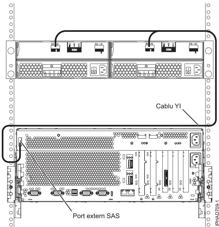
Figura 151. Port de adaptor SAS extern de sistem la un sertar de expansiune pentru discuri
