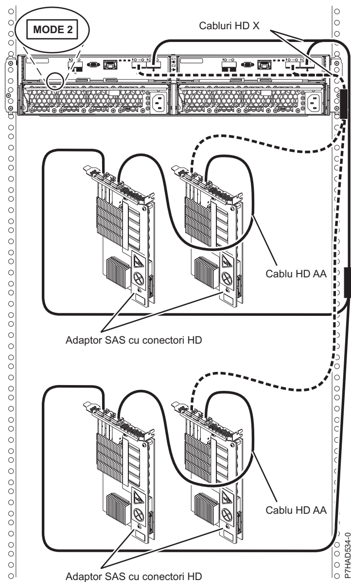
Figura 176. Conexiune de mod 2 a unui sertar 5887 utilizând conectori HD către două perechi de adaptoare SAS
