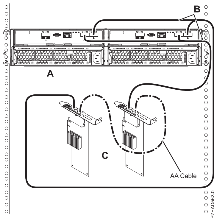
Figura 165. Conexiune mod 1 a unui sertar 5887 utilizând cabluri YO către adaptoare duble SAS
