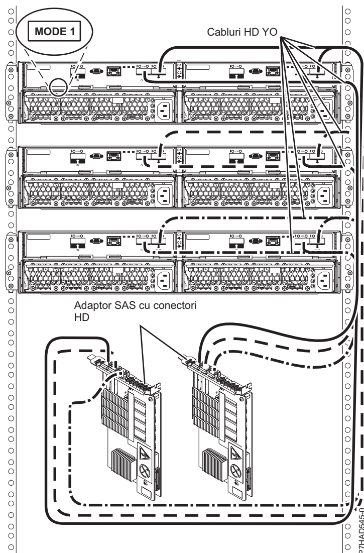
Figura 175. Conexiune de mod 1 a trei sertare 5887 la două adaptoare SAS cu conectori HD
