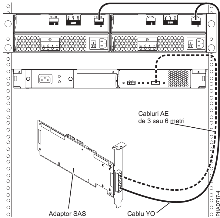
Figura 150. Adaptor SAS la un sertar de expansiune pentru discuri sau un sertar de expansiune pentru medii
