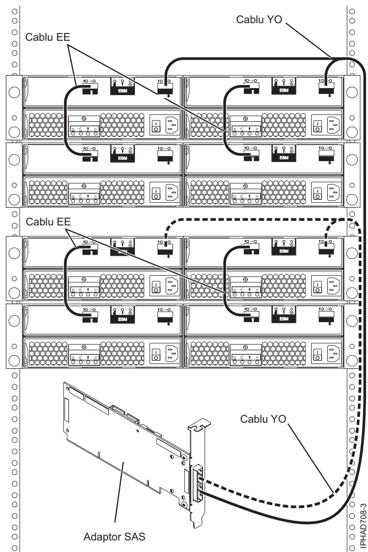
Figura 147. Adaptor SAS la patru sertare de expansiune pentru discuri
