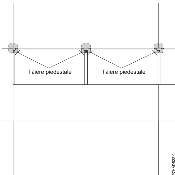
Figura 5. Tăiere pedestale
