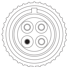
Figura 118. Tip de priză RS 7328DP
