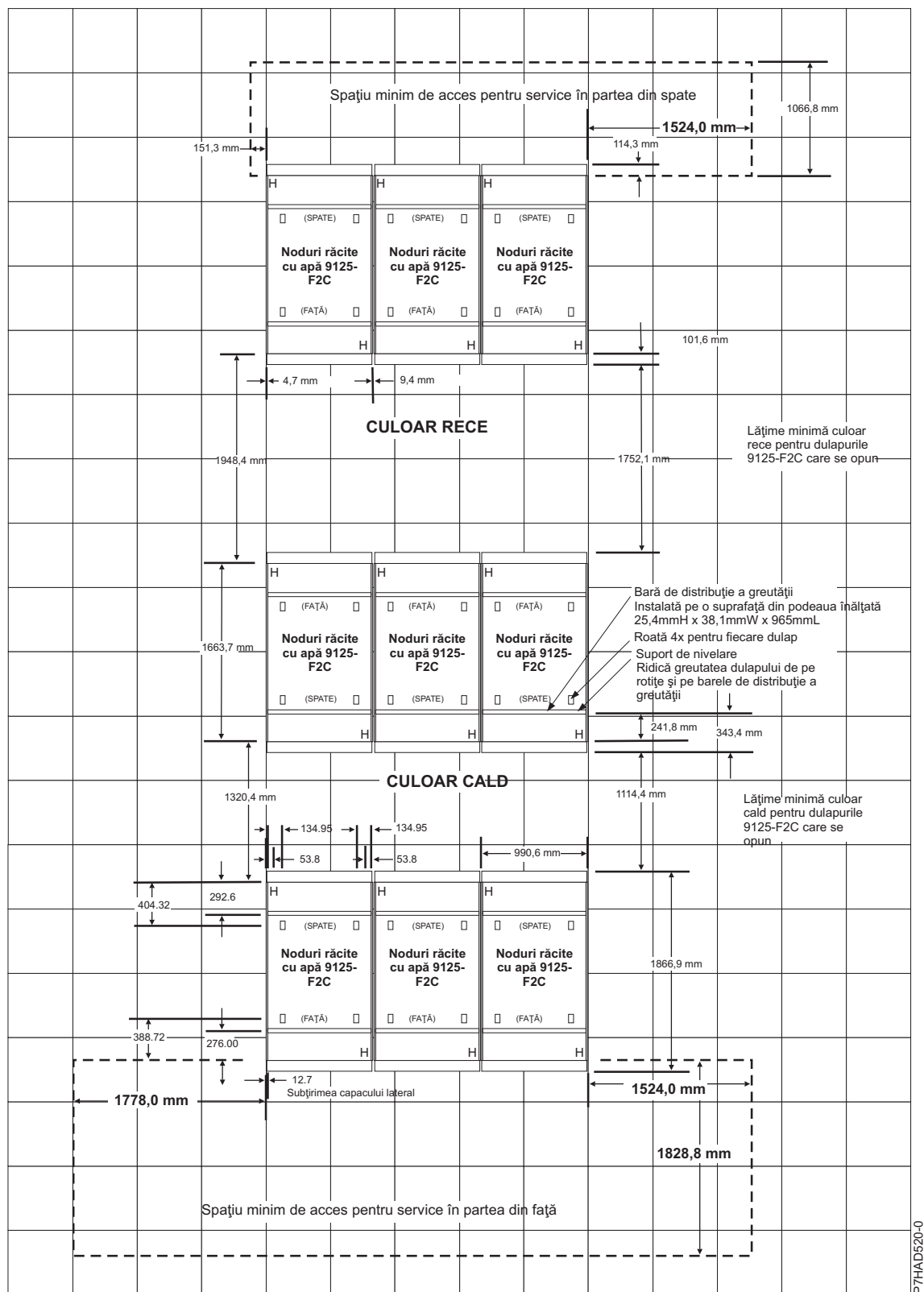
Figura 2. Spațiul de acces pentru service pentru dulapuri multiple - Culoar cald și culoar rece
