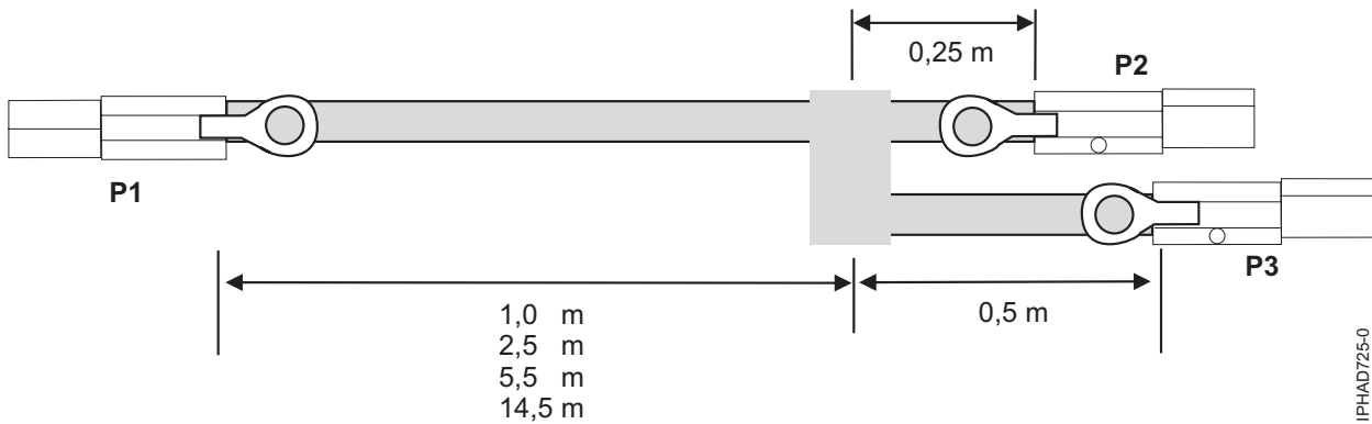
Figura 143. Lungimile de cablu pentru ansamblul cablu YO extern SAS
