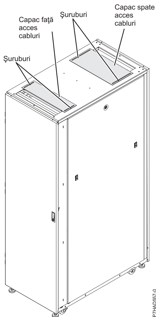
Figura 31. Capacele de acces la cabluri
