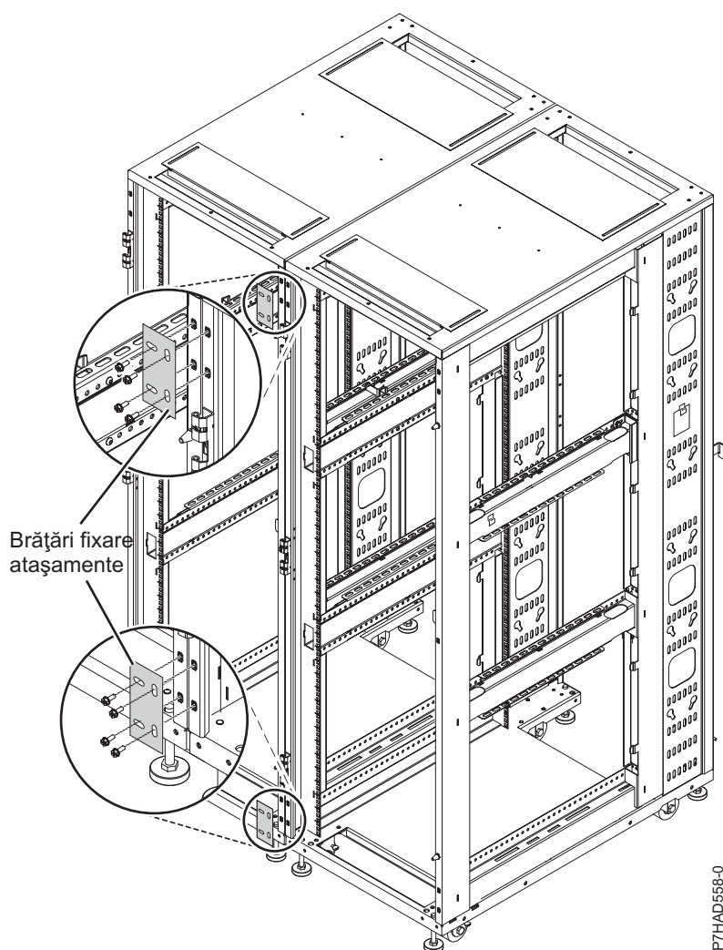
Figura 33. Colțare de atașare
