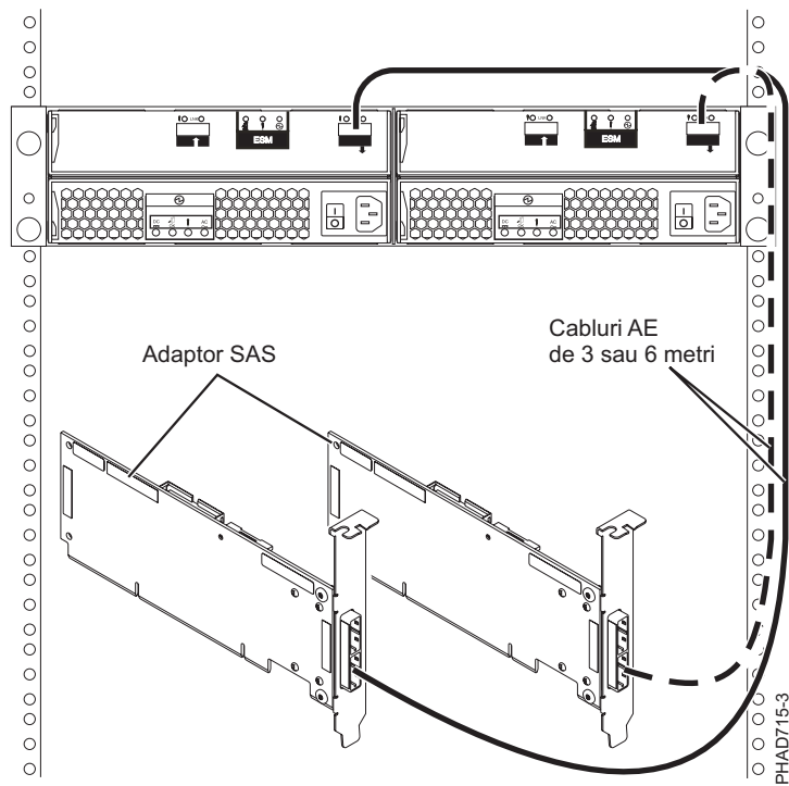
Figura 162. Două adaptoare SAS RAID la un sertar de expansiune pentru discuri într-o configurație JBOD HA inițializator multiplu
