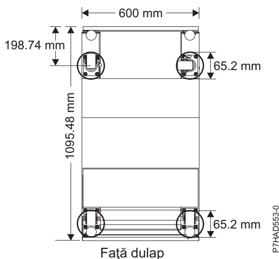
Figura 28. Locațiile roților
