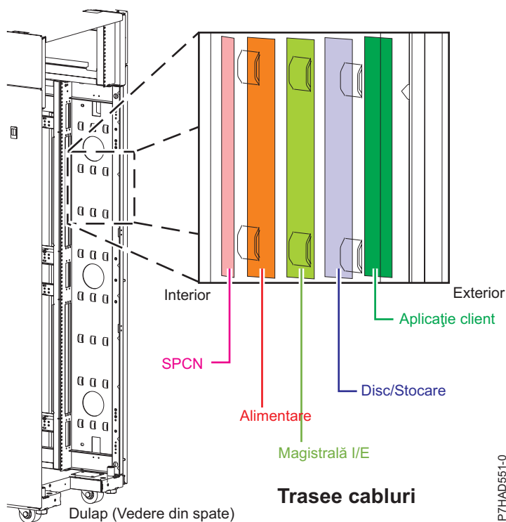
Figura 139. Clemele punții de pozare a cablurilor
