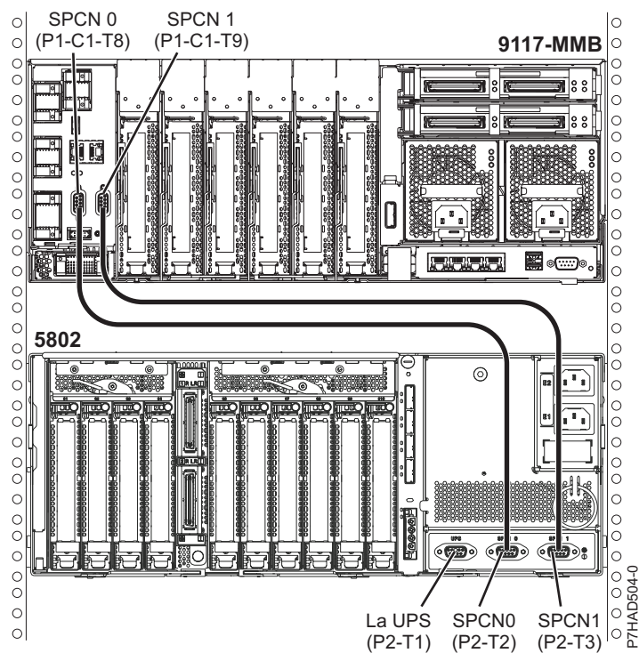
Figura 135. 8412-EAD, 9117-MMB, 9117-MMC, 9117-MMD, 9179-MHB, 9179-MHC, 9179-MHD și locația instalării cablurilor 5208 sau 5877 - vedere din spate
