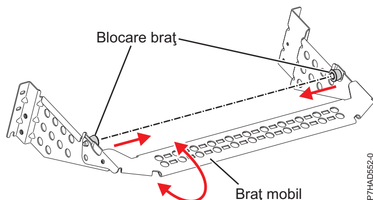
Figura 141. Colțar pentru pozarea cablurilor
