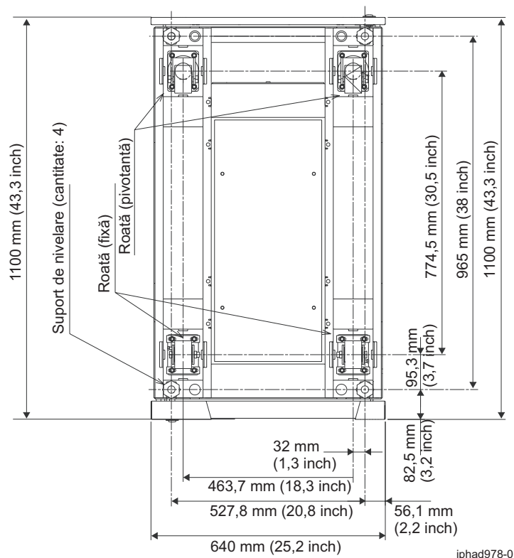
Figura 26. Locațiile roților și nivelatoarelor
