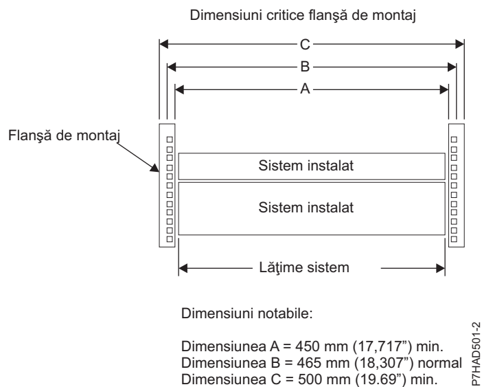
Figura 34. Dimensiuni de bordură de montare critice
