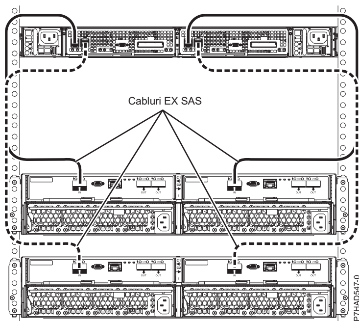
Figura 178. Conectarea a două sertare 5887 utilizând cabluri HD EX la un EDR1
