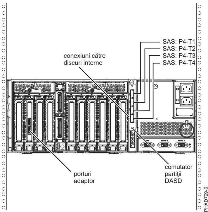
Figura 163. Două adaptoare SAS RAID la un sertar de expansiune pentru discuri într-o configurație JBOD HA inițializator multiplu
