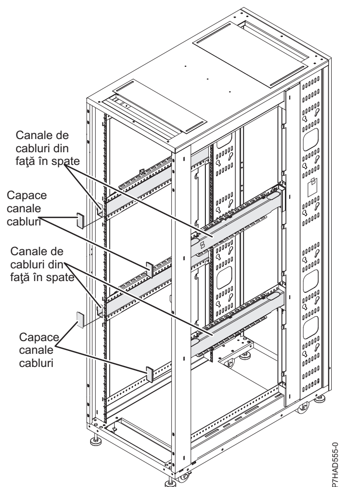
Figura 29. Cablarea în dulap
