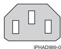
Figura 78. Tipul de priză 15
