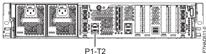
Figura 136. 8231-E2B, 8231-E1C, 8231-E1D, 8231-E2C, 8231-E2D și 8268-E1D - vedere din spate cu locația instalării cablurilor
