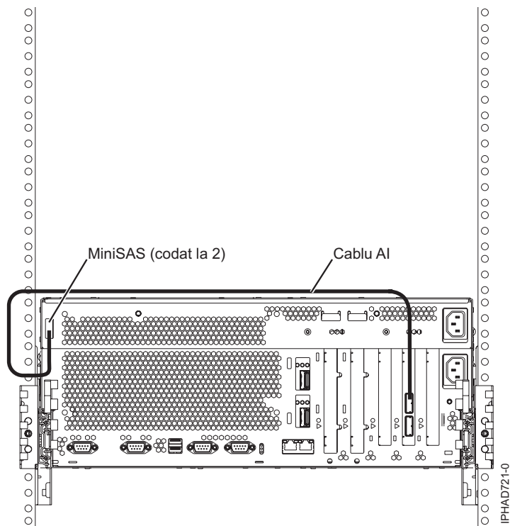
Figura 152. Adaptorul SAS la sloturi de disc SAS intern prin portul SAS extern al sistemului
