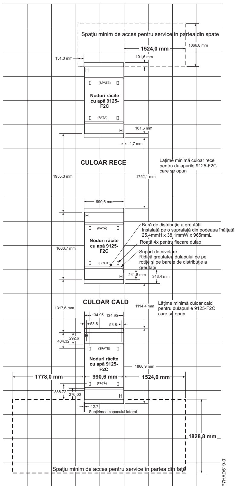
Figura 1. Spațiul de acces pentru service pentru un singur dulap - Culoar cald și culoar rece
