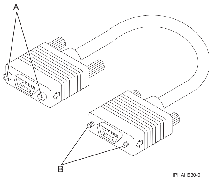
Figura 131. Conector de sursă de alimentare neîntreruptibilă pentru cablul de comunicații al sursei de alimentare neîntreruptibilă
