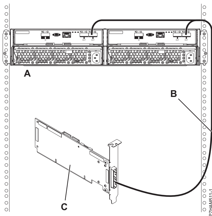
Figura 164. Conexiune mod 1 a sertarului 5887 utilizând un cablu YO către un adaptor singular SAS
