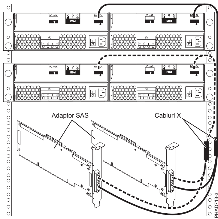
Figura 155. Două adaptoare RAID SAS la două sertare de expansiune pentru discuri într-o configurație RAID HA inițiator multiplu
