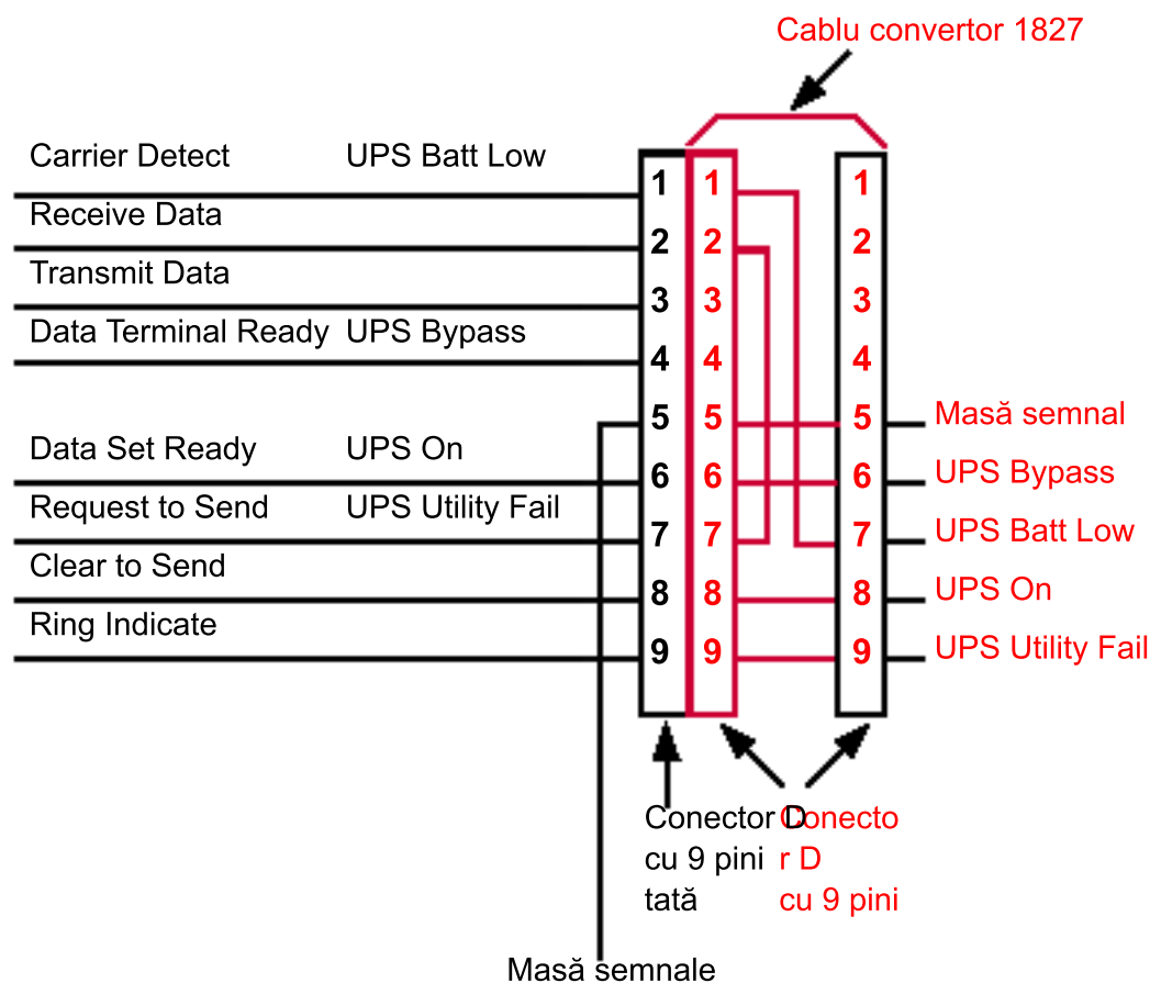
Figura 132. Conectarea cablului 1827
