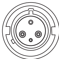
Figura 42. Tipul de priză 60309 P+N+E
