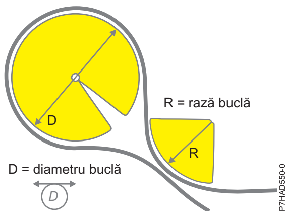
Figura 140. Raza de îndoire a cablului
