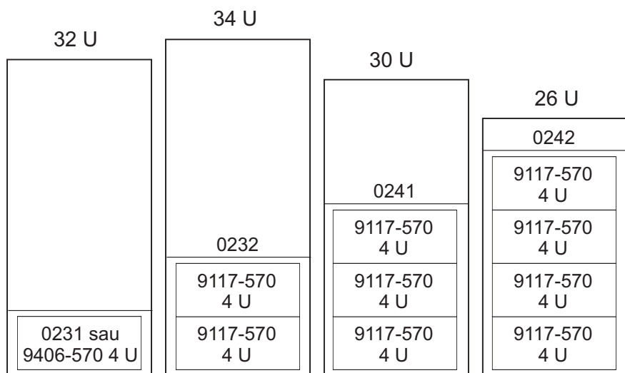
Figura 12. 570 în dulap
