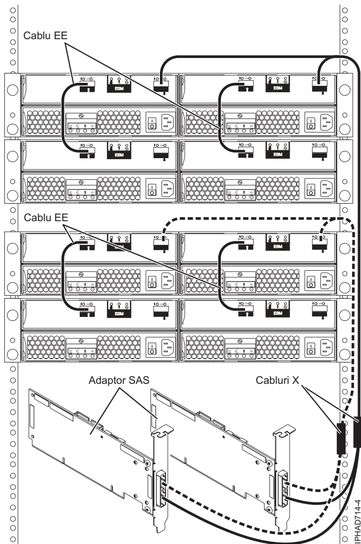
Figura 156. Două adaptoare RAID SAS la patru sertare de expansiune pentru discuri într-o configurație RAID HA inițiator multiplu
