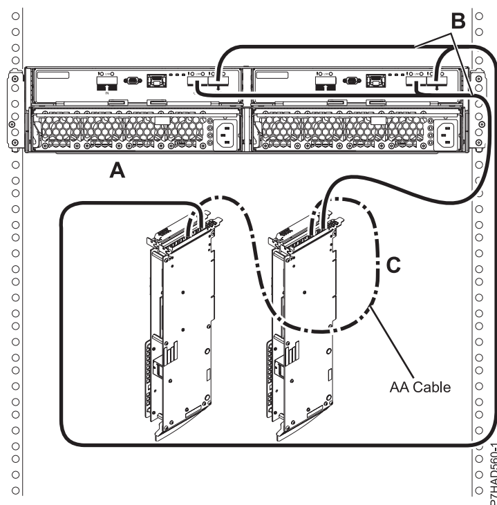
Figura 172. Conexiune mod 1 a unui sertar 5887 utilizând cabluri YO către adaptoare duble SAS
