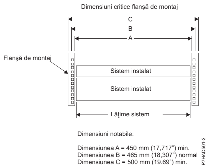
Figura 179. Dimensiuni de bordură de montare critice
