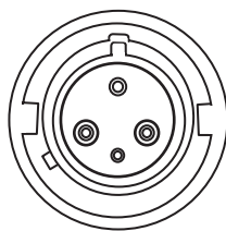
Figura 38. Tipul de priză IEC 60309 P+N+E
