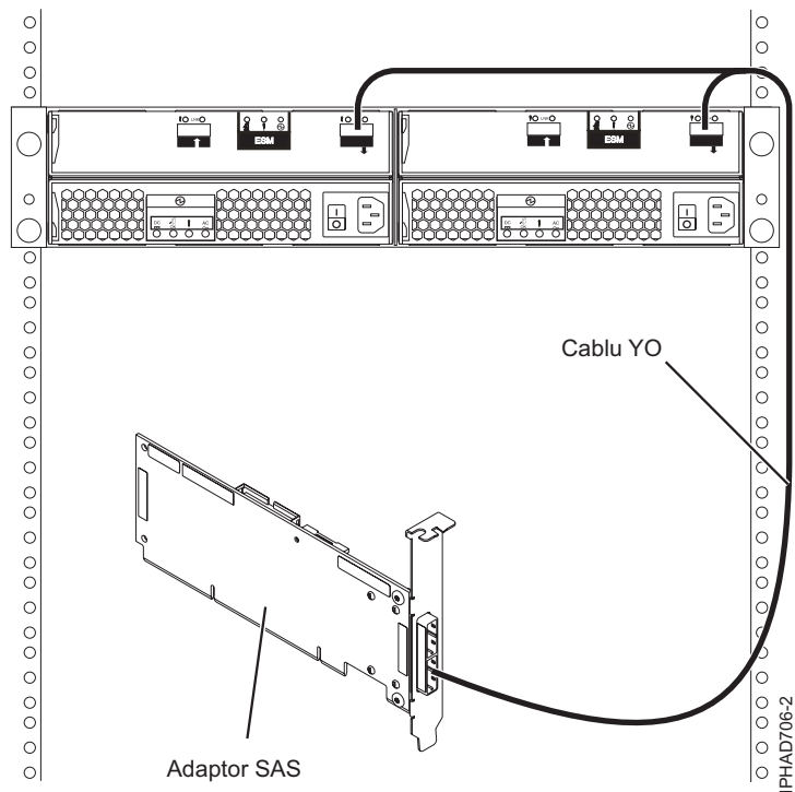
Figura 145. Adaptor SAS la un sertar de expansiune pentru discuri
