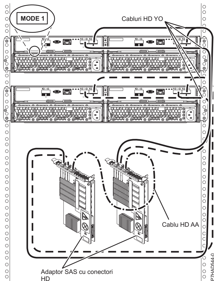
Figura 174. Conectarea de mod 1 a două sertare 5887 utilizând conectori HD la două adaptoare SAS
