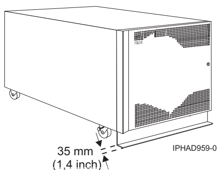
Figura 20. Model 0554 și 7014-S11 cu bară de stabilizator
