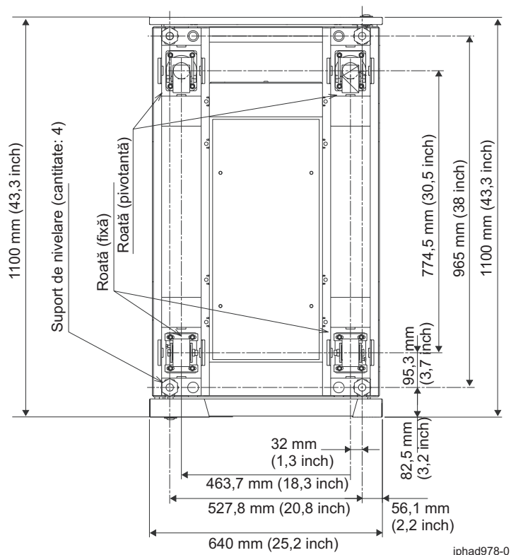
Figura 9. Locațiile roților și nivelatoarelor
