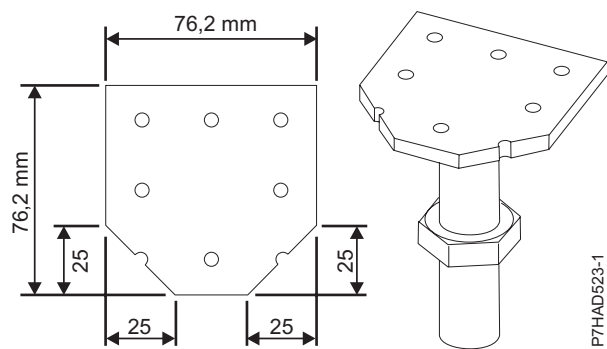
Figura 4. Tăiere dimensiuni pedestal
