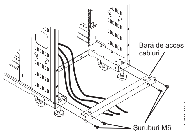
Figura 30. Bară de acces la cabluri
