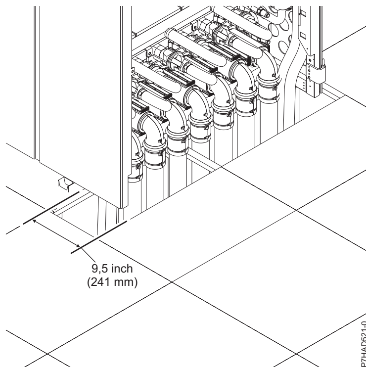
Figura 3. Decuparea în podea
