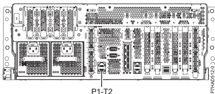
Figura 137. Vedere din spate cu locația instalării cablurilor pentru 8202-E4B, 8202-E4C, 8202-E4D, 8205-E6B, 8205-E6C și 8205-E6D
