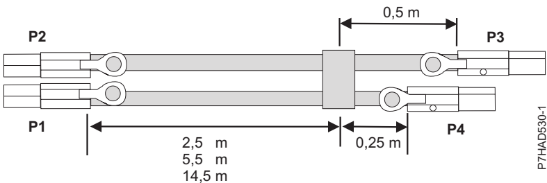
Figura 142. Lungimile de cablu pentru ansamblul cablu X extern SAS
