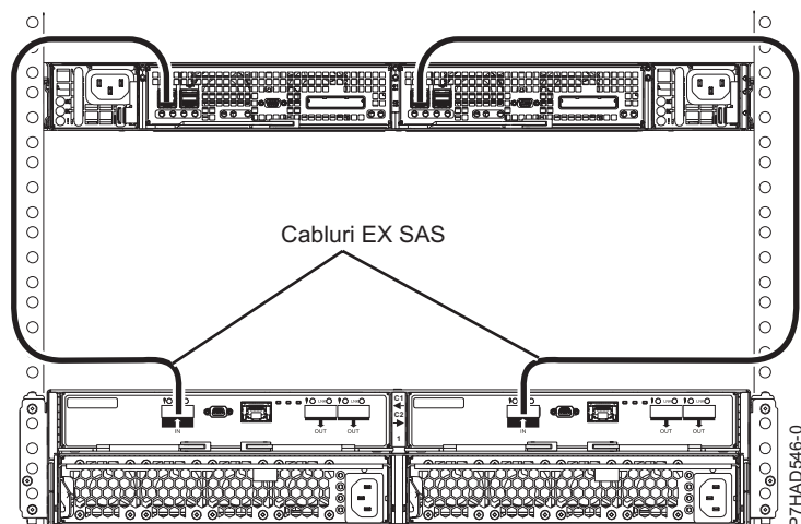
Figura 177. Conectarea unui sertar 5887 utilizând cabluri HD EX la un EDR1
