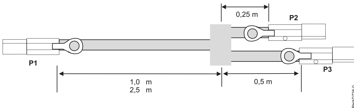
Figura 144. Lungimile de cablu pentru ansamblul cablu YI extern SAS
