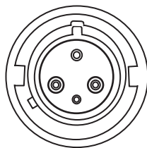
Figura 53. Tipul de priză IEC 60309 2P+E
