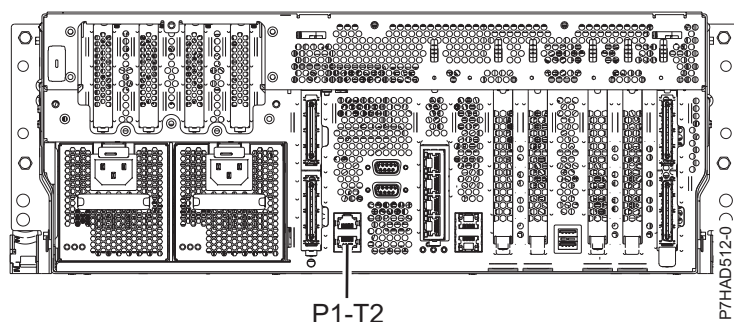
Figura 132. Vedere din spate cu locația instalării cablurilor pentru 8202-E4B, 8202-E4C, 8202-E4D, 8205-E6B, 8205-E6C și 8205-E6D
