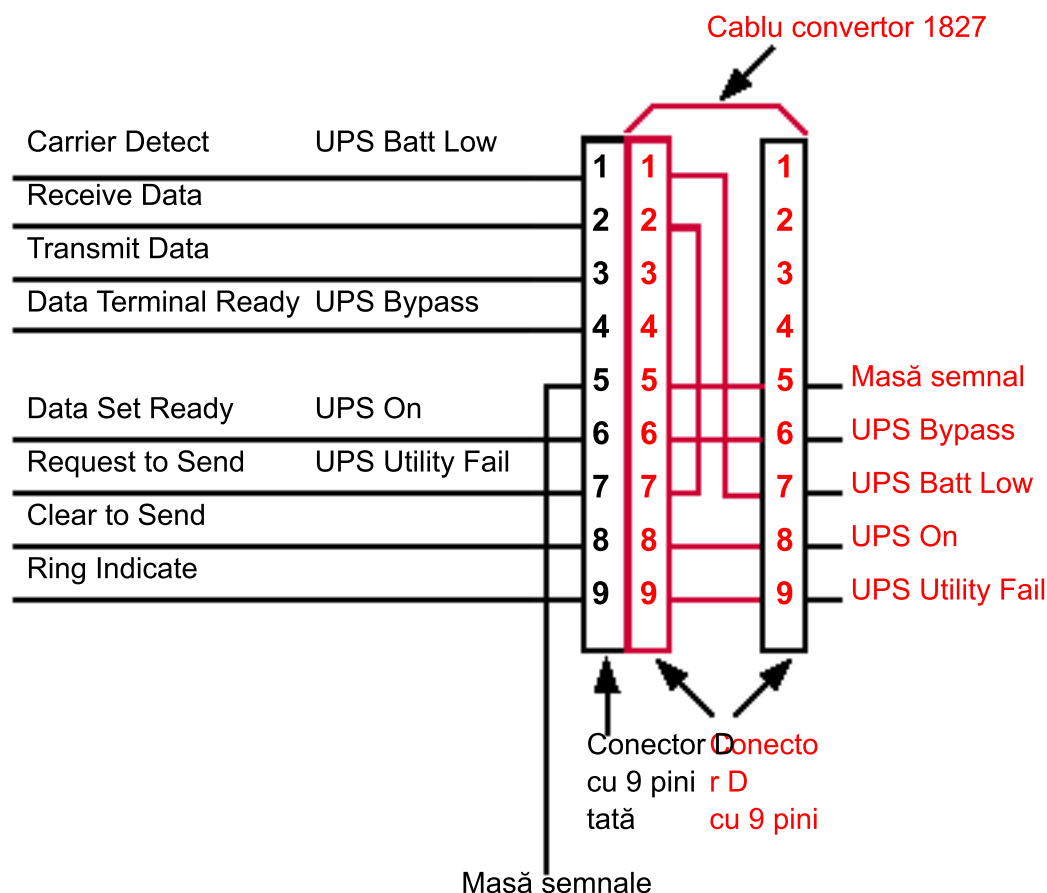
Figura 127. Conectarea cablului 1827
