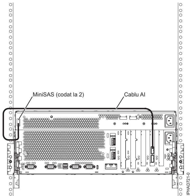
Figura 148. Adaptorul SAS la sloturi de disc SAS intern prin portul SAS extern al sistemului
