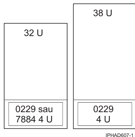
Figura 6. Cod caracteristică 7884: 9406-520 și 9111-520 într-un dulap
