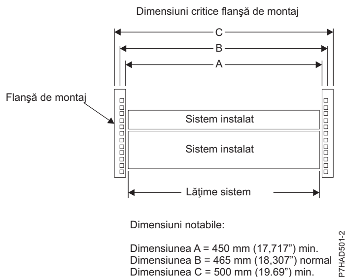
Figura 175. Dimensiuni de bordură de montare critice
