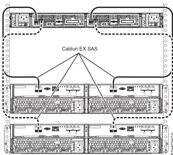
Figura 174. Conectarea a două sertare 5887 utilizând cabluri HD EX la un EDR1
