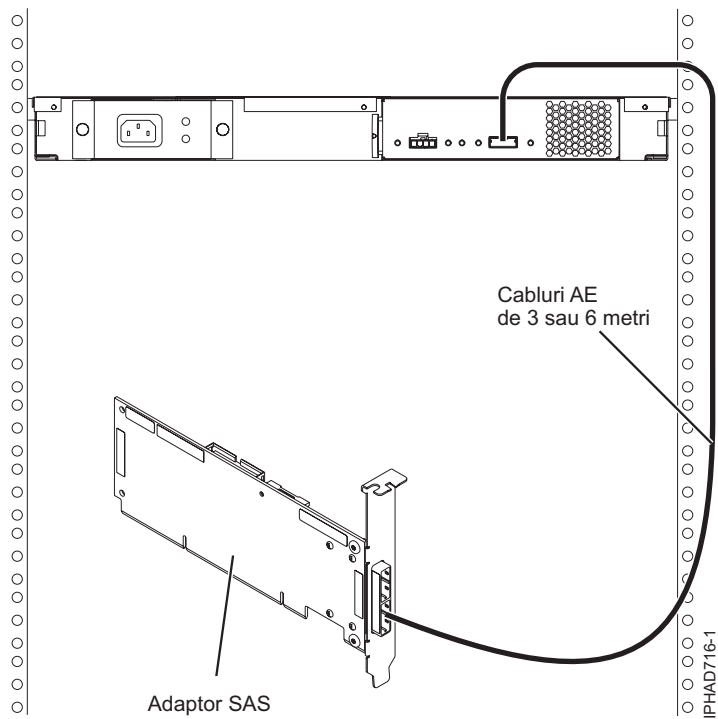
Figura 145. Adaptor SAS la un sertar de expansiune pentru medii
