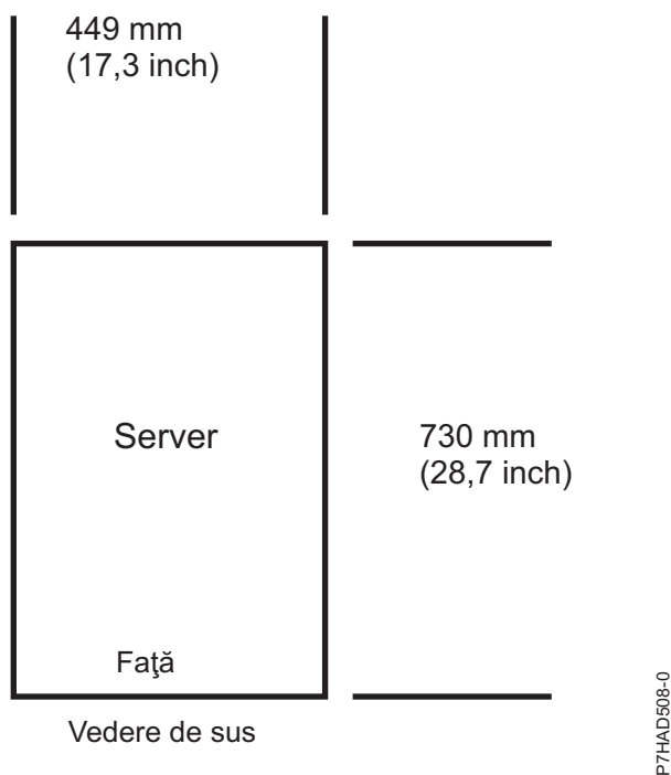
Figura 1. Vedere în plan pentru modelul 8202-E4B, 8202-E4C, 8202-E4D, 8205-E6B, 8205-E6C și 8205-E6D (servere montate în dulap)
