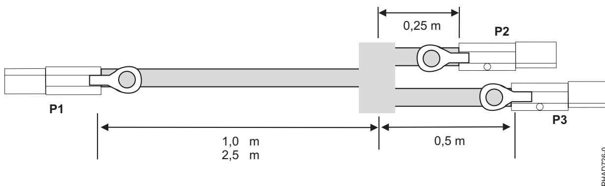
Figura 140. Lungimile de cablu pentru ansamblul cablu YI extern SAS
