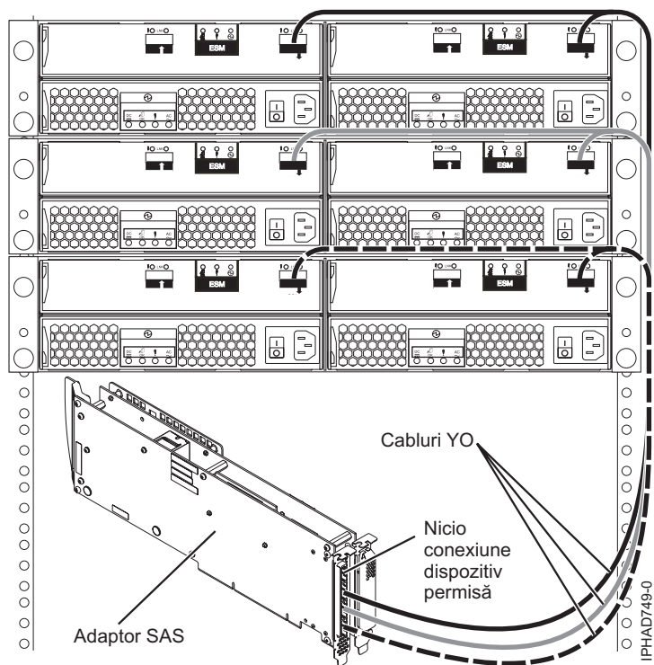
Figura 144. Adaptor SAS cu trei porturi la sertare de expansiune pentru discuri
