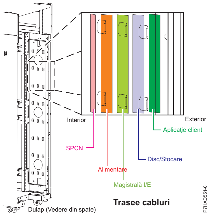
Figura 135. Clemele punții de pozare a cablurilor
