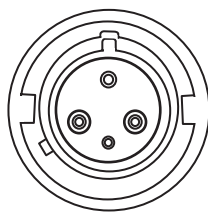
Figura 34. Tipul de priză IEC 60309 P+N+E
