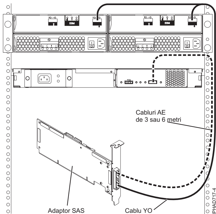
Figura 146. Adaptor SAS la un sertar de expansiune pentru discuri sau un sertar de expansiune pentru medii
