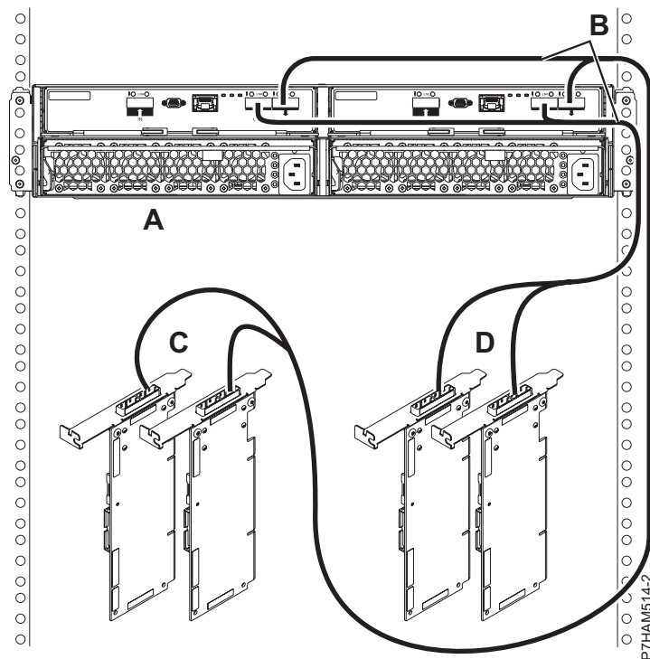
Figura 163. Conexiune mod 2 a unui sertar 5887 utilizând cabluri X către două perechi de adaptoare SAS
