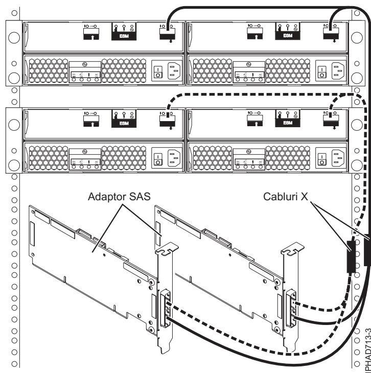
Figura 151. Două adaptoare RAID SAS la două sertare de expansiune pentru discuri într-o configurație RAID HA inițiator multiplu
