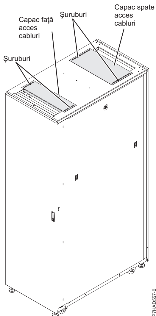
Figura 27. Capacele de acces la cabluri
