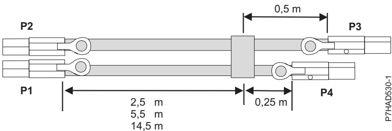
Figura 138. Lungimile de cablu pentru ansamblul cablu X extern SAS
