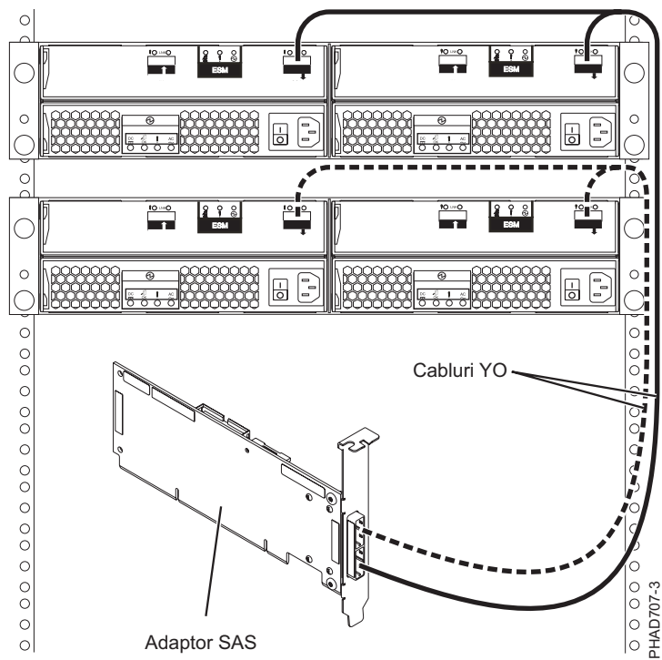
Figura 142. Adaptor SAS la două sertare de expansiune pentru discuri
