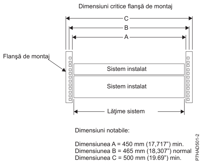
Figura 30. Dimensiuni de bordură de montare critice
