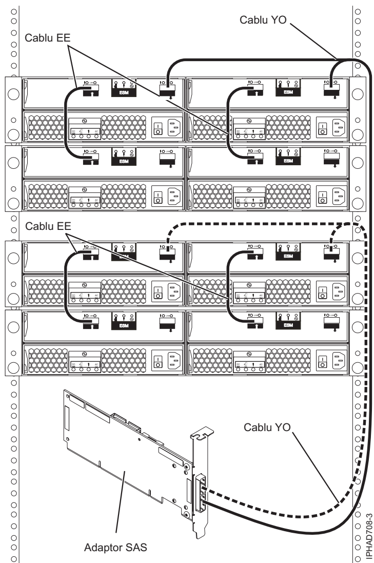
Figura 143. Adaptor SAS la patru sertare de expansiune pentru discuri
