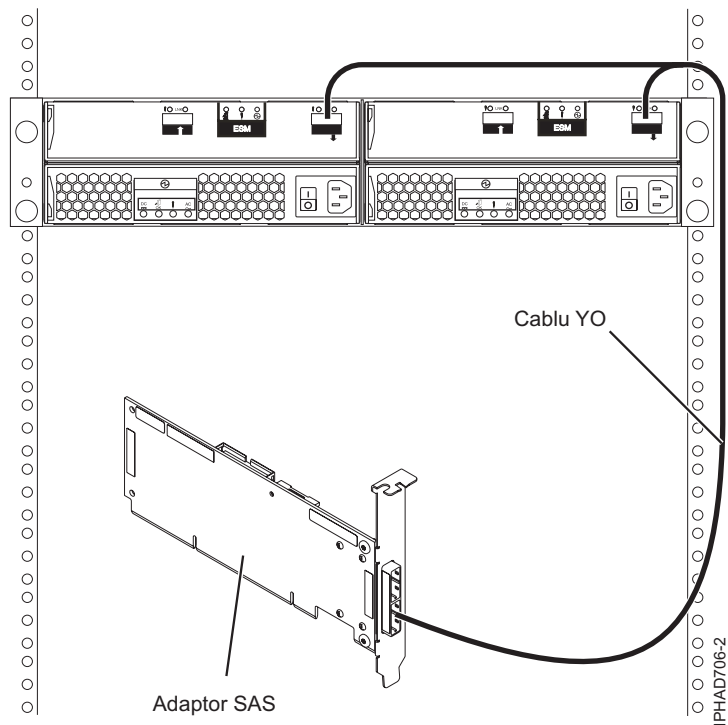
Figura 141. Adaptor SAS la un sertar de expansiune pentru discuri
