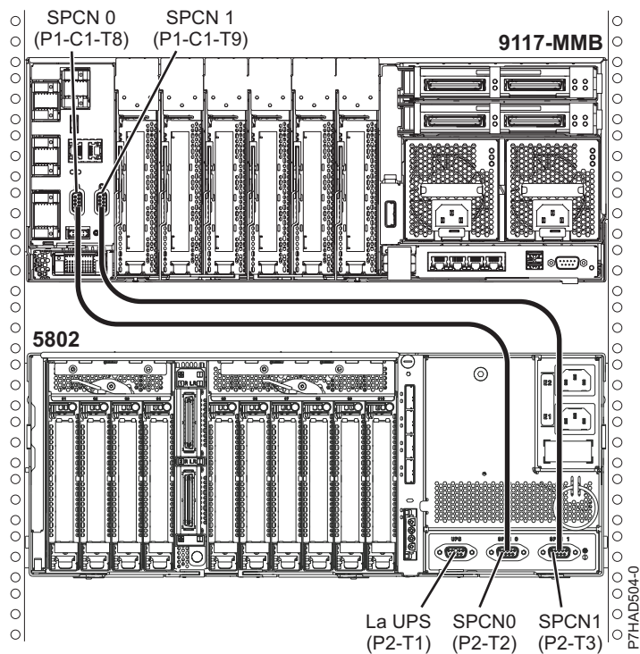
Figura 131. 8412-EAD, 9117-MMB, 9117-MMC, 9117-MMD, 9179-MHB, 9179-MHC, 9179-MHD și locația instalării cablurilor 5208 sau 5877 - vedere din spate
