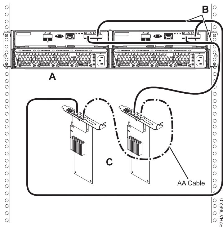
Figura 161. Conexiune mod 1 a unui sertar 5887 utilizând cabluri YO către adaptoare duble SAS
