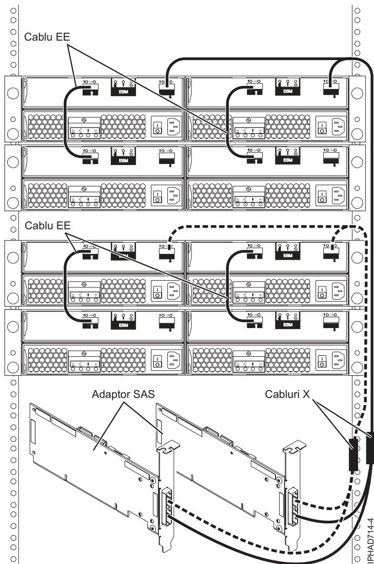
Figura 152. Două adaptoare RAID SAS la patru sertare de expansiune pentru discuri într-o configurație RAID HA inițiator multiplu
