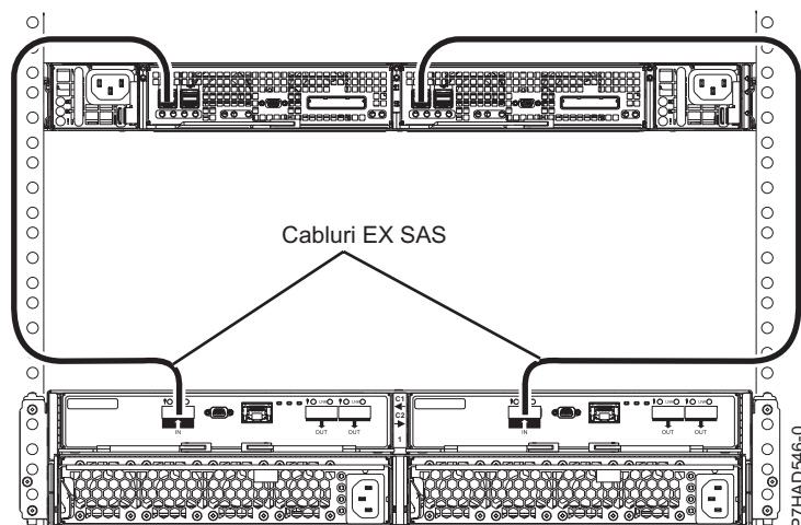
Figura 173. Conectarea unui sertar 5887 utilizând cabluri HD EX la un EDR1
