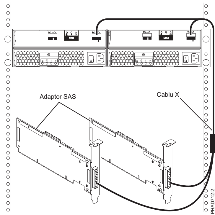
Figura 150. Două adaptoare RAID SAS la un sertar de expansiune pentru discuri într-o configurație RAID HA inițiator multiplu
