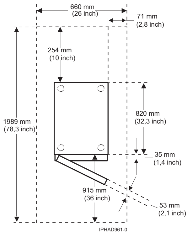
Figura 17. Vedere în plan pentru modelul 0554 și 7014-S11
