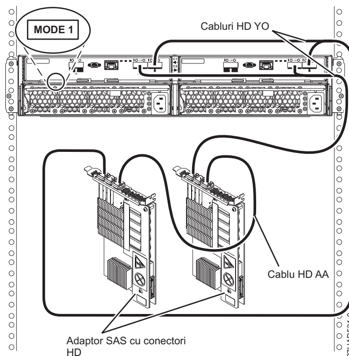
Figura 169. Conexiune de mod 1 a unui sertar 5887 la două adaptoare SAS cu conectori HD
