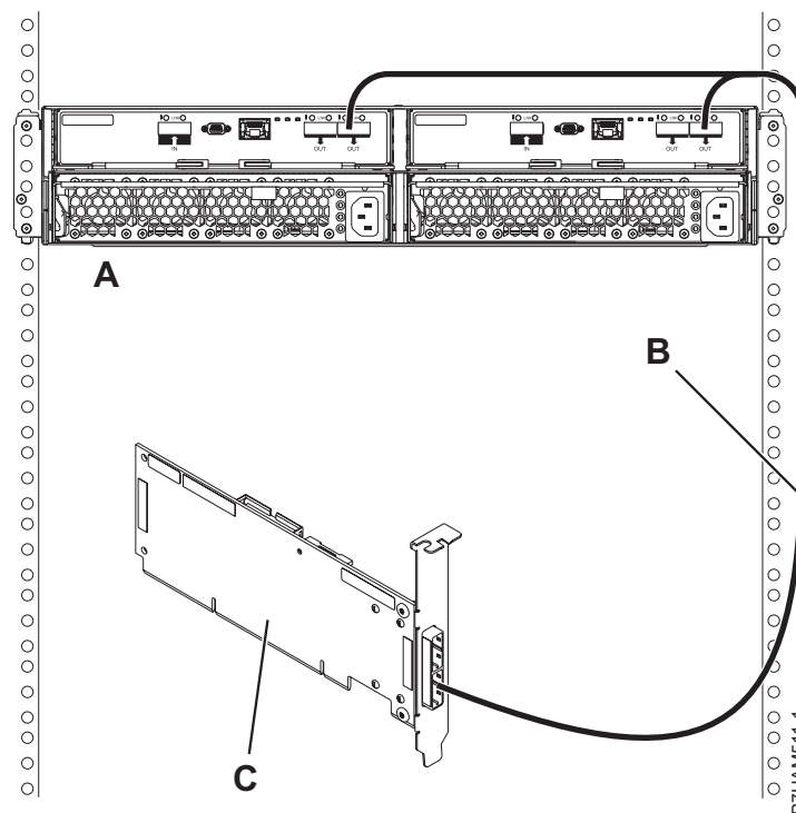
Figura 160. Conexiune mod 1 a sertarului 5887 utilizând un cablu YO către un adaptor singular SAS
