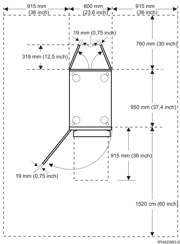
Figura 8. Vedere în plan pentru modelul 0555 și 7014-S25
