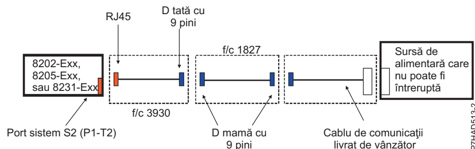
Figura 115. Cablarea sursei de alimentare neîntreruptibilă pentru 8246-L1C, 8246-L1S, 8246-L2C, și 8246-L2S
