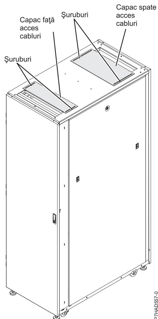
Figura 15. Capace de acces cabluri
