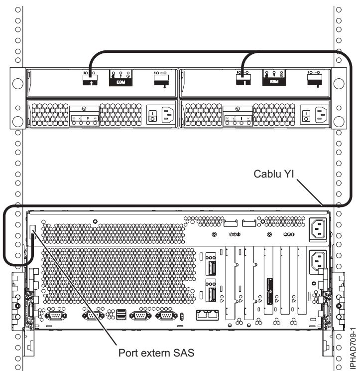
Figura 128. Port de adaptor SAS extern de sistem la un sertar de expansiune pentru discuri
