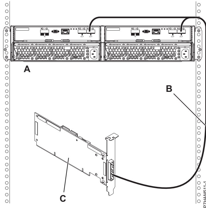
Figura 148. Conexiune mod 1 a sertarului 5887 utilizând un cablu YO către un adaptor singular SAS
