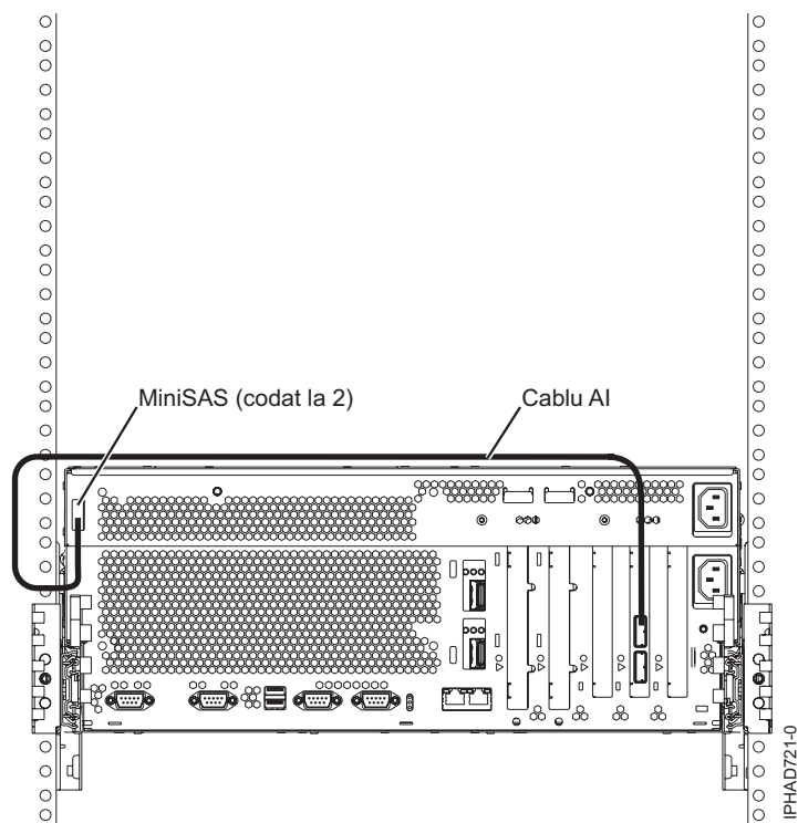
Figura 129. Adaptorul SAS la sloturi de disc SAS intern prin portul SAS extern al sistemului
