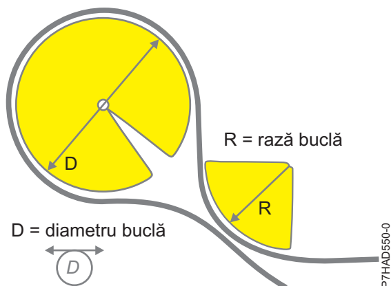
Figura 117. Rază arc cablu
