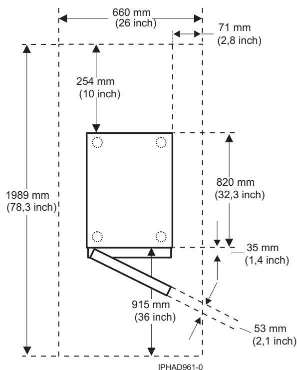
Figura 5. Vedere în plan pentru modelul 0554 și 7014-S11
