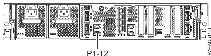
Figura 114. , 8246-L1C, 8246-L1D, 8246-L1S, 8246-L1T, 8246-L2C, 8246-L2D, 8246-L2S, and 8246-L2T- vedere din spate cu locația instalării cablurilor
