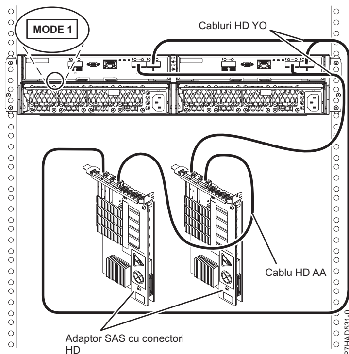
Figura 150. Conexiune de mod 1 a unui sertar 5887 la două adaptoare SAS cu conectori HD
