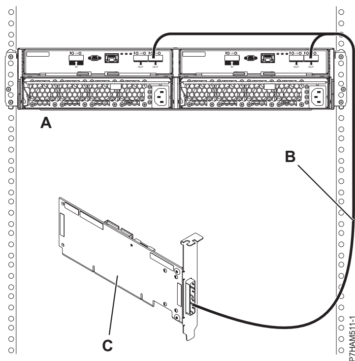
Figura 141. Conexiune mod 1 a sertarului 5887 utilizând un cablu YO către un adaptor singular SAS
