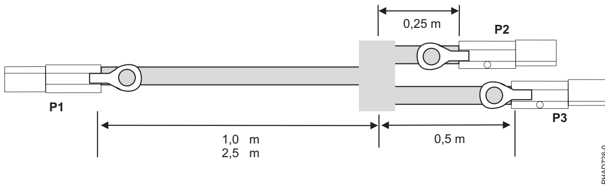
Figura 121. Lungimile de cablu pentru ansamblul cablu YI extern SAS
