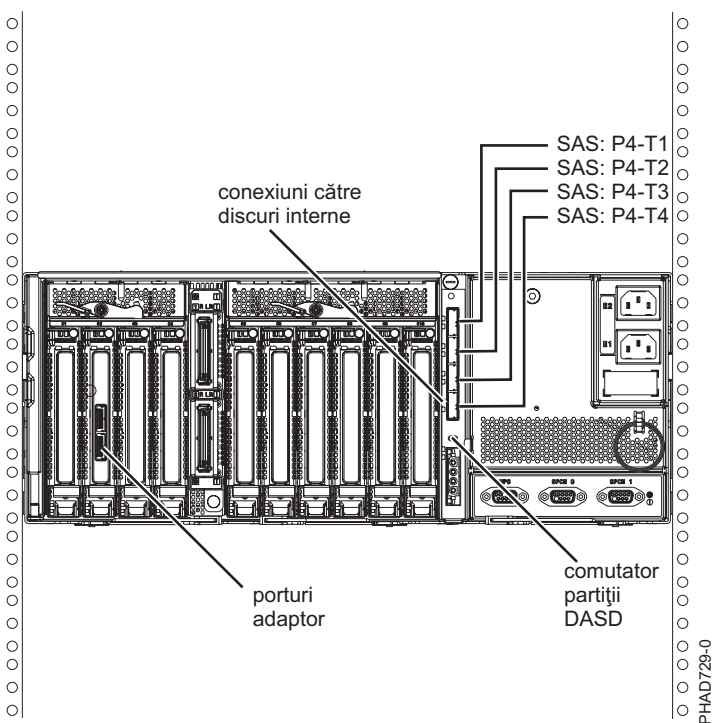
Figura 140. Două adaptoare SAS RAID la un sertar de expansiune pentru discuri într-o configurație JBOD HA inițializator multiplu
