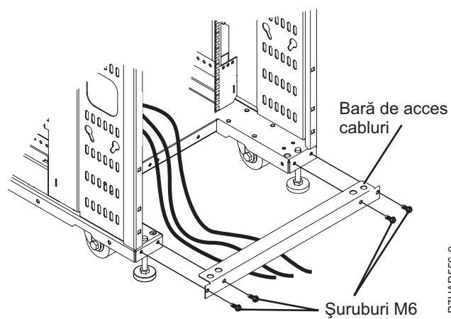
Figura 14. Bară de acces cabluri
