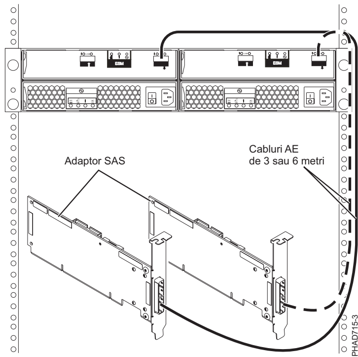
Figura 139. Două adaptoare SAS RAID la un sertar de expansiune pentru discuri într-o configurație JBOD HA inițializator multiplu
