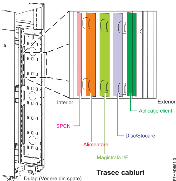
Figura 116. Lance punte gestiune de cabluri
