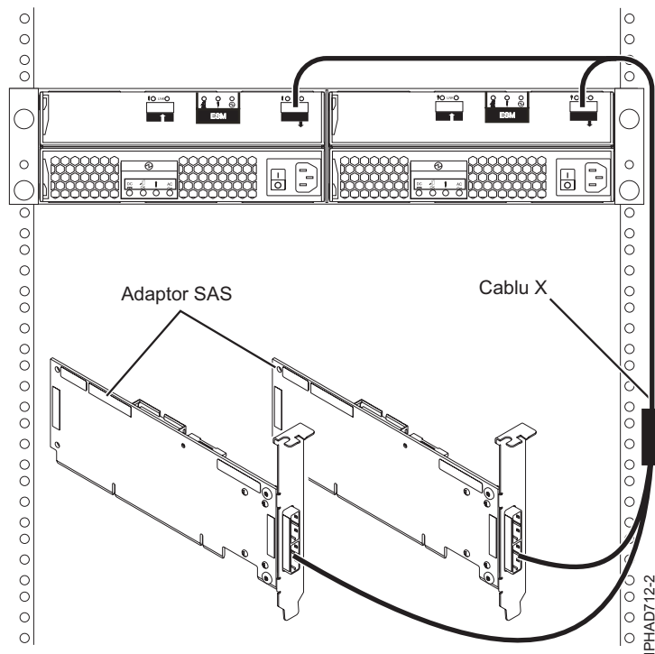
Figura 131. Două adaptoare RAID SAS la un sertar de expansiune pentru discuri într-o configurație RAID HA inițiator multiplu
