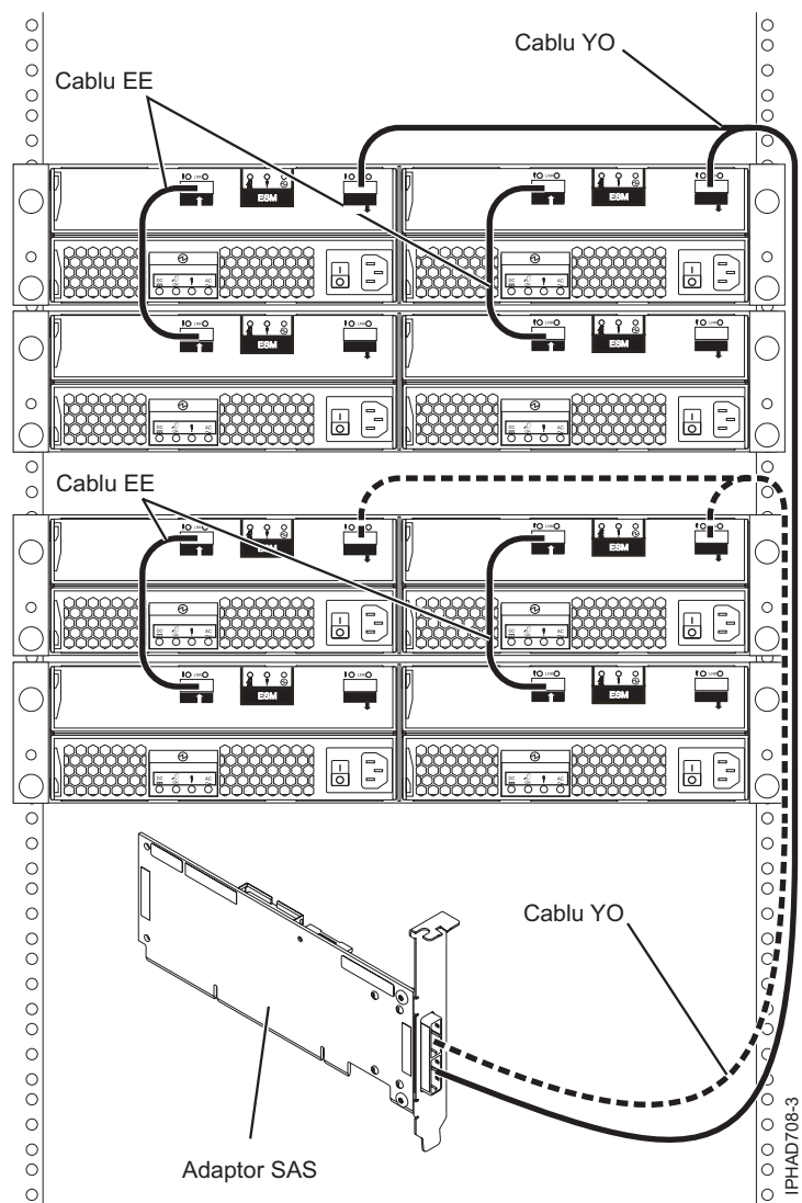
Figura 124. Adaptor SAS la patru sertare de expansiune pentru discuri
