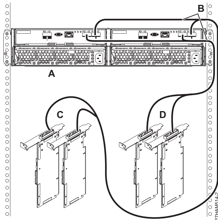
Figura 144. Conexiune mod 2 a unui sertar 5887 utilizând cabluri X către două perechi de adaptoare SAS
