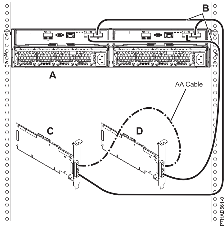
Figura 143. Conexiunea de mod 2 a unui sertar 5887 utilizând cabluri YO către două adaptoare simple SAS
