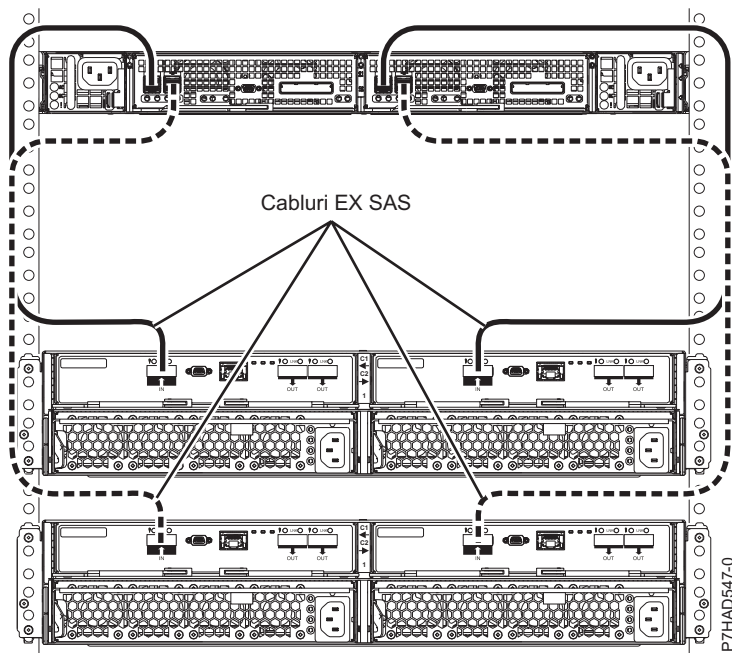
Figura 155. Conectarea a două sertare 5887 utilizând cabluri HD EX la un EDR1
