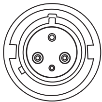
Figura 21. Tipul de priză IEC 60309 P+N+E
