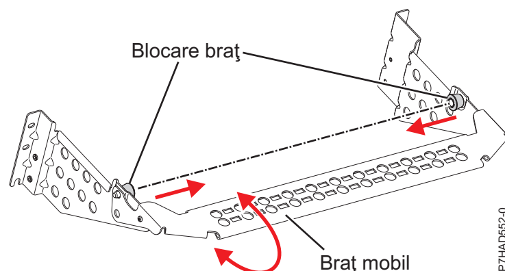
Figura 118. Colțar gestiune cablu
