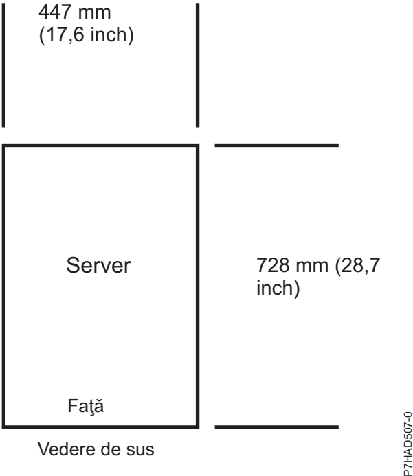
Figura 1. Vedere în plan pentru modelele 8246-L1C, 8246-L1D, 8246-L1S, 8246-L1T, 8246-L2C, 8246-L2D, 8246-L2S și 8246-L2T (server montat în dulap)
