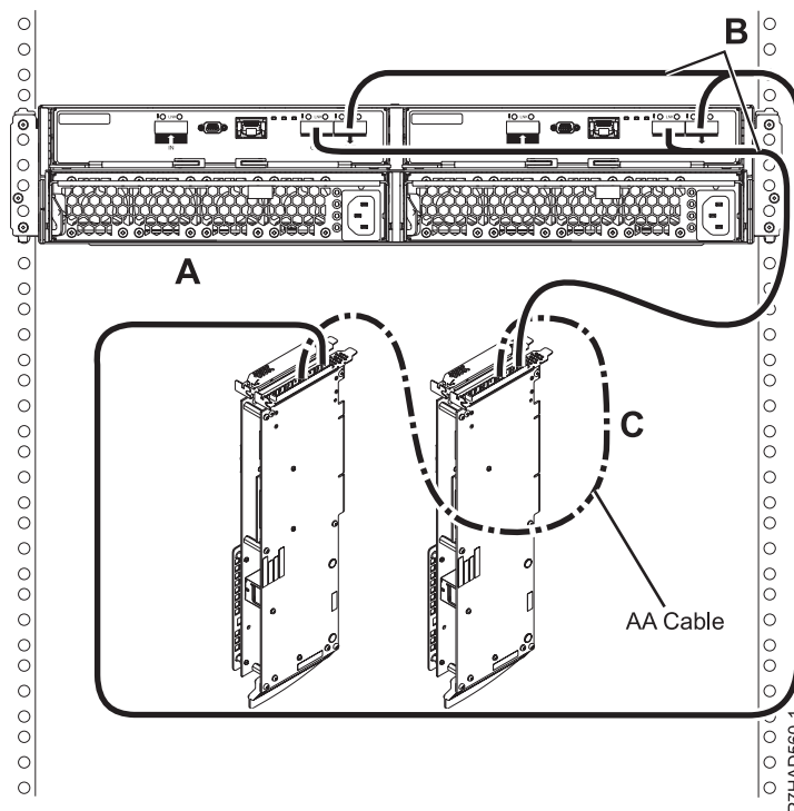
Figura 149. Conexiune mod 1 a unui sertar 5887 utilizând cabluri YO către adaptoare duble SAS
