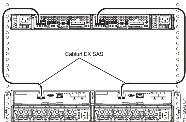
Figura 154. Conectarea unui sertar 5887 utilizând cabluri HD EX la un EDR1
