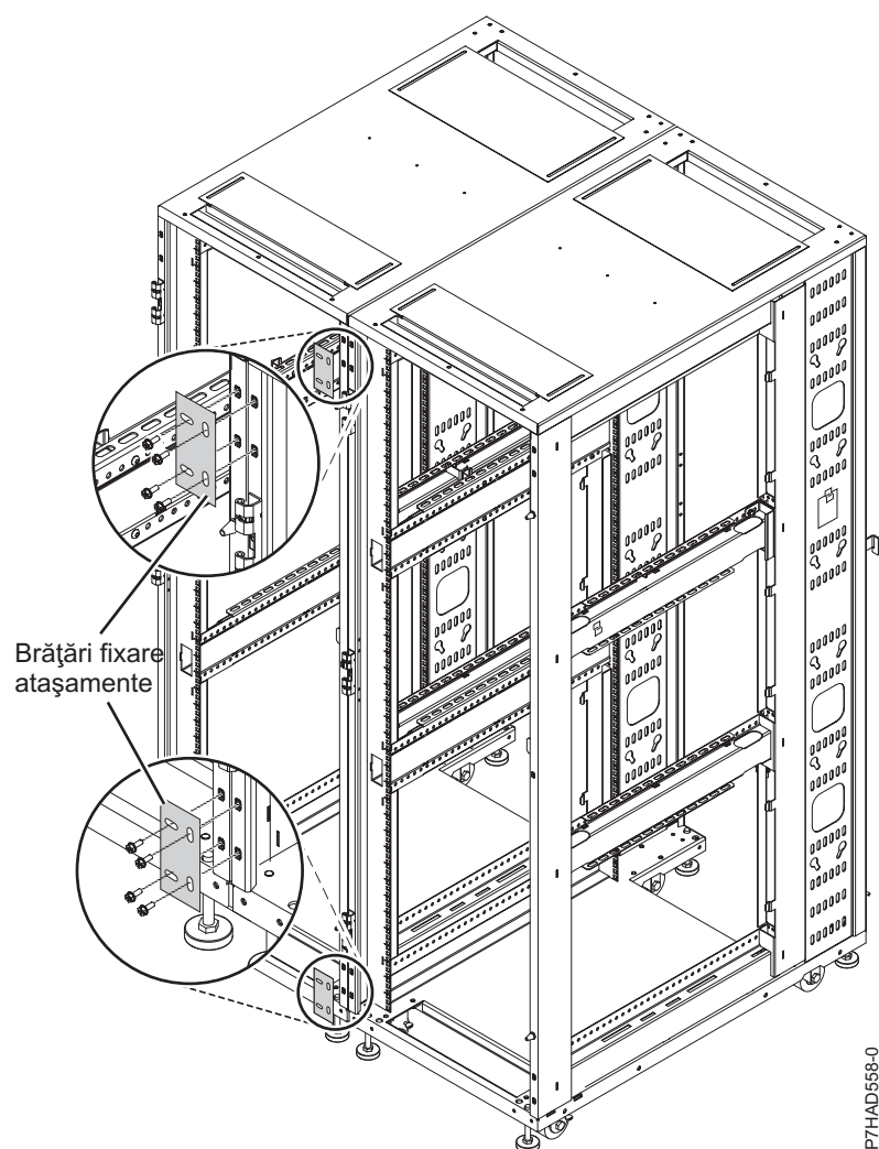
Figura 29. Colțare de atașare
