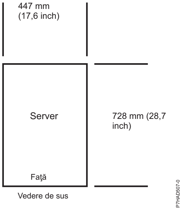
Figura 1. Vedere în plan pentru modelele 8231-E2B, 8231-E1C, 8231-E1D, 8231-E2C, 8231-E2D și 8268-E1D (server montat în dulap)
