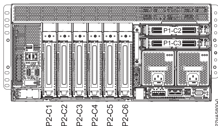
Figura 1. Vederea din spate a sistemului cu coduri de locație
