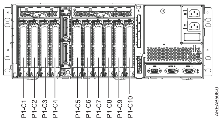
Figura 2. Vedere din spate. Această imagine prezintă vederea din spate a unității de expansiune.
