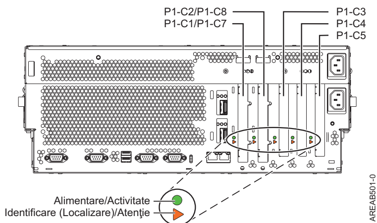
Figura 1. Vederea din spate a sistemului cu coduri de locație. Tabela 4 la pagina 11 afișează vederea din spate a sistemului cu codurile de locație pentru sloturile de adaptoare PCI și GX.
