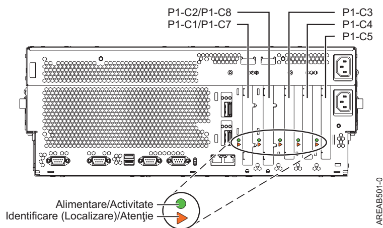
Figura 2. Vederea din spate a incintei cu codurile de locație. Tabela 11 afișează vederea din spate a unității sistemului cu codurile locației pentru sloturile PCI și GX+.
