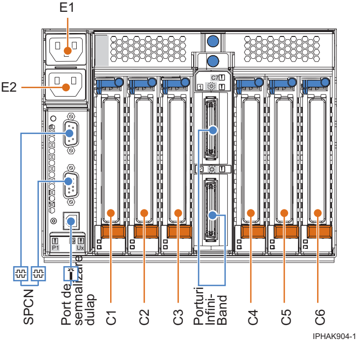
Figura 5. Vedere din spate
