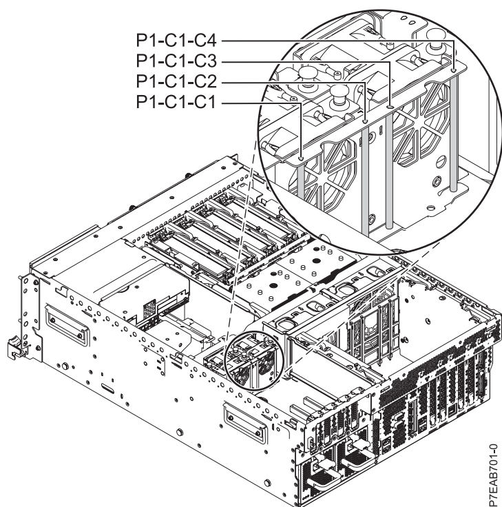
Figura 3. Extenderul PCI cu codurile de locație în sistemele 8202-E4B și 8205-E6B
