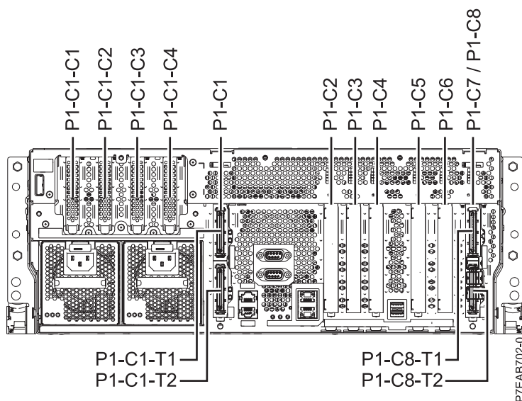
Figura 4. Vedere din spate a sistemului indicând sloturile PCI cu codurile lor de locație
