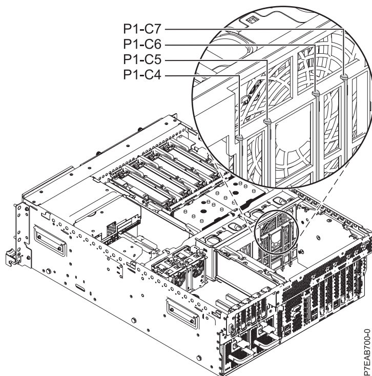
Figura 2. Codurile de locație ale sloturilor PCI în sistemele 8202-E4B și 8205-E6B
