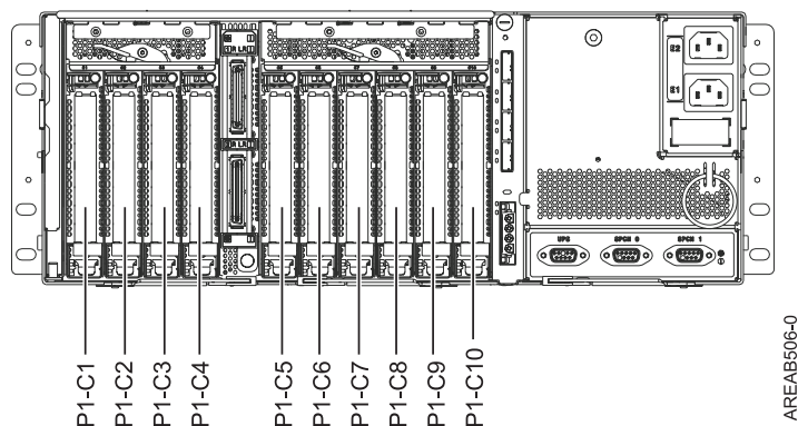
Figura 6. Vedere din spate. Această imagine prezintă vederea din spate a unității de expansiune.
