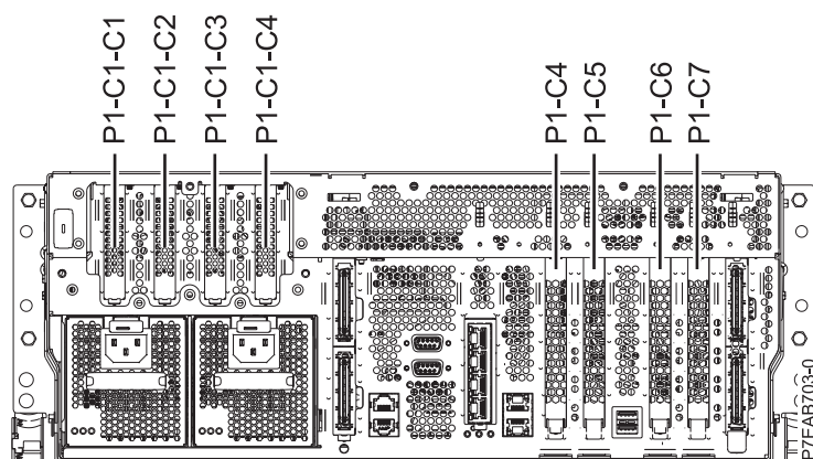
Figura 1. Vederea din spate pentru sistemele 8202-E4B și 8205-E6B cu codurile de locație ale sloturilor PCI
