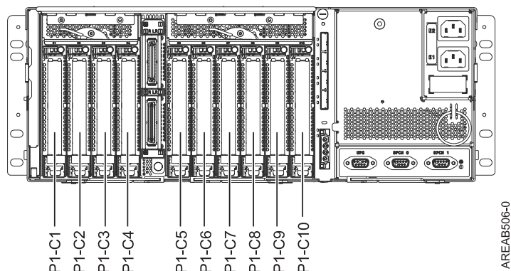
Figura 3. Vedere din spate. Această imagine prezintă vederea din spate a unității de expansiune.
