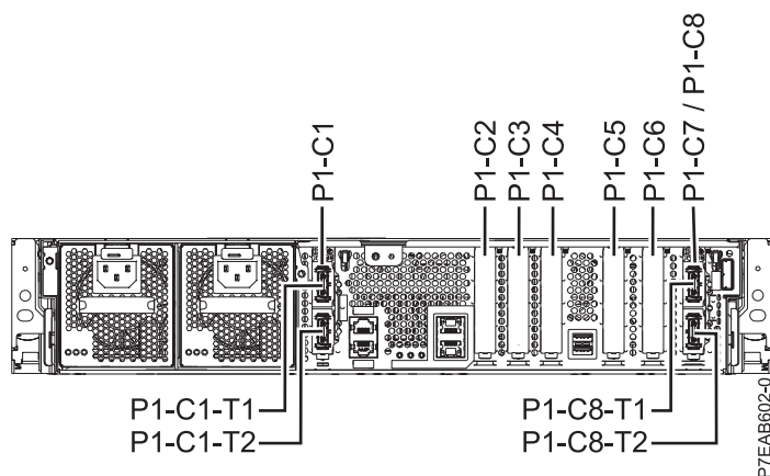
Figura 1. Vederea din spate a sistemului cu coduri de locație
