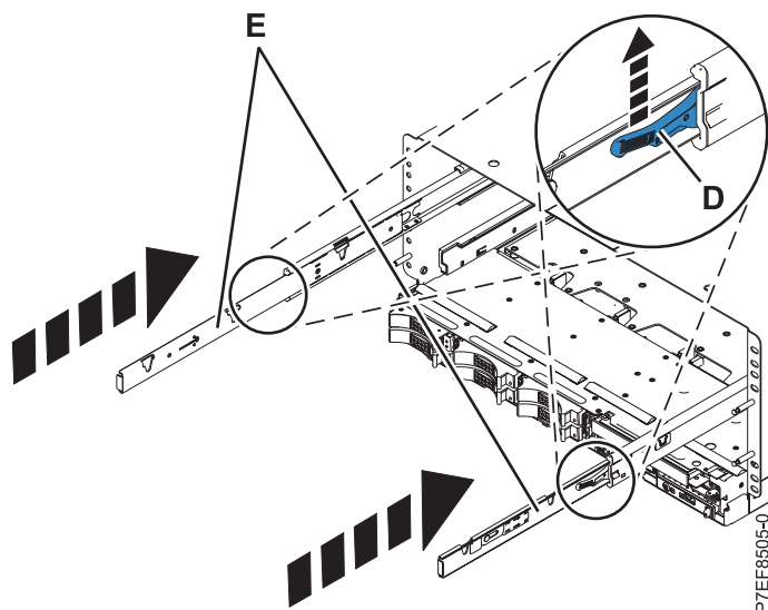
Figura 10. Desbloquear os trincos de segurança da calha
