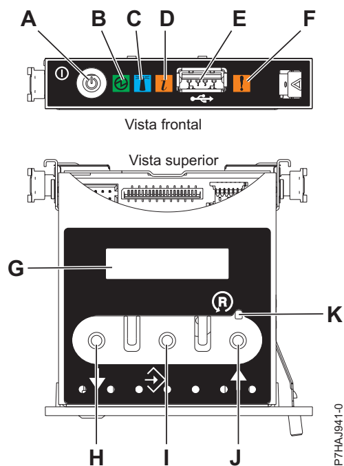
Figura 5. Painel de controlo
