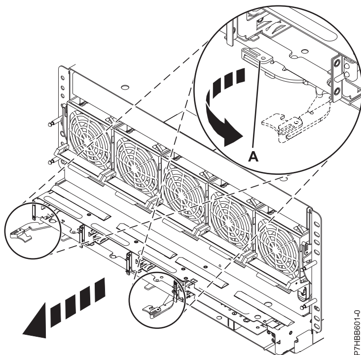
Figura 2. Remover o painel posterior da unidade de disco
