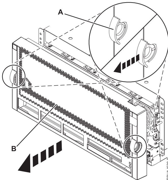
Figura 6. Remover a parte frontal
