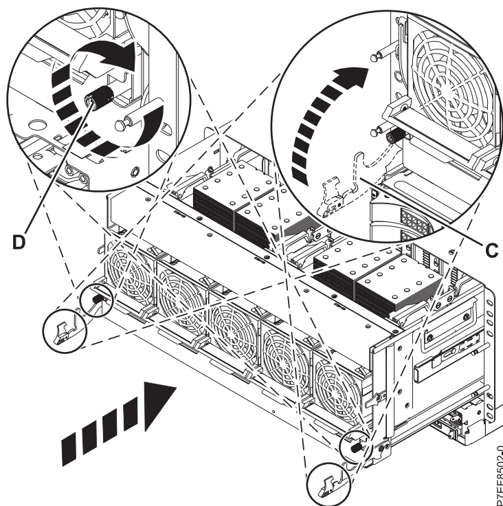
Figura 11. Bloquear os fechos da unidade de sistema
