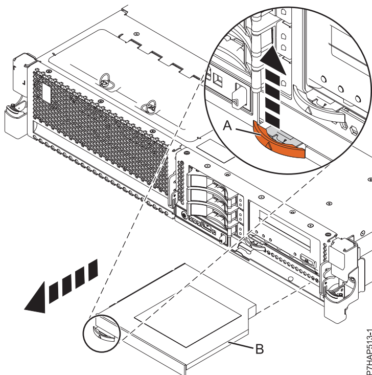
Figura 5. Remover o dispositivo de suporte de dados SAS do painel posterior da unidade de disco
