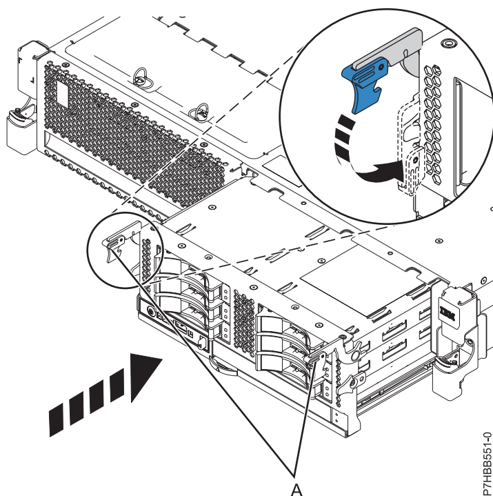
Figura 9. Instalar o painel posterior preenchido com unidades de disco num modelo instalado em bastidor
