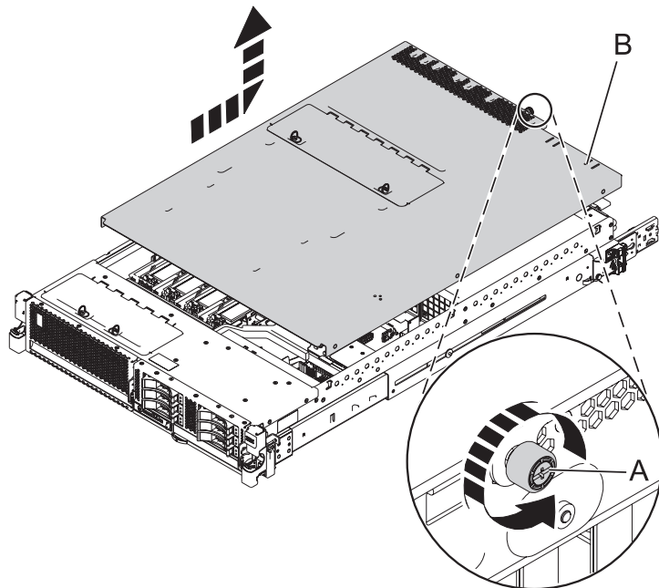
Figura 15. Remover a tampa de acesso ao serviço
