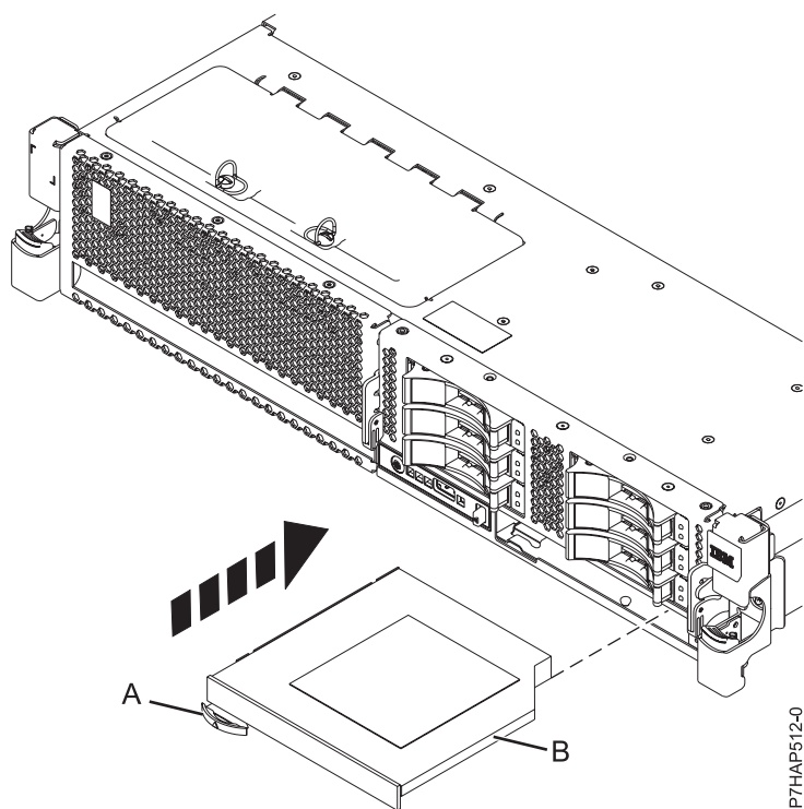
Figura 12. Instalar o dispositivo de suporte de dados Slimline
