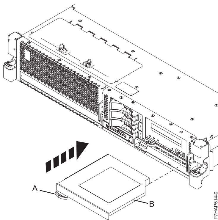
Figura 11. Instalar o dispositivo de suporte de dados SAS
