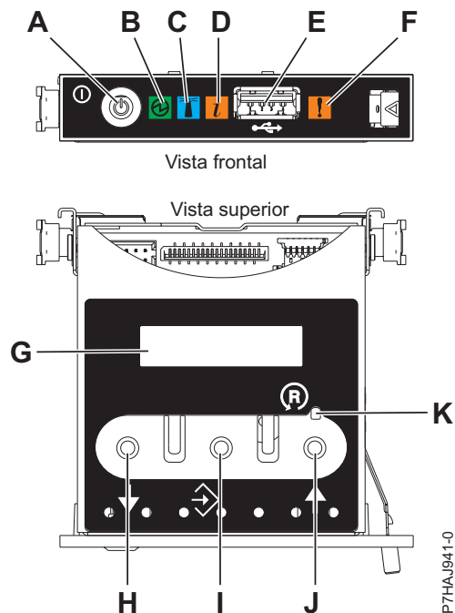
Figura 13. Painel de controlo
