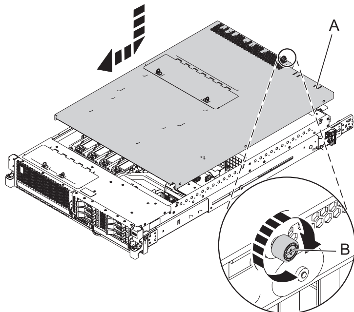
Figura 16. Instalar a tampa de acesso a assistência
