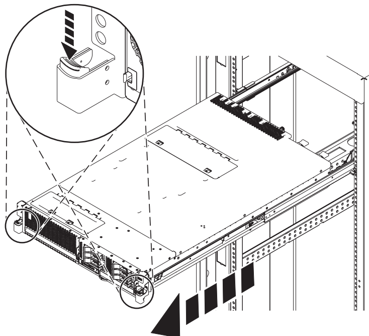
Figura 17. Colocar o sistema em posição de assistência
