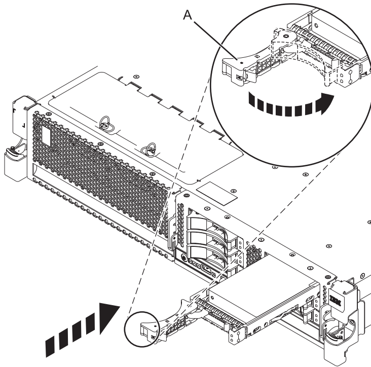
Figura 10. Instalar as unidades de disco do painel posterior
