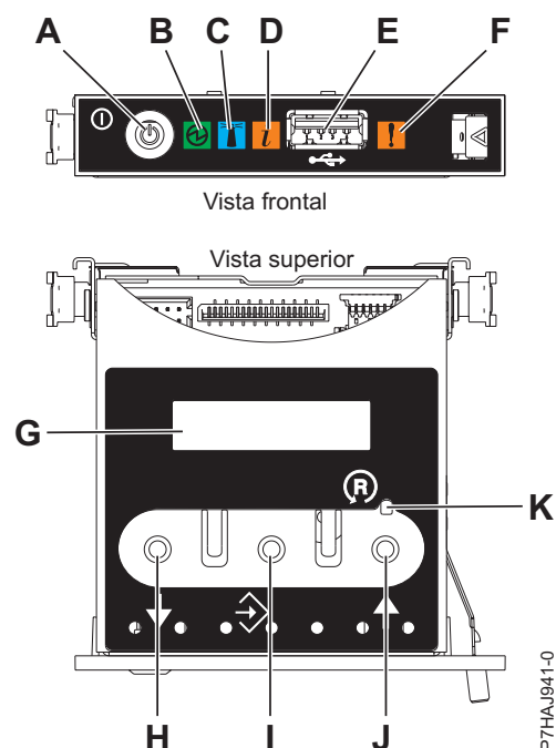
Figura 21. Painel de controlo
