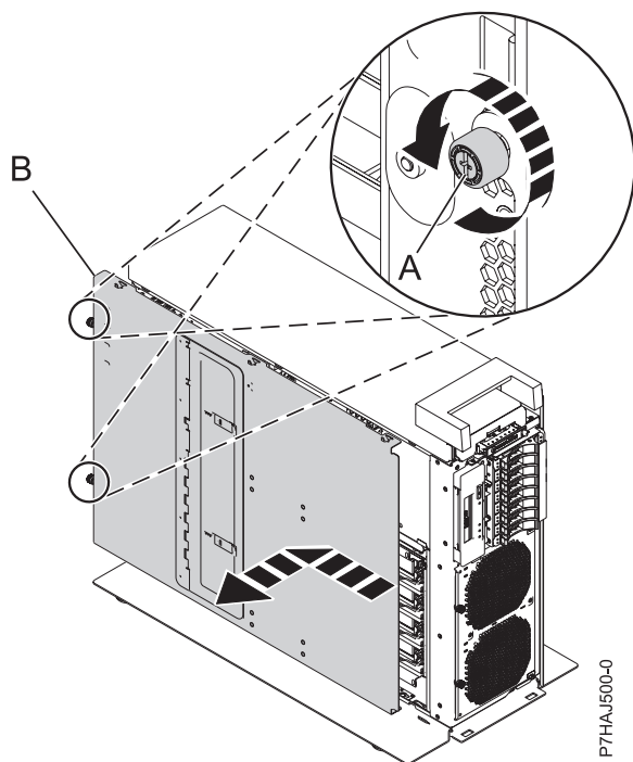
Figura 29. Remover a tampa de acesso a assistência interna
