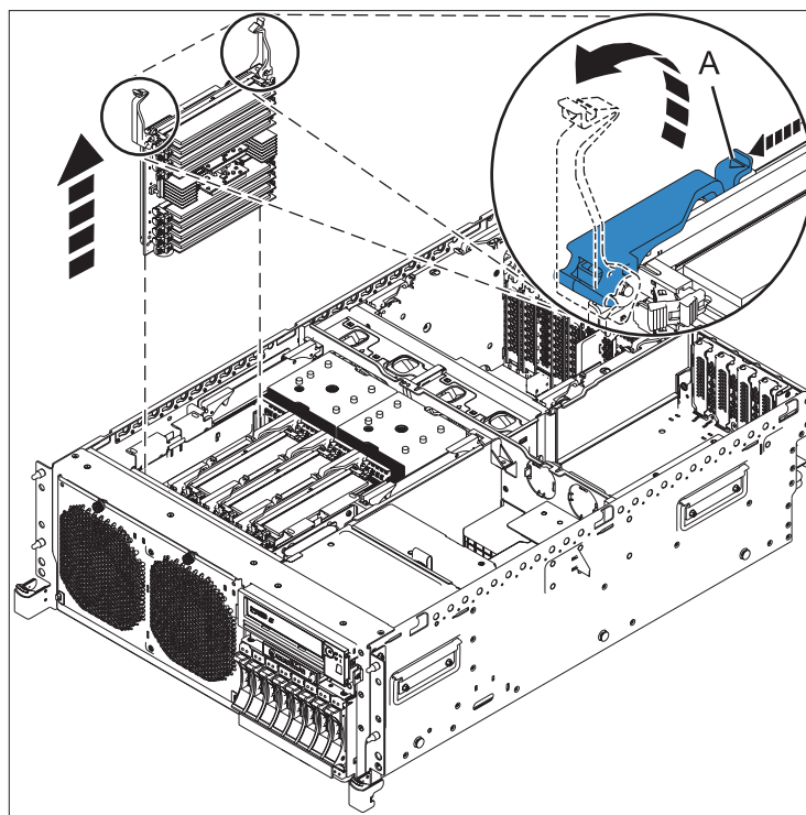
Figura 8. Remover o alimentador de memória
