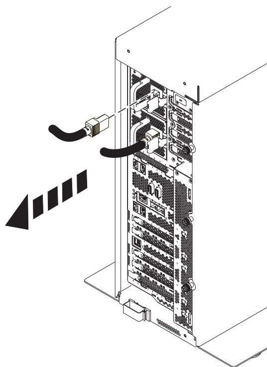
Figura 38. Remover os cabos de alimentação de um sistema autónomo
