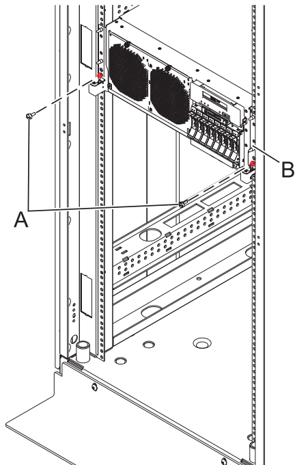
Figura 36. Colocar a unidade de sistema na posição de funcionamento
