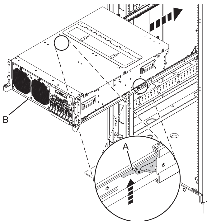
Figura 35. Colocar a unidade de sistema na posição de funcionamento
