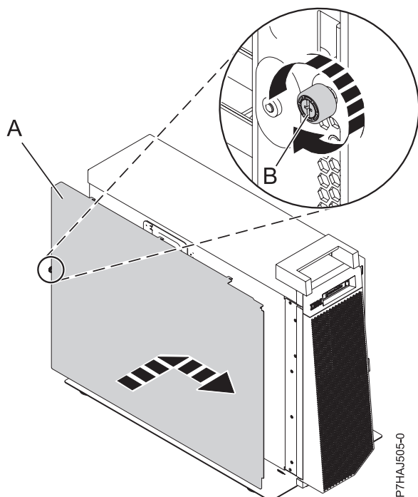
Figura 32. Instalar a tampa de acesso a assistência externa
