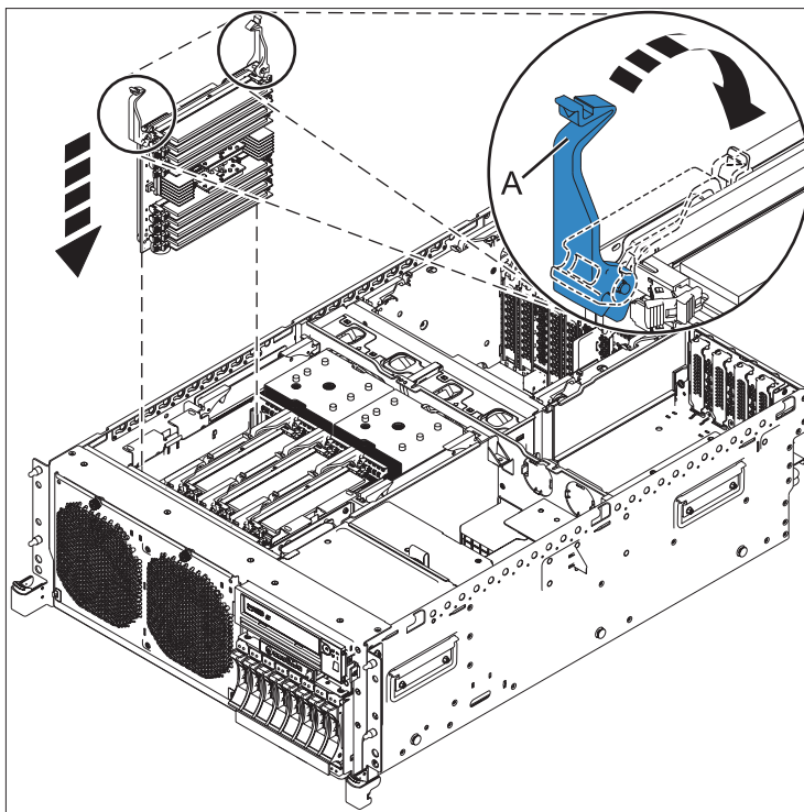
Figura 2. Instalar um alimentador de memória
