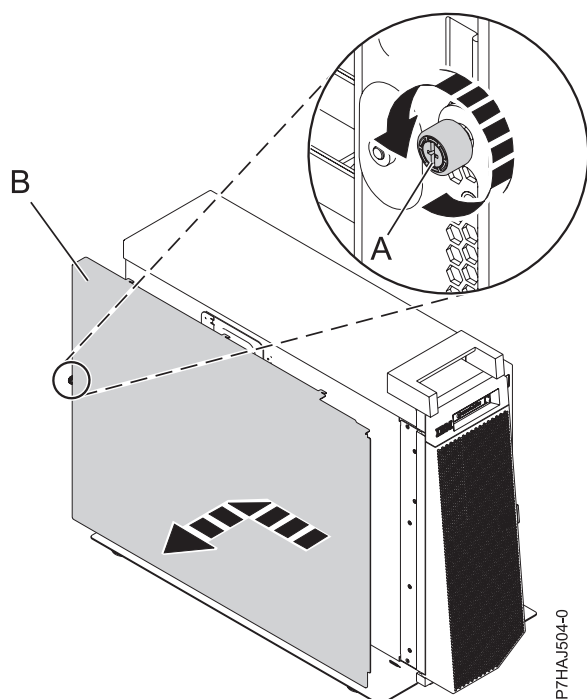
Figura 28. Instalar a tampa de acesso a assistência externa
