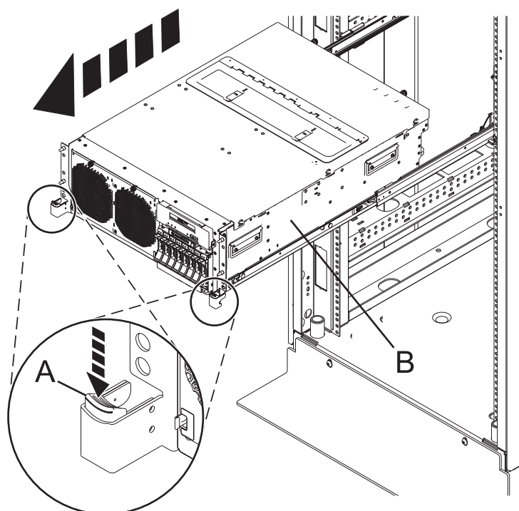
Figura 34. Bloquear a unidade de sistema em posição de assistência
