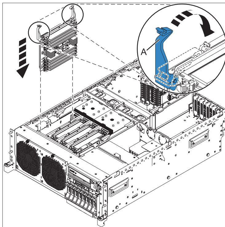
Figura 6. Substituir um alimentador de memória
