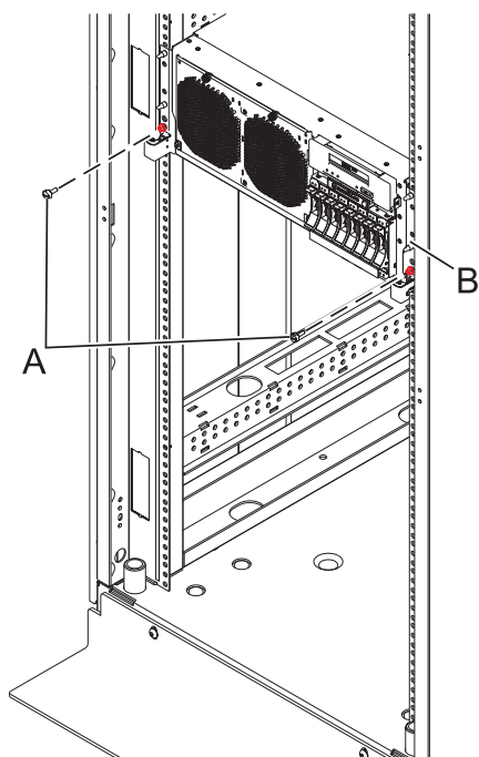
Figura 33. Colocar a unidade de sistema em posição de assistência
