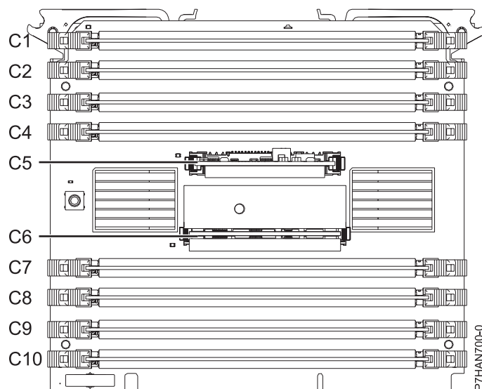
Figura 11. Posições das ranhuras para módulos de memória para o 8202-E4B ou 8205-E6B
