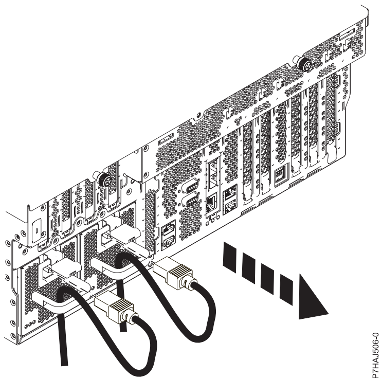
Figura 13. Desligar os cabos de alimentação
