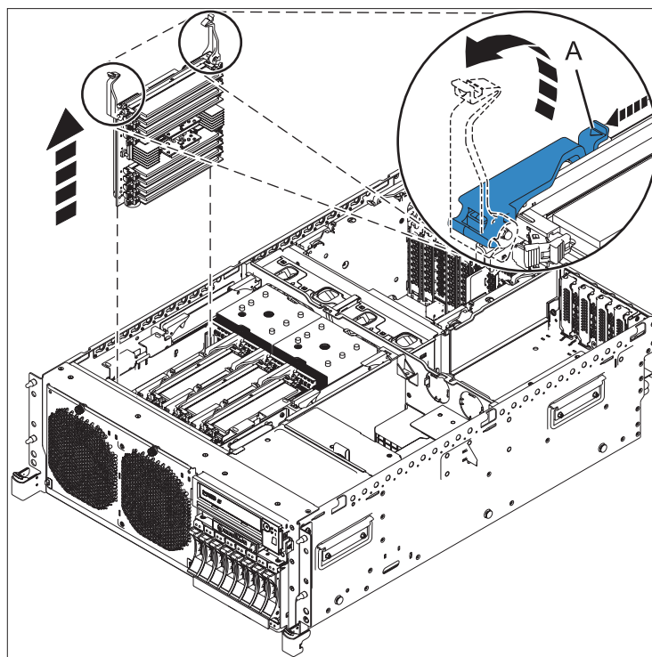
Figura 14. Remover um alimentador de memória
