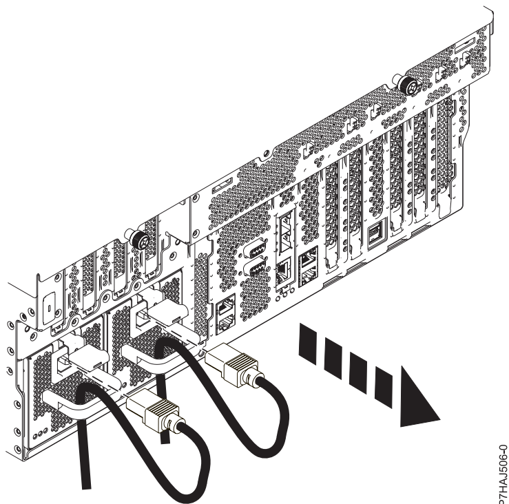
Figura 17. Desligar os cabos de alimentação
