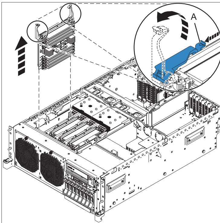
Figura 4. Remover um alimentador de memória
