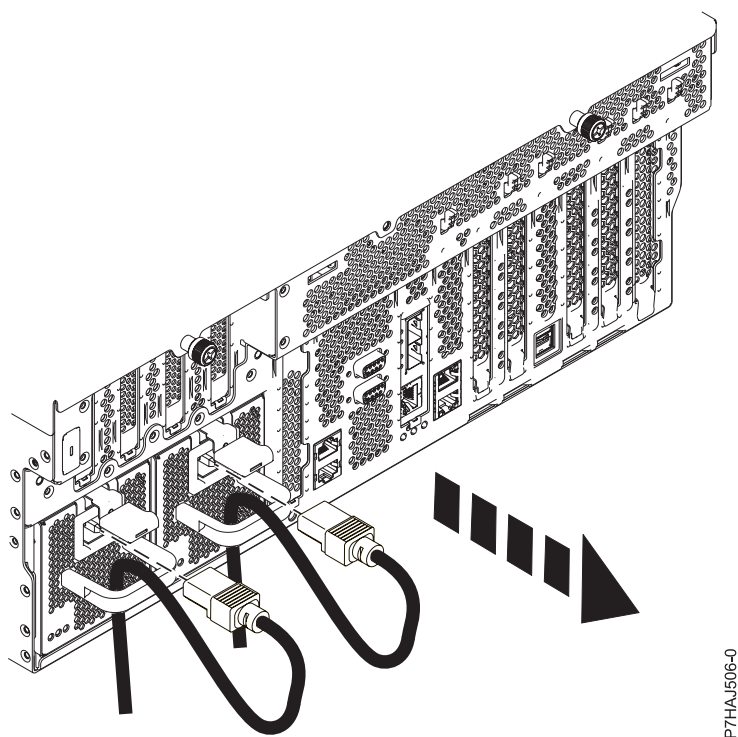
Figura 5. Desligar os cabos de alimentação
