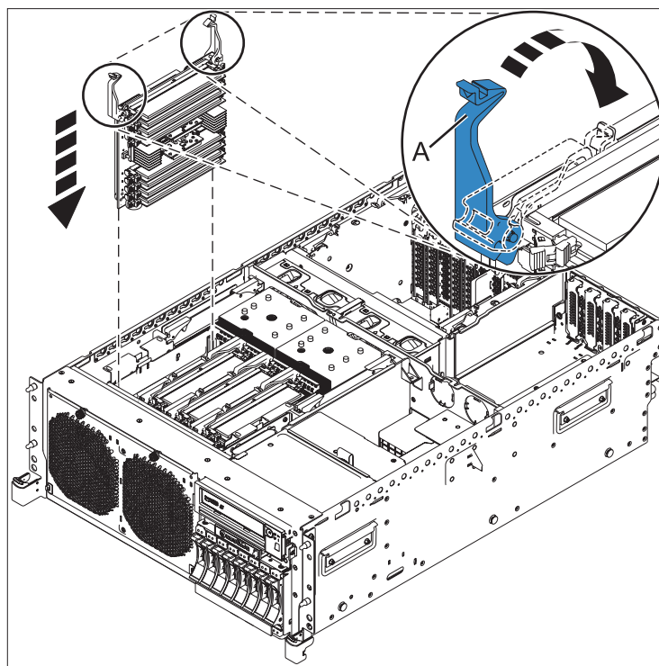
Figura 19. Substituir um alimentador de memória
