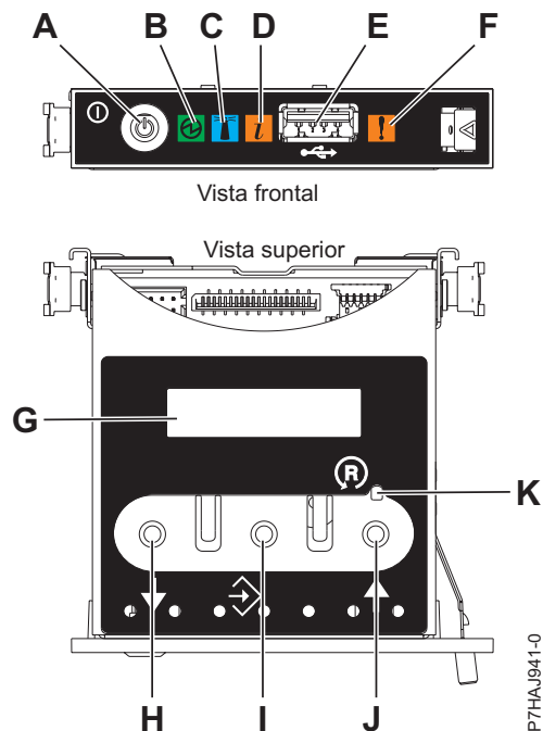
Figura 20. Painel de controlo
