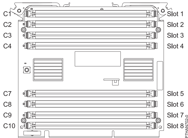
Figura 12. Localizações de ranhuras de módulos de memória para o 8202-E4C, 8202-E4D, 8205-E6C ou 8205-E6D
