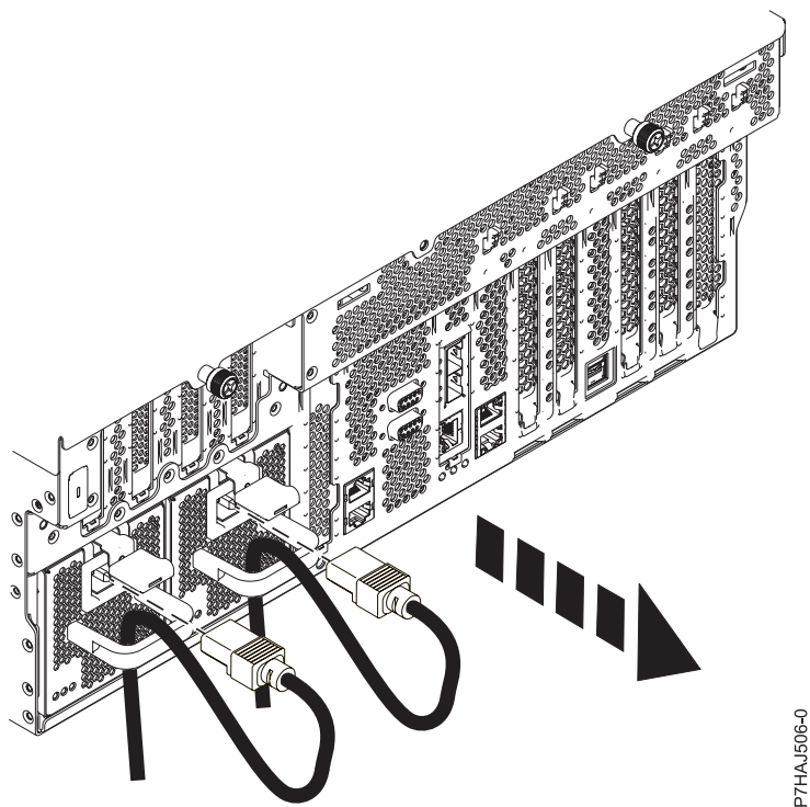
Figura 37. Remover os cabos de alimentação de um sistema instalado em bastidor
