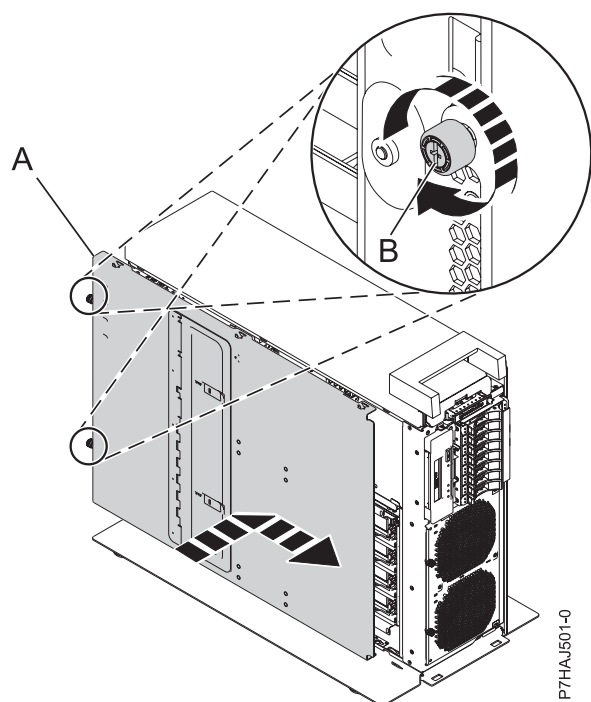
Figura 31. Instalar a tampa de acesso a assistência interna
