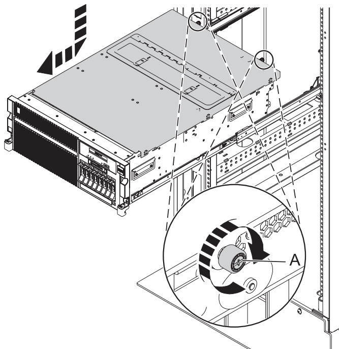
Figura 30. Instalar a tampa de acesso a assistência
