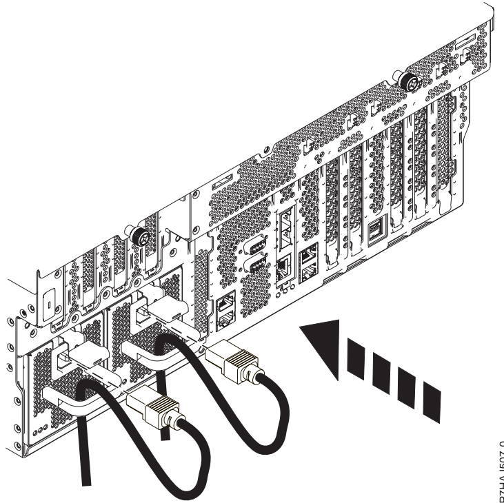
Figura 39. Ligar os cabos de alimentação
