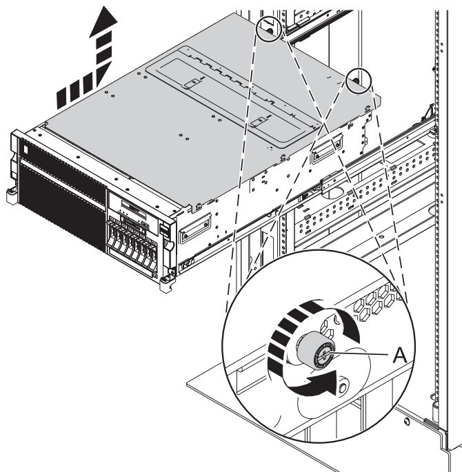
Figura 27. Remover a tampa de acesso a assistência
