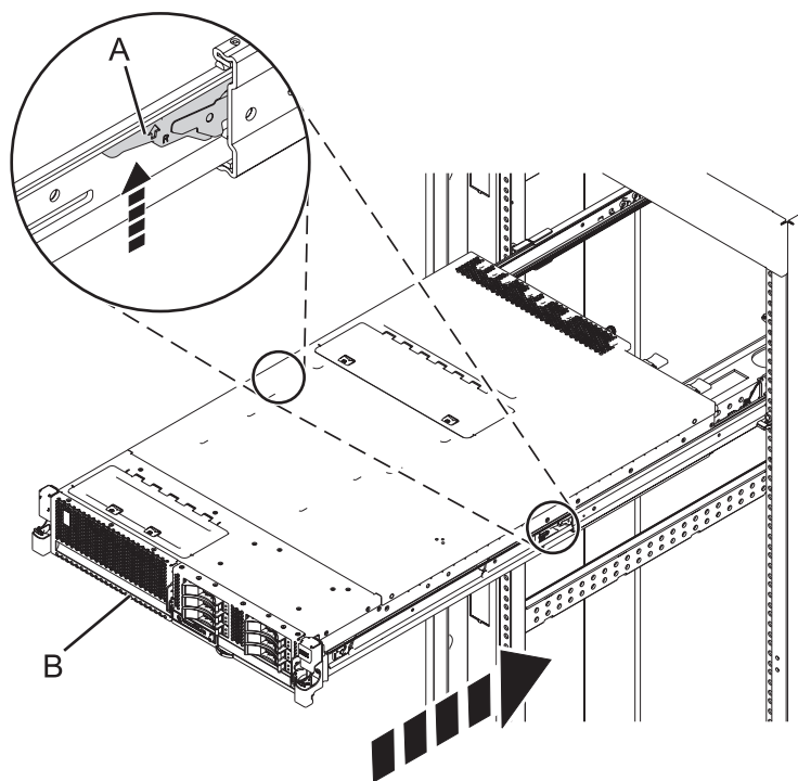
Figura 16. Soltar os trincos da calha de segurança
