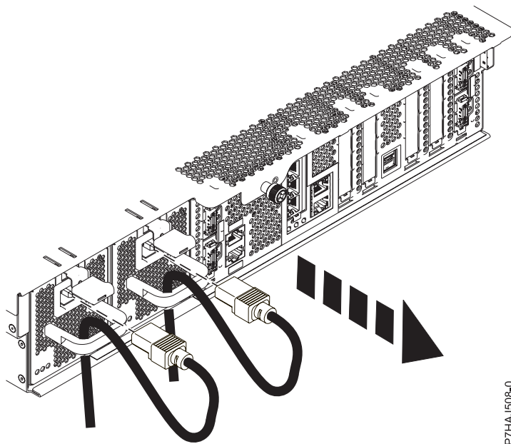
Figura 20. Remover os cabos de alimentação
