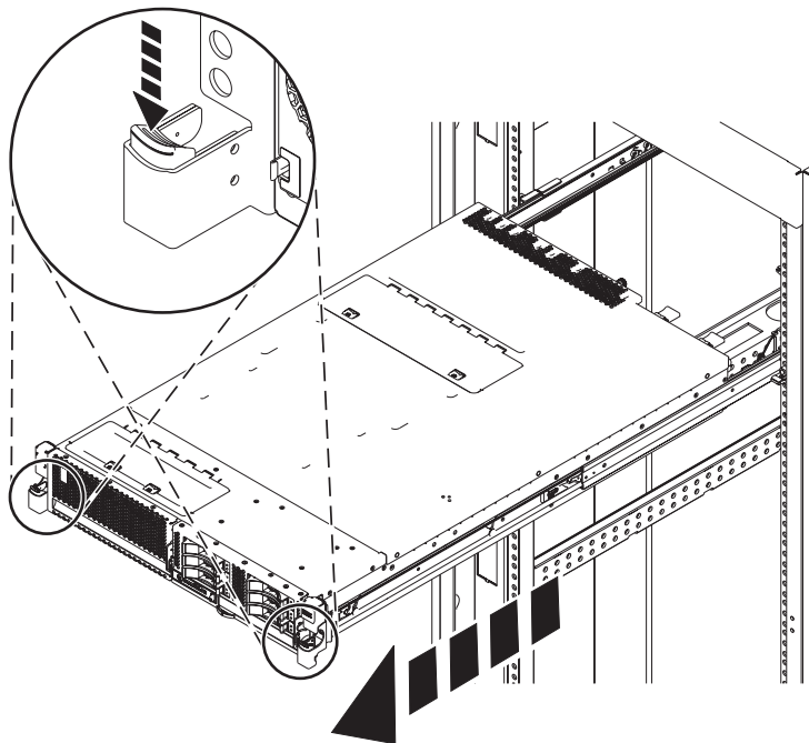
Figura 15. Colocar o sistema em posição de assistência
