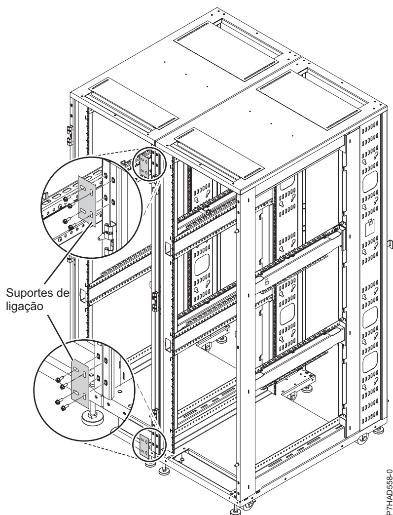
Figura 28. Suportes de ligação
