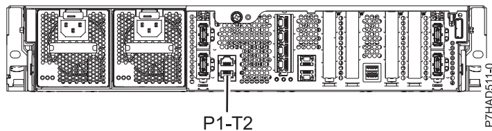
Figura 131. Vista posterior de 8231-E2B, 8231-E1C, 8231-E1D, 8231-E2C, 8231-E2D, e 8268-E1D com localização da instalação dos cabos
