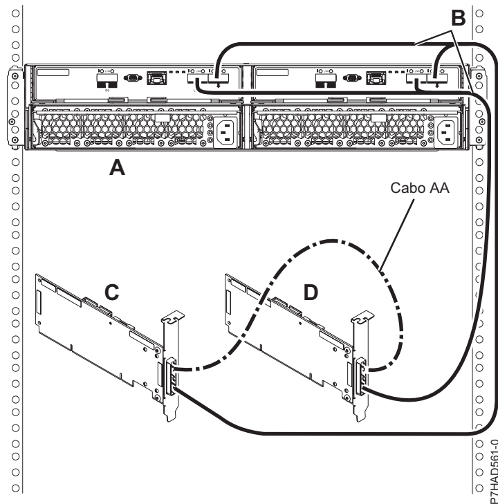
Figura 162. Ligação de modo 2 de uma gaveta 5887 utilizando cabos YO a dois adaptadores SAS únicos
