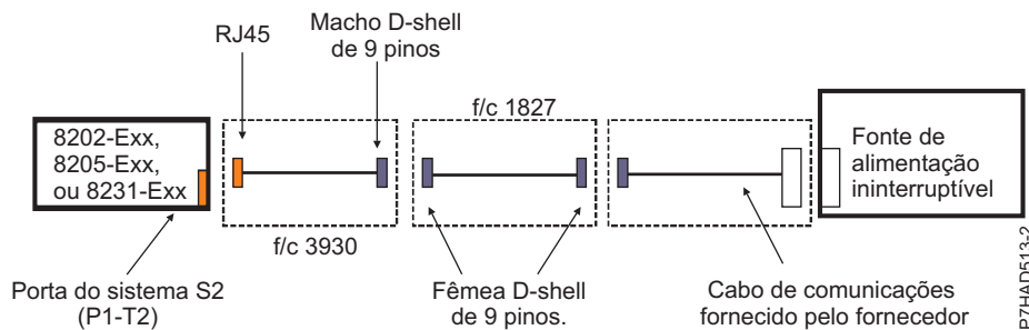
Figura 134. Ligações da fonte de alimentação ininterruptível para o 8202-E4B, 8202-E4C, 8205-E6B, 8205-E6C, 8231-E2B, 8231-E1C, 8231-E1D, 8231-E2C, 8231-E2D, e 8268-E1D
