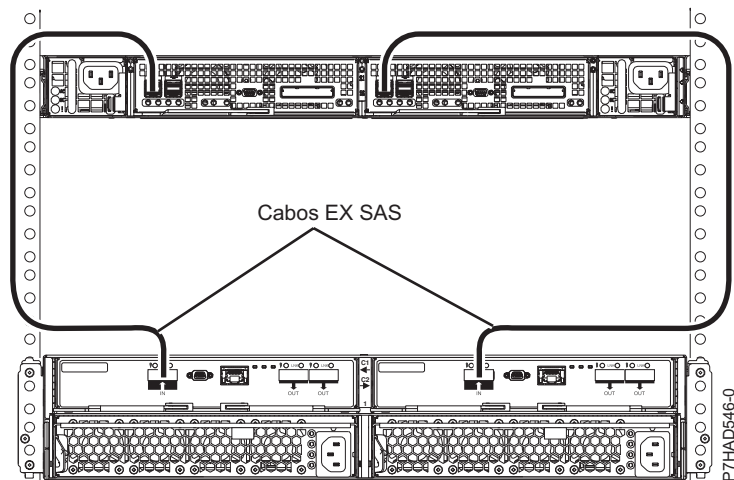
Figura 173. Ligação de uma gaveta 5887 utilizando cabos HD EX para um EDR1
