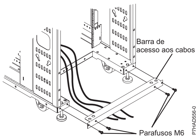
Figura 26. Barra de acesso de cabos
