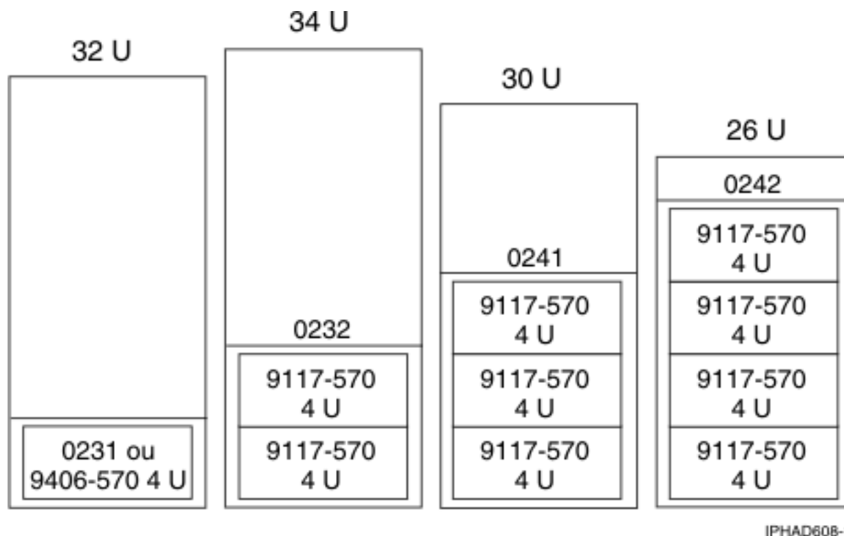
Figura 8. 570 no bastidor
