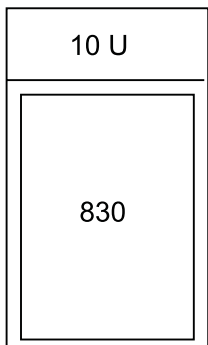
Figura 3. Configuração do bastidor 0550
