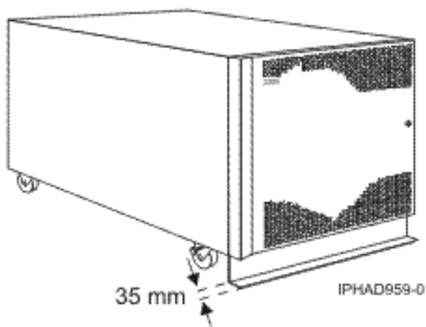
Figura 16. Modelo 0554 e 7014-S11 com barra estabilizadora
