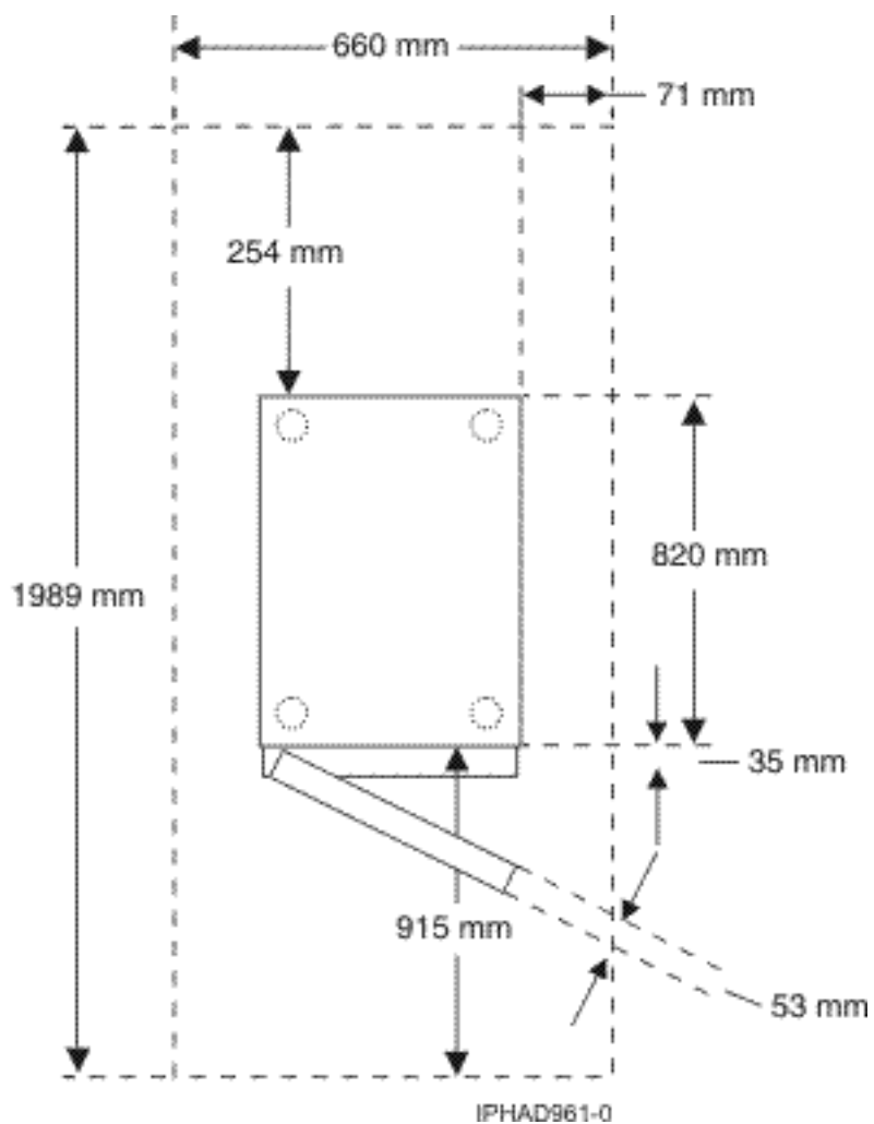
Figura 17. Vista de plano do modelo 0554 e 7014-S11
