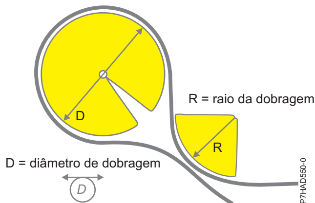
Figura 136. Raio da dobragem dos cabos
