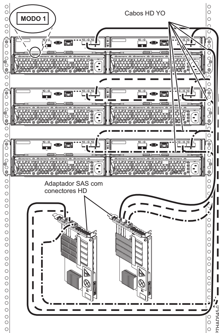
Figura 171. Ligação de modo 1 de três gavetas 5887 para dois adaptadores SAS com conectores HD
