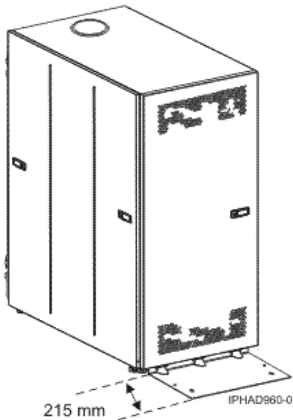
Figura 19. Modelo 0555 e 7014-S25 com pés estabilizadores
