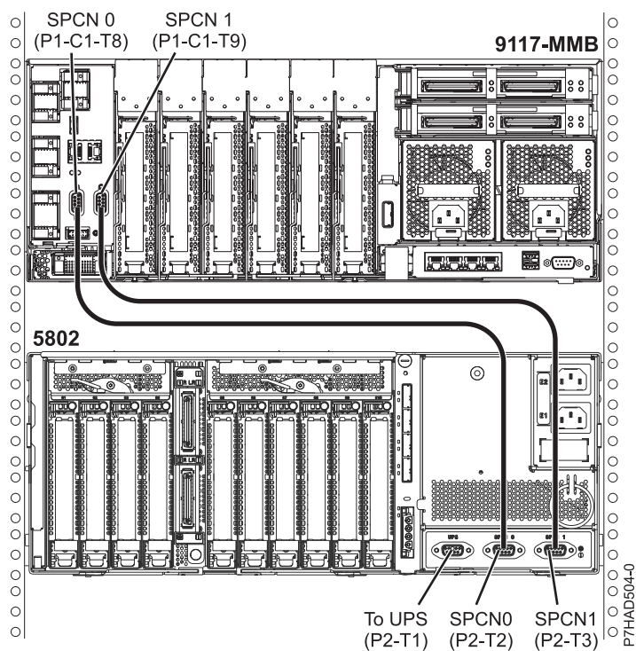
Figura 131. Localização da instalação dos cabos na vista posterior de 8412-EAD, 9117-MMB, 9117-MMC, 9117-MMD, 9179-MHB, 9179-MHC, 9179-MHD, e 5208 ou 5877
