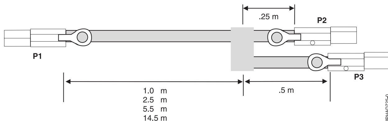
Figura 139. Comprimentos de cabo de montagem de cabo YO externo SAS
