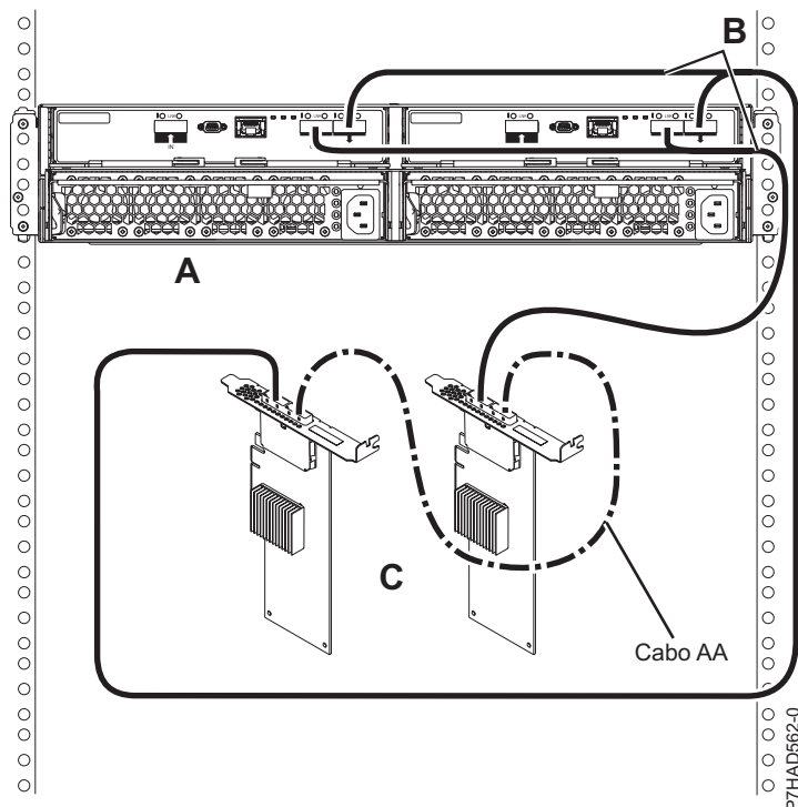
Figura 161. Ligação de modo 1 de uma gaveta 5887 utilizando cabos YO para adaptadores SAS duplos
