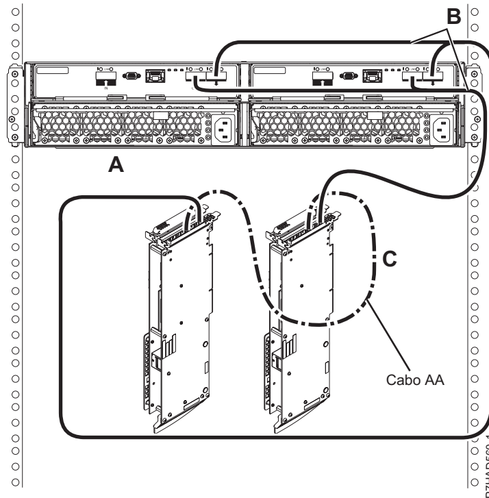
Figura 168. Ligação de modo 1 de uma gaveta 5887 utilizando cabos YO para adaptadores SAS duplos
