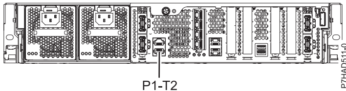
Figura 132. Vista posterior de 8231-E2B, 8231-E1C, 8231-E1D, 8231-E2C, 8231-E2D, e 8268-E1D com localização da instalação dos cabos
