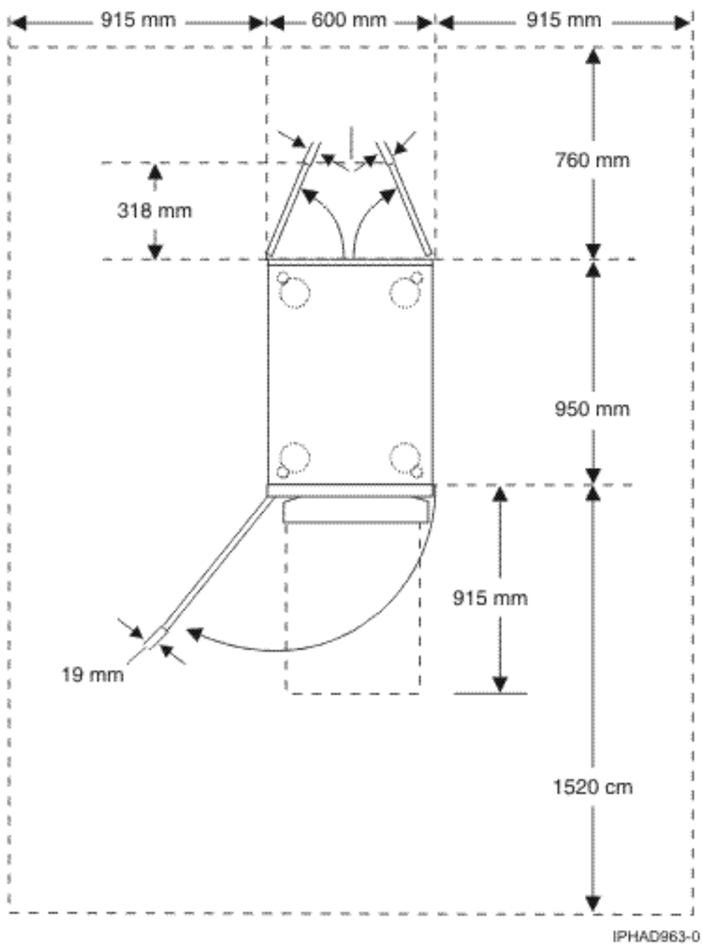
Figura 20. Vista em plano do modelo 0555 e 7014-S25
