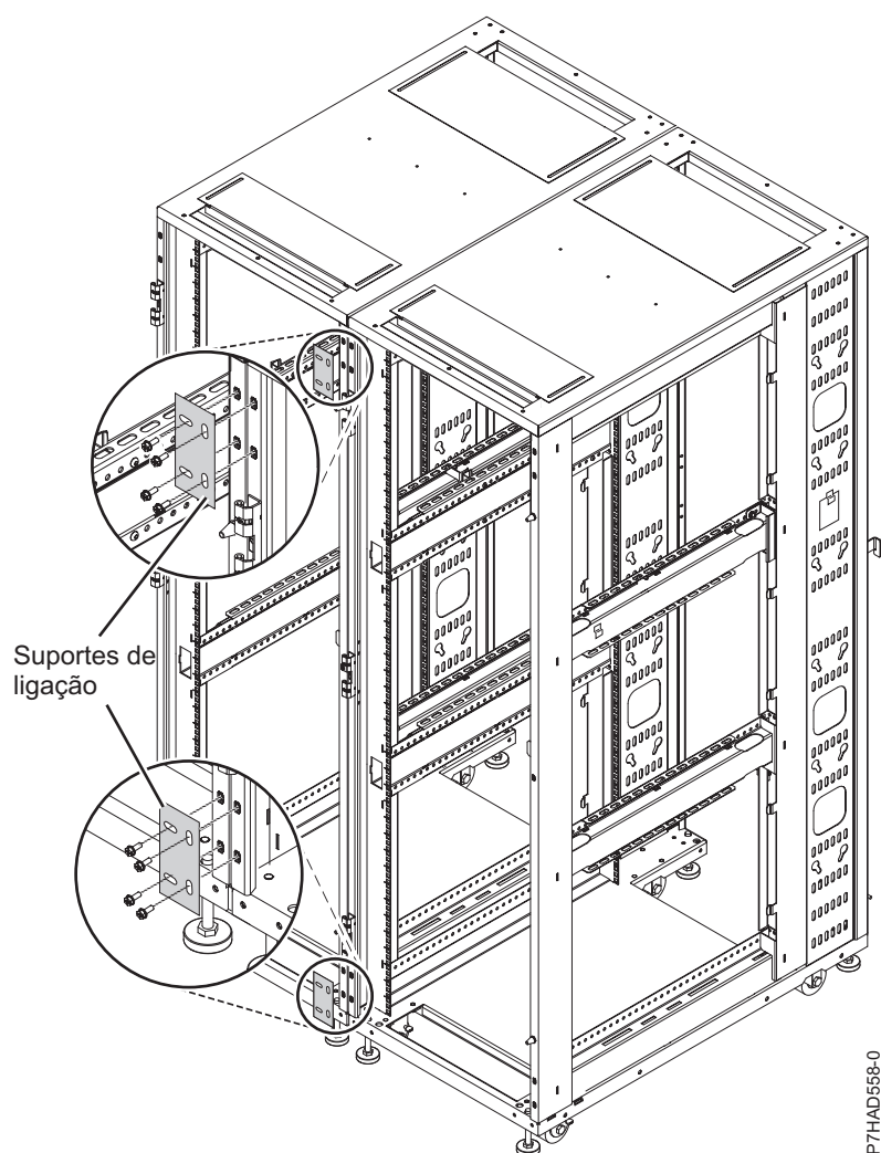
Figura 29. Suportes de ligação
