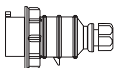
Figura 31. Tipo de conector IEC 60309 3P+N+E
