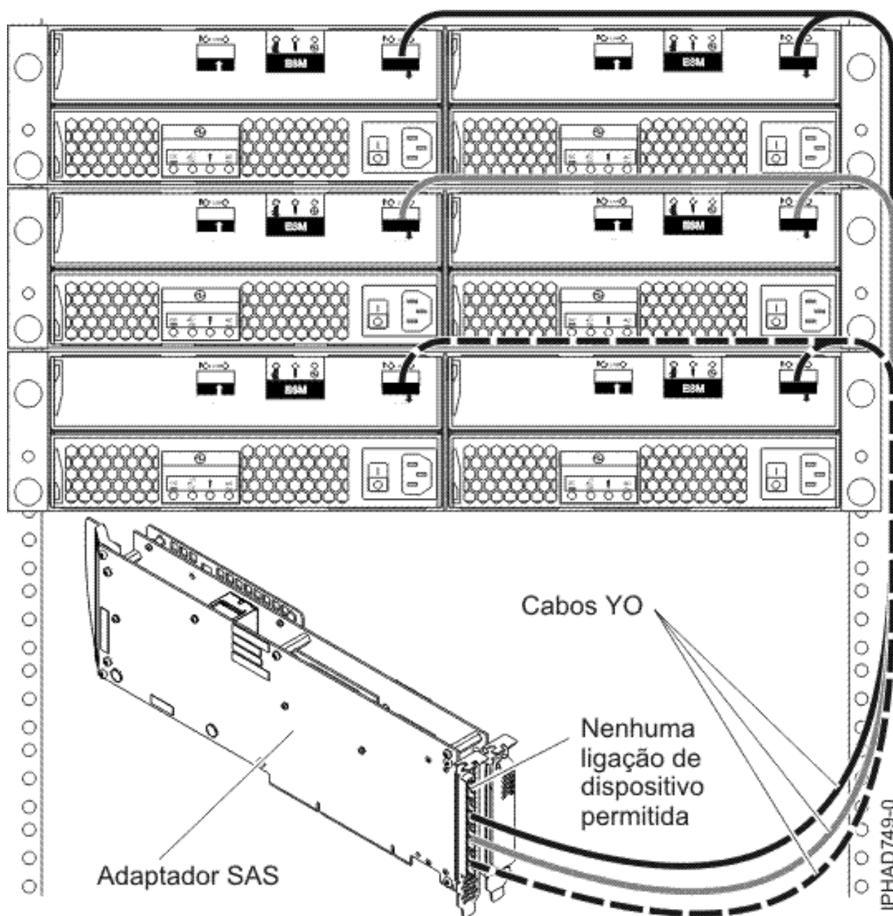
Figura 144. Adaptador SAS de três portas para gavetas de expansão de disco
