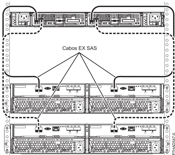
Figura 174. Ligação de duas gavetas 5887 utilizando cabos HD EX para um EDR1
