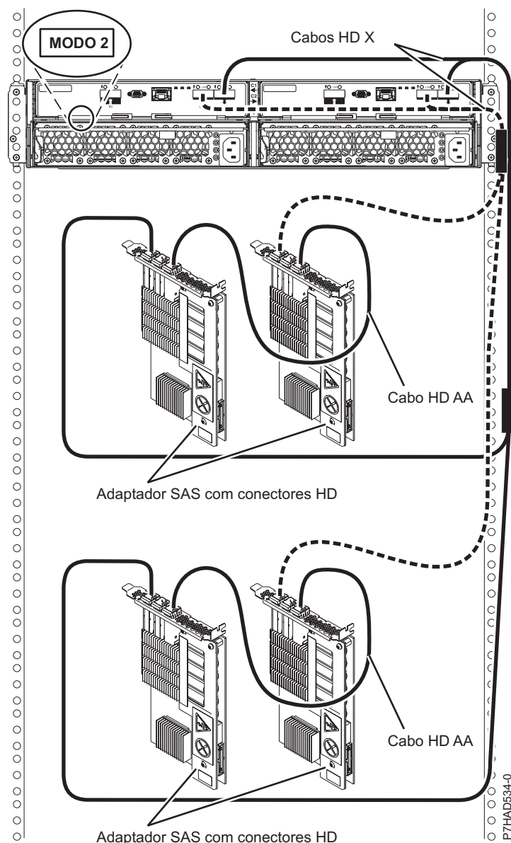
Figura 172. Ligação de modo 2 de uma gaveta 5887 utilizando conectores HD para dois pares de adaptadores SAS
