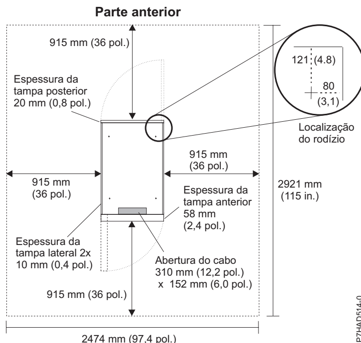
Figura 23. Áreas livres para os serviços de assistência e localização de conjuntos de unidades para bastidores 7014-T00, 7014-T42 e 0553
