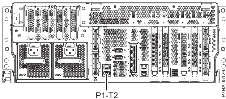
Figura 133. Vista posterior do 8202-E4B, 8202-E4C, 8202-E4D, 8205-E6B, 8205-E6C e 8205-E6D com a localização da instalação dos cabos
