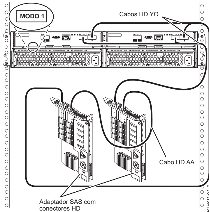
Figura 169. Ligação de modo 1 de uma gaveta 5887 para dois adaptadores SAS com conectores HD
