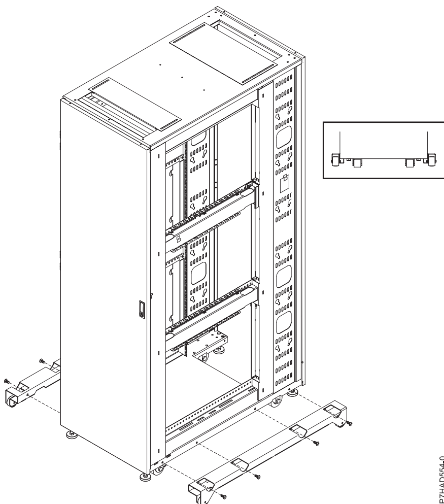
Figura 28. Localizações dos niveladores
