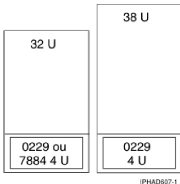
Figura 6. Código de opção 7884: 9406-520 e 9111-520 num bastidor
