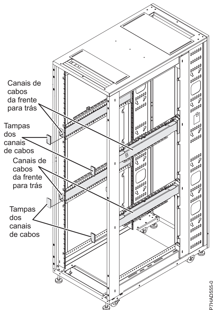
Figura 25. Cablagem no bastidor
