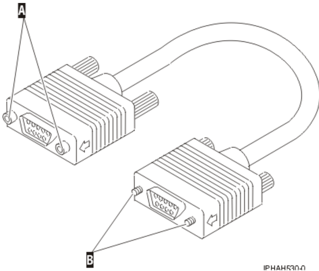
Figura 127. Conector de fonte de alimentação ininterruptível para cabo de comunicações de fonte de alimentação ininterruptível
