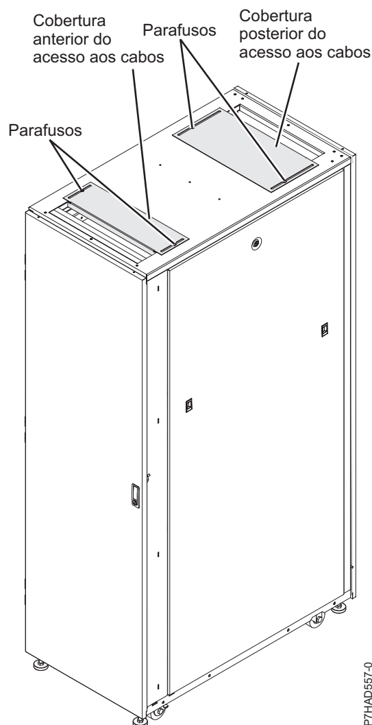
Figura 27. Tampas de acesso de cabos
