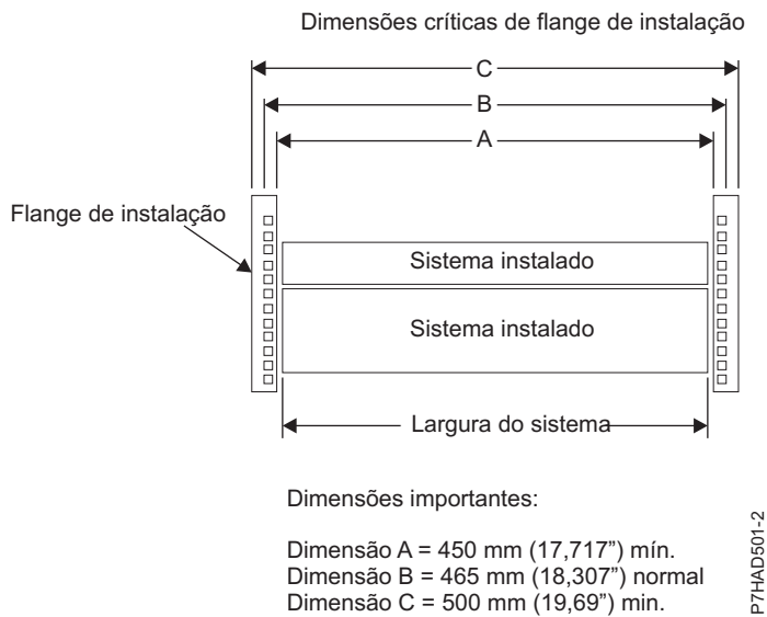
Figura 30. Dimensões das flanges de instalação críticas
