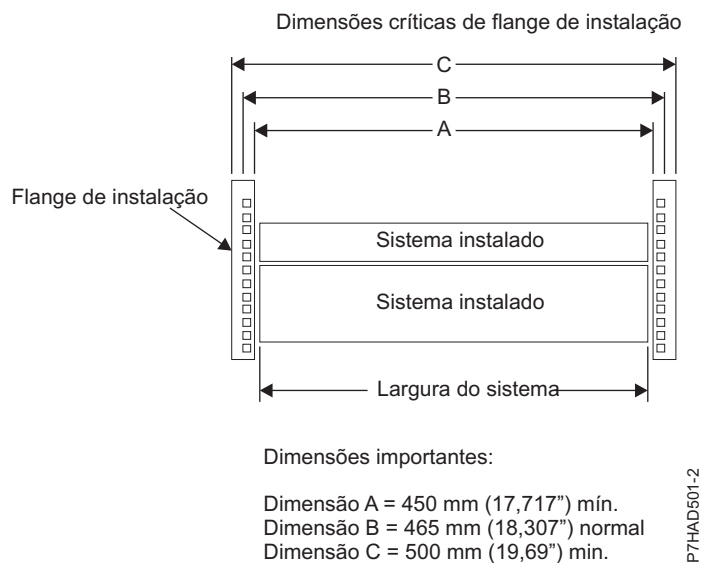
Figura 175. Dimensões das flanges de instalação críticas
