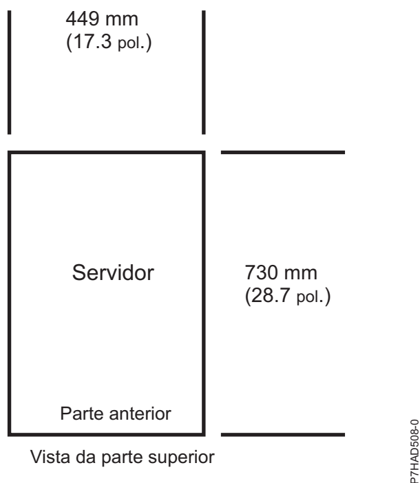
Figura 1. Vista de plano (servidores montados em bastidor) para o modelo 8202-E4B, 8202-E4C, 8202-E4D, 8205-E6B, 8205-E6C e 8205-E6D
