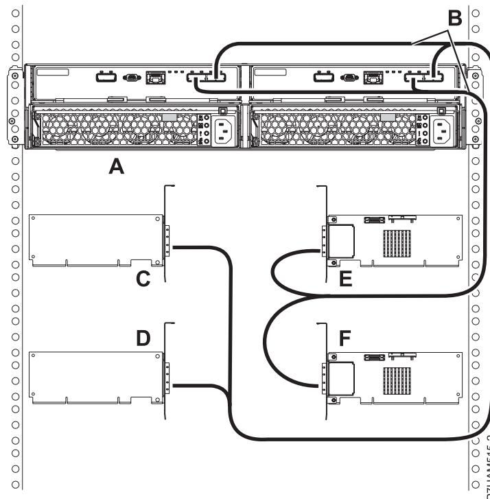
Figura 164. Ligação de modo 4 de uma gaveta 5887 utilizando cabos X para quatro adaptadores SAS únicos.
