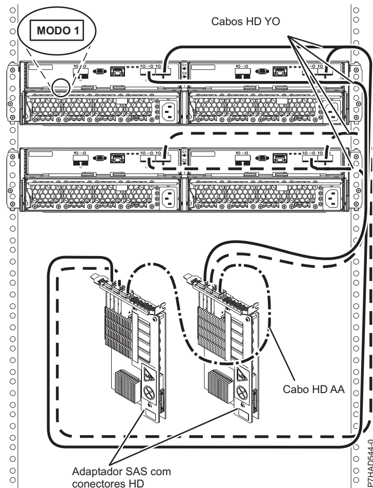
Figura 170. Ligação de modo 1 de duas gavetas 5887 utilizando conectores HD para dois adaptadores SAS
