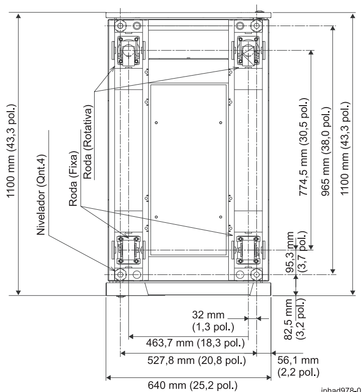
Figura 22. Localizações dos rodízios e parafusos de nivelamento
