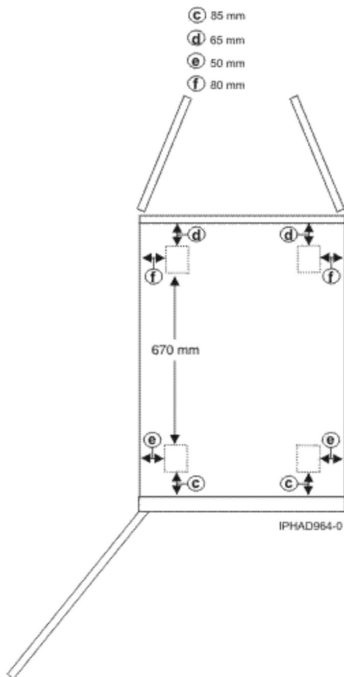
Figura 21. Localizações dos rodízios do modelo 0555 e 7014-S25
