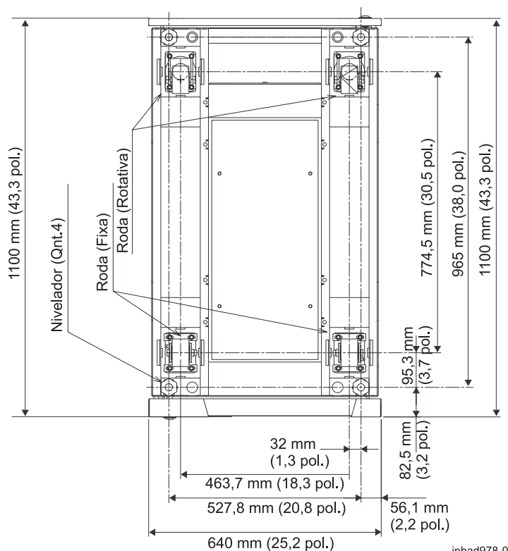
Figura 5. Localizações dos rodízios e parafusos de nivelamento
