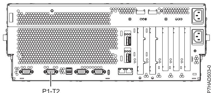
Figura 130. Vista posterior do 8233-E8B e 8236-E8C com localização da instalação dos cabos
