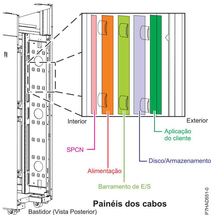
Figura 135. Lanças da ponte da gestão de cabos
