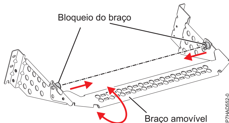
Figura 137. Braços de gestão de cabos
