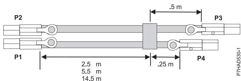
Figura 119. Comprimentos de cabos de montagem de cabo X externo SAS
