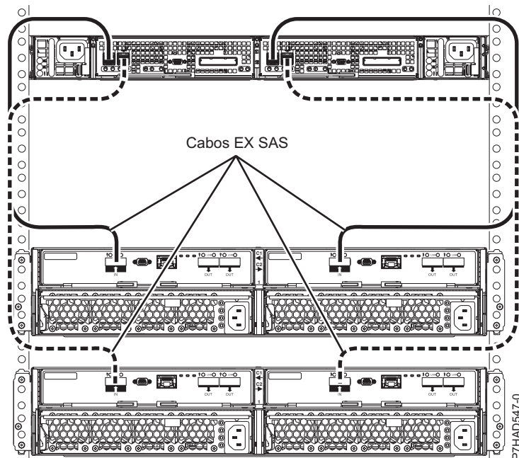
Figura 155. Ligação de duas gavetas 5887 utilizando cabos HD EX para um EDR1
