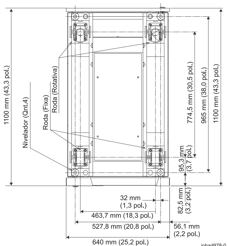
Figura 10. Localizações dos rodízios e parafusos de nivelamento
