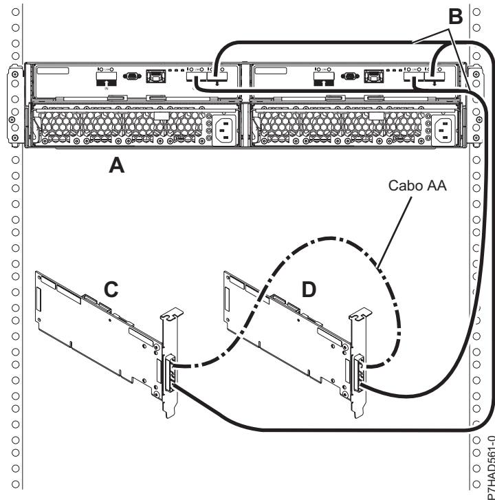
Figura 143. Ligação de modo 2 de uma gaveta 5887 utilizando cabos YO a dois adaptadores SAS únicos
