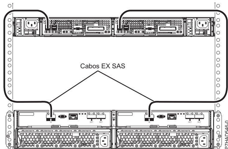
Figura 154. Ligação de uma gaveta 5887 utilizando cabos HD EX para um EDR1
