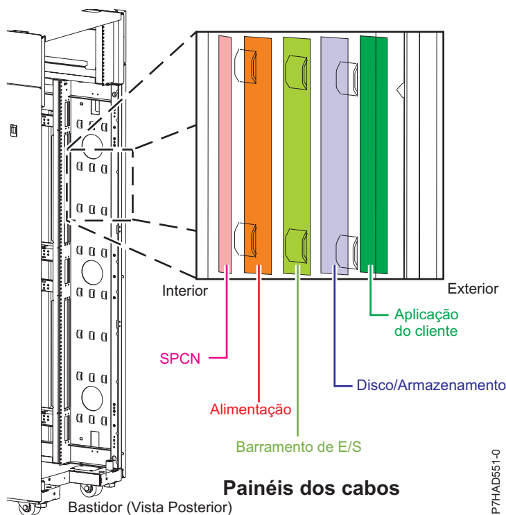
Figura 116. Lanças da ponte da gestão de cabos
