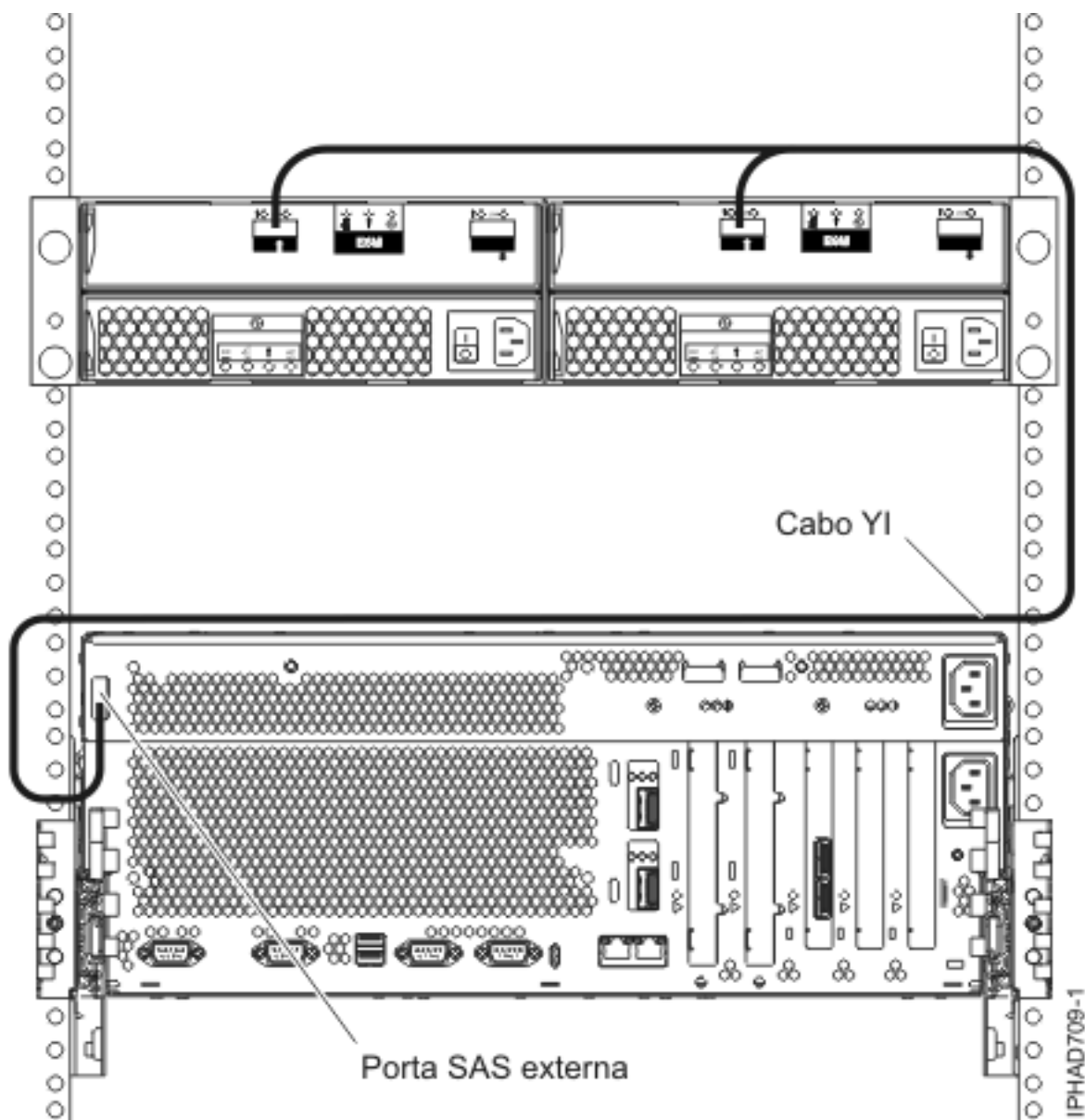
Figura 128. Porta de adaptador SAS externa ao sistema para uma gaveta de expansão de disco
