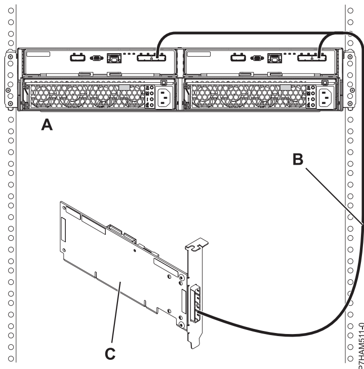
Figura 141. Ligação de modo 1 de uma gaveta 5887 utilizando um cabo YO para um adaptador SAS único
