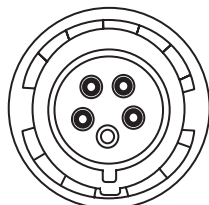
Figura 19. Saída de pinos do conector
