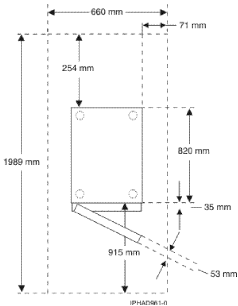
Figura 5. Vista de plano do modelo 0554 e 7014-S11
