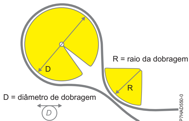
Figura 117. Raio da dobragem dos cabos
