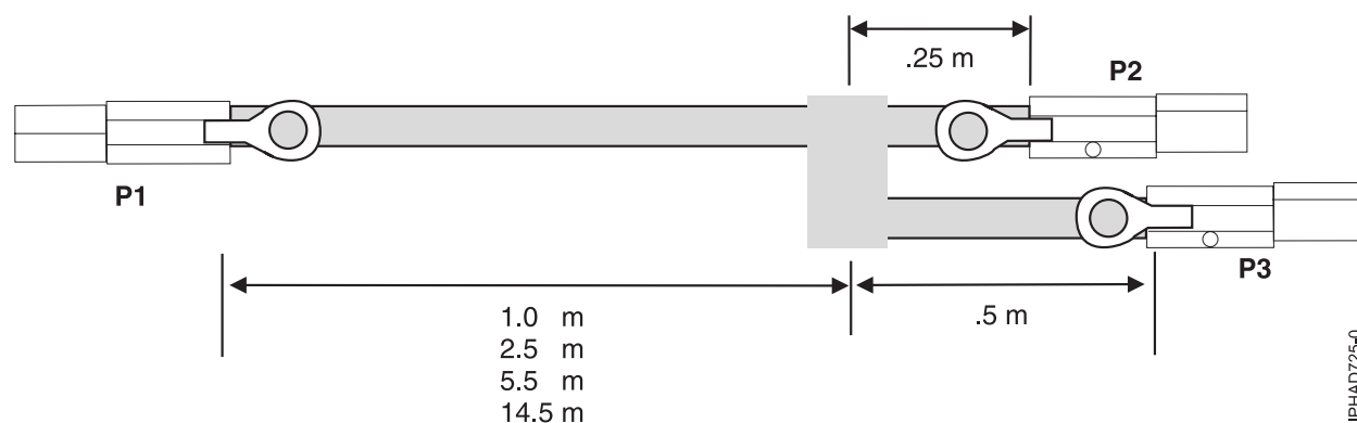
Figura 120. Comprimentos de cabo de montagem de cabo YO externo SAS
