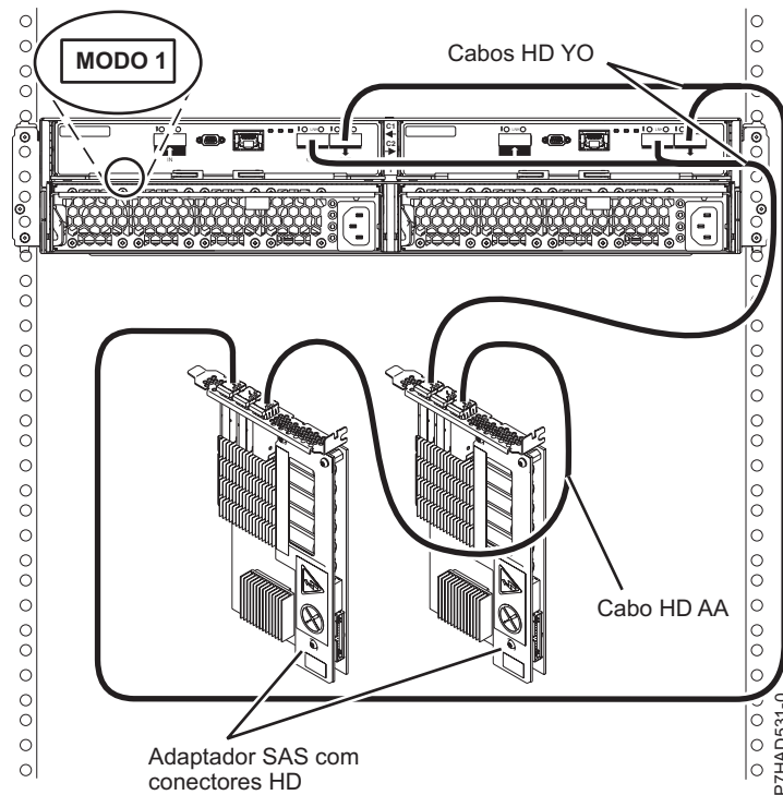
Figura 150. Ligação de modo 1 de uma gaveta 5887 para dois adaptadores SAS com conectores HD
