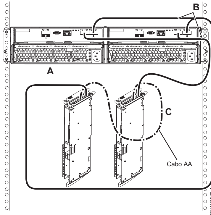
Figura 149. Ligação de modo 1 de uma gaveta 5887 utilizando cabos YO para adaptadores SAS duplos
