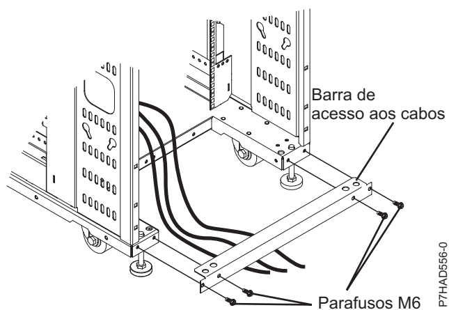
Figura 14. Barra de acesso de cabos
