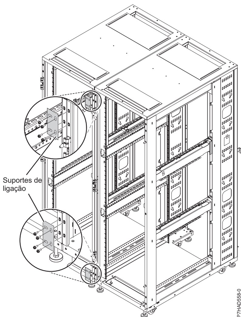
Figura 17. Suportes de ligação
