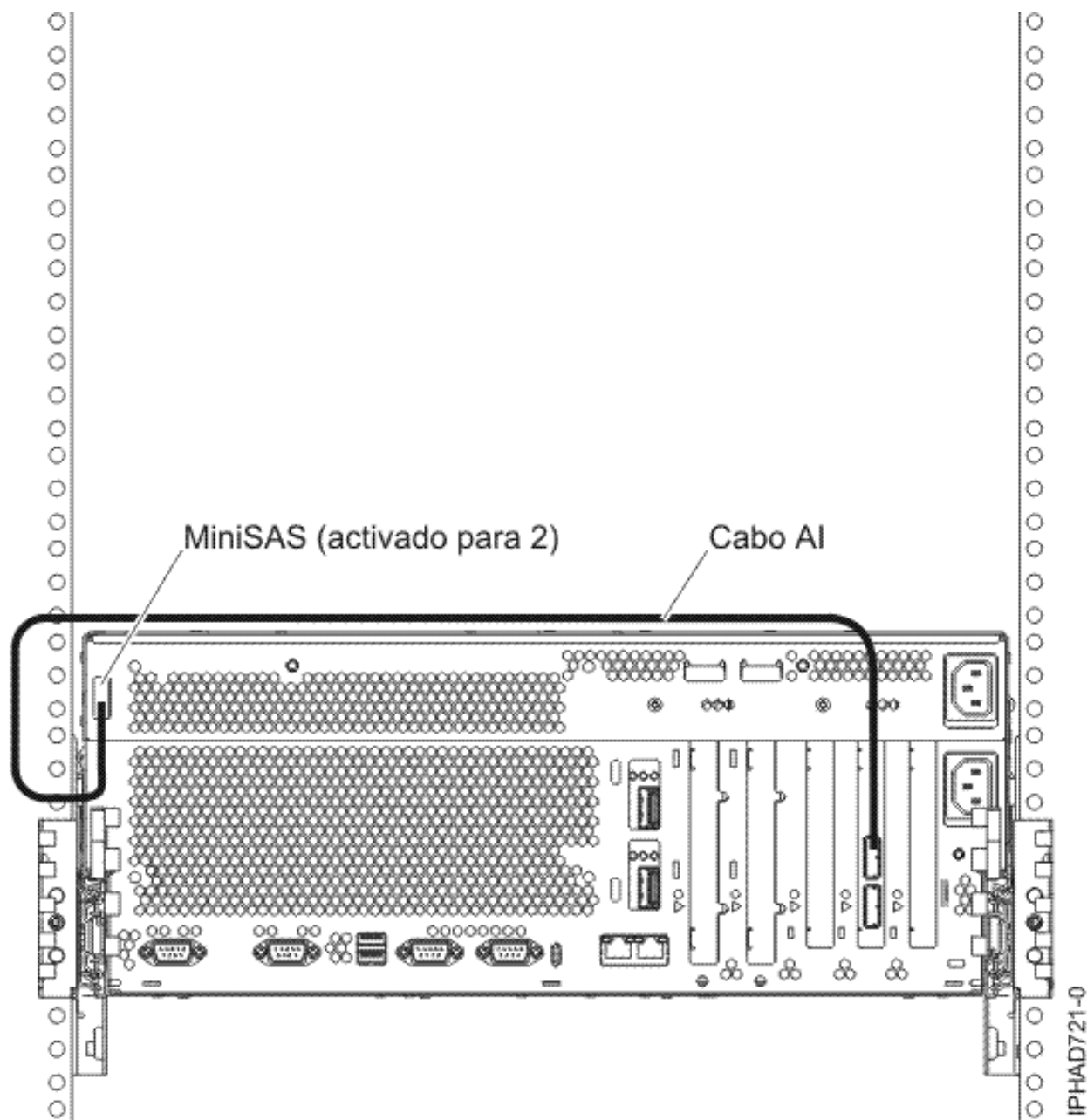
Figura 129. Adaptador SAS a ranhuras de disco SAS internas através de porta SAS externa do sistema
