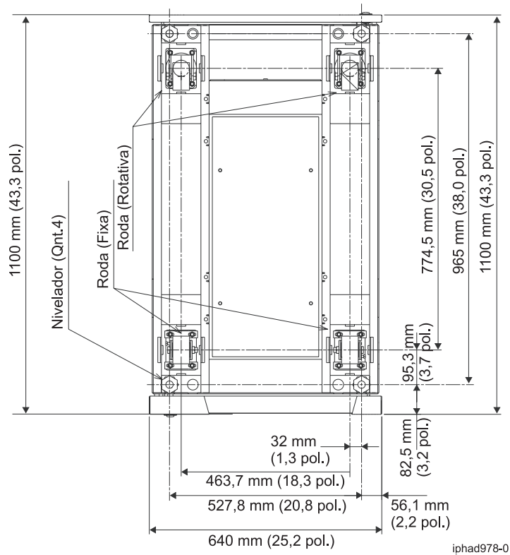
Figura 3. Localizações dos rodízios e parafusos de nivelamento
