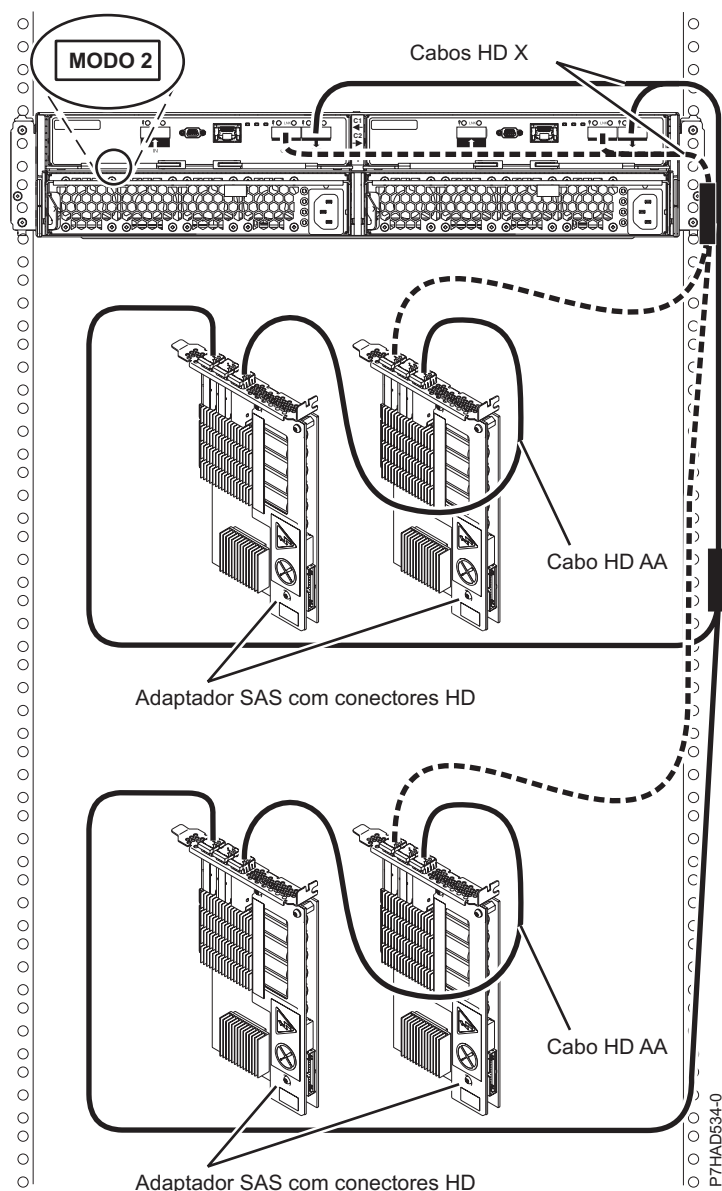
Figura 153. Ligação de modo 2 de uma gaveta 5887 utilizando conectores HD para dois pares de adaptadores SAS
