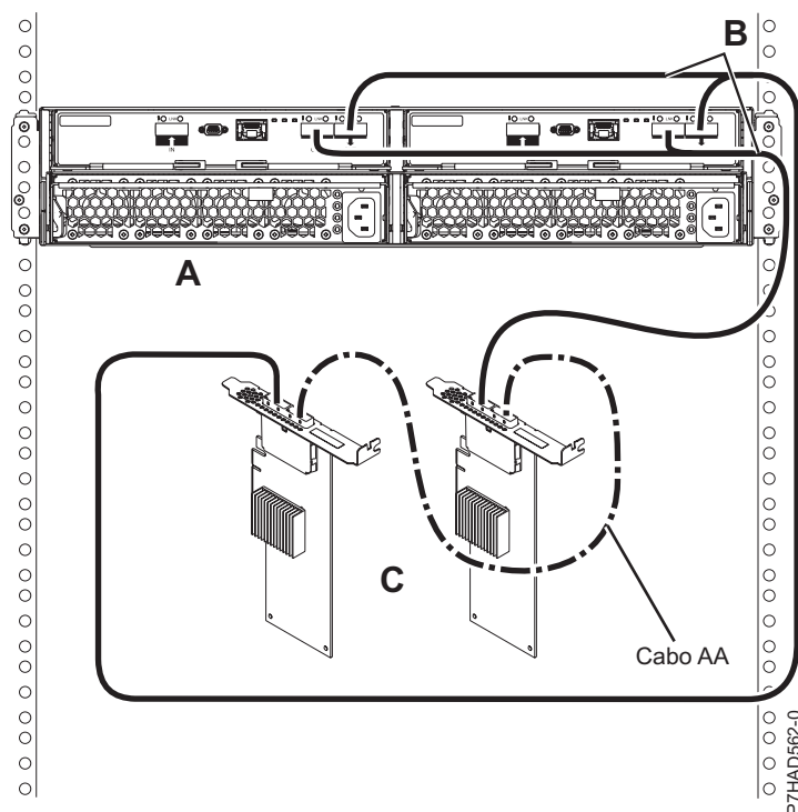
Figura 142. Ligação de modo 1 de uma gaveta 5887 utilizando cabos YO para adaptadores SAS duplos
