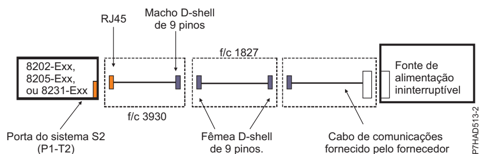
Figura 115. Ligações da fonte de alimentação ininterruptível para o 8246-L1C, 8246-L1S, 8246-L2C, e 8246-L2S
