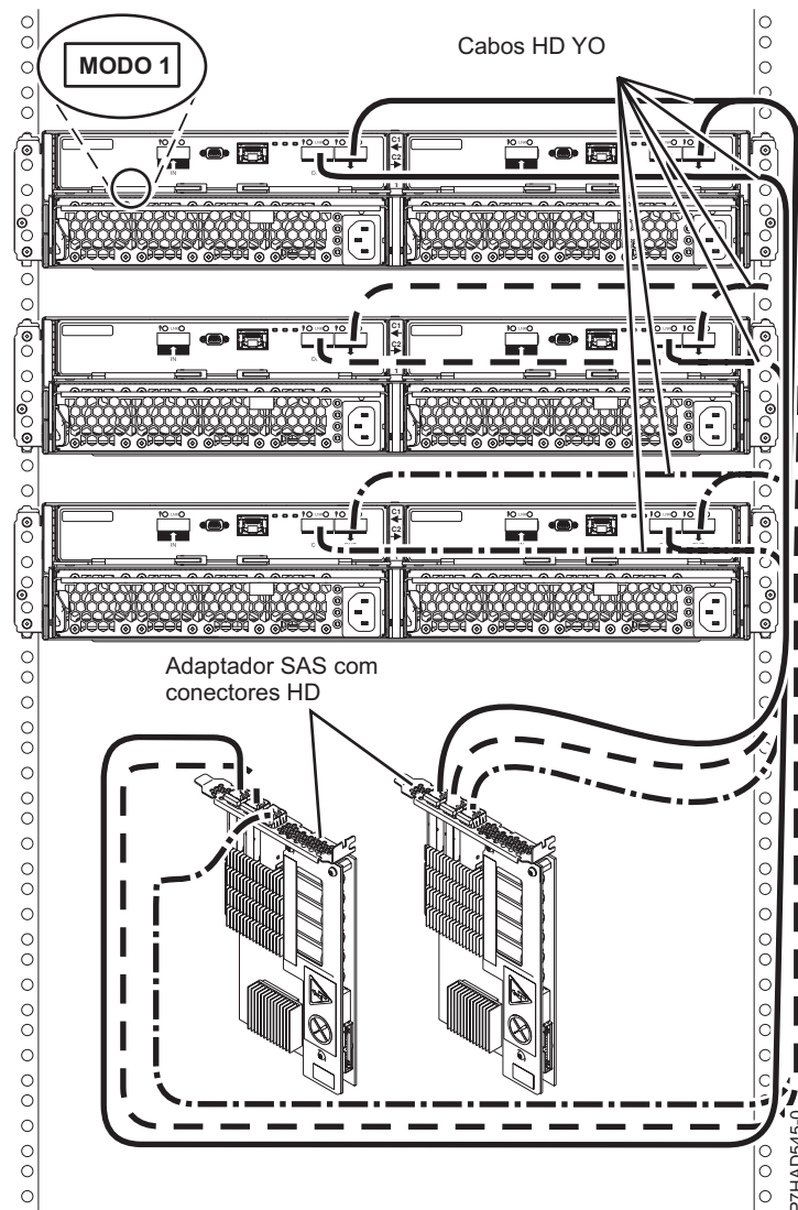
Figura 152. Ligação de modo 1 de três gavetas 5887 para dois adaptadores SAS com conectores HD
