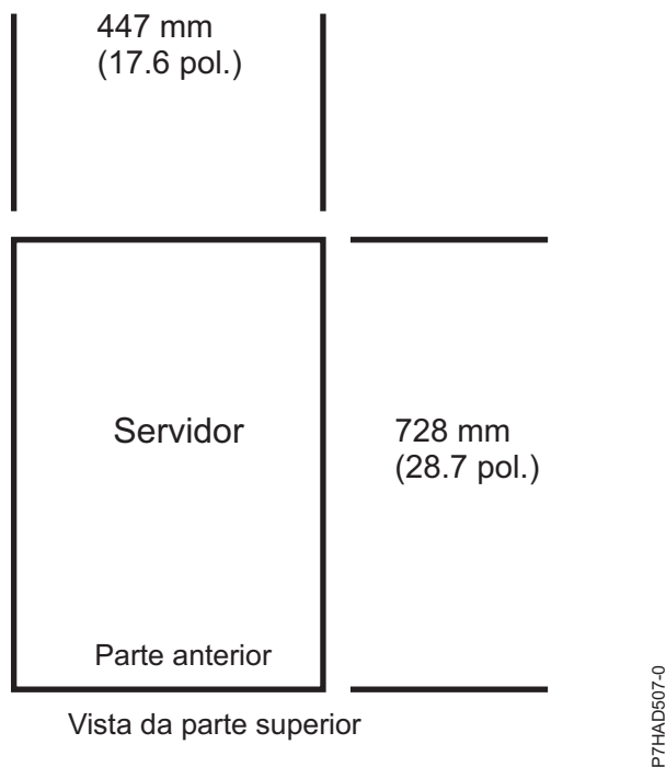
Figura 1. Vista de planeamento do modelo 8246-L1C, 8246-L1D, 8246-L1S, 8246-L1T, 8246-L2C, 8246-L2D, 8246-L2S, e 8246-L2T (servidor montado em bastidor)
