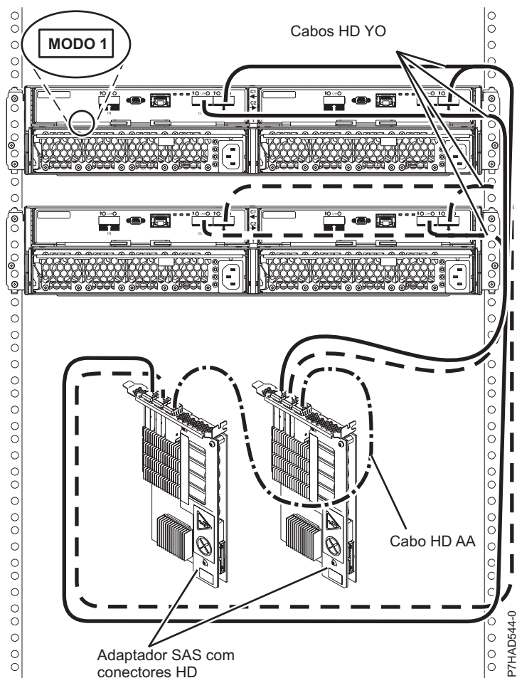
Figura 151. Ligação de modo 1 de duas gavetas 5887 utilizando conectores HD para dois adaptadores SAS
