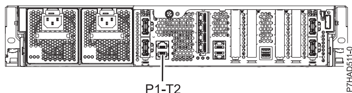
Figura 114. Vista posterior do , 8246-L1C, 8246-L1D, 8246-L1S, 8246-L1T, 8246-L2C, 8246-L2D, 8246-L2S, e 8246-L2T com a localização da instalação dos cabos
