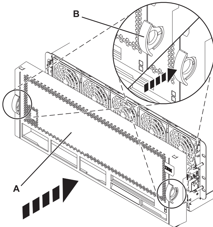
Figura 13. Instalar a tampa anterior
