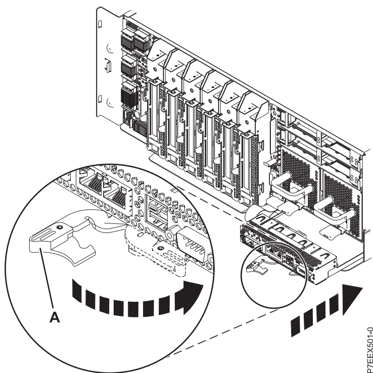
Figura 2. Instalar a placa de multifunções integrada num modelo montado em bastidor para 8412-EAD, 9117-MMC, 9117-MMD, 9179-MHC, ou 9179-MHD
