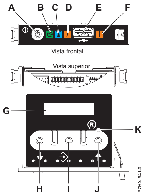
Figura 3. Painel de controlo
