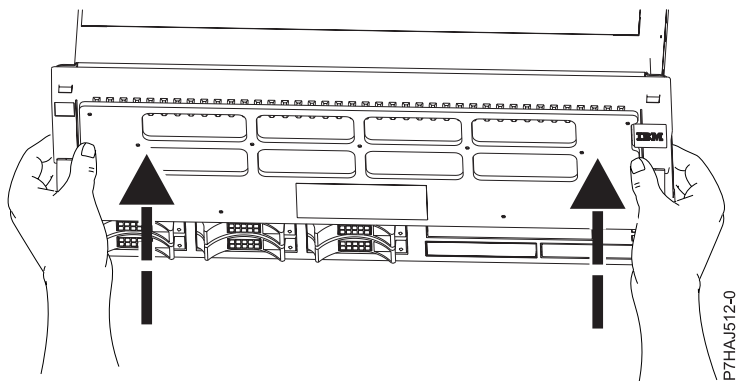
Figura 9. Utilização da ferramenta de remoção da tampa
