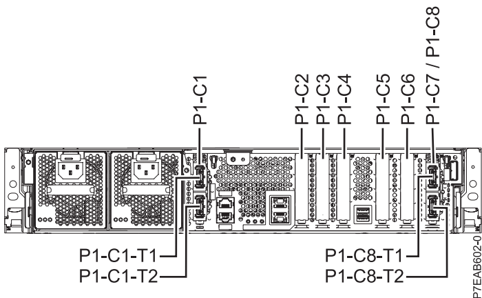
Figura 1. Vista posterior do sistema com códigos de localização
