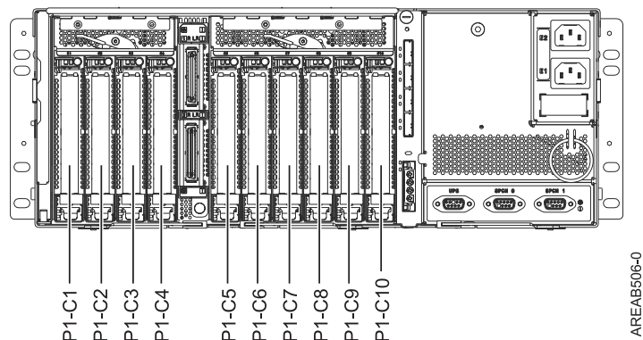
Figura 3. Vista posterior. Esta figura apresenta a vista posterior da unidade de expansão.
