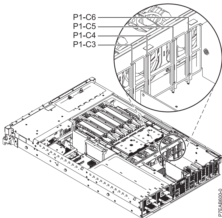
Figura 1. Vista posterior do sistema 8231-E2B com os códigos de localização das ranhuras PCI
