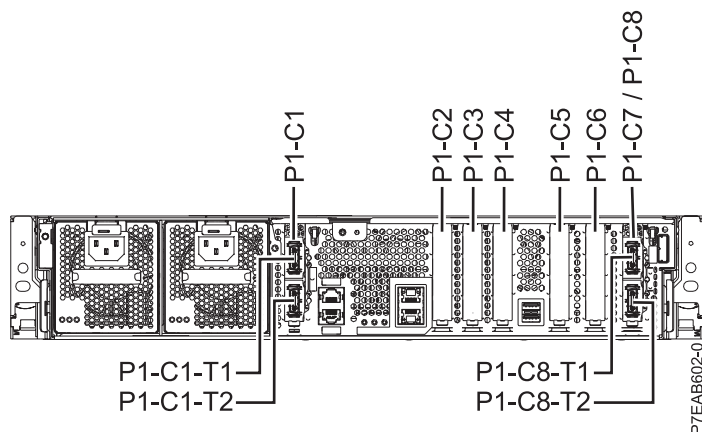
Figura 2. Vista posterior do sistema com códigos de localização
