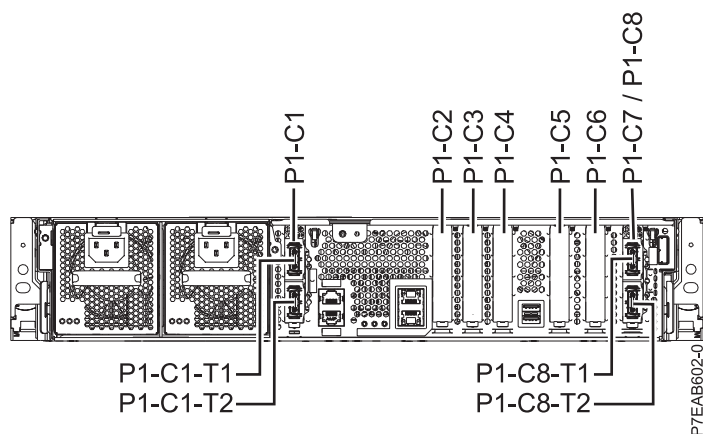
Figura 3. Vista posterior do sistema com códigos de localização
